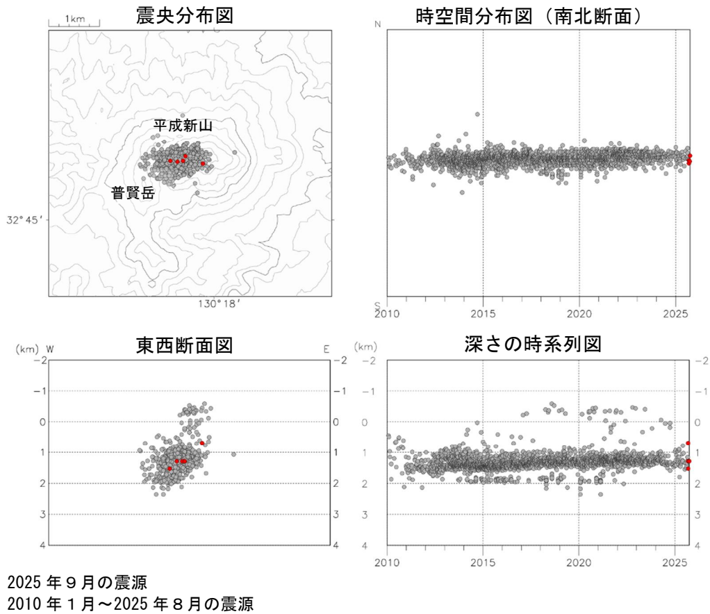
図4 雲仙岳 震源分布図 ①広域図 ②狭域図（2010年1月～2025年9月）
