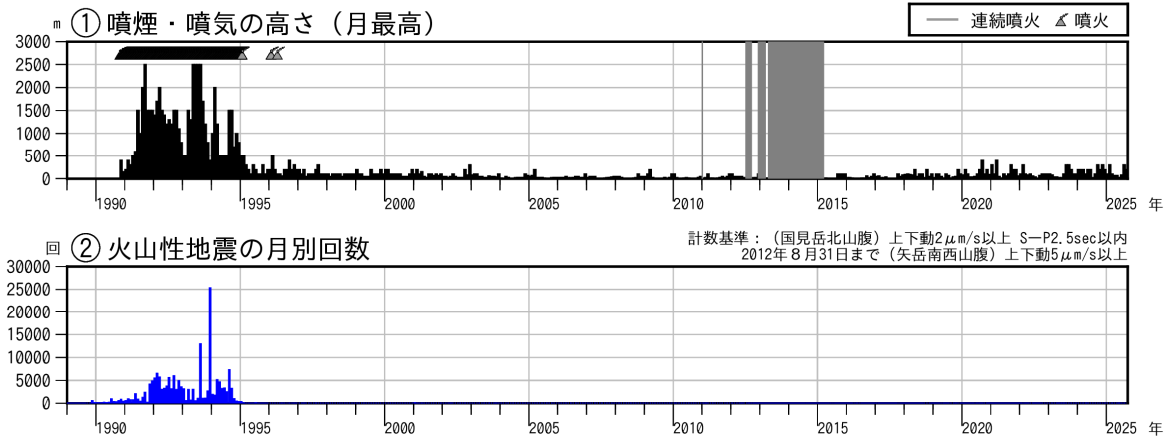
図2 雲仙岳 長期の火山活動経過図（1989年1月～2025年9月）
