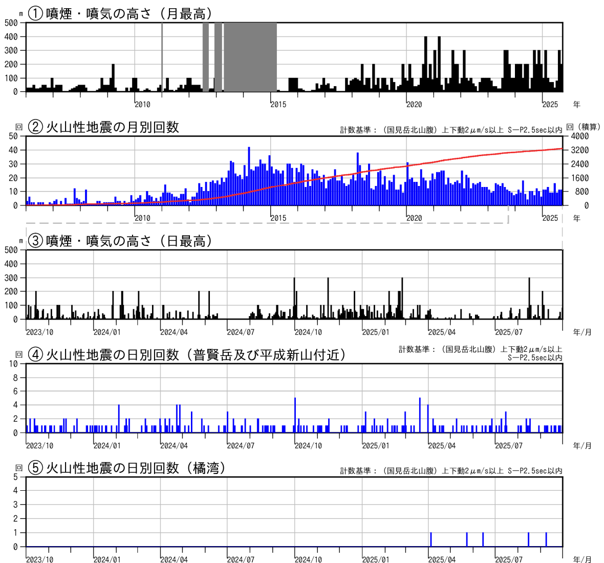
図3 雲仙岳 火山活動経過図（2006年1月～2025年9月）
