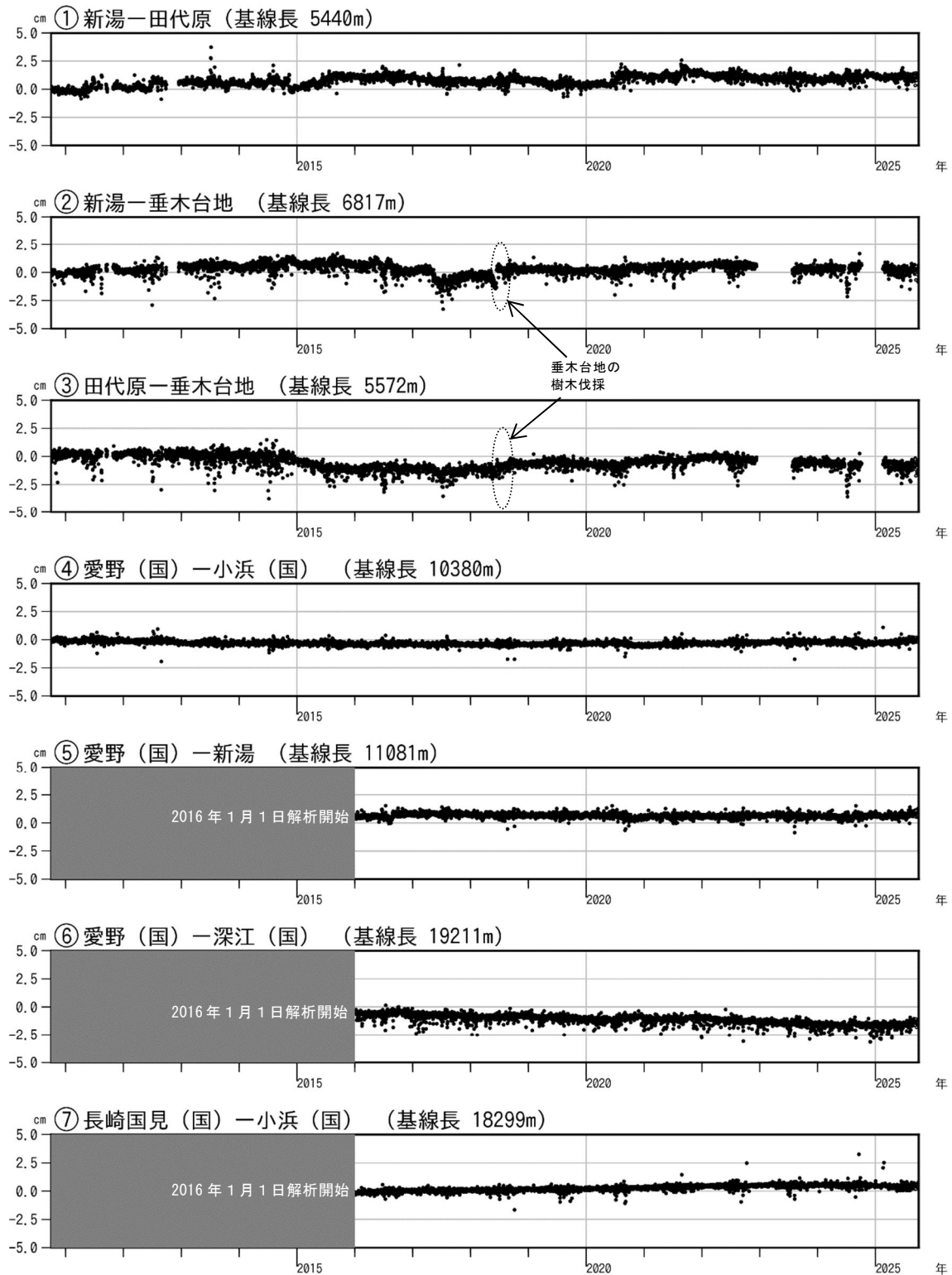
図5 雲仙岳 GNSS連続観測による基線長変化（2010年10月～2025年9月）
