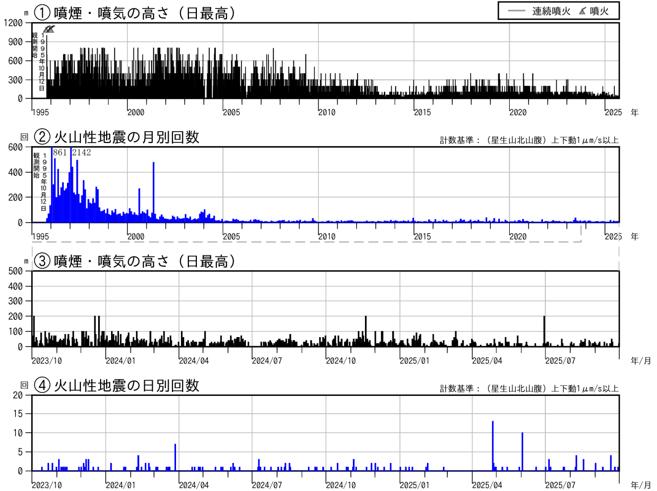
図2 九重山 火山活動経過図（1995年1月～2025年9月）
