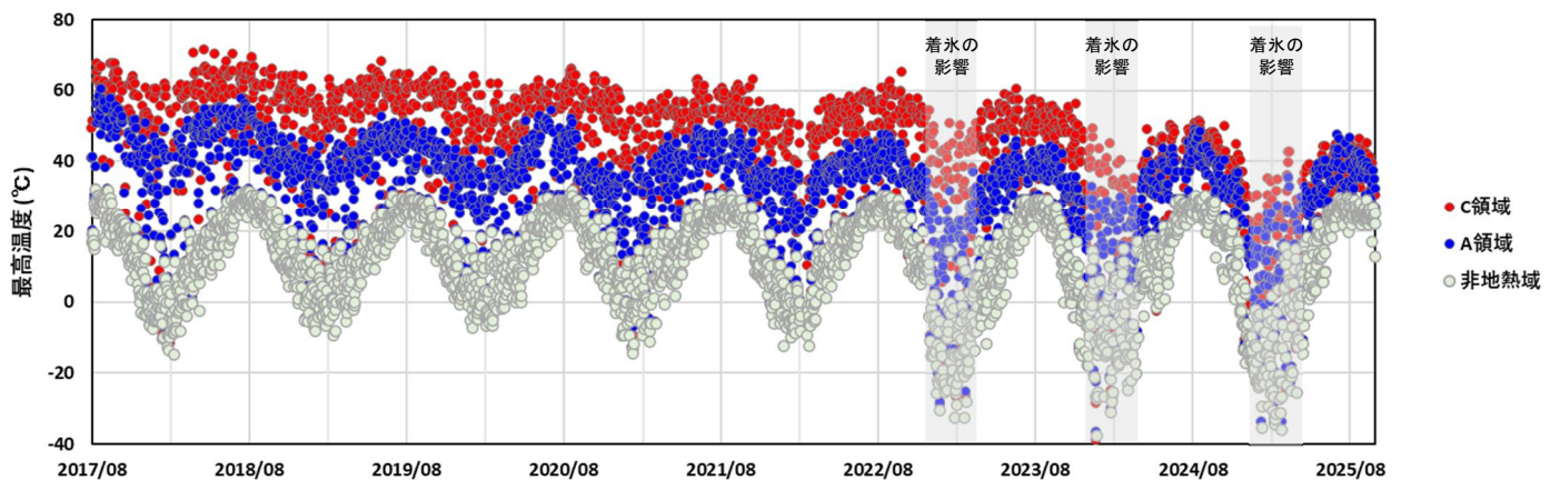
図 1-2 九重山 星生山北尾根の赤外熱映像装置による日別最高温度（2017 年 8 月～2025 年 9 月）
