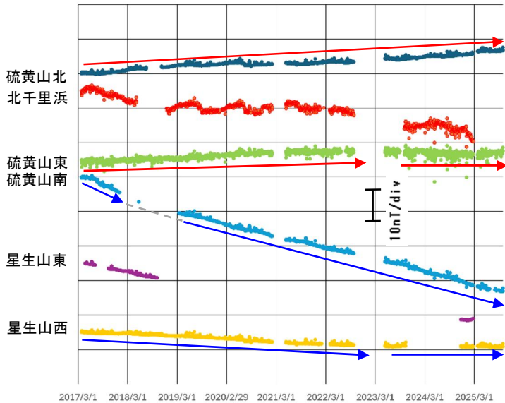
図 4-1 九重山 連続観測による全磁力の変化 (2017年3月～2025年9月)
