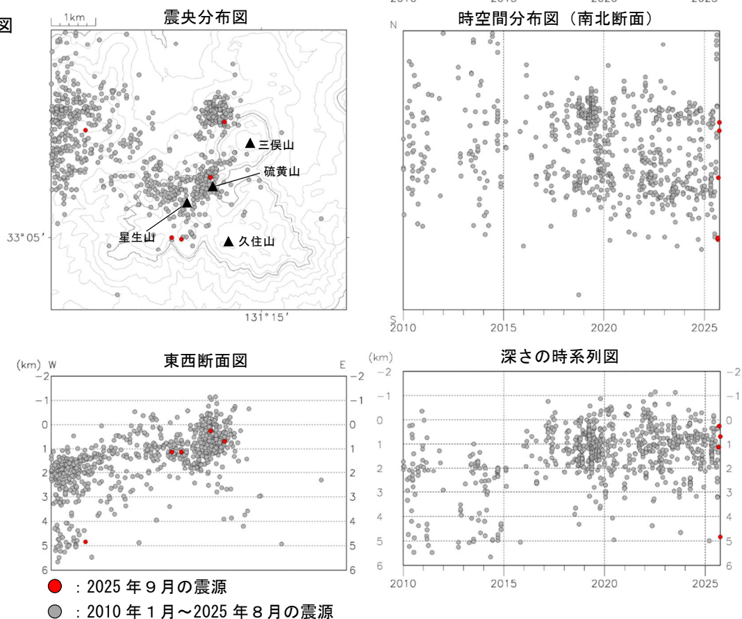
図3 九重山 震源分布図 ①広域図 ②狭域図（2010年1月～2025年9月）
