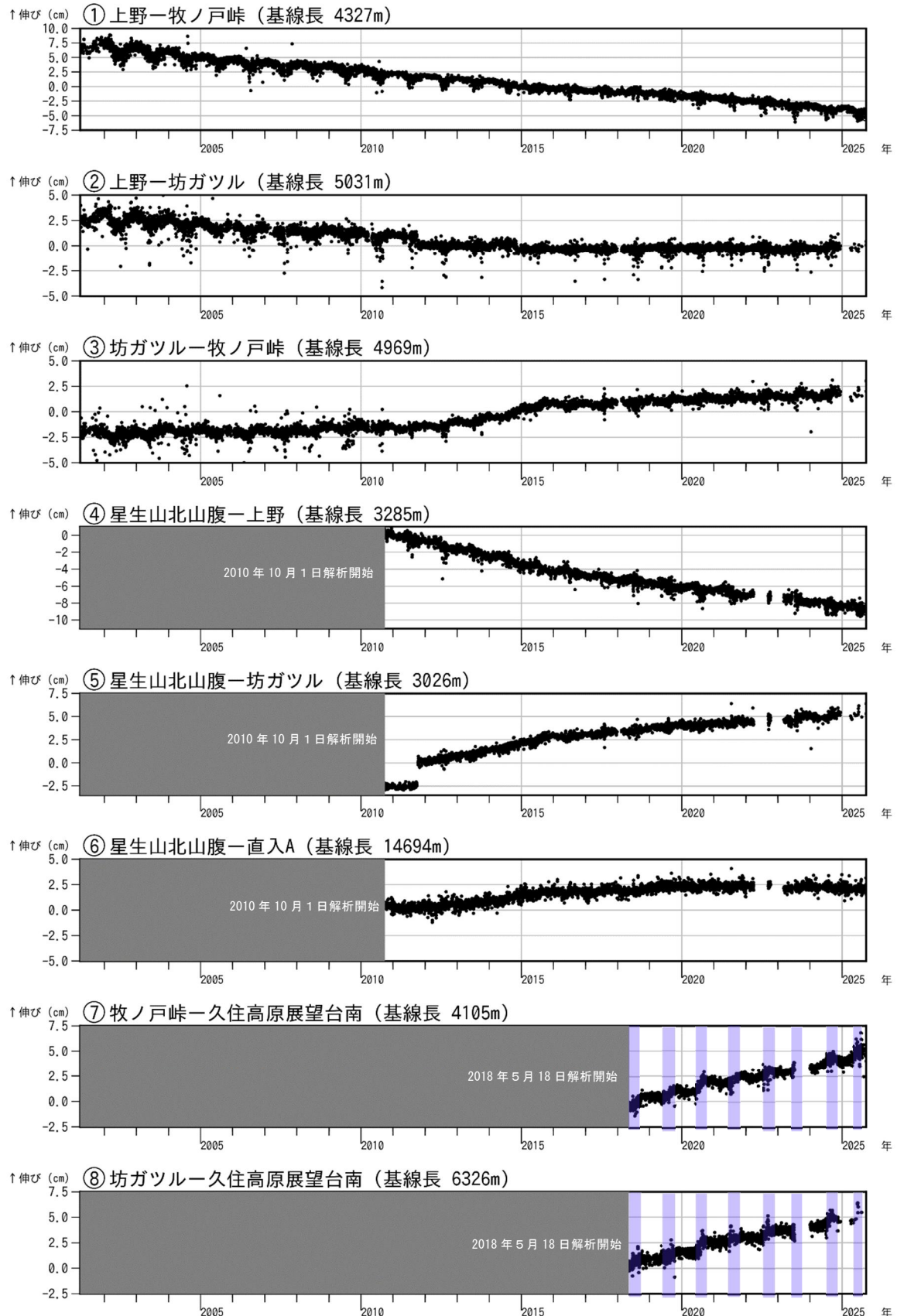
図5 九重山 GNSS 連続観測による基線長変化（2001年4月～2025年9月）
