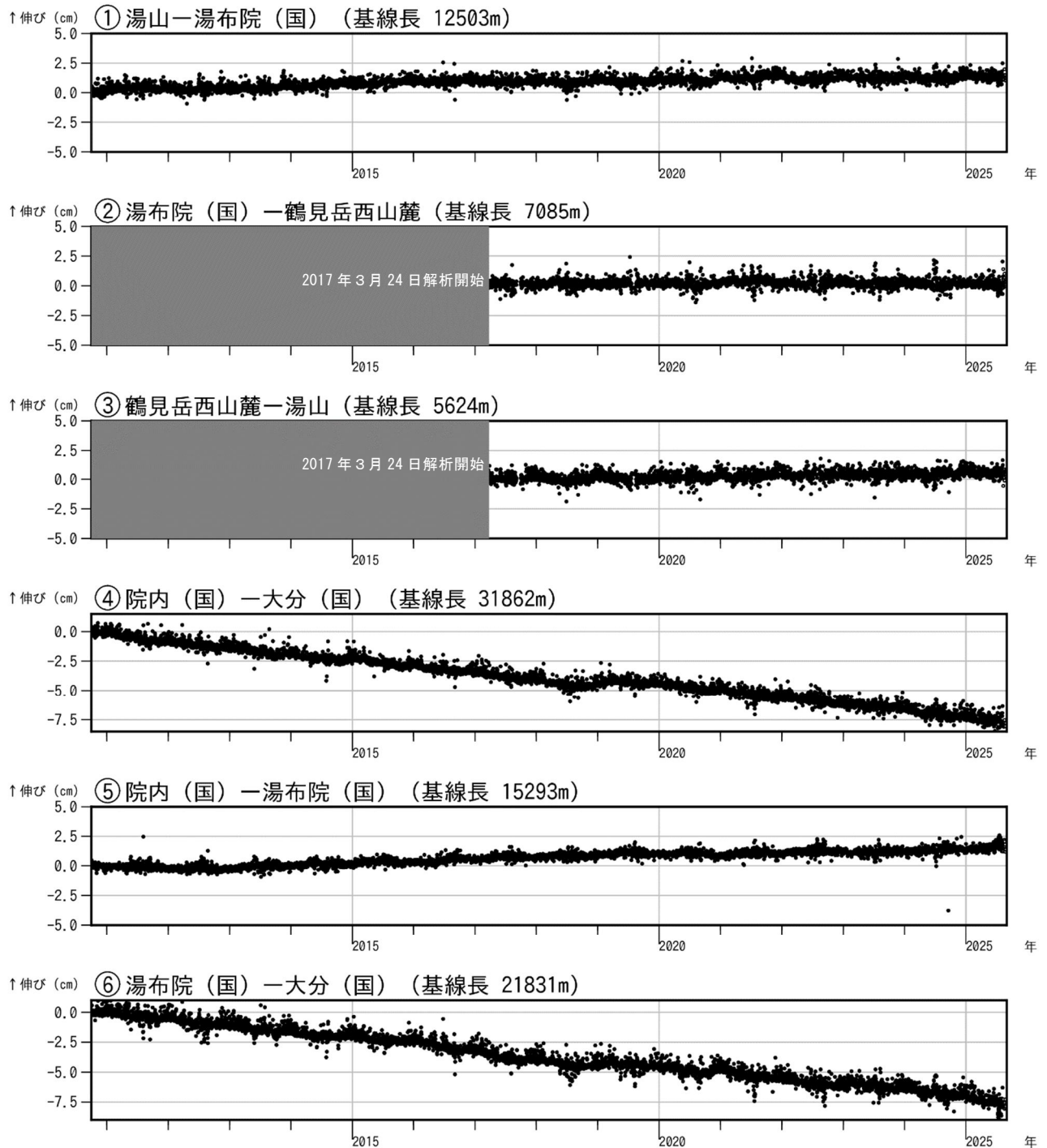
図5 鶴見岳・伽藍岳 GNSS連続観測による基線長変化（2010年10月～2025年8月）
