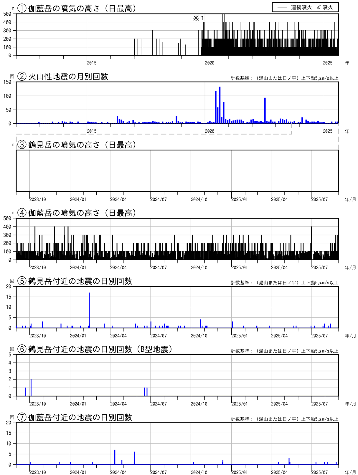
図3 鶴見岳・伽藍岳 火山活動経過図（2012年1月～2025年8月）
