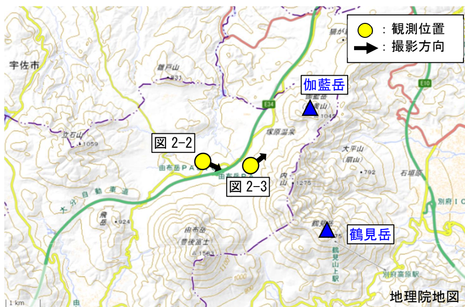
図 2-1 鶴見岳・伽藍岳 26日に実施した機上観測位置及び撮影方向
