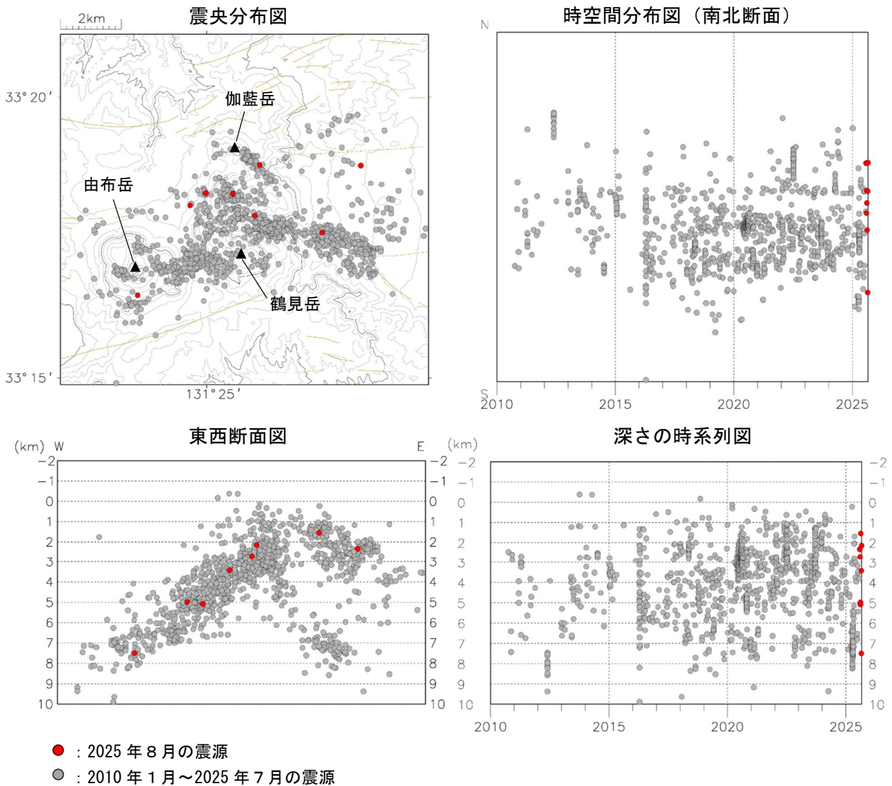
図 4 鶴見岳・伽藍岳 震源分布図（2010 年 1 月～2025 年 8 月）
