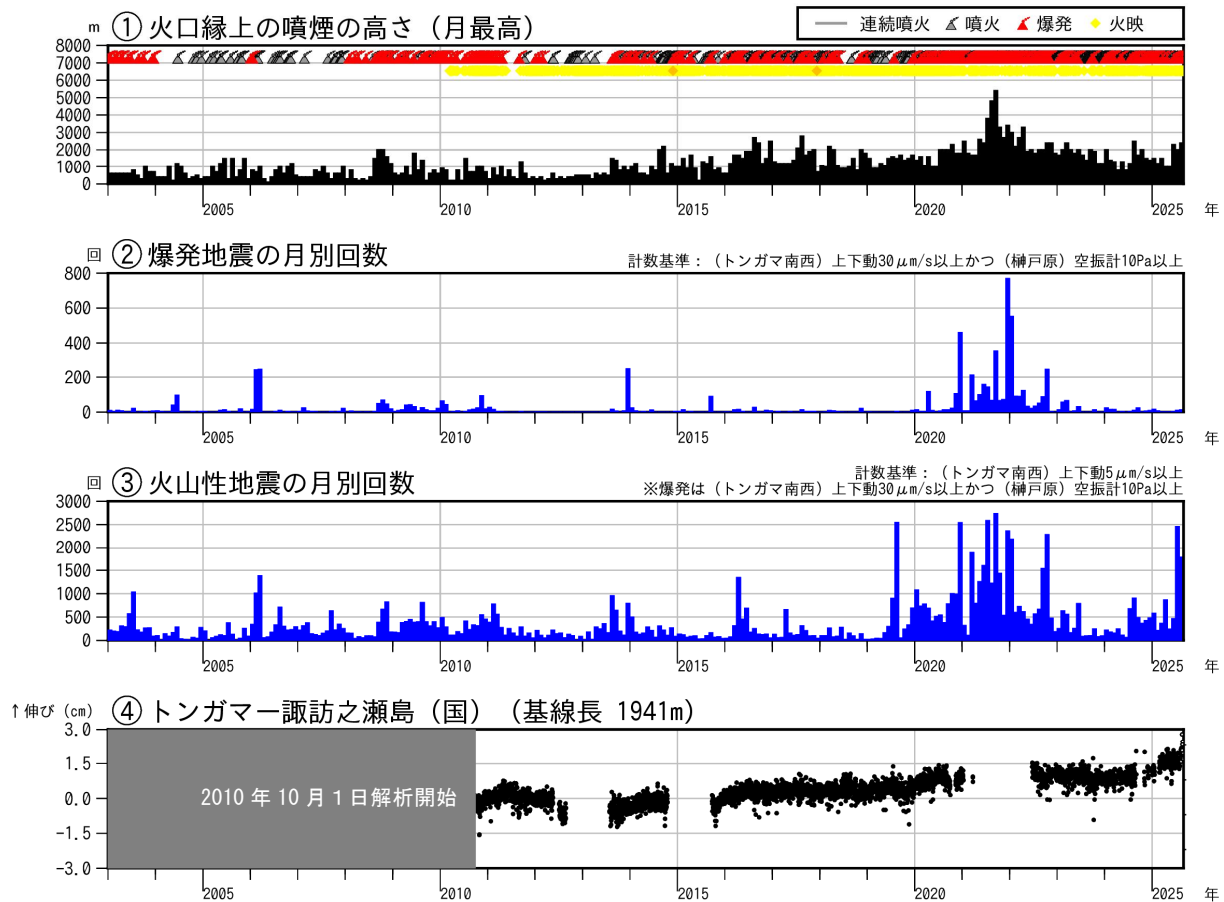
図2 諏訪之瀬島 長期の火山活動経過図（2003年1月～2025年8月）
