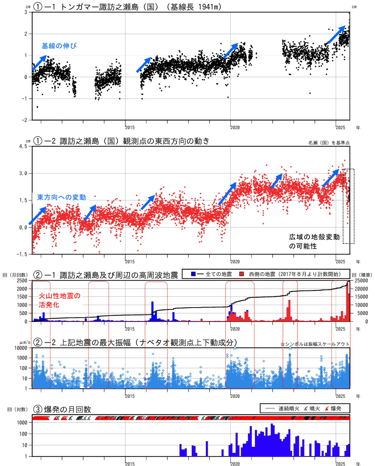
図6 諏訪之瀬島 GNSS連続観測と周辺の火山性地震（2010年8月～2025年8月）
