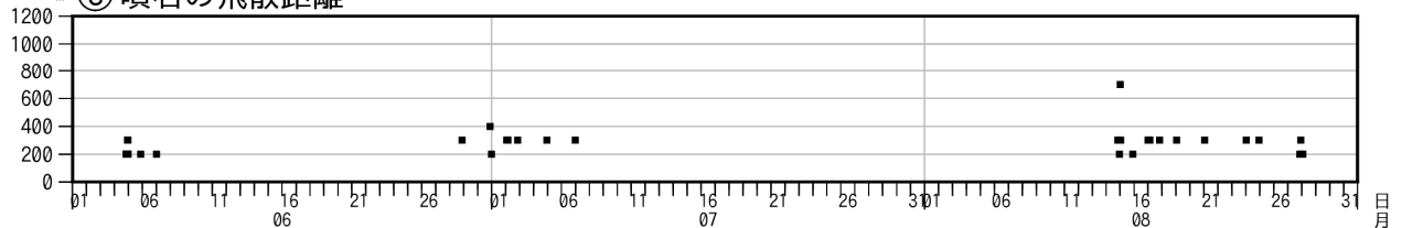
図5 諏訪之瀬島 ナベタオ観測点の傾斜変動と噴火活動（2025年6月～8月）
