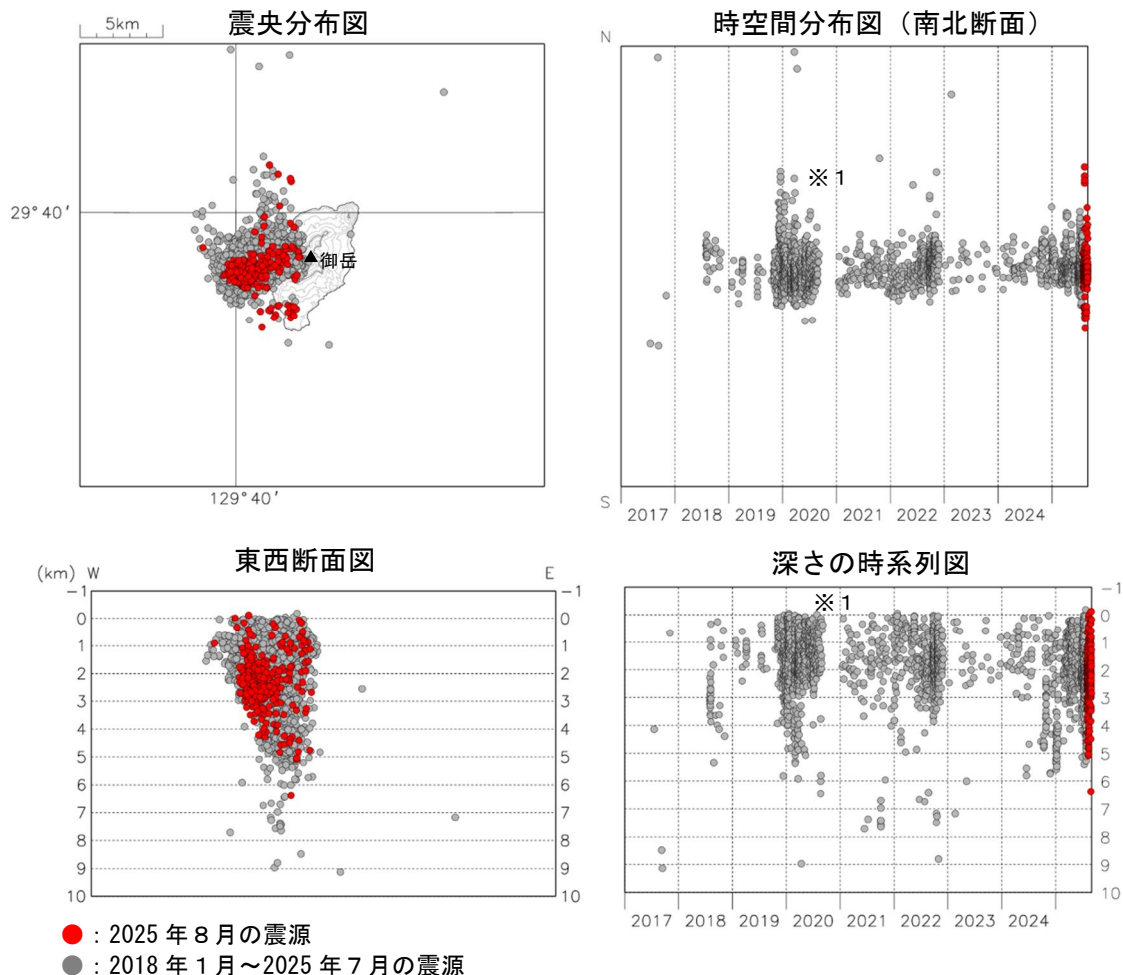
図4 諏訪之瀬島 震源分布図（2018年1月～2025年8月）
