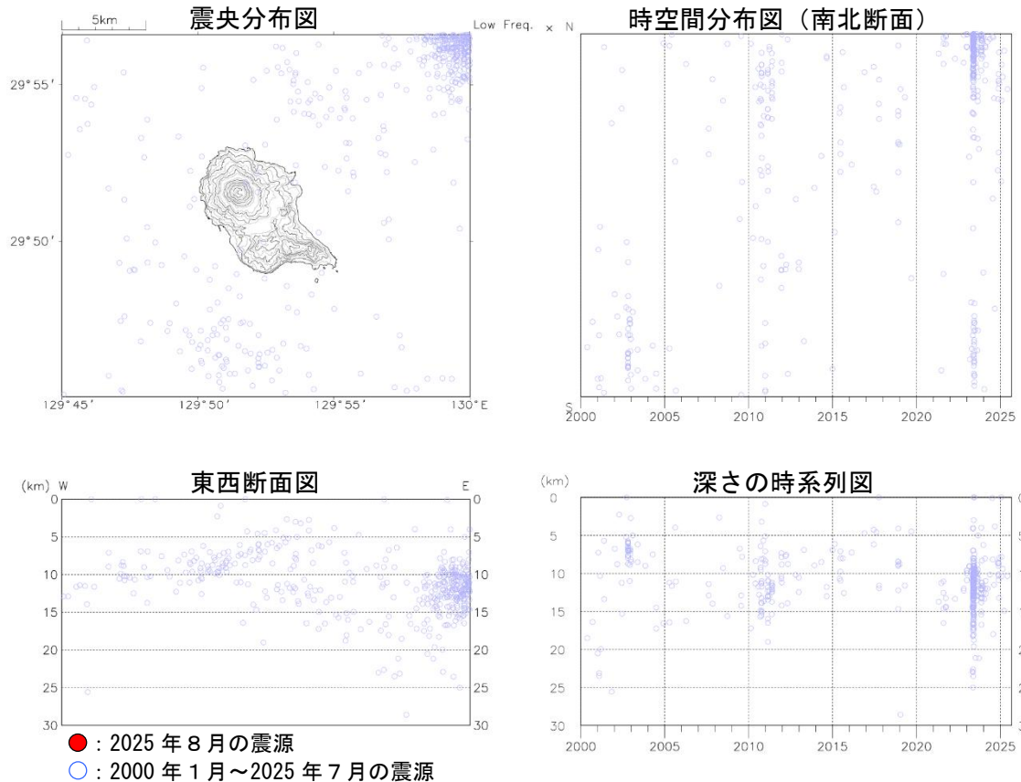
図3 中之島 中之島周辺の震源分布図（2000年1月～2025年8月）
