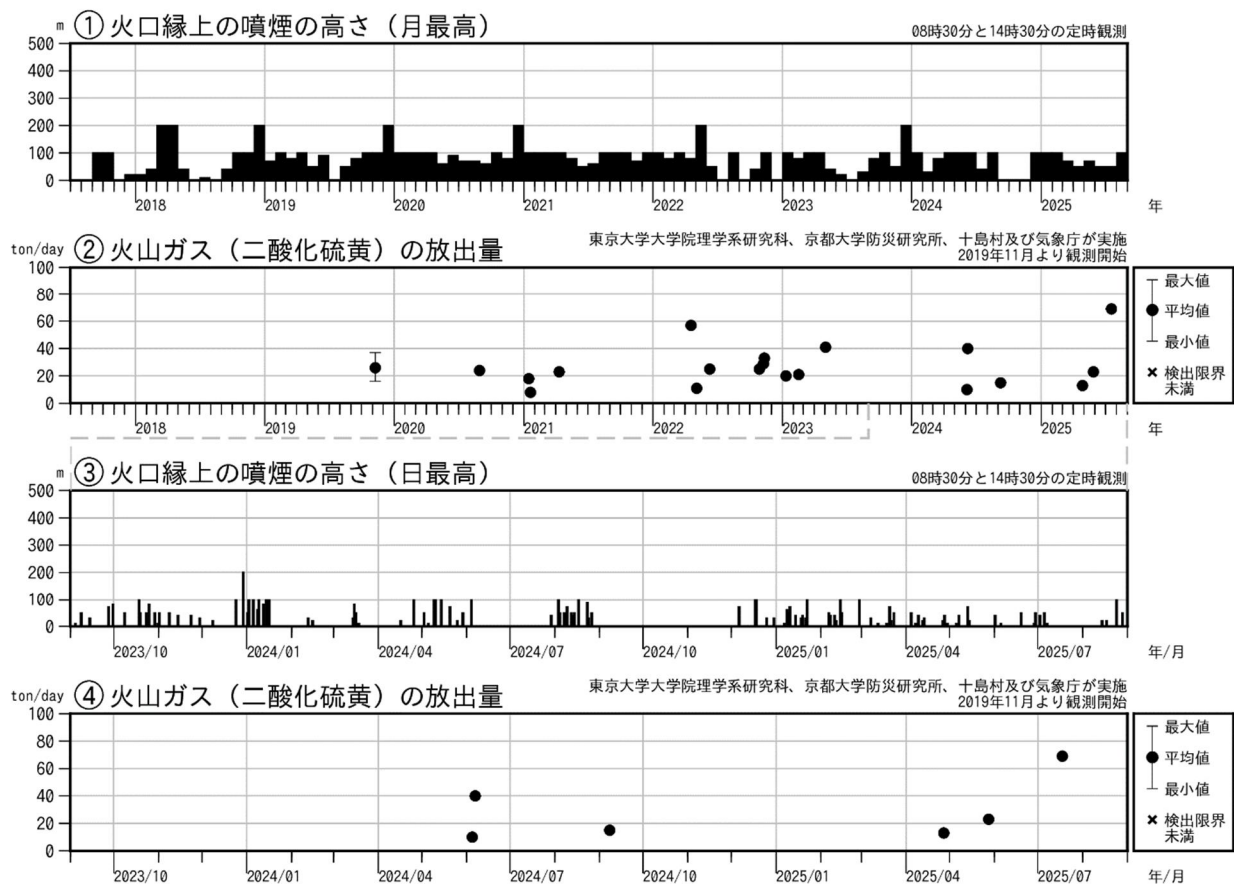
図2 中之島 火山活動経過図（2017年7月～2025年8月）
