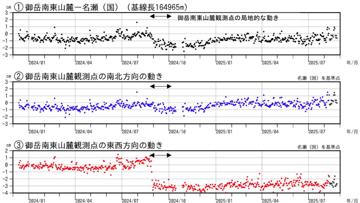
図4 中之島 GNSS連続観測（2023年12月～2025年8月）
