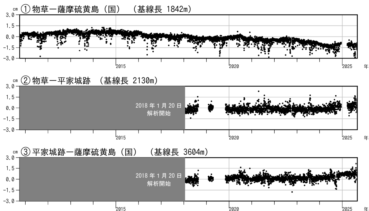
図5 薩摩硫黄島 GNSS連続観測による基線長変化(2010年10月～2025年8月)
