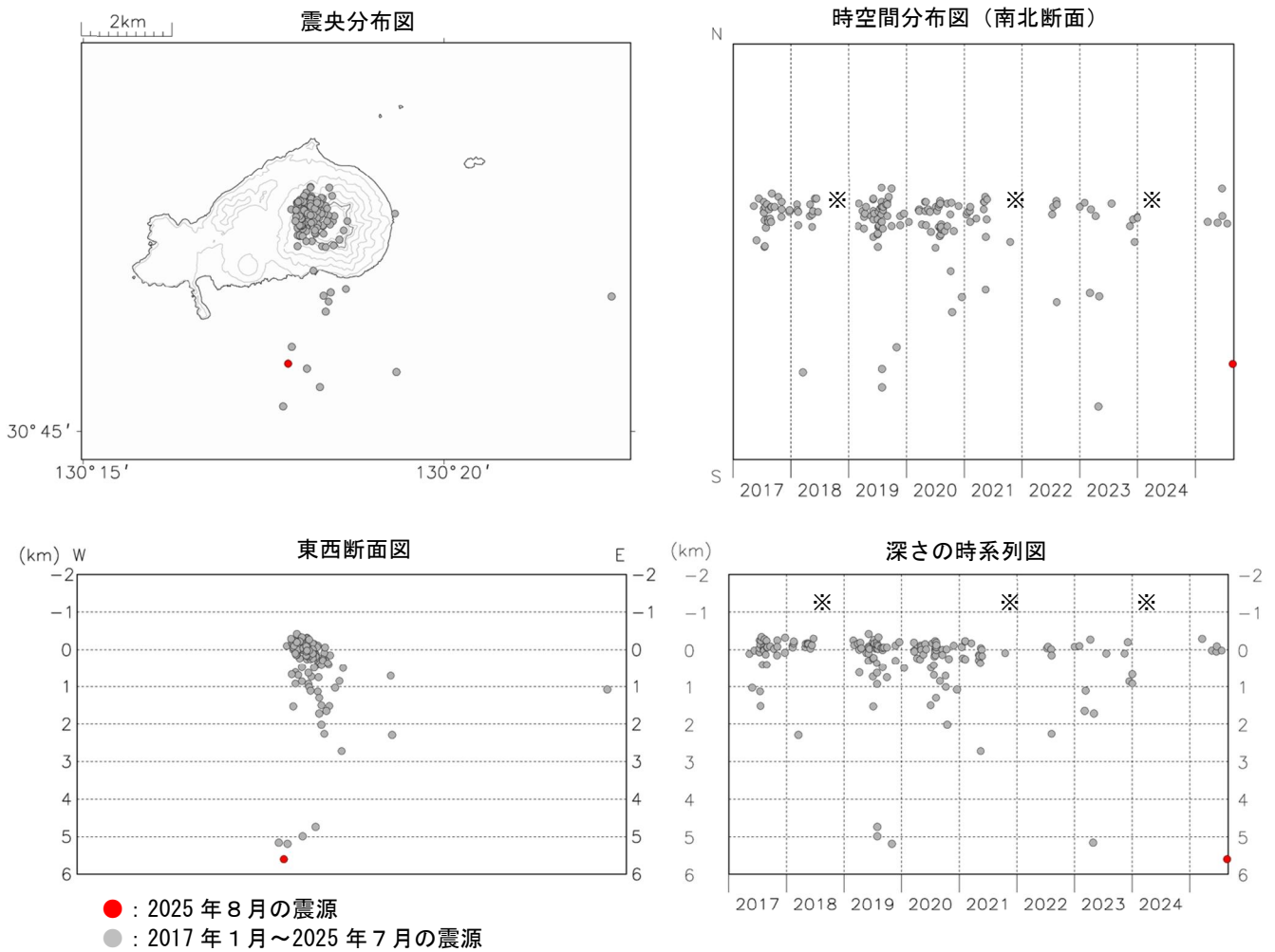
図 4 薩摩硫黄島 火山性地震の震源分布図（2017 年 1 月～2025 年 8 月）
