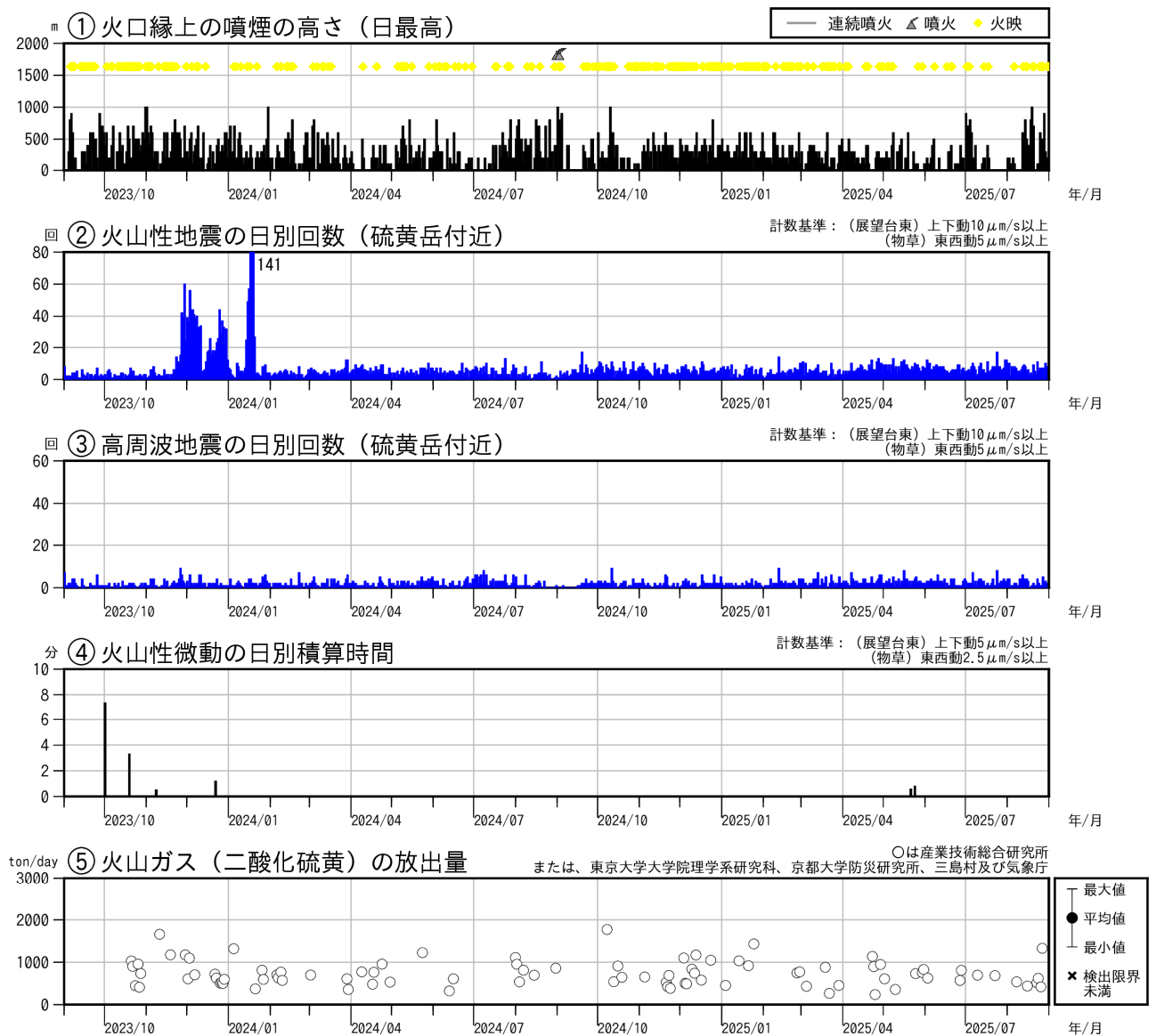
図3 薩摩硫黄島 火山活動経過図（2023年9月～2025年8月）
