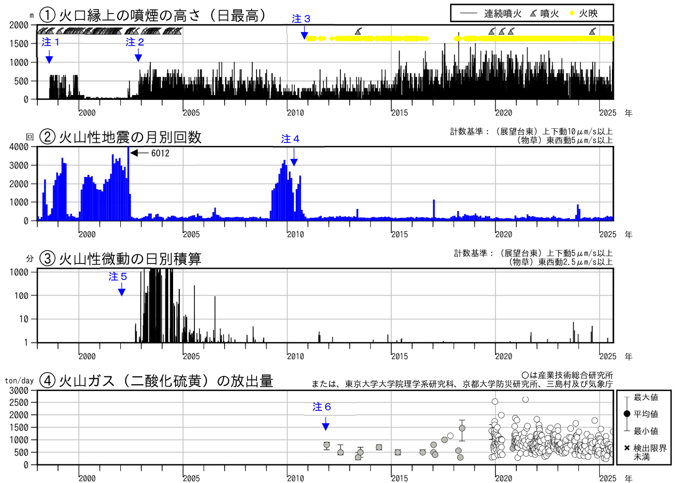
図2 薩摩硫黄島 火山活動経過図（1998年1月～2025年8月）
