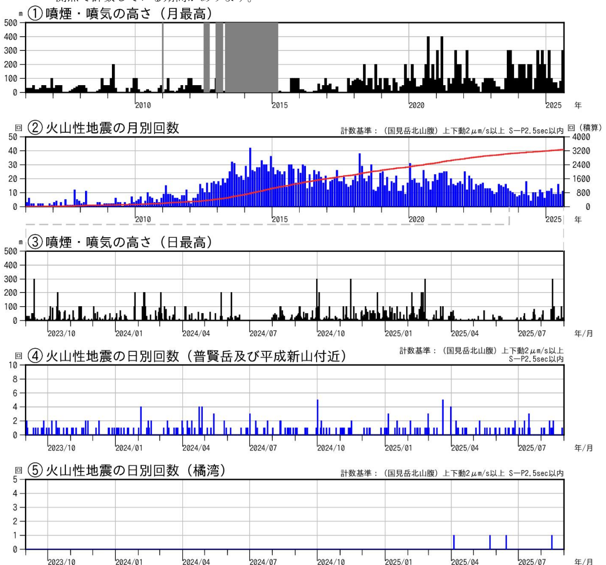
図3 雲仙岳 火山活動経過図（2006年1月～2025年8月）
