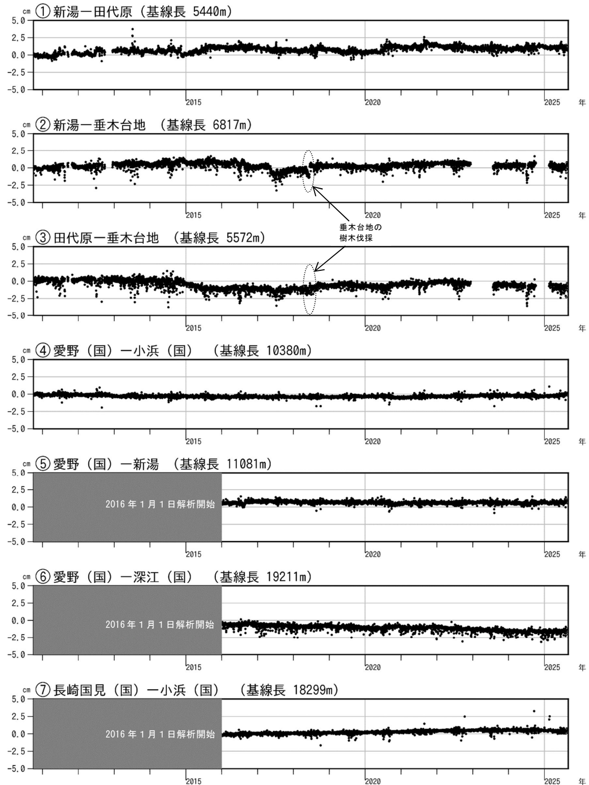
図5 雲仙岳 GNSS連続観測による基線長変化（2010年10月～2025年8月）
