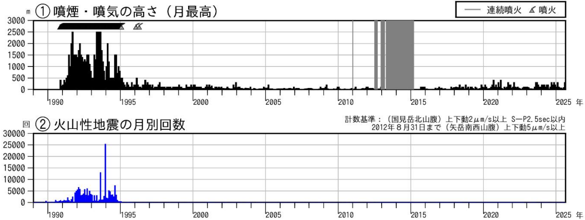
図2 雲仙岳 長期の火山活動経過図（1989年1月～2025年8月）
