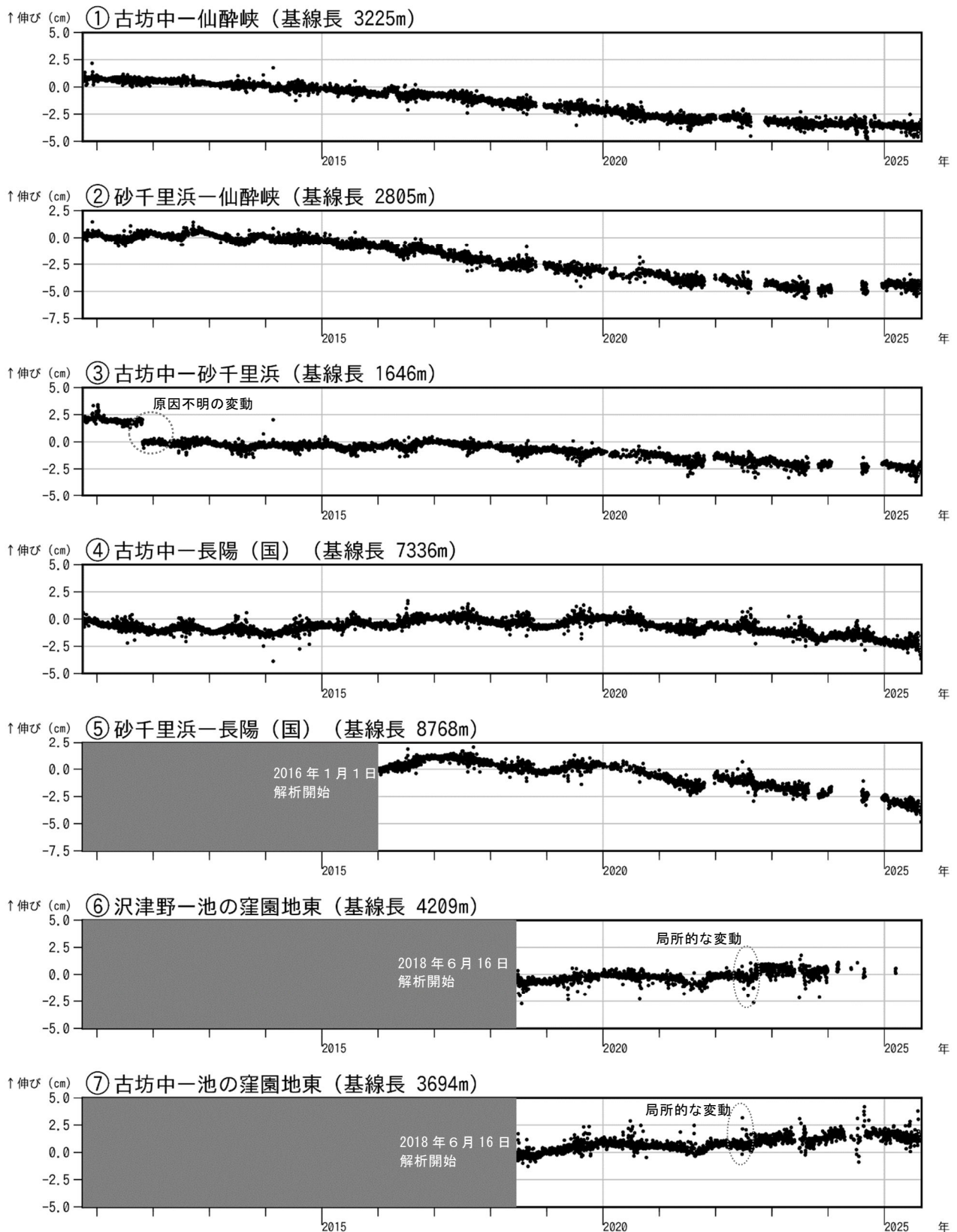
図5 阿蘇山 GNSS 連続観測による基線長変化（2010年10月～2025年8月）
