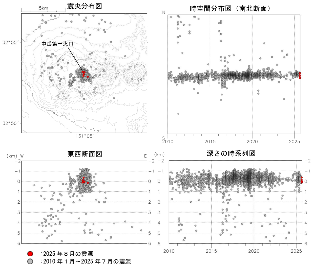
図4 阿蘇山 火山性地震の震源分布
