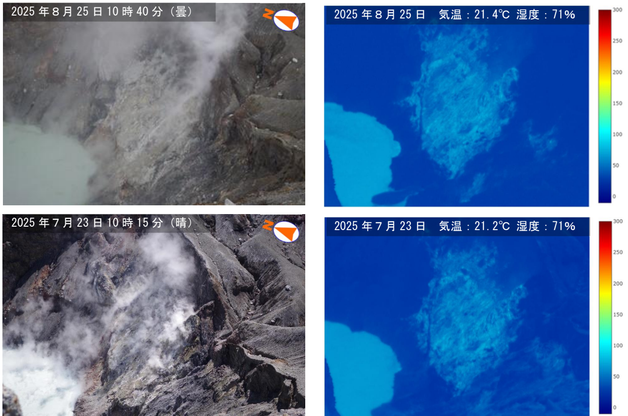
図 2-2 阿蘇山 中岳第一火口 南側火口壁の状況 （火口南西側観測定点から撮影 上図：8月25日、下図：7月23日）
