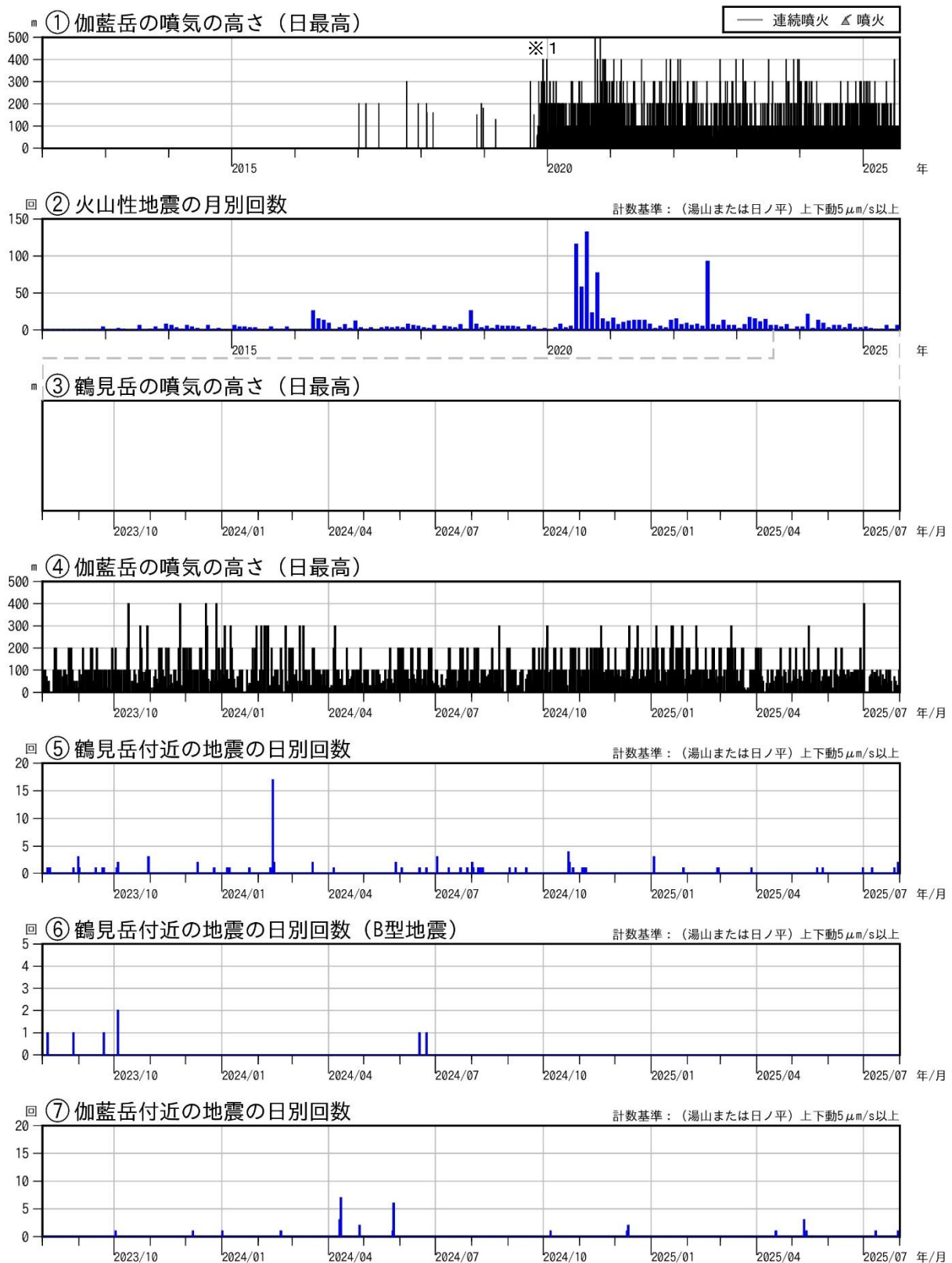
図2 鶴見岳・伽藍岳 火山活動経過図（2012年1月～2025年7月）
