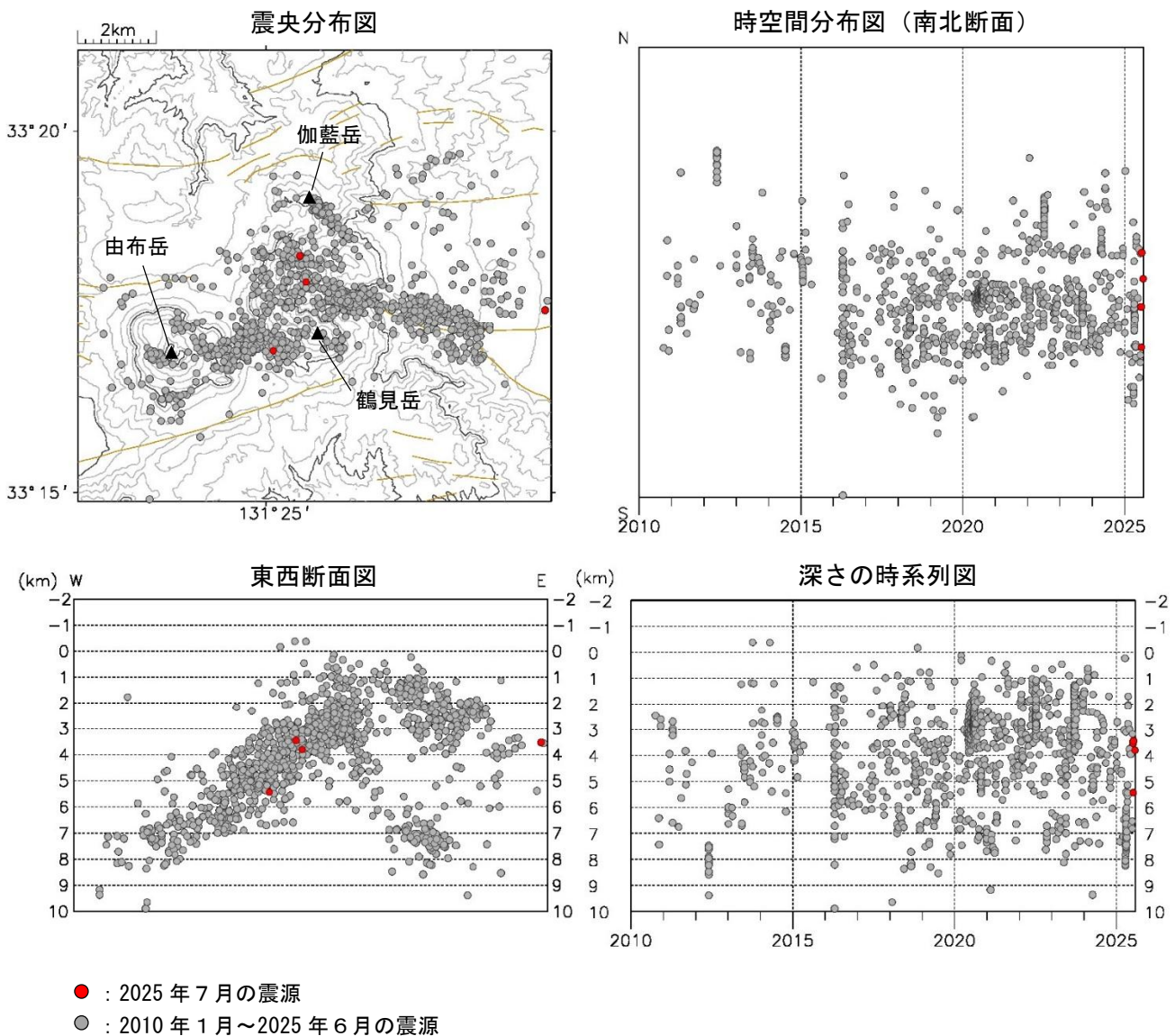
図 3 鶴見岳・伽藍岳 震源分布図（2010 年 1 月～2025 年 7 月）
