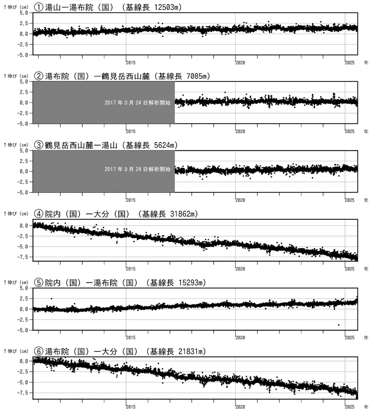
図 4 鶴見岳・伽藍岳 GNSS連続観測による基線長変化（2010 年 10 月～2025 年 7 月）
