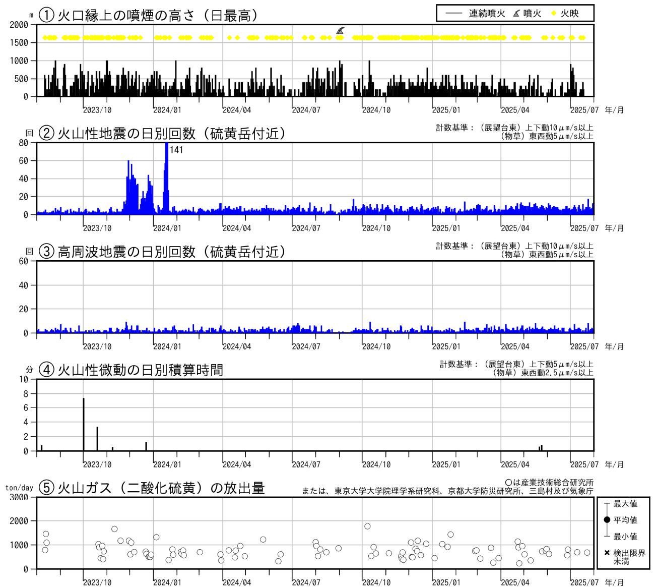
図4 薩摩硫黄島 火山活動経過図（2023年8月～2025年7月）
