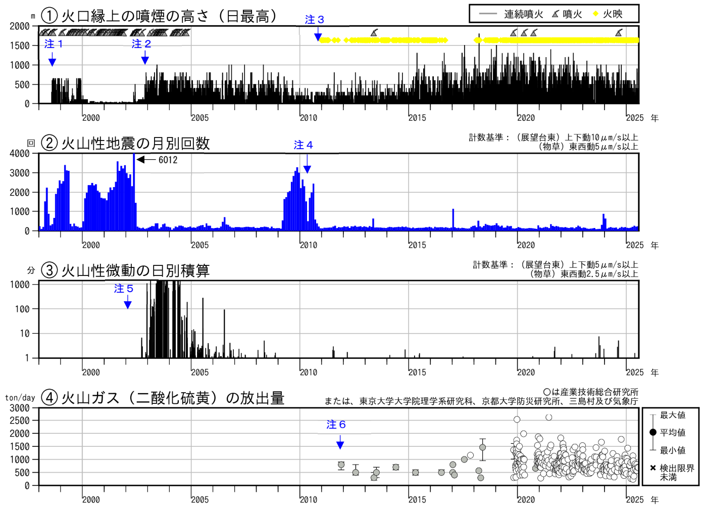
図3 薩摩硫黄島 火山活動経過図（1998年1月～2025年7月）
