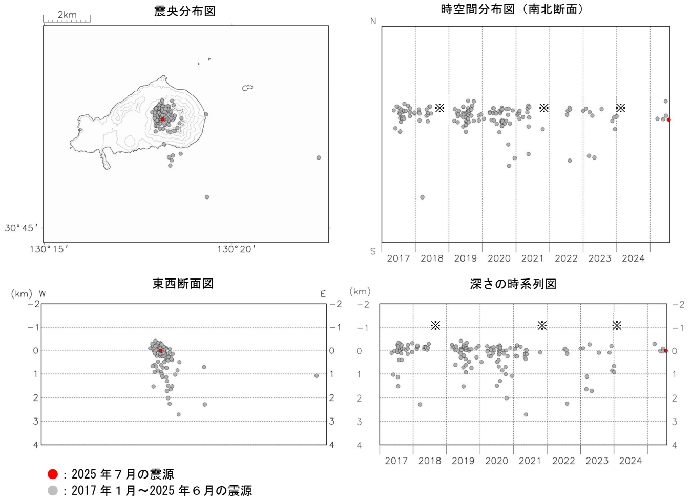
図5 薩摩硫黄島 火山性地震の震源分布図（2017 年 1 月～2025 年 7 月）
