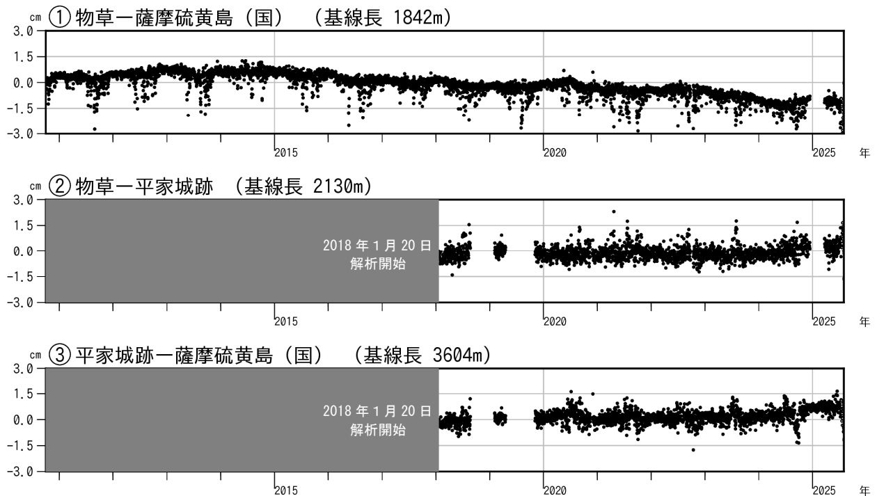
図6 薩摩硫黄島 GNSS連続観測による基線長変化（2010年10月～2025年7月）
