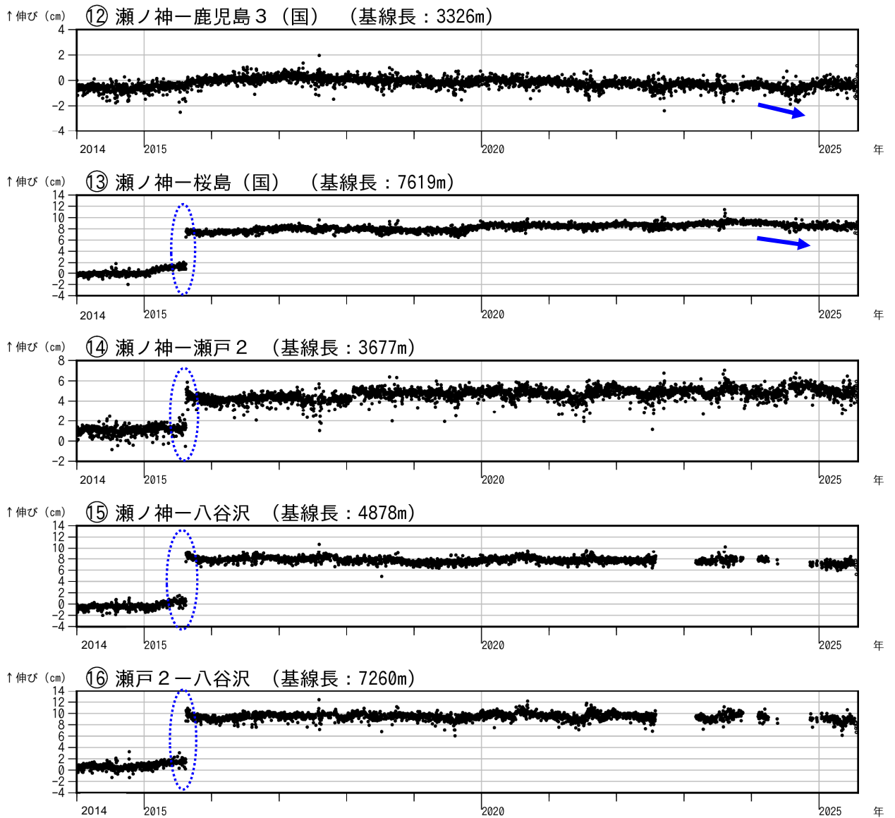
図 10-3 桜島 GNSS 連続観測による基線長変化（2014 年 1 月～2025 年 7 月）
