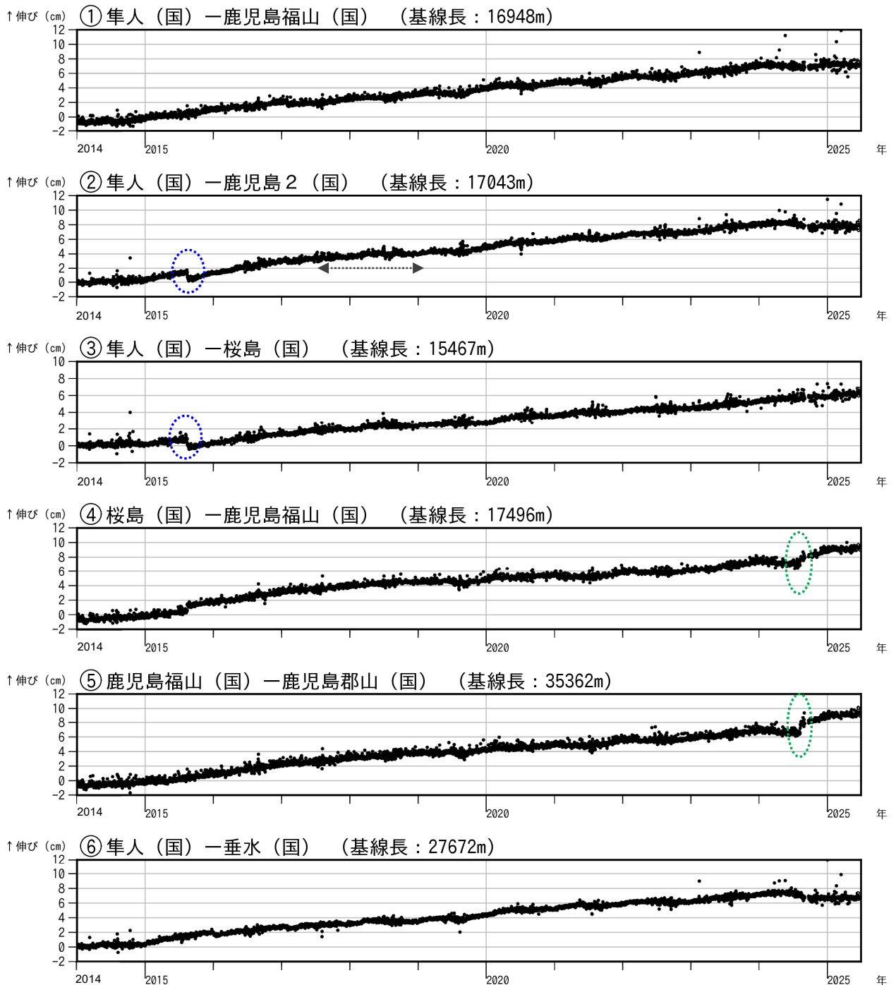
図 10-1 桜島 GNSS 連続観測による基線長変化 (2014 年 1 月～2025 年 7 月)
