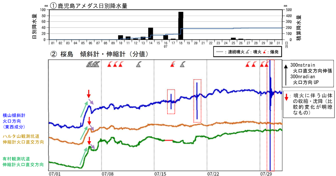
図9 桜島 傾斜計及び伸縮計による地殻変動の状況（2025年7月1日～7月31日）
