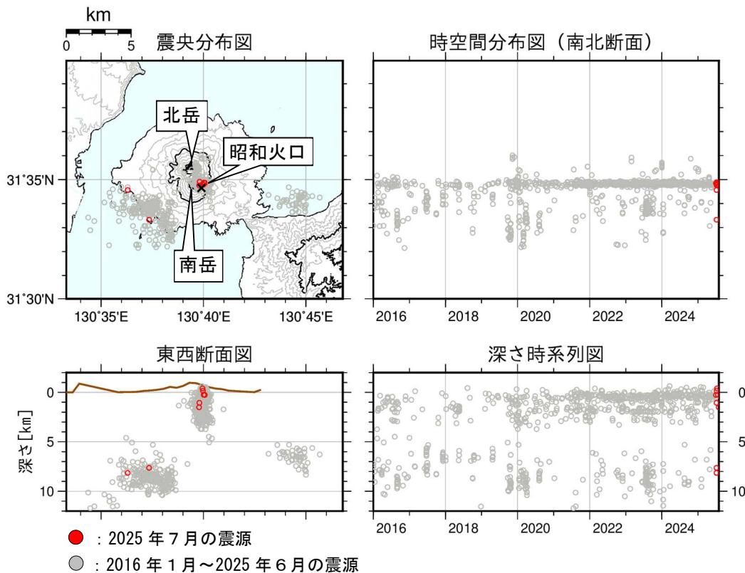
図 5-2 桜島 桜島付近の震源分布図（2016 年 1 月～2025 年 7 月）
