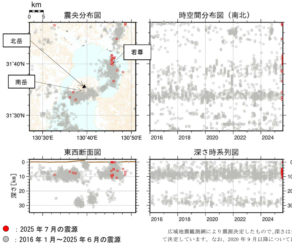
図 5-1 桜島 始良カルデラ周辺の震源分布図（2016 年 1 月～2025 年 7 月）
