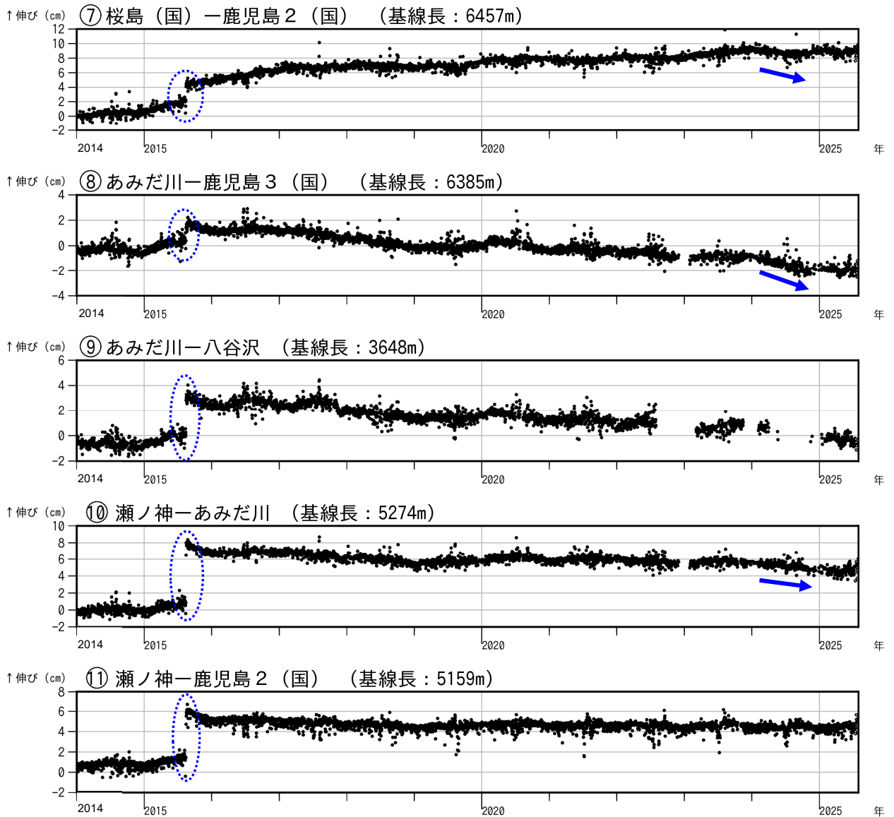
図 10-2 桜島 GNSS 連続観測による基線長変化 (2014 年 1 月～2025 年 7 月)
