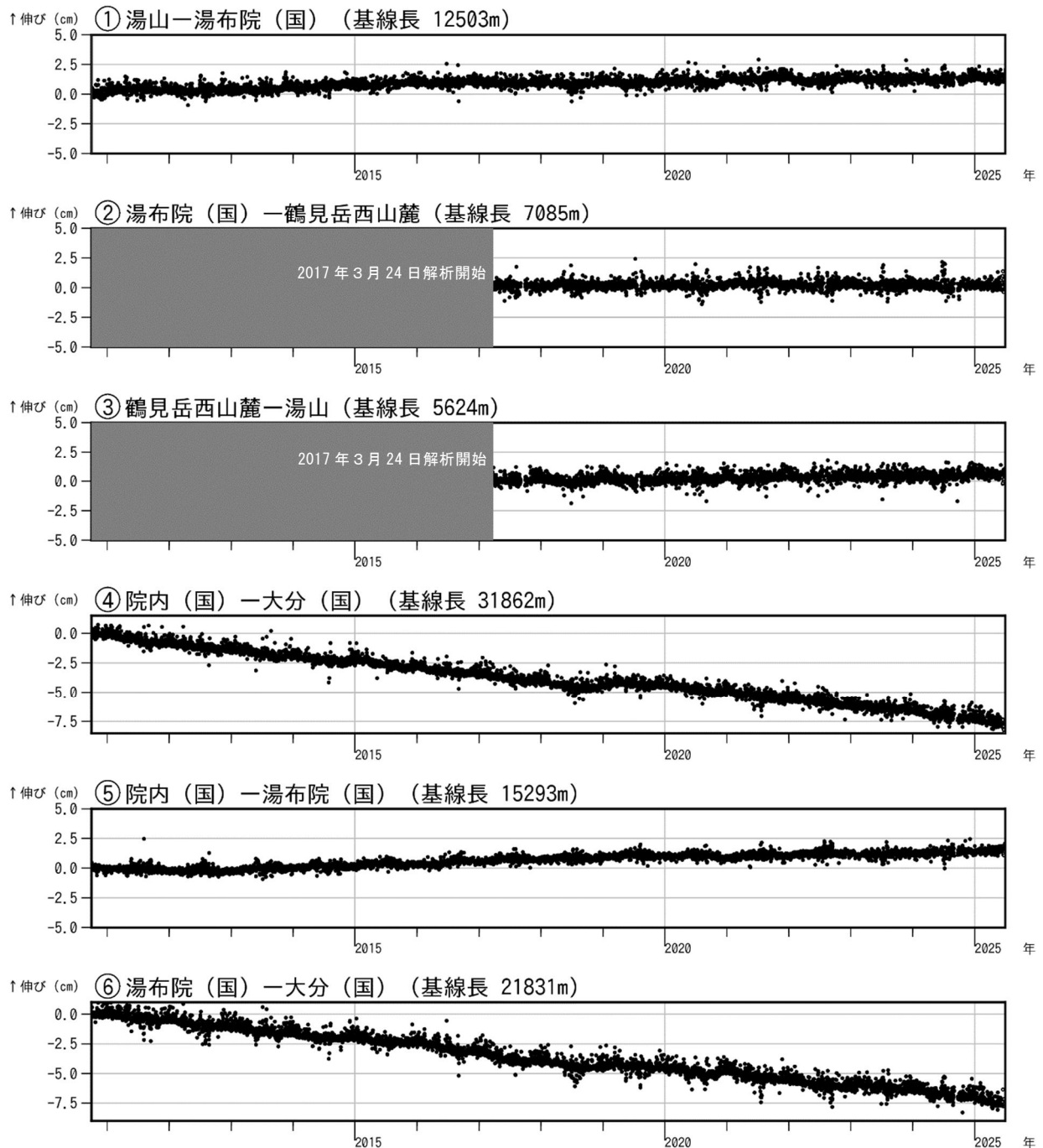
図4 鶴見岳・伽藍岳 GNSS連続観測による基線長変化（2010年10月～2025年6月）
