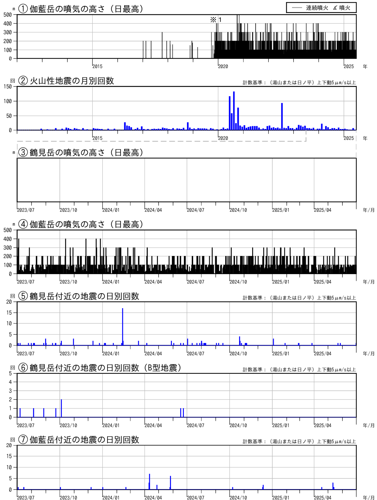
図2 鶴見岳・伽藍岳 火山活動経過図（2012年1月～2025年6月）
