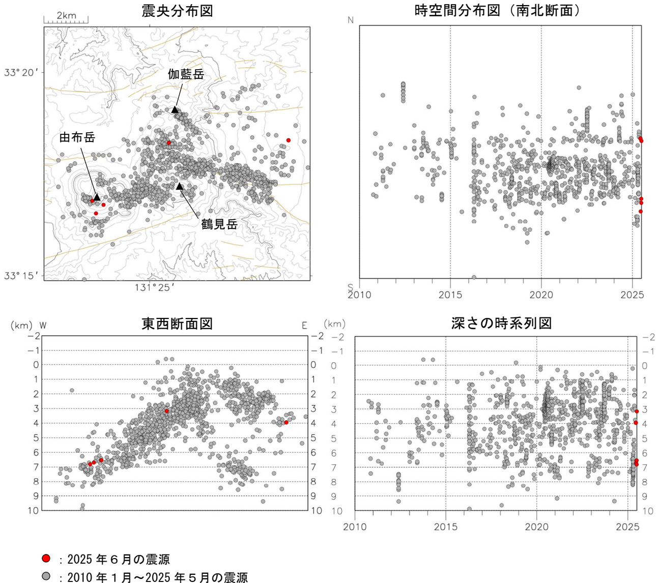
図3 鶴見岳・伽藍岳 震源分布図（2010年1月～2025年6月）
