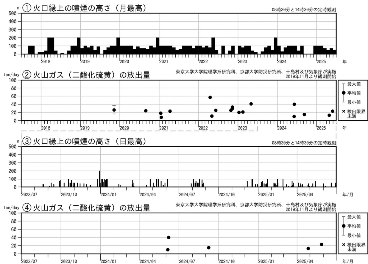
図2 中之島 火山活動経過図（2017年7月～2025年6月）
