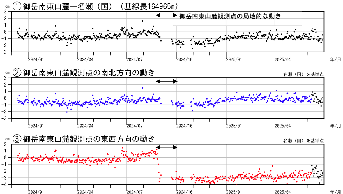
図4 中之島 GNSS連続観測（2023 年 12 月～2025 年 6 月）
