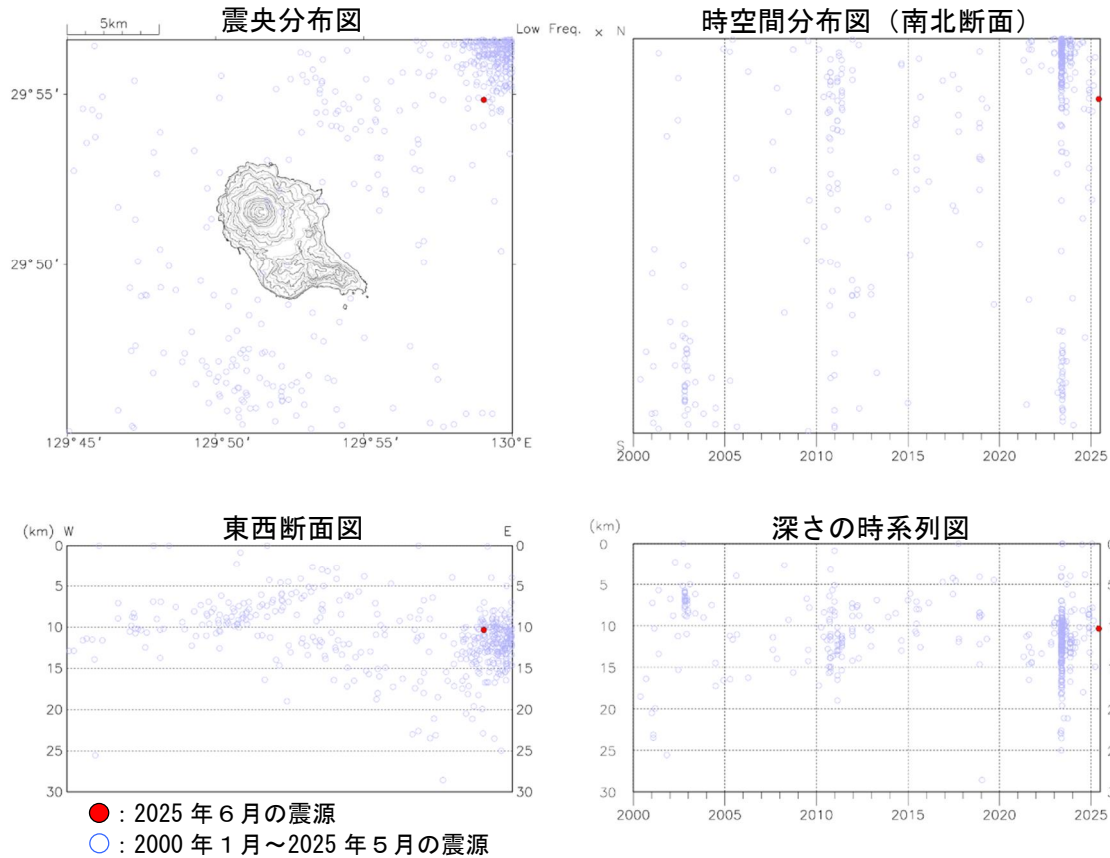
図3 中之島 中之島周辺の震源分布図（2000 年 1 月～2025 年 6 月）
