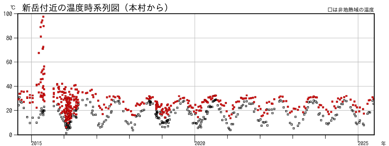
図 3-5 口永良部島 新岳火口西側割れ目付近の地熱域の温度時系列 (2014 年 9 月～2025 年 6 月、本村から観測)
