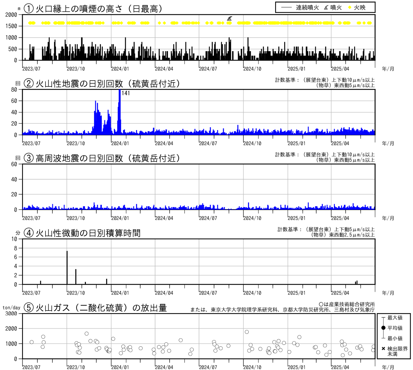
図3 薩摩硫黄島 火山活動経過図（2023年7月～2025年6月）
