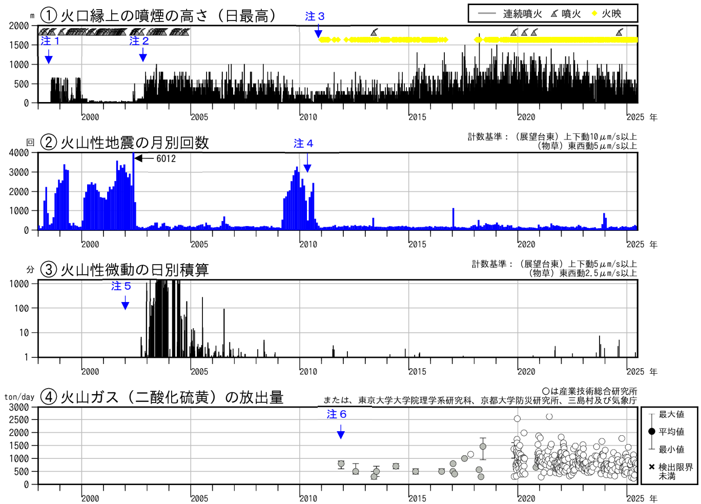
図2 薩摩硫黄島 火山活動経過図（1998年1月～2025年6月）
