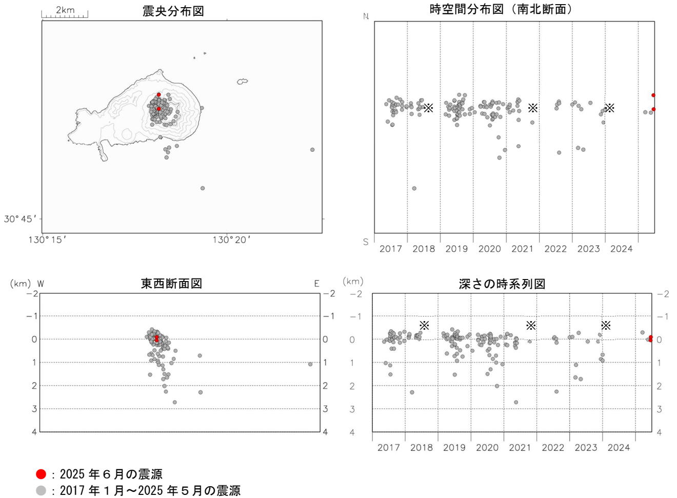
図4 薩摩硫黄島 火山性地震の震源分布図（2017 年 1 月～2025 年 6 月）
