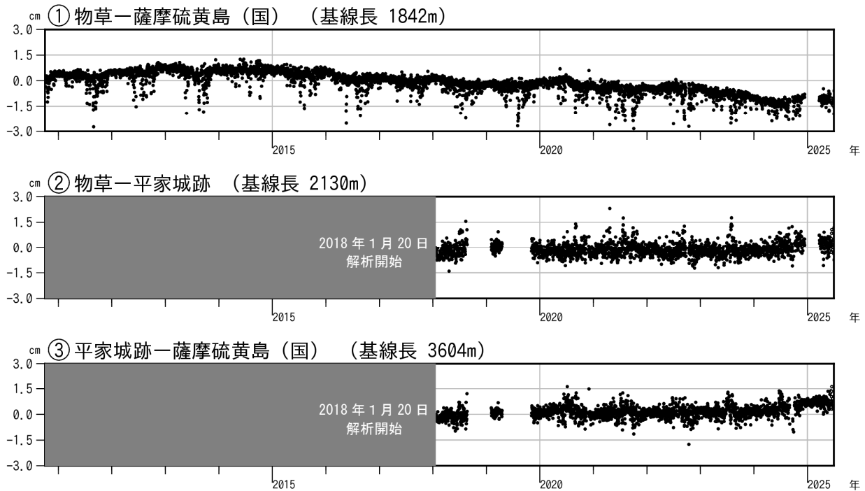
図5 薩摩硫黄島 GNSS連続観測による基線長変化（2010年10月～2025年6月）
