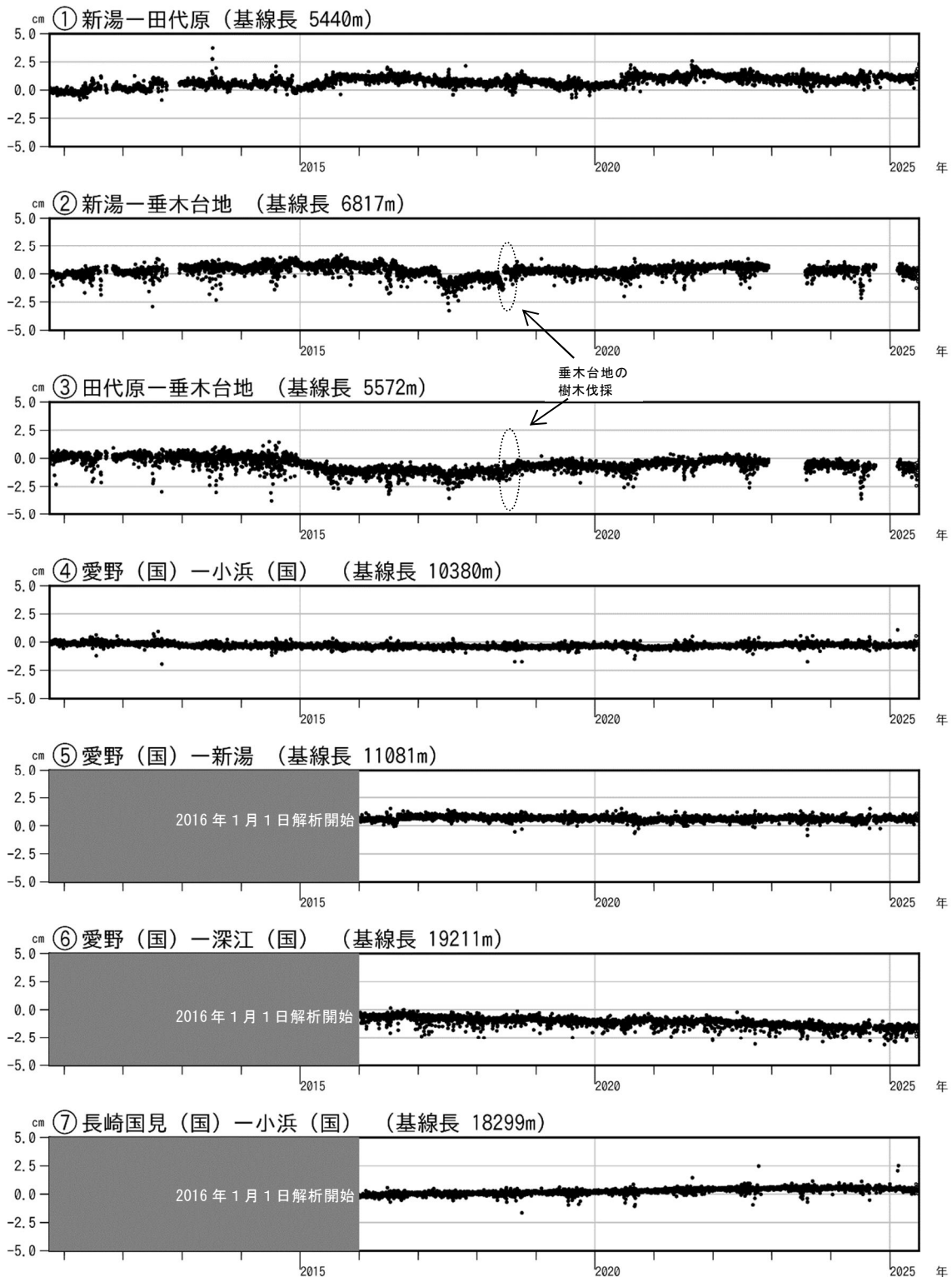
図5 雲仙岳 GNSS連続観測による基線長変化（2010年10月～2025年6月）
