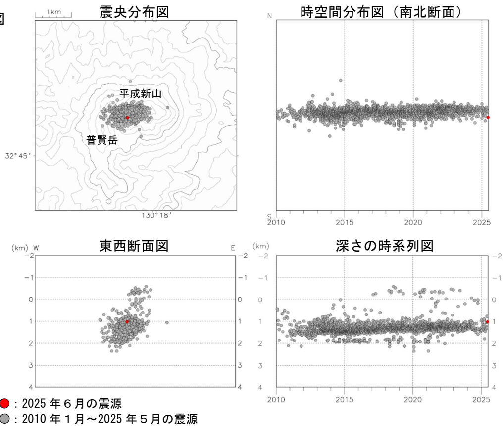
図 4 雲仙岳 震源分布図 ①広域図 ②狭域図（2010 年 1 月～2025 年 6 月）
