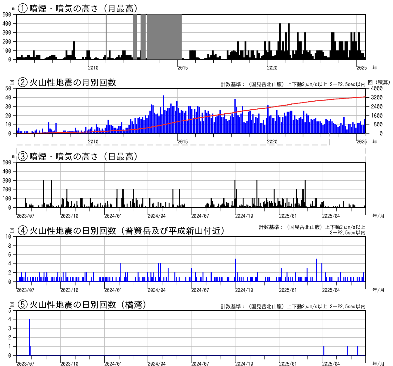
図3 雲仙岳 火山活動経過図（2006年1月～2025年6月）
