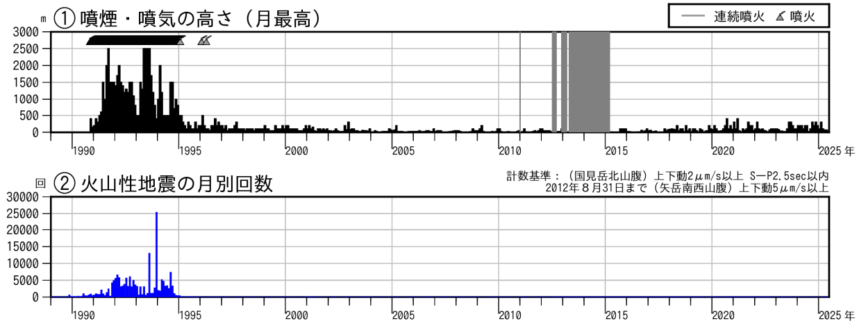
図2 雲仙岳 長期の火山活動経過図（1989年1月～2025年6月）
