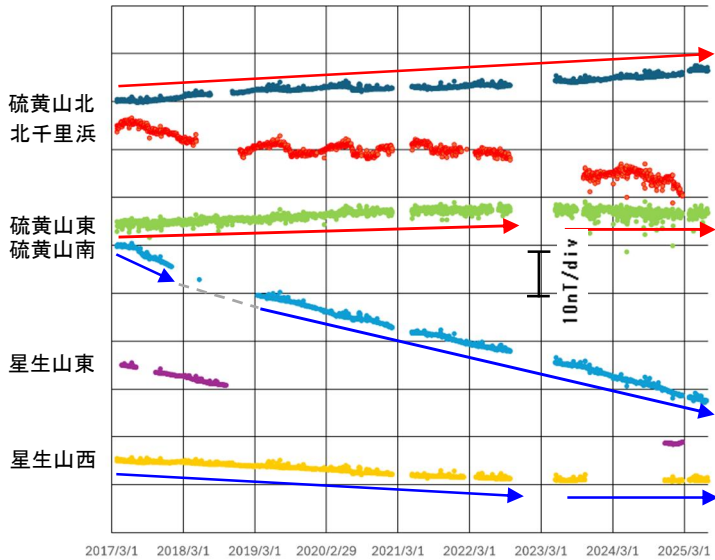
図 4-1 九重山 連続観測による全磁力の変化 (2017年3月～2025年6月)
