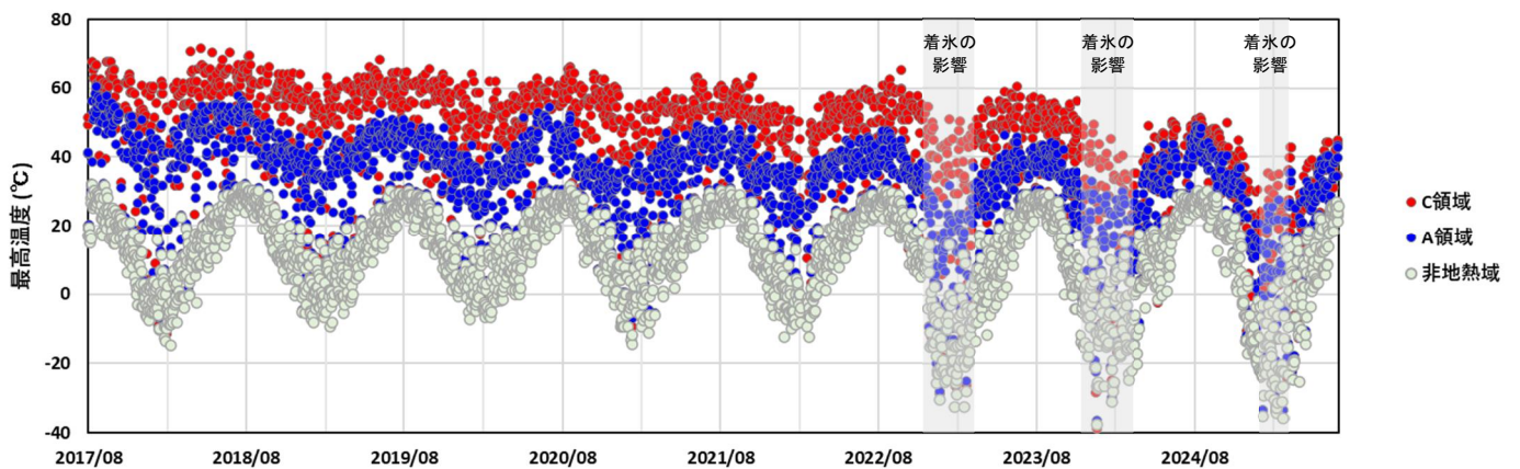
図 1-2 九重山 星生山北尾根の赤外熱映像装置による日別最高温度（2017 年 8 月～2025 年 6 月）
