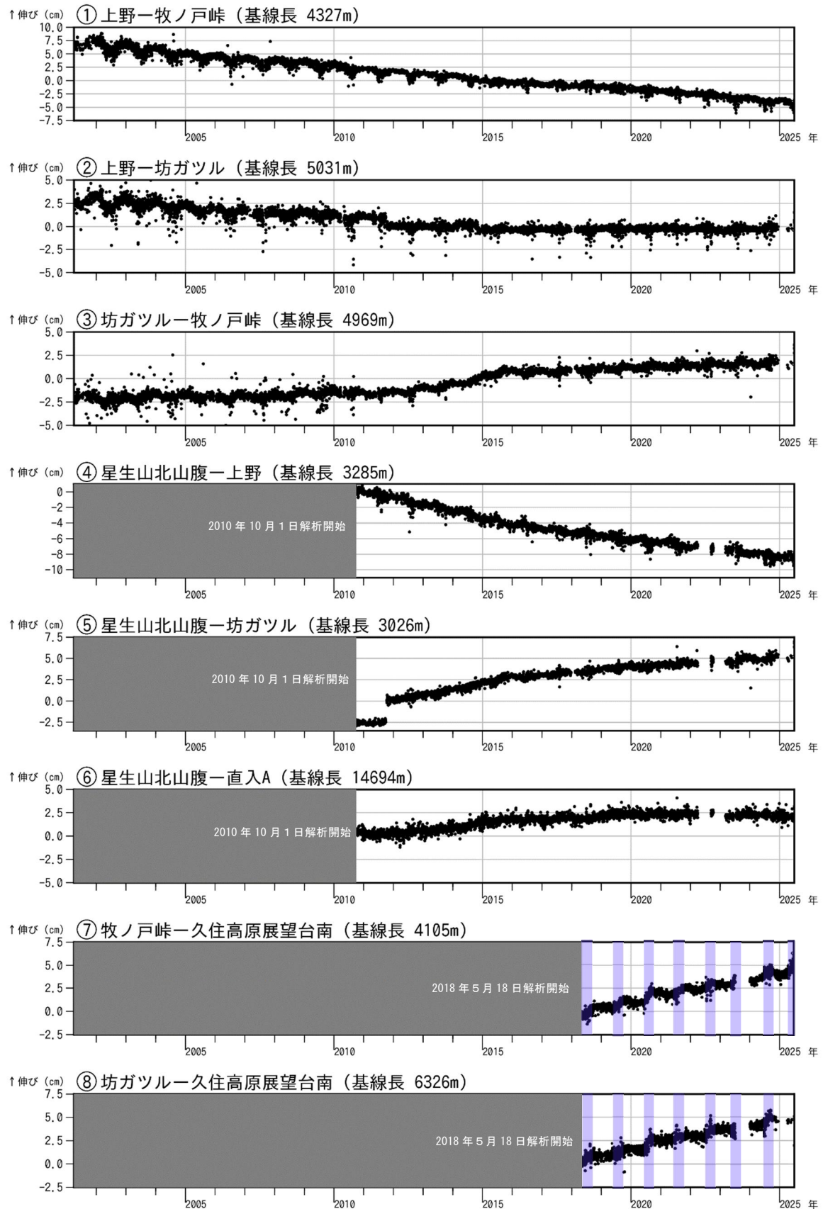
図5 九重山 GNSS 連続観測による基線長変化（2001年4月～2025年6月）
