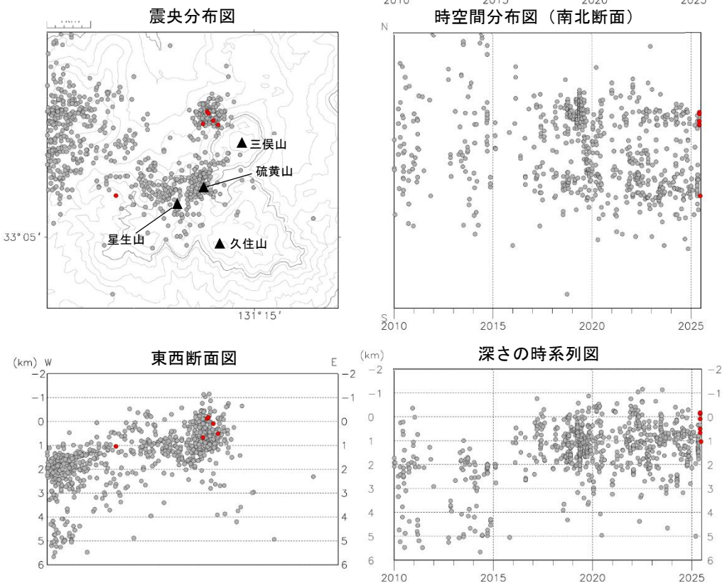
図3 九重山 震源分布図 ①広域図 ②狭域図（2010 年 1 月～2025 年 6 月）
