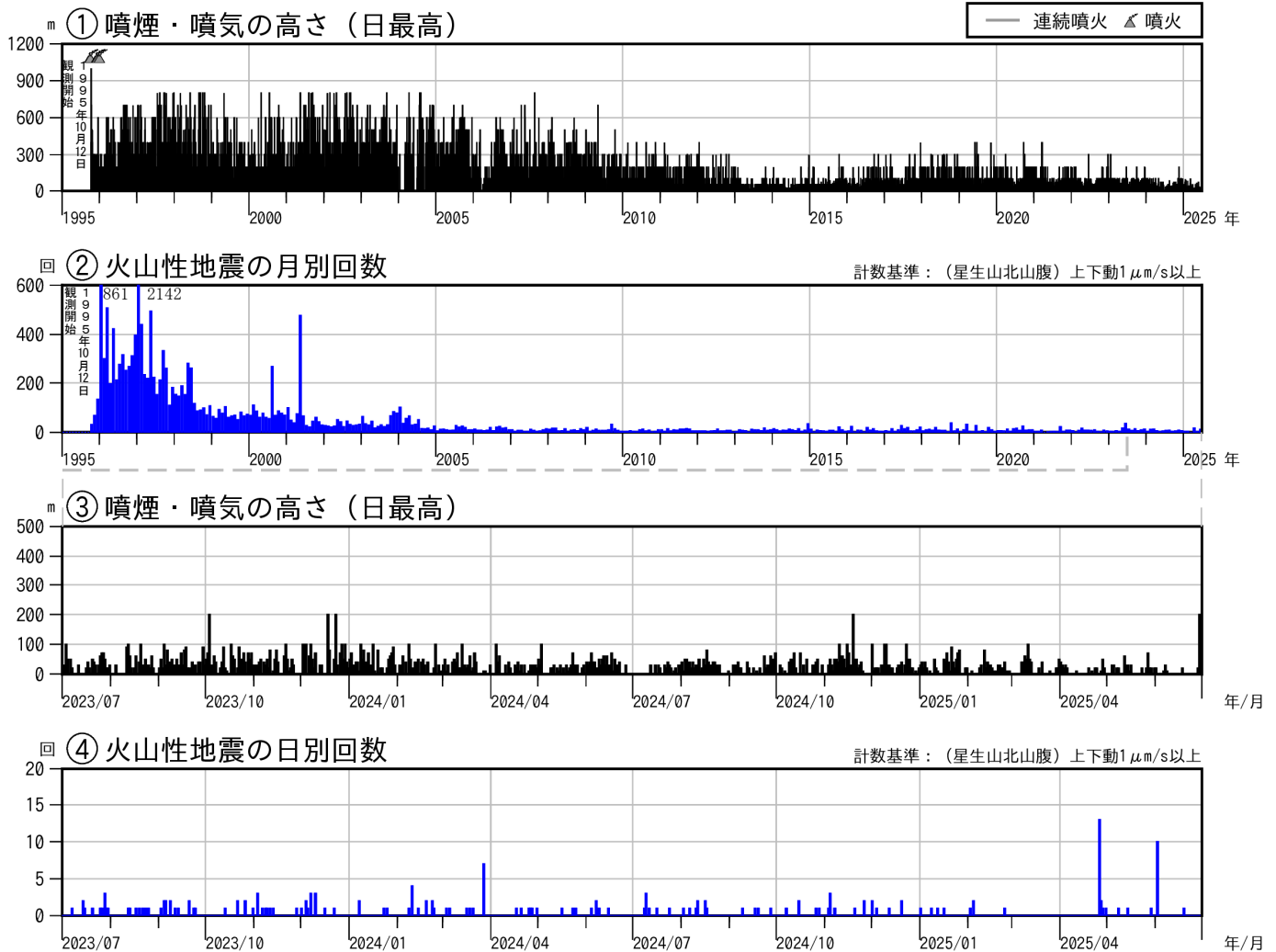
図2 九重山 火山活動経過図（1995年1月～2025年6月）
