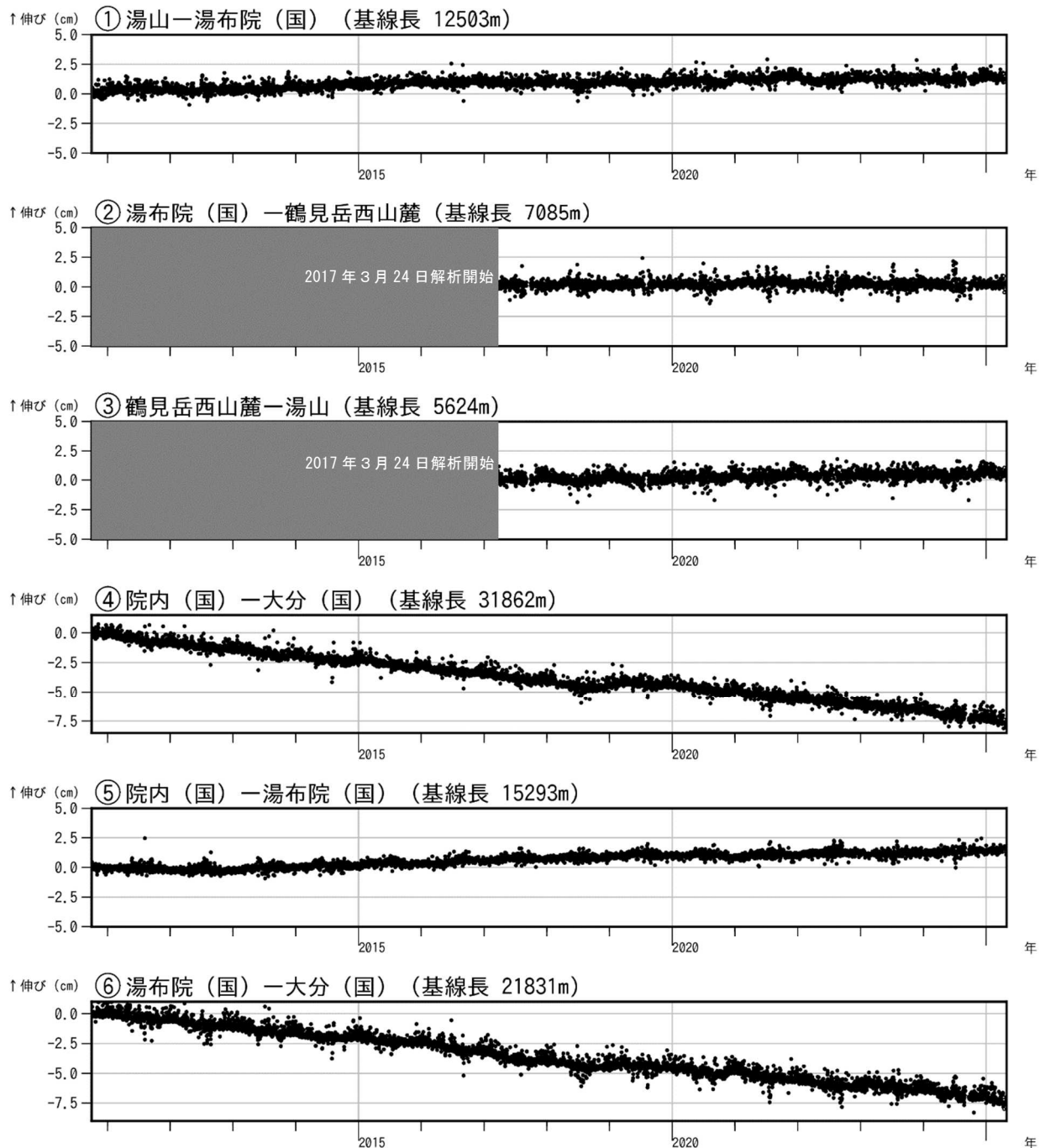
図4 鶴見岳・伽藍岳 GNSS連続観測による基線長変化（2010年10月～2025年4月）
