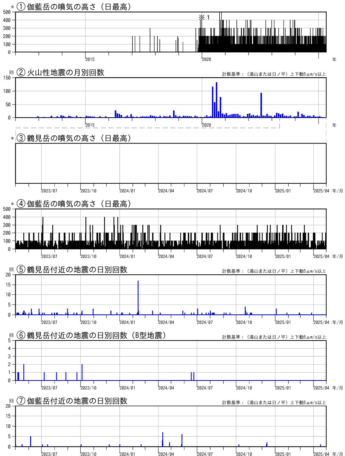
図2 鶴見岳・伽藍岳 火山活動経過図（2012年1月～2025年4月）
