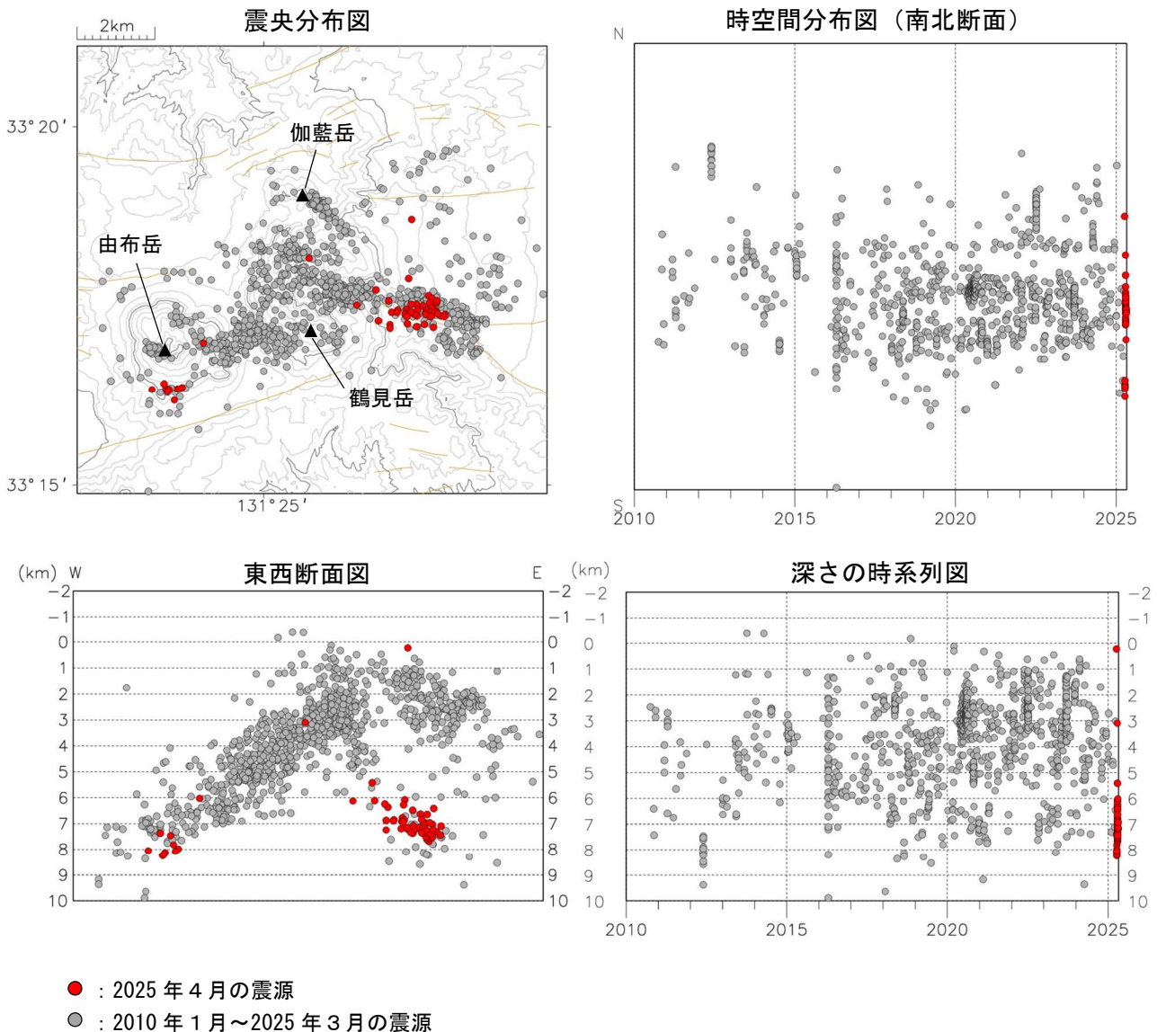
図 3 鶴見岳・伽藍岳 震源分布図（2010 年 1 月～2025 年 4 月）
