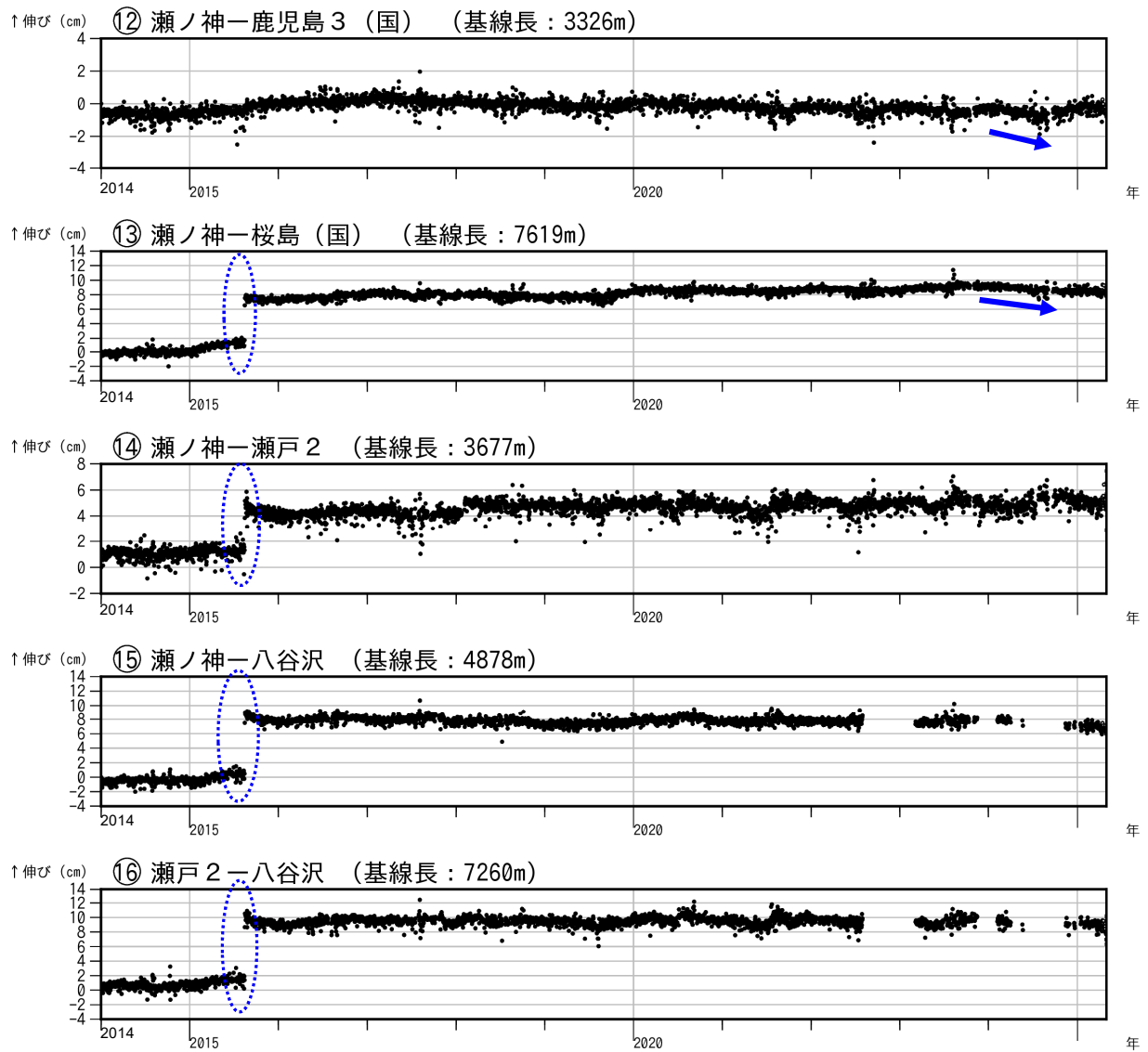
図 7-3 桜島 GNSS 連続観測による基線長変化（2014 年 1 月～2025 年 4 月）
