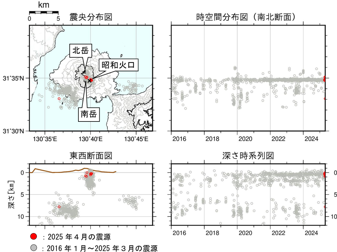
図 2-2 桜島 桜島付近の震源分布図（2016 年 1 月～2025 年 4 月）
