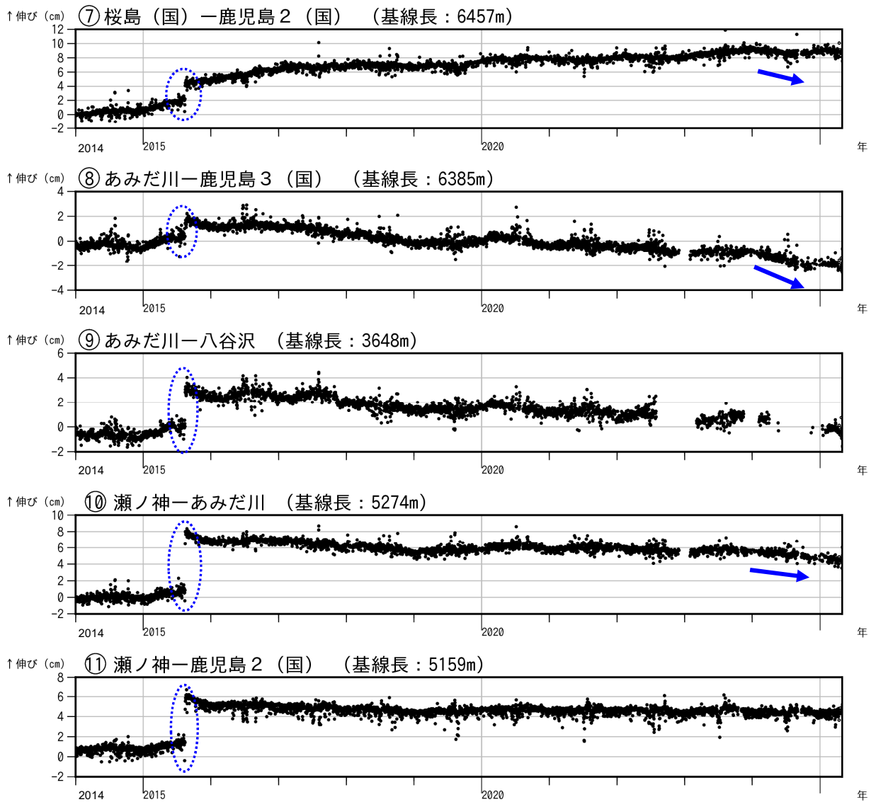
図 7-2 桜島 GNSS 連続観測による基線長変化（2014 年 1 月～2025 年 4 月）
