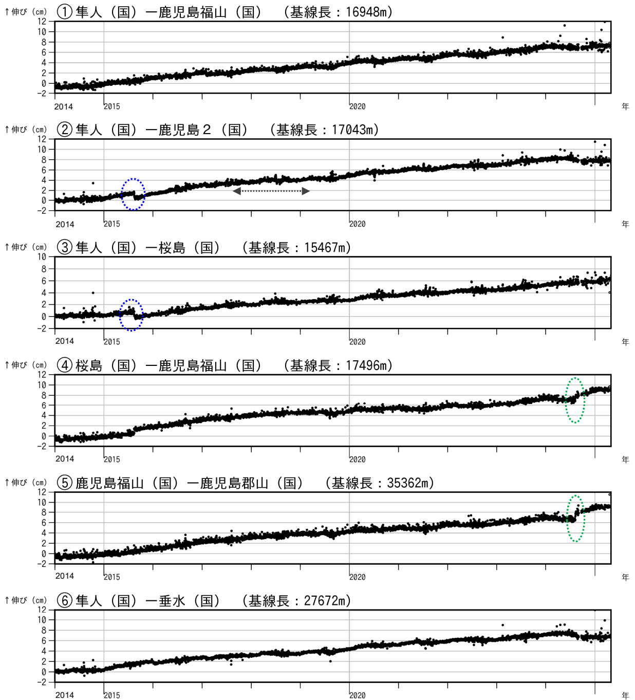
図 7-1 桜島 GNSS 連続観測による基線長変化 (2014 年 1 月～2025 年 4 月)
