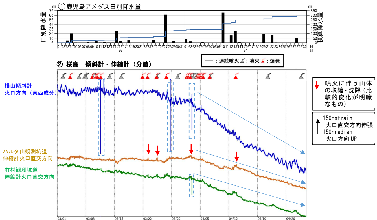
図 6 桜島 傾斜計及び伸縮計による地殻変動の状況（2025 年 3～4 月）
