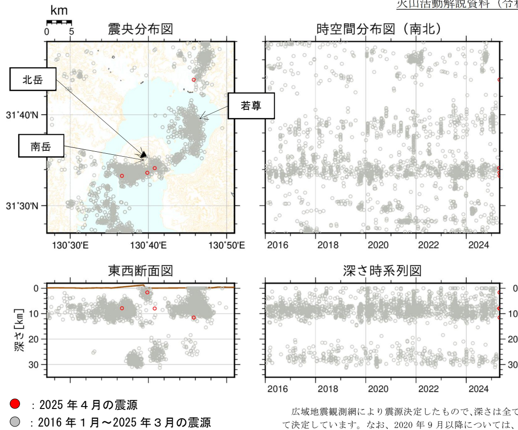
図 2-1 桜島 始良カルデラ周辺の震源分布図（2016 年 1 月～2025 年 4 月）
