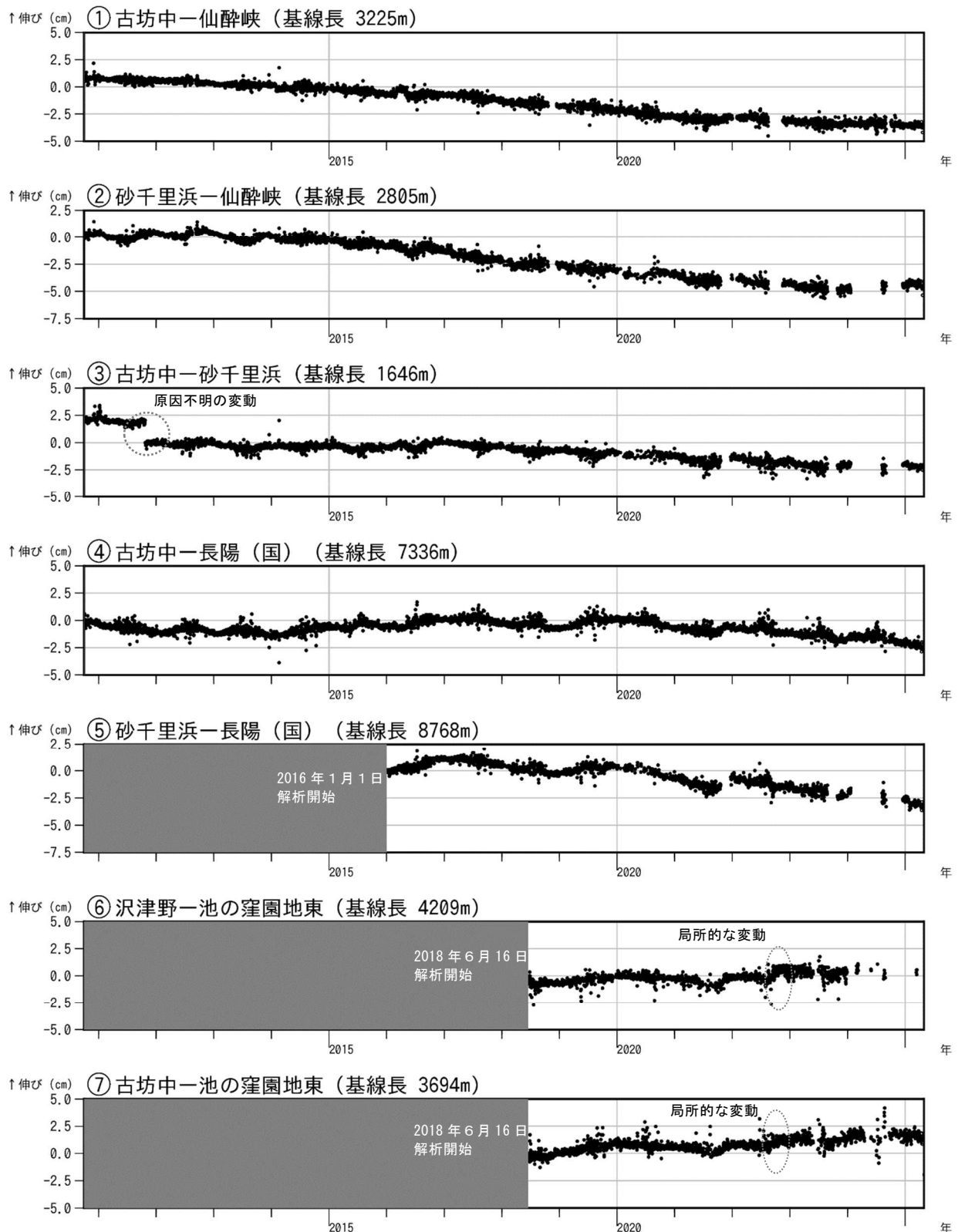
図5 阿蘇山 GNSS 連続観測による基線長変化（2010年10月～2025年4月）
