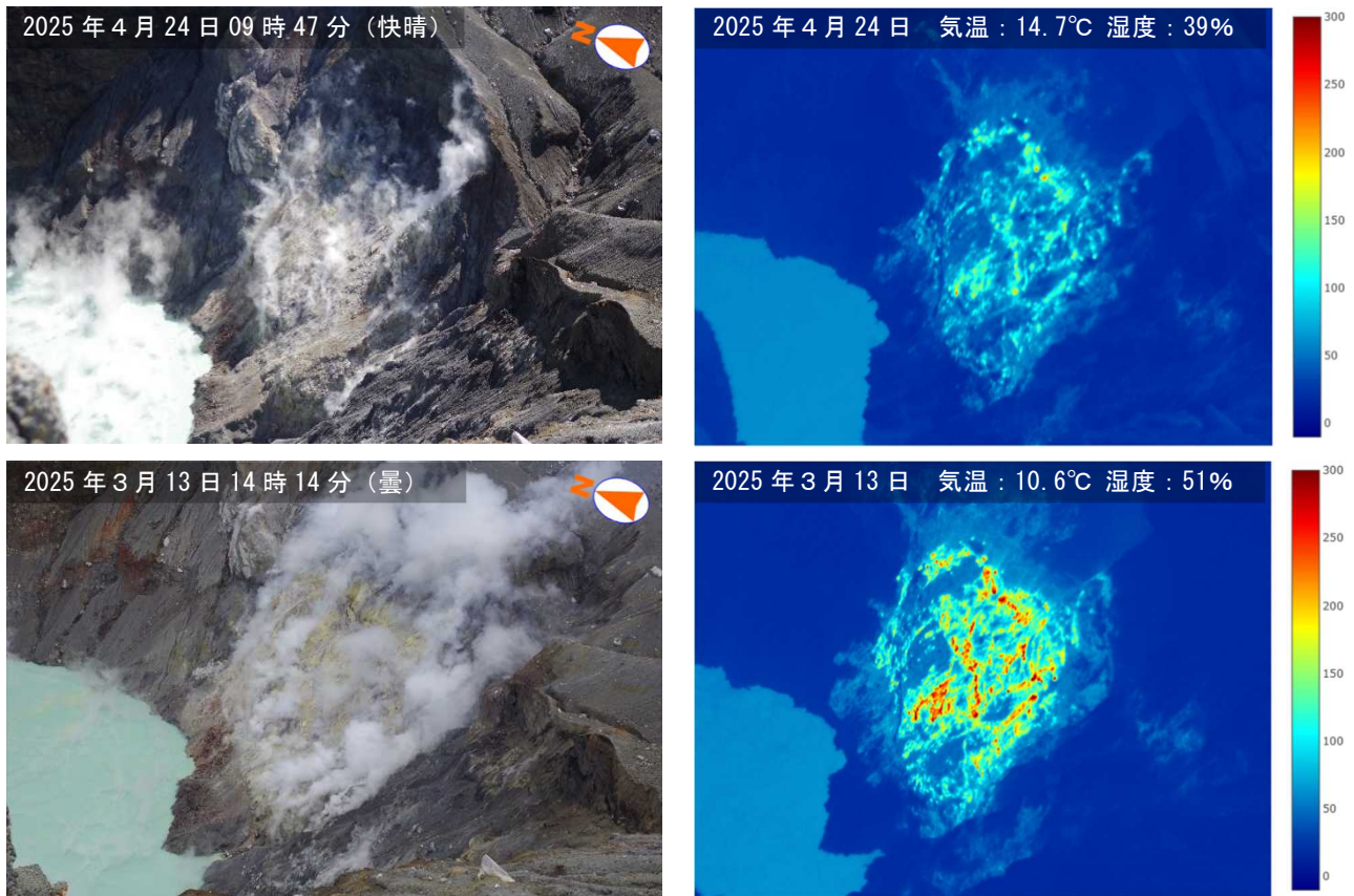
図 2-2 阿蘇山 中岳第一火口 南側火口壁の状況 （火口南西側観測定点から撮影 上図：4月24日、下図：3月13日）
