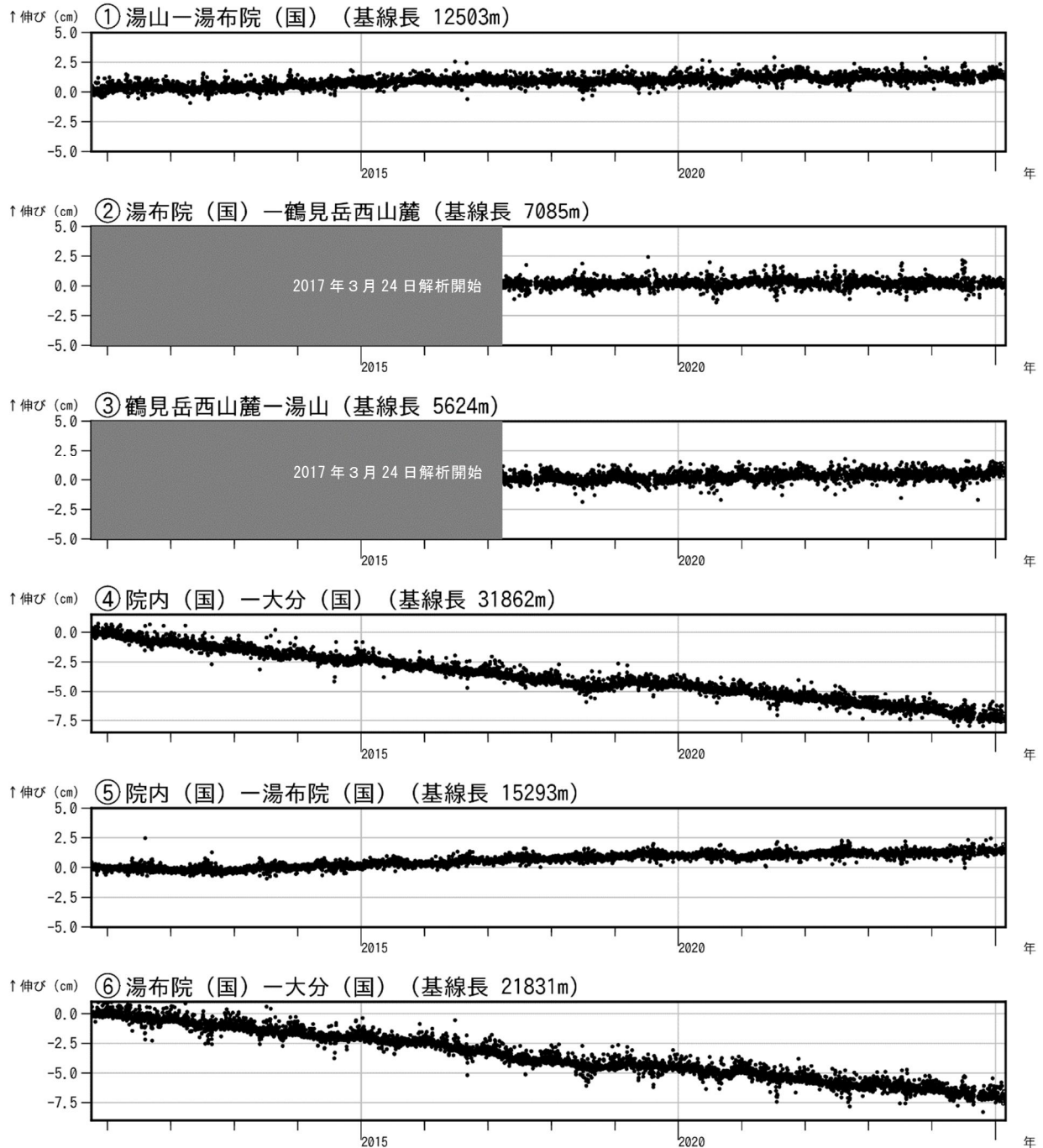
図4 鶴見岳・伽藍岳 GNSS連続観測による基線長変化（2010年10月～2025年2月）
