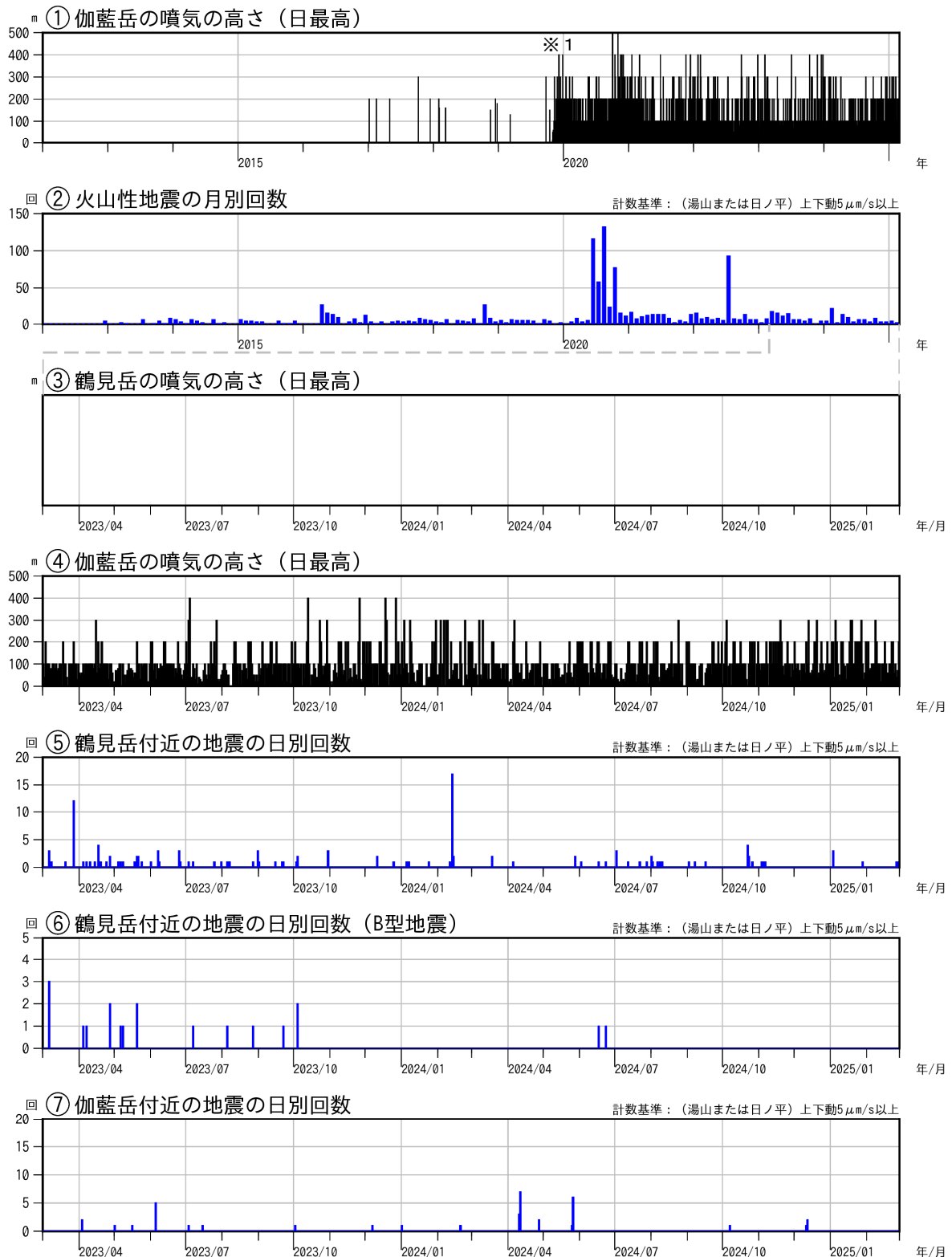
図2 鶴見岳・伽藍岳 火山活動経過図（2012年1月～2025年2月）
