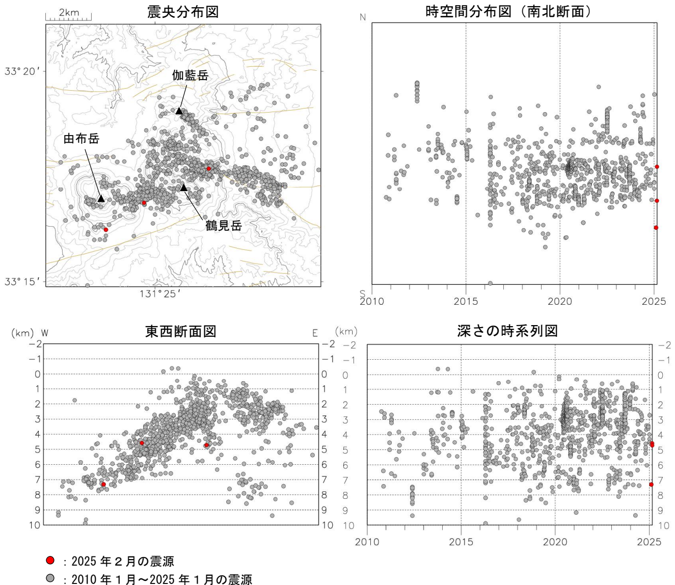
図3 鶴見岳・伽藍岳 震源分布図（2010 年 1 月～2025 年 2 月）
