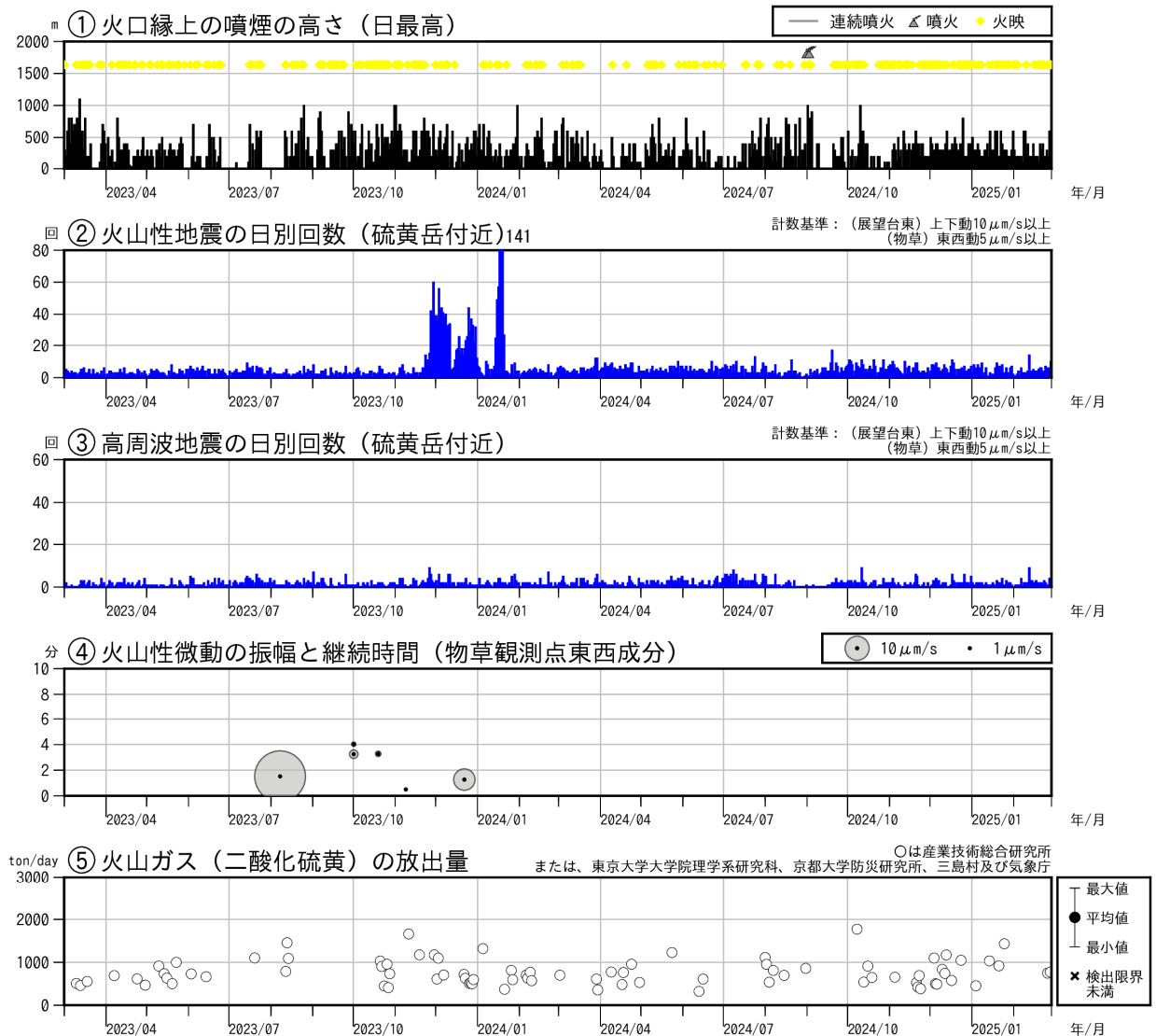
図3 薩摩硫黄島 火山活動経過図（2023年3月～2025年2月）
