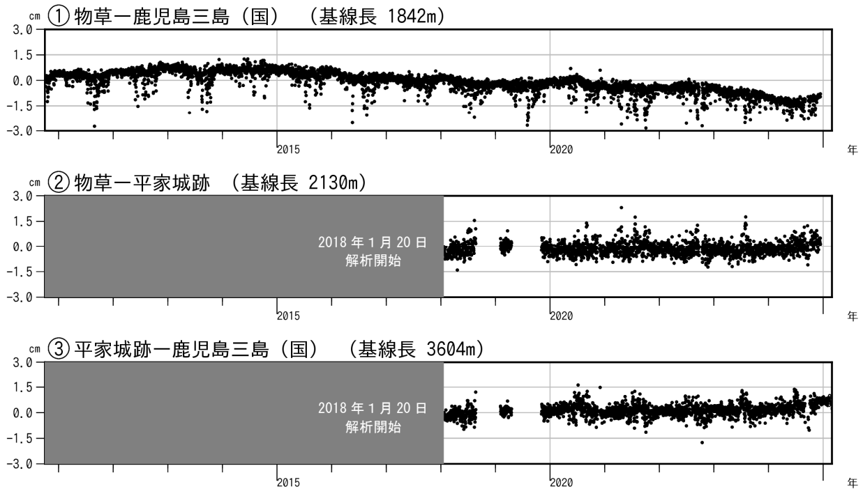
図 4 薩摩硫黄島 GNSS連続観測による基線長変化（2010 年 10 月～2025 年 2 月）
