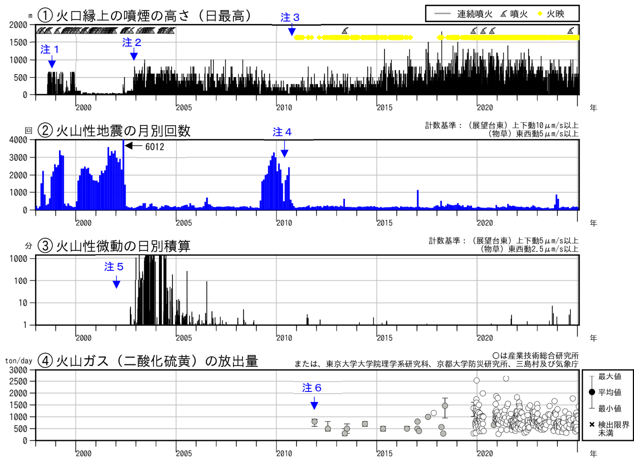
図2 薩摩硫黄島 火山活動経過図（1998年1月～2025年2月）
