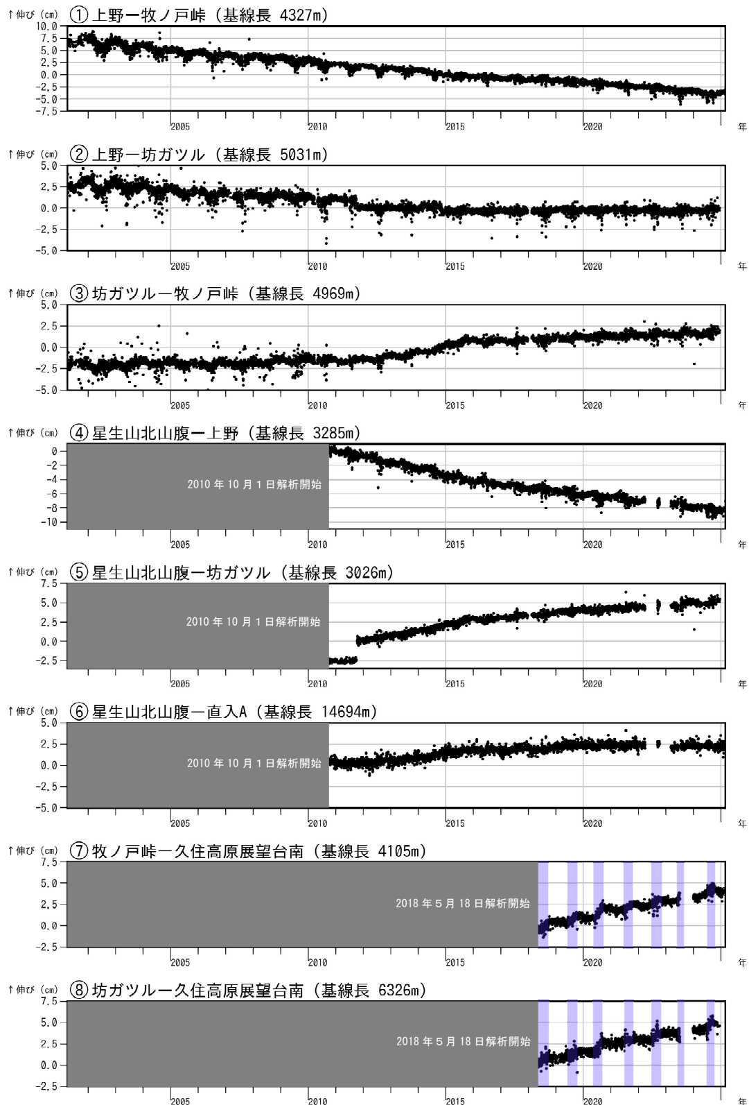
図5 九重山 GNSS 連続観測による基線長変化（2001年4月～2025年2月）
