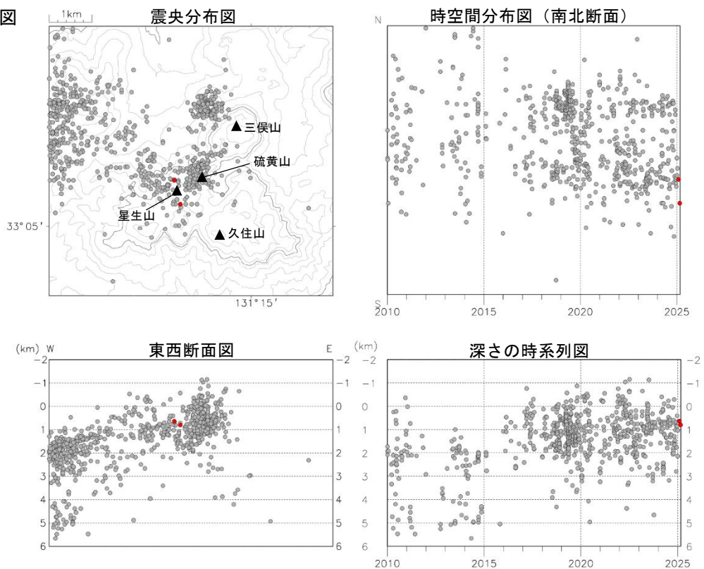
図 3 九重山 震源分布図 ①広域図 ②狭域図（2010 年 1 月～2025 年 2 月）
