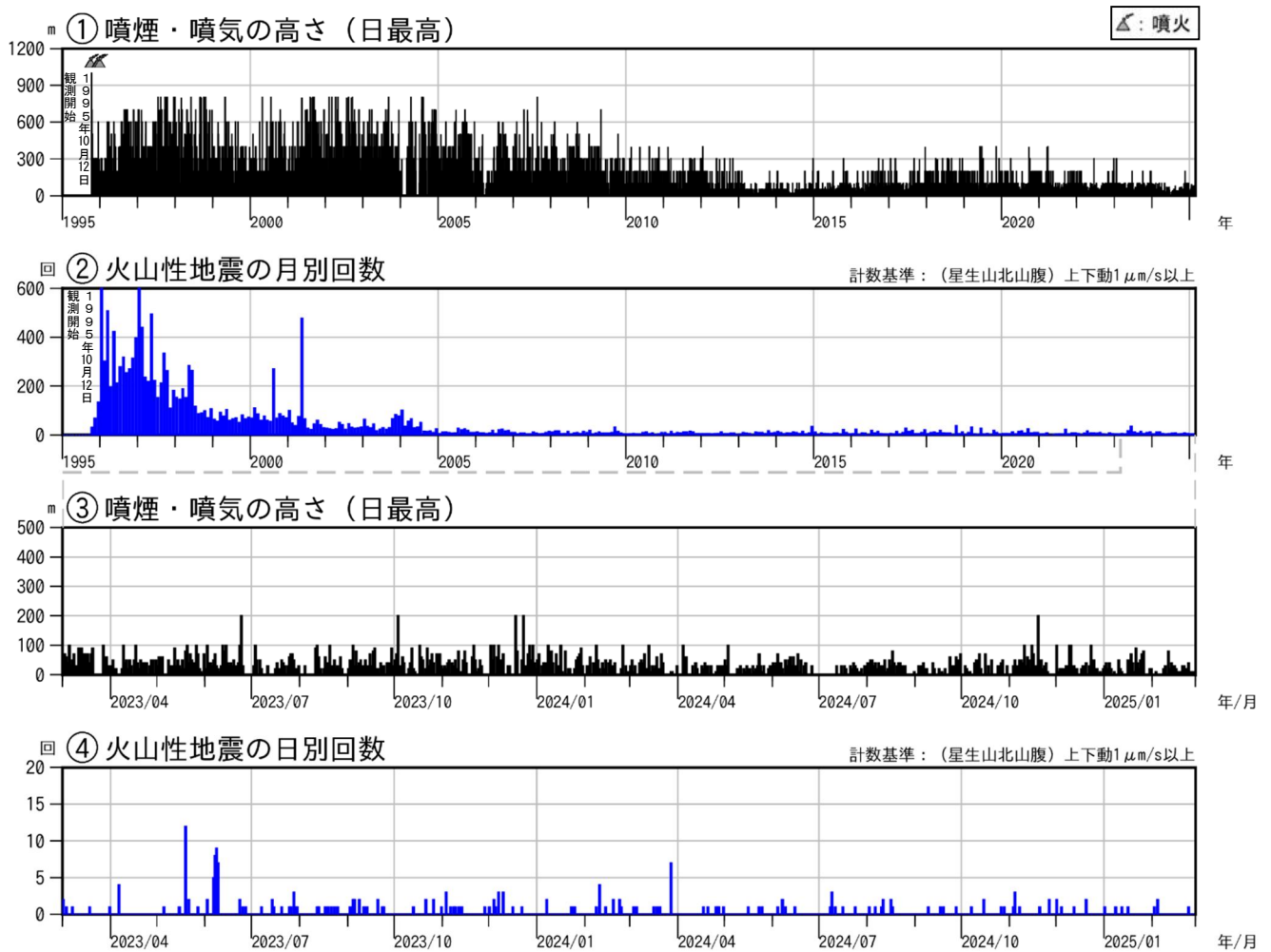
図2 九重山 火山活動経過図（1995年1月～2025年2月）
