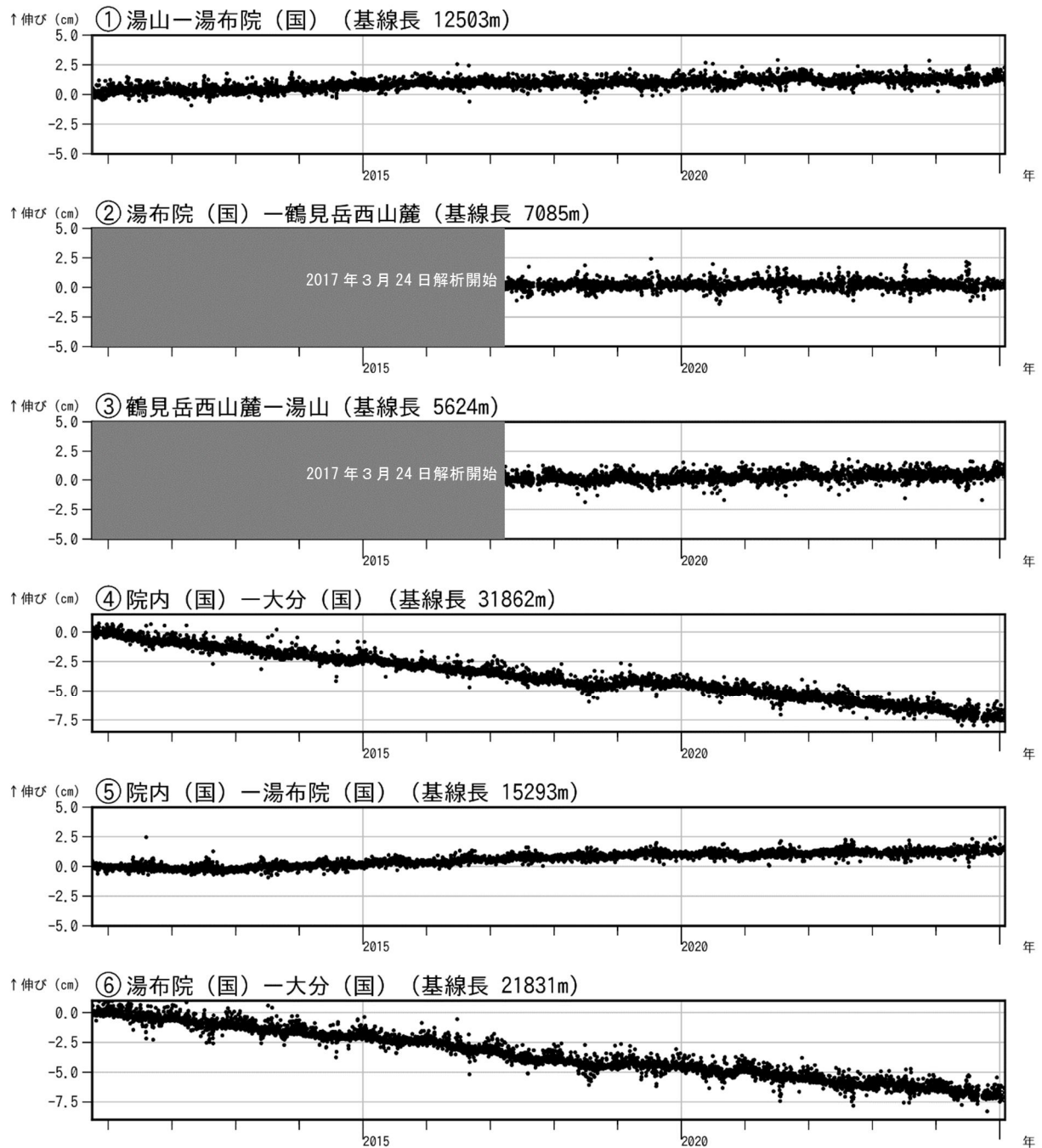
図4 鶴見岳・伽藍岳 GNSS連続観測による基線長変化（2010年10月～2025年1月）
