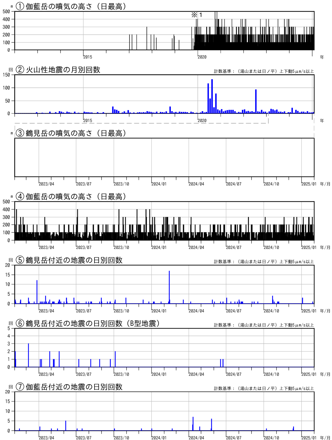
図2 鶴見岳・伽藍岳 火山活動経過図（2012年1月～2025年1月）
