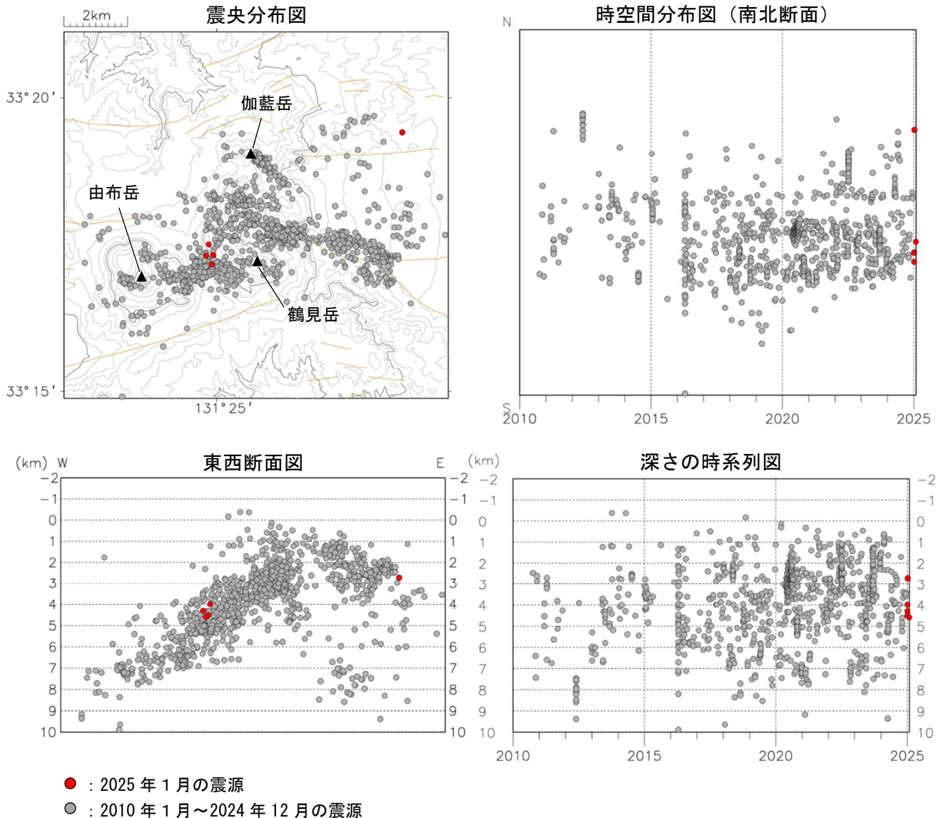
図3 鶴見岳・伽藍岳 震源分布図（2010 年 1 月～2025 年 1 月）
