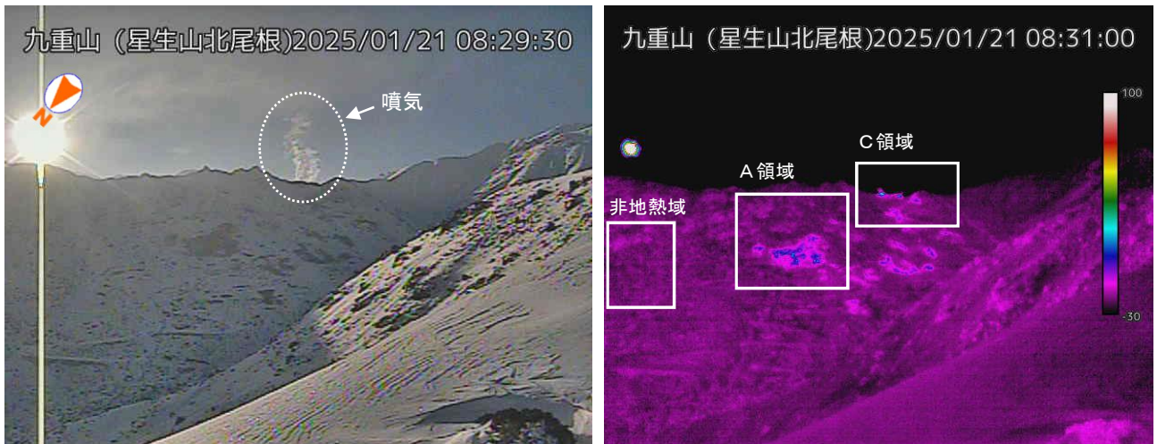
図 1-1 九重山 硫黄山の噴気及び地熱域の状況（1月21日 星生山北尾根監視カメラ）
