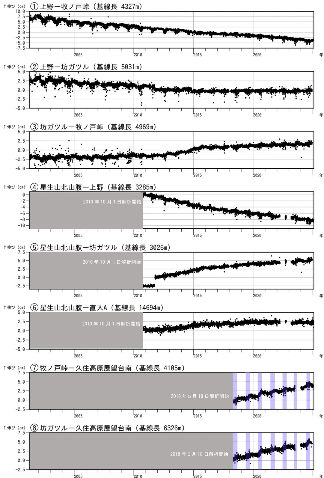
図5 九重山 GNSS 連続観測による基線長変化（2001年4月～2025年1月）
