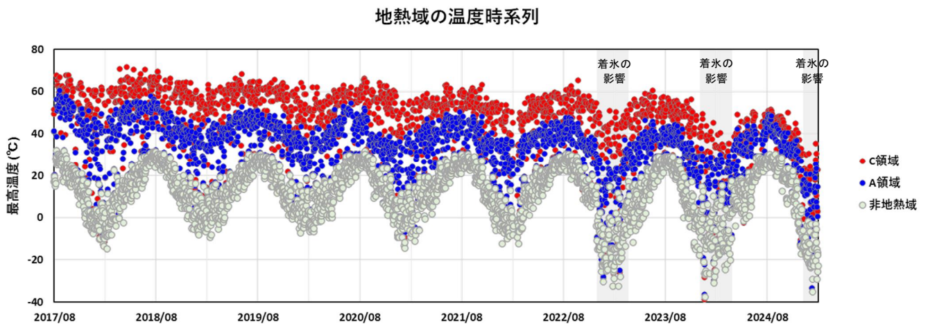
図 1-2 九重山 星生山北尾根の赤外熱映像装置による日別最高温度（2017 年 8 月～2025 年 1 月）
