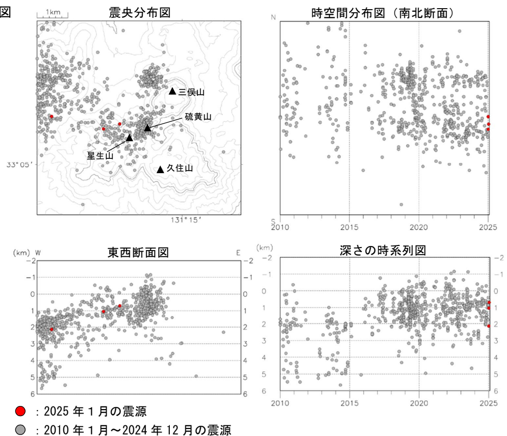
図 3 九重山 震源分布図 ①広域図 ②狭域図（2010 年 1 月～2025 年 1 月）
