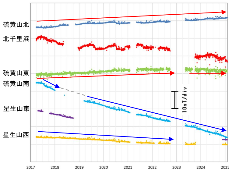
図 4-1 九重山 連続観測による全磁力の変化 (2017年3月～2025年1月)
