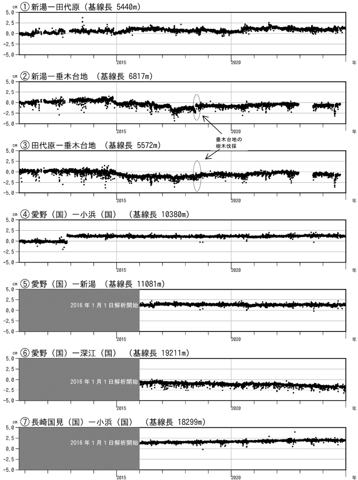
図5 雲仙岳 GNSS連続観測による基線長変化（2010年10月～2024年12月）
