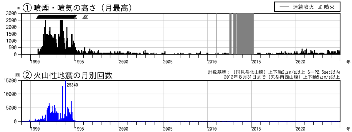
図2 雲仙岳 長期の火山活動経過図（1989年1月～2024年12月）
