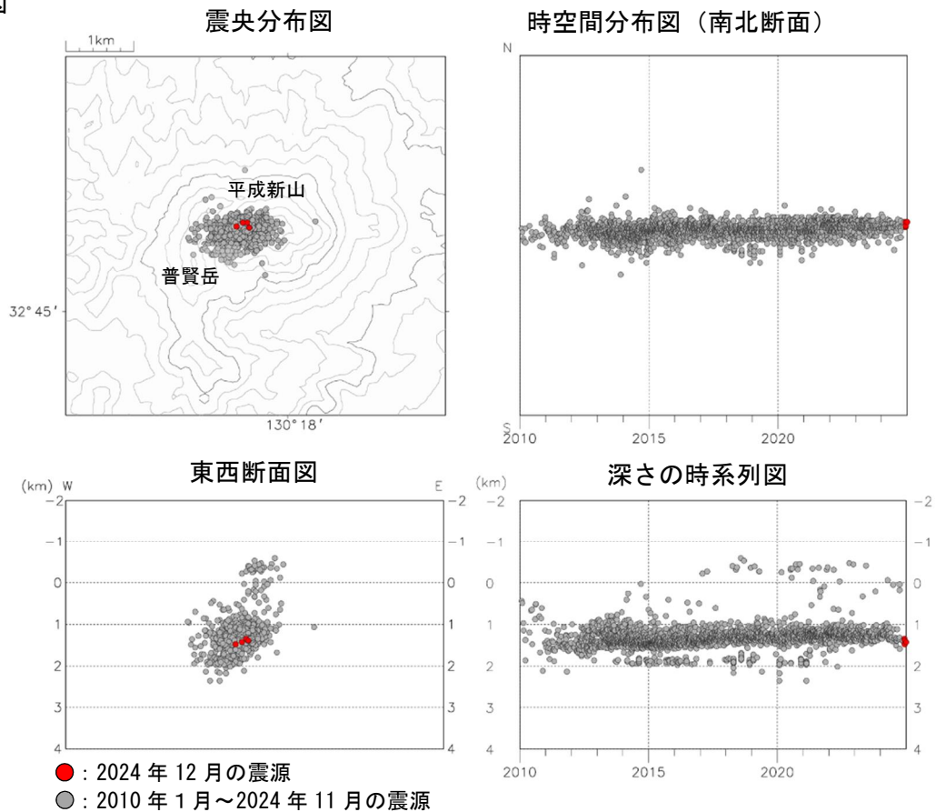
図4 雲仙岳 震源分布図 ①広域図 ②狭域図（2010年1月～2024年12月）
