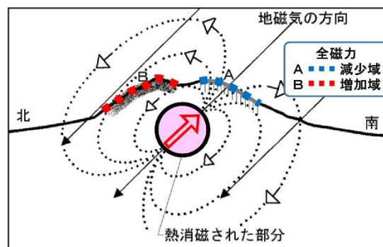
図 5-3 九重山 熱消磁に伴う全磁力変化のモデル 火山体周辺の全磁力変化と火山体内部の温度
