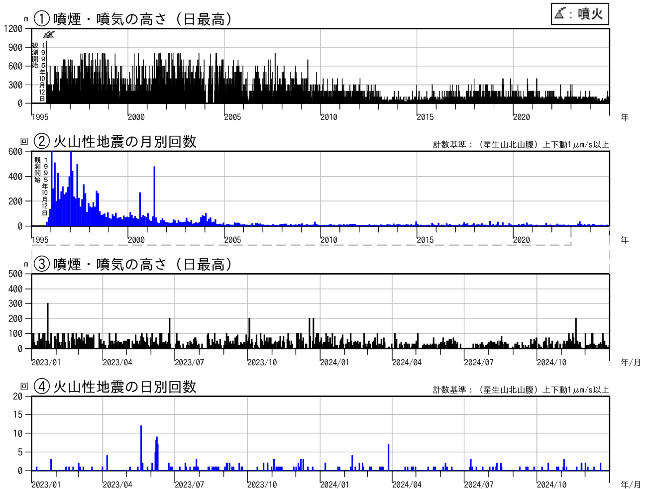
図3 九重山 火山活動経過図（1995年1月～2024年12月）
