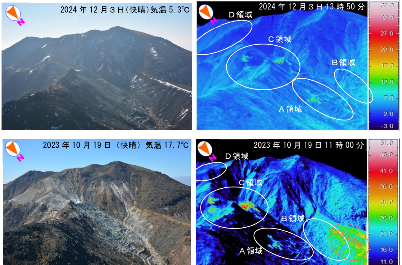
図 2-3 九重山 全領域（A、B、C、D）の可視画像及び赤外熱映像装置による地表面温度分布
