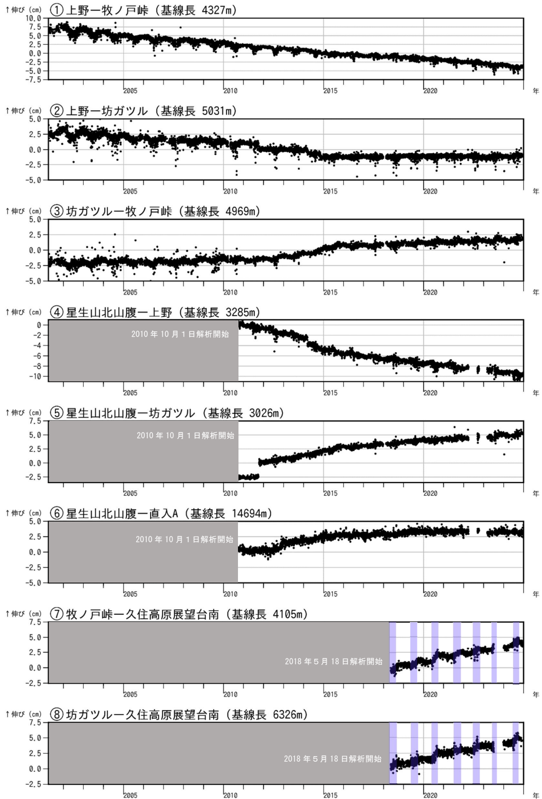
図6 九重山 GNSS 連続観測による基線長変化（2001年4月～2024年12月）
