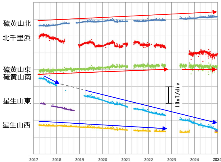
図 5-1 九重山 連続観測による全磁力の変化 (2017年3月～2024年12月)
