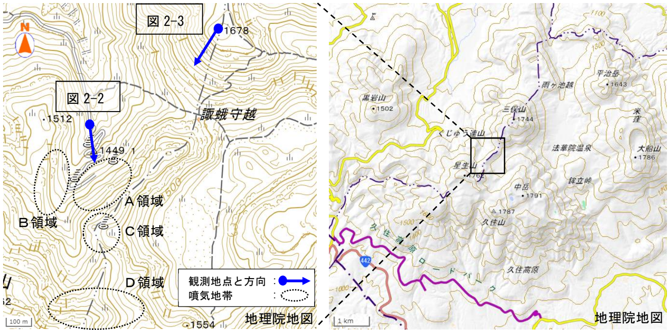
図 2-1 九重山 現地調査観測位置及び撮影方向
