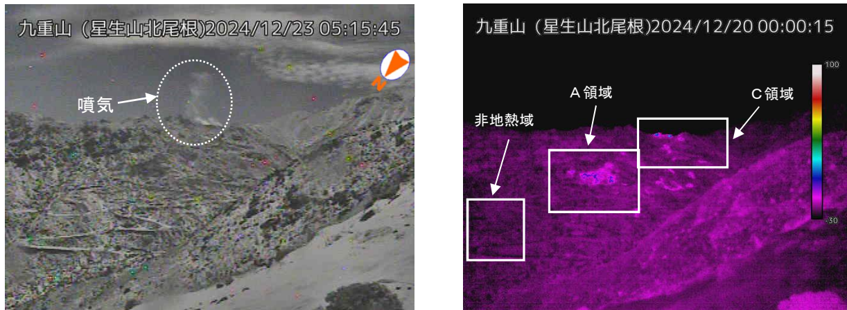
図 1-1 九重山 硫黄山の噴気（12 月 23 日）及び地熱域の状況（12 月 20 日） （星生山北尾根監視カメラ）
