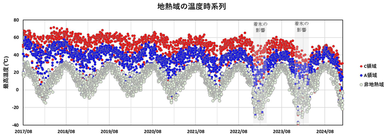
図 1-2 九重山 星生山北尾根の赤外熱映像装置による日別最高温度（2017 年 8 月～2024 年 12 月）
