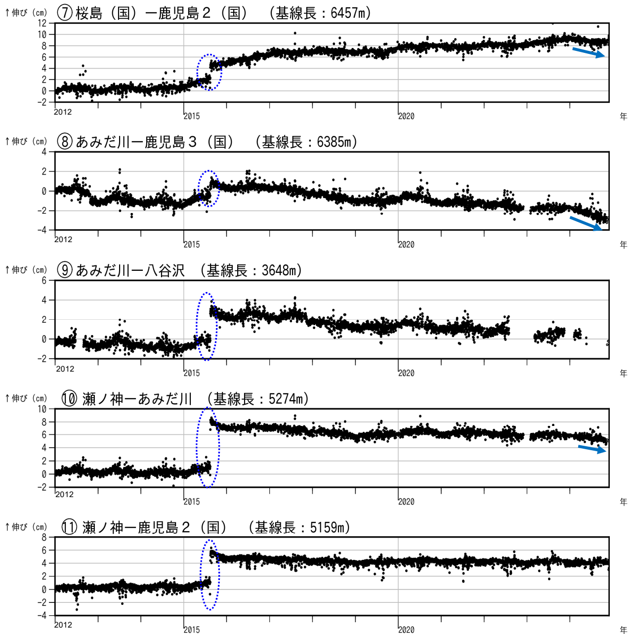
図 7-2 桜島 GNSS 連続観測による基線長変化（2012 年 1 月～2024 年 11 月）
