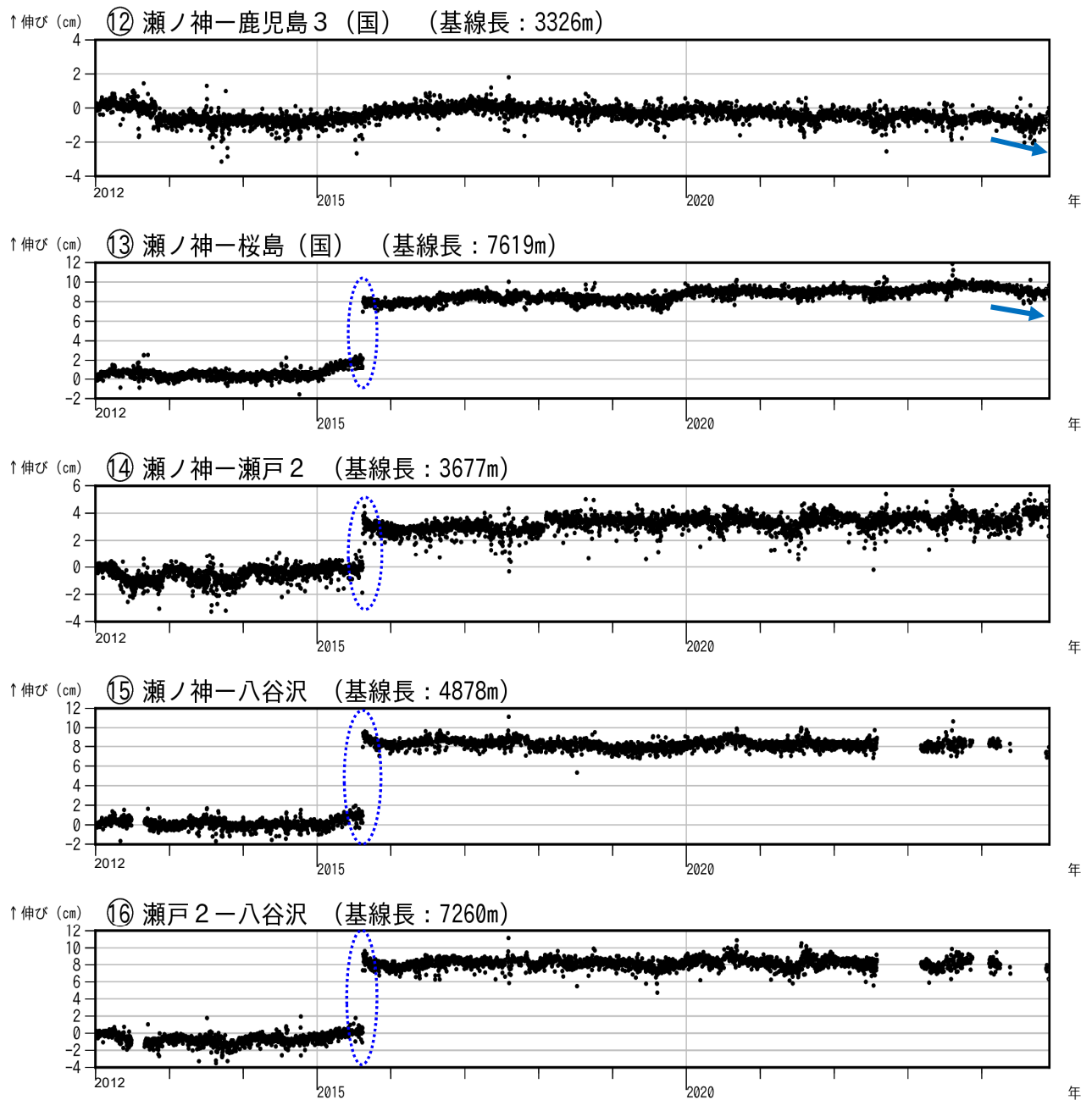
図 7-3 桜島 GNSS 連続観測による基線長変化（2012 年 1 月～2024 年 11 月）
