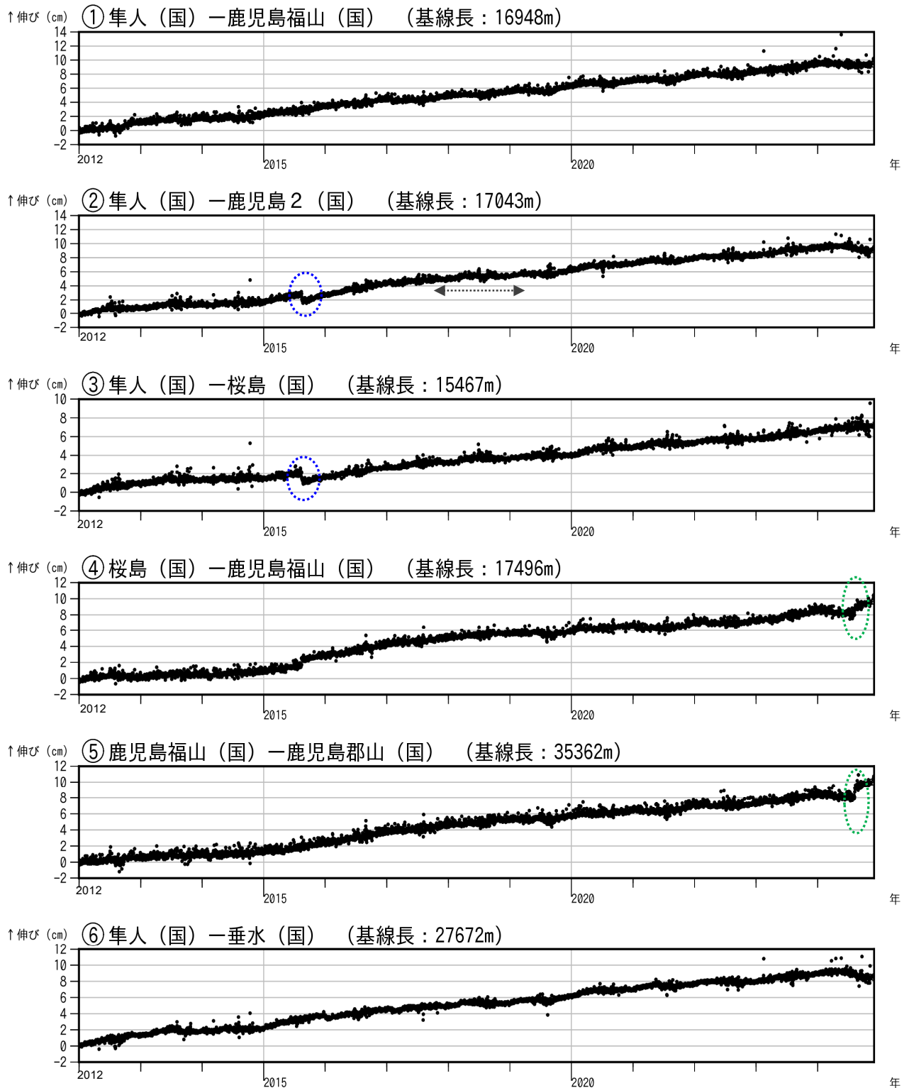
図 7-1 桜島 GNSS 連続観測による基線長変化 (2012 年 1 月～2024 年 11 月)
