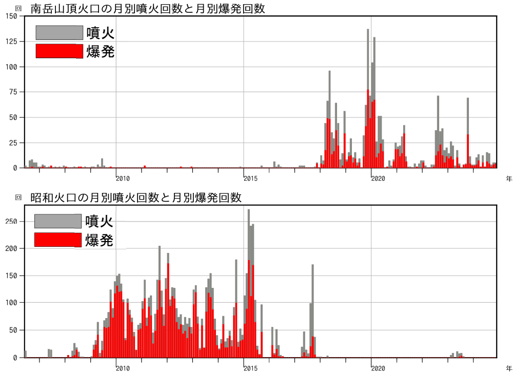
図3 桜島 南岳山頂火口（上図）と昭和火口（下図）の月別噴火回数と月別爆発回数 （2006年6月～2024年11月）
