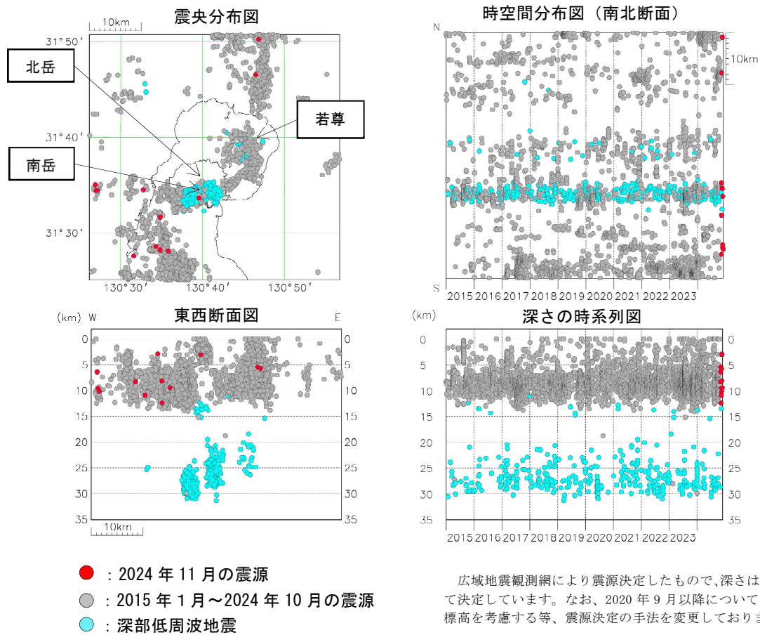
図 2-1 桜島 始良カルデラ周辺の震源分布図（2015 年 1 月～2024 年 11 月）
