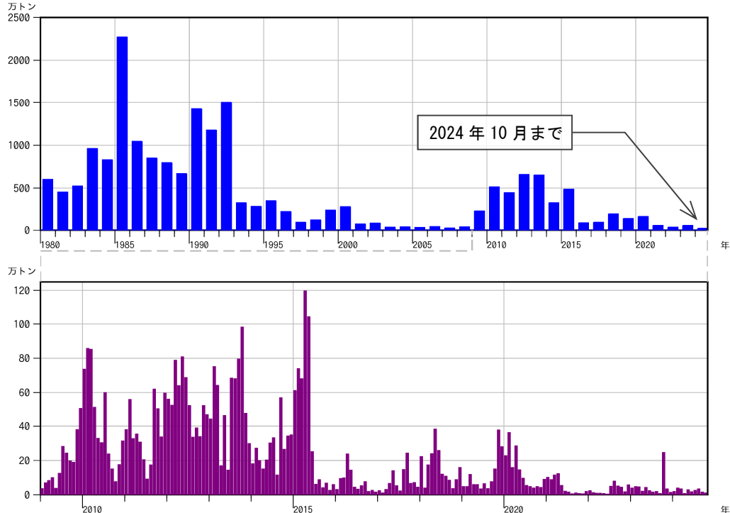
図4 桜島 鹿児島県が実施している降灰の観測データから推定した火山灰の総噴出量 （上段：1980年1月～2024年10月までの年別値、下段：2009年1月～2024年10月の月別値）
