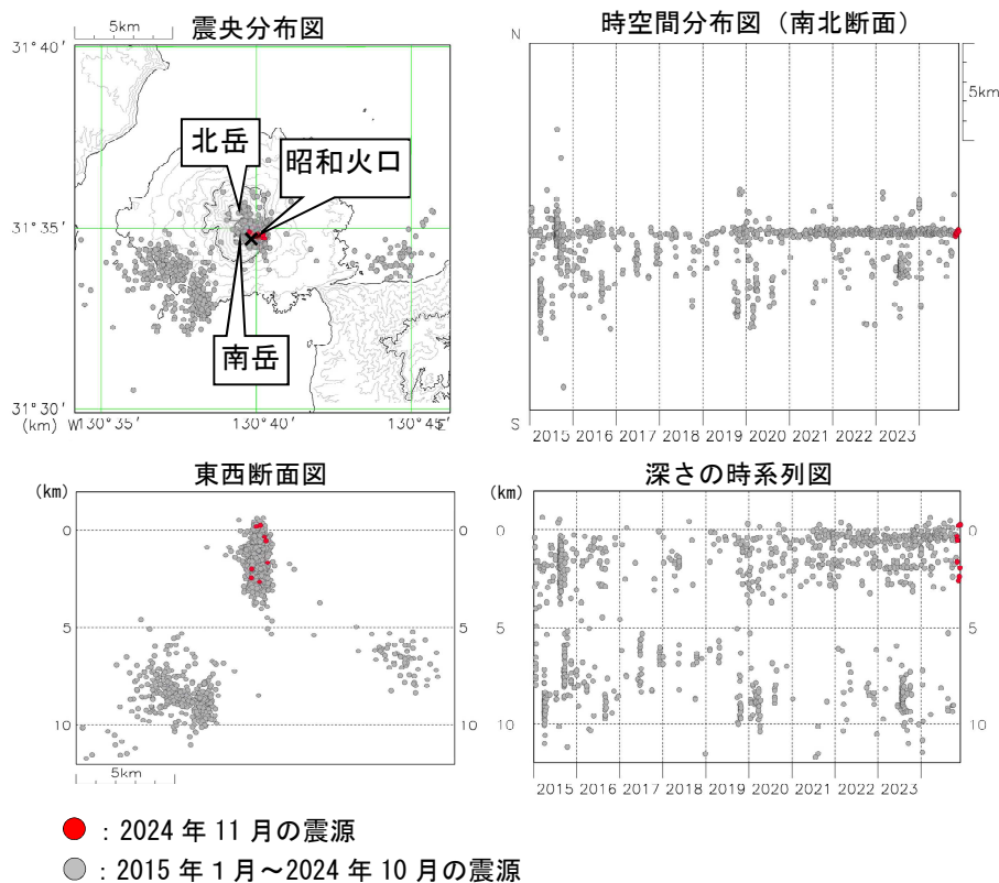
図 2-2 桜島 桜島付近の震源分布図（2015 年 1 月～2024 年 11 月）
