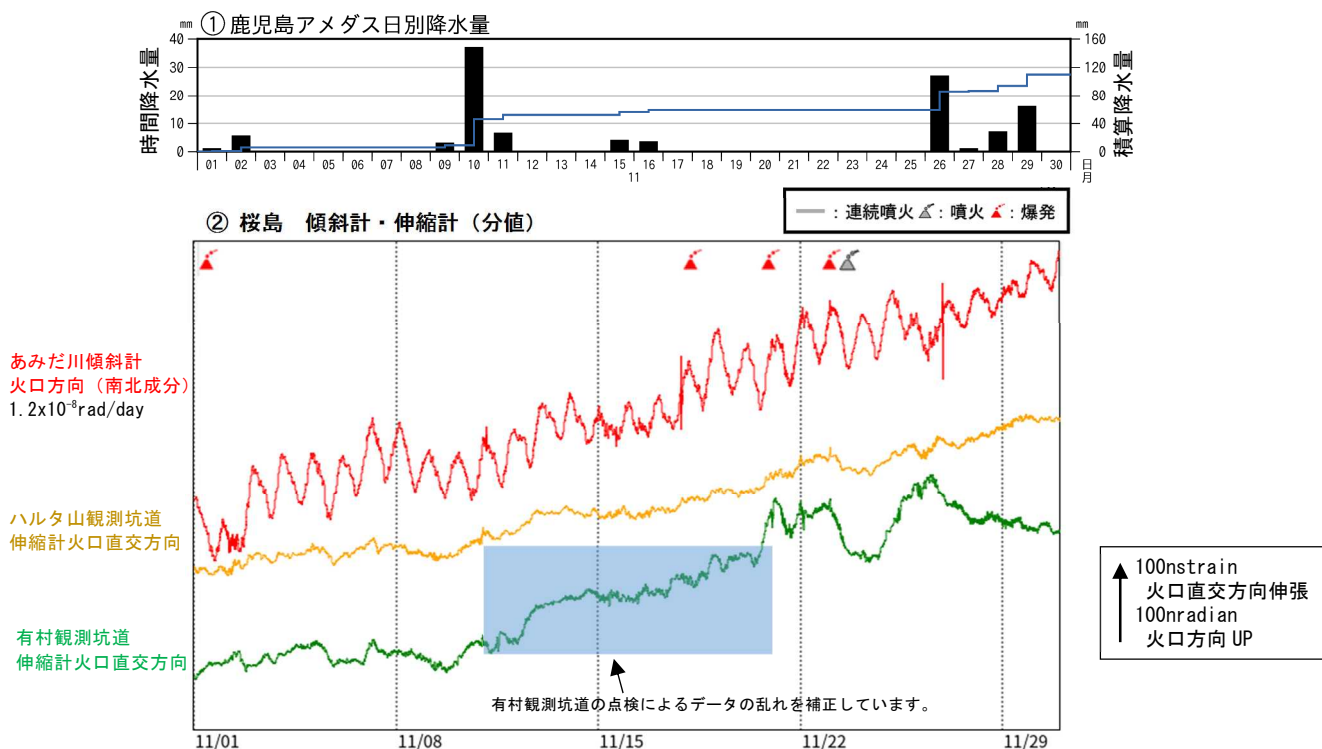
図6 桜島 傾斜計及び伸縮計による地殻変動の状況（2024年11月1日～11月30日）
