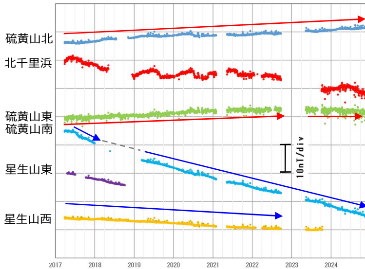
図 4-1 九重山 連続観測による全磁力の変化 (2017年3月～2024年11月)
