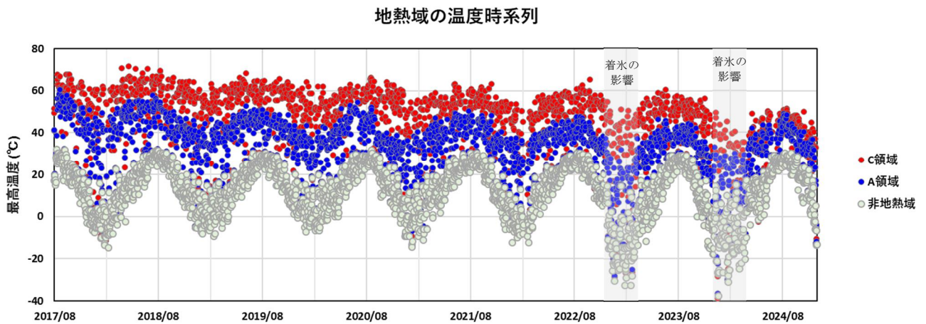
図 1-2 九重山 星生山北尾根の赤外熱映像装置による日別最高温度（2017 年 8 月～2024 年 11 月）
