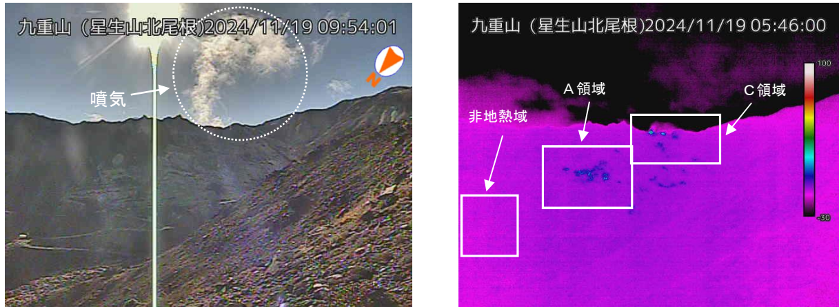
図 1-1 九重山 硫黄山の噴気及び地熱域の状況（11 月 19 日 星生山北尾根監視カメラ）
