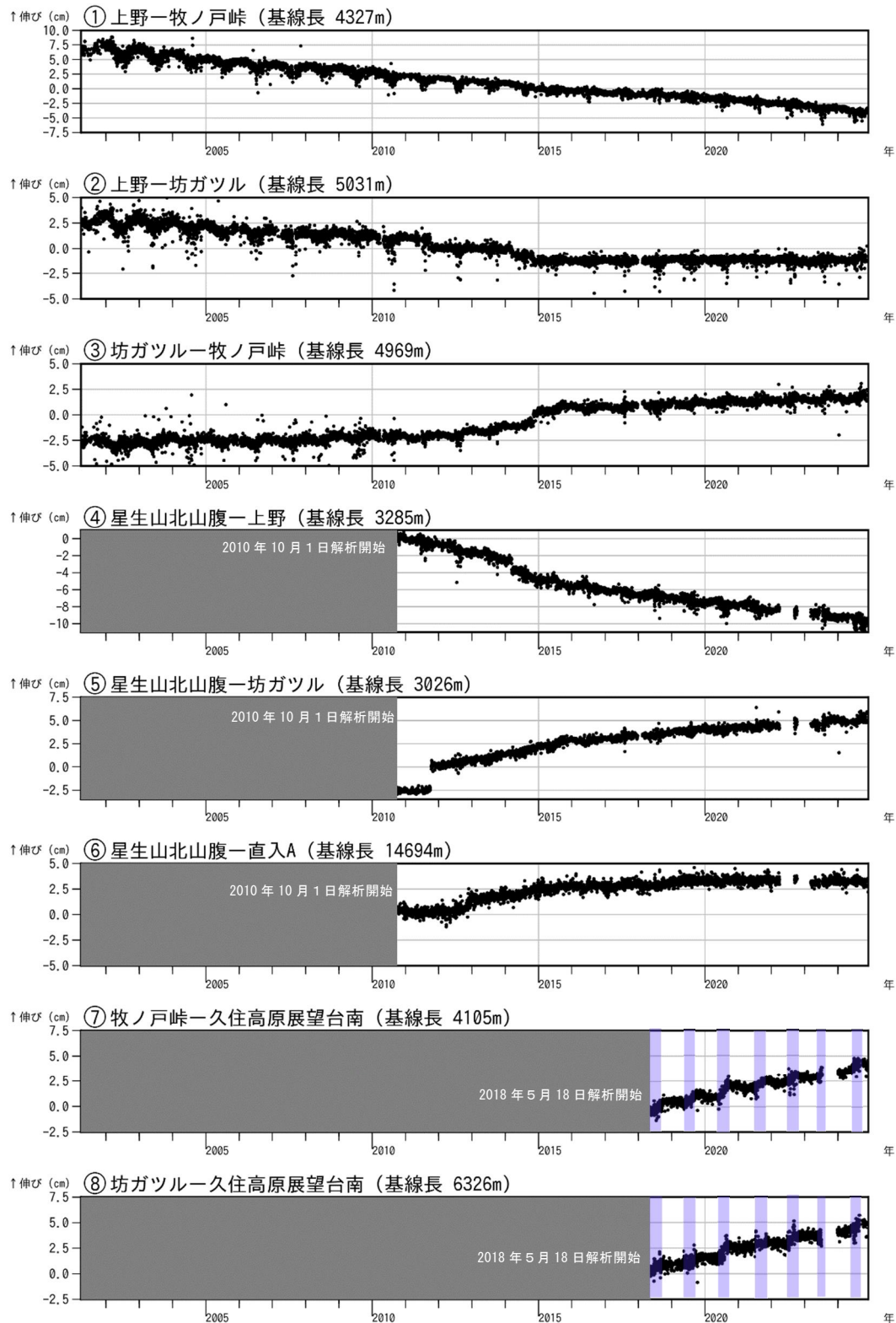
図5 九重山 GNSS 連続観測による基線長変化（2001年4月～2024年11月）
