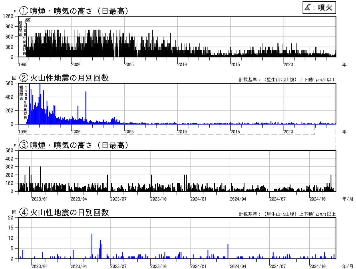
図2 九重山 火山活動経過図（1995年1月～2024年11月）
