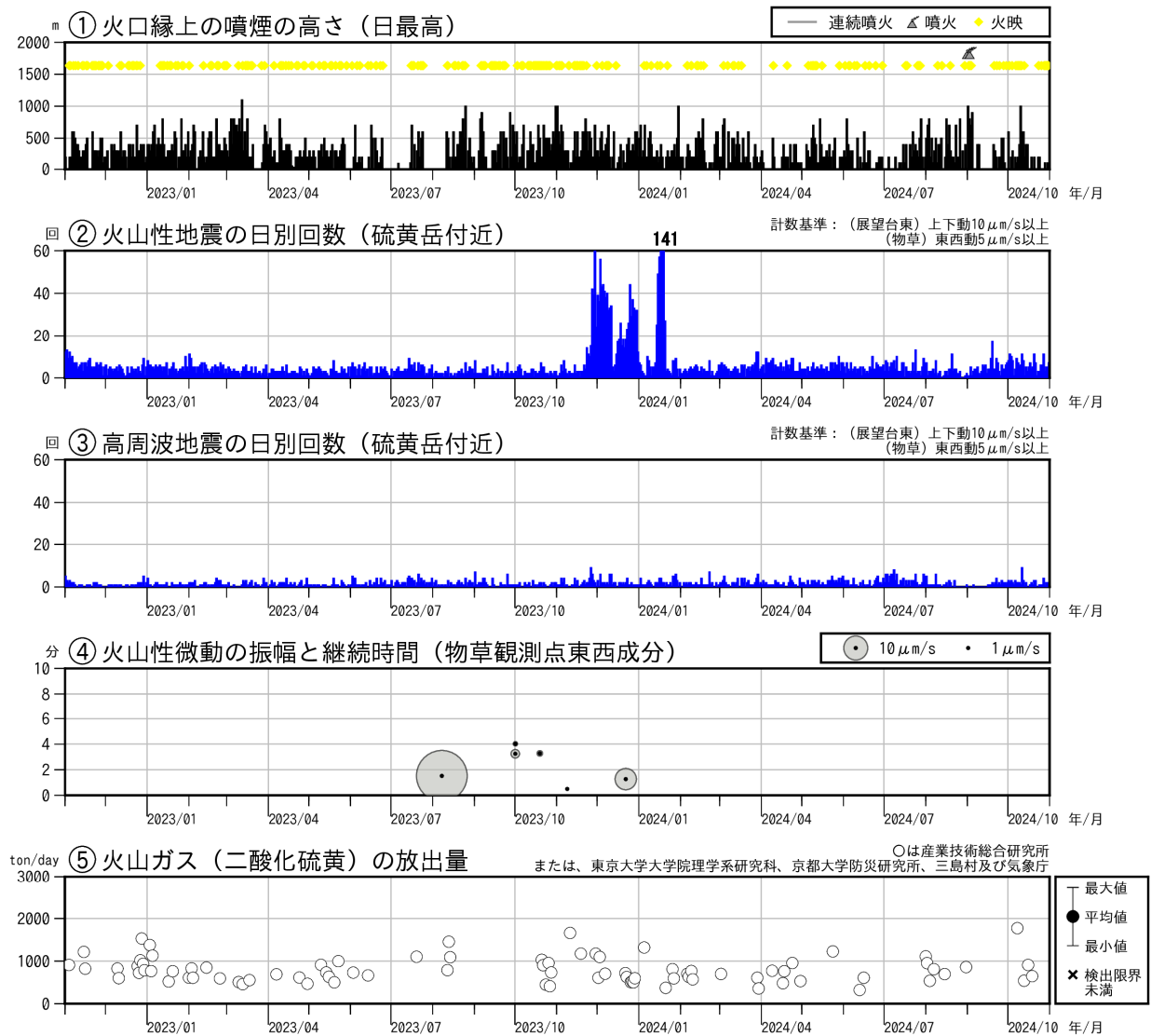
図4 薩摩硫黄島 火山活動経過図（2022年11月～2024年10月）
