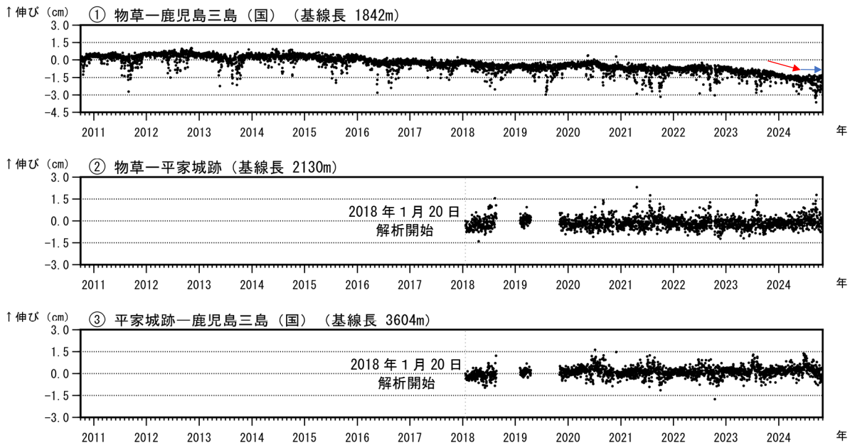
図5 薩摩硫黄島 GNSS連続観測による基線長変化（2010年10月～2024年10月）
