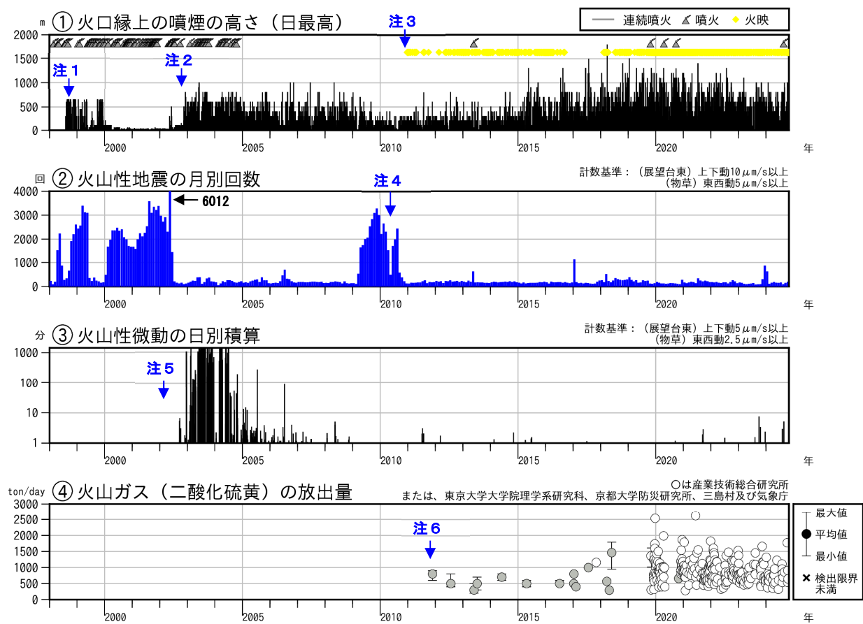
図3 薩摩硫黄島 火山活動経過図（1998年1月～2024年10月）
