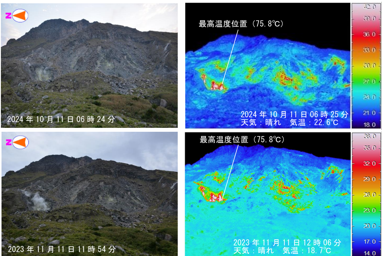
図 2-2 薩摩硫黄島 硫黄岳の状況
