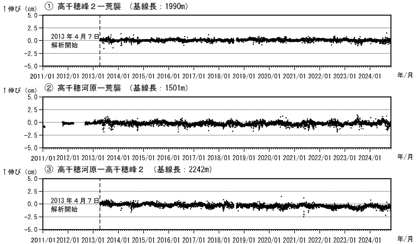
図4 霧島山（御鉢） GNSS 連続観測による基線長変化（2011年1月～2024年10月）
