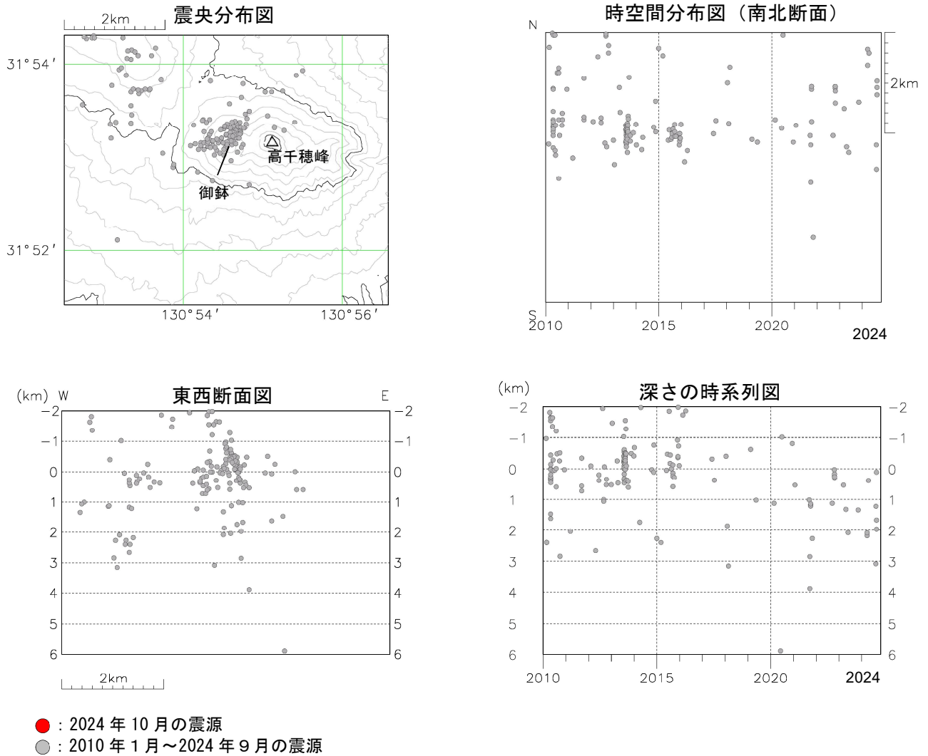
図2 霧島山（御鉢） 震源分布図（2010年1月～2024年10月）
