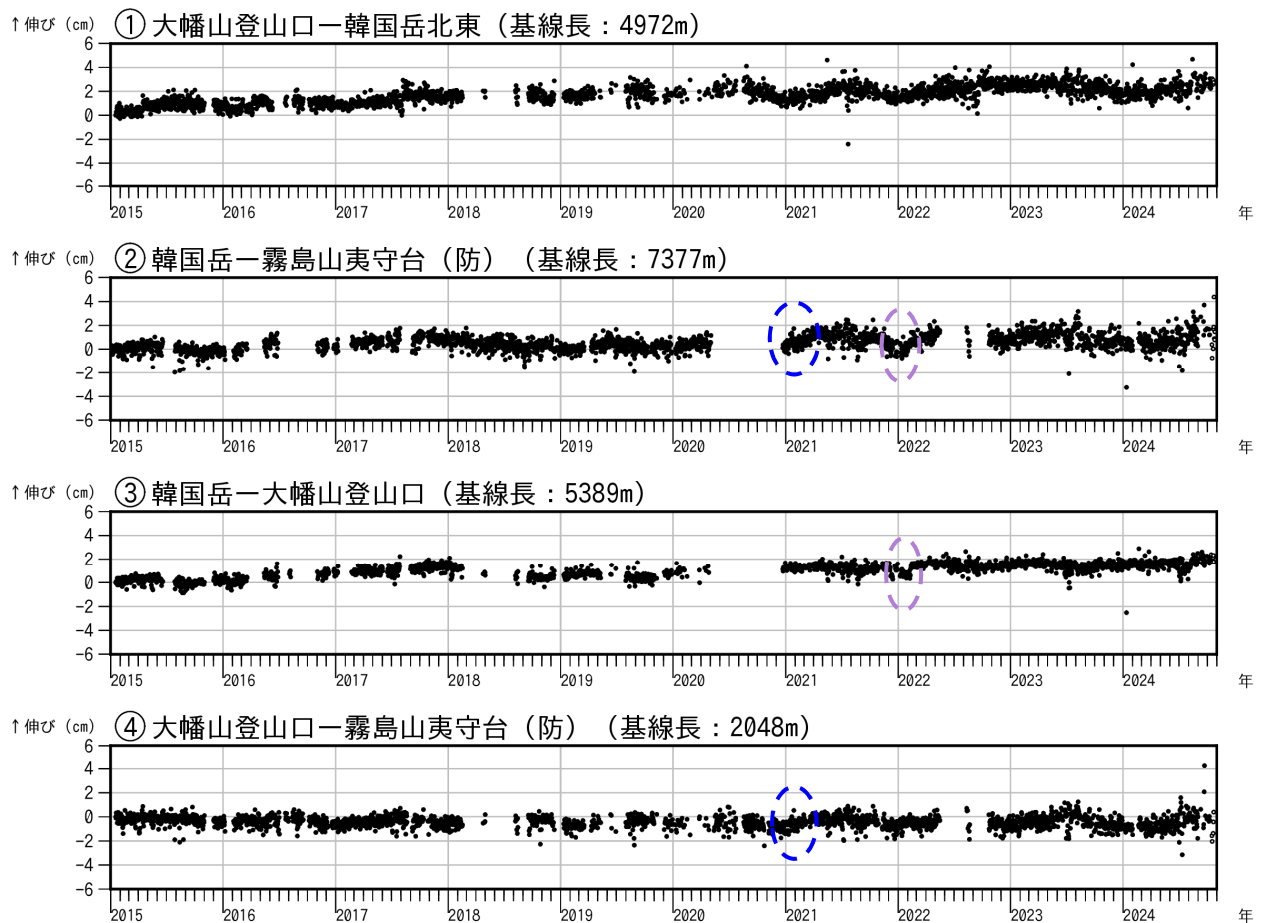
図4 霧島山（大幡池） GNSS 連続観測による基線長変化（2015年1月～2024年10月）
