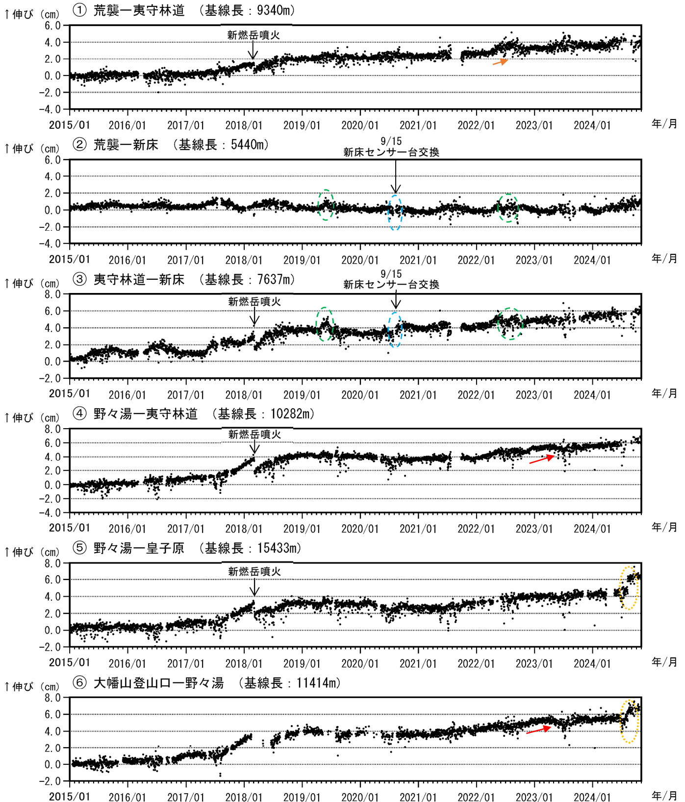
図4 霧島山（新燃岳） GNSS 連続観測による基線長変化（2015年1月～2024年10月）
