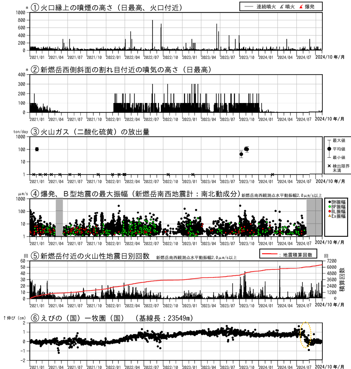
図2 霧島山（新燃岳） 火山活動経過図（2021年1月～2024年10月）
