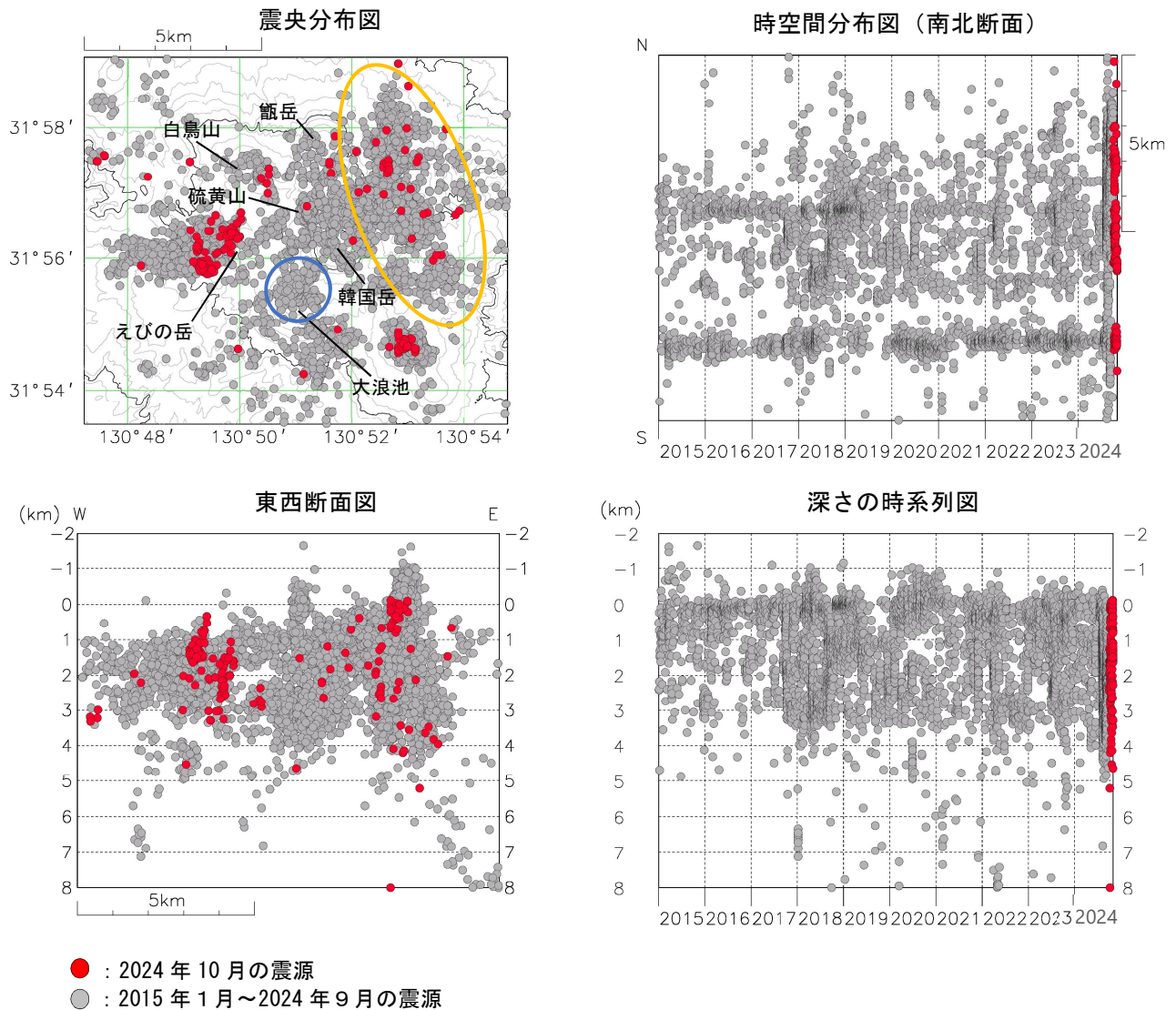
図4 霧島山（えびの高原（硫黄山）周辺） 震源分布図（2015 年 1 月～2024 年 10 月）
