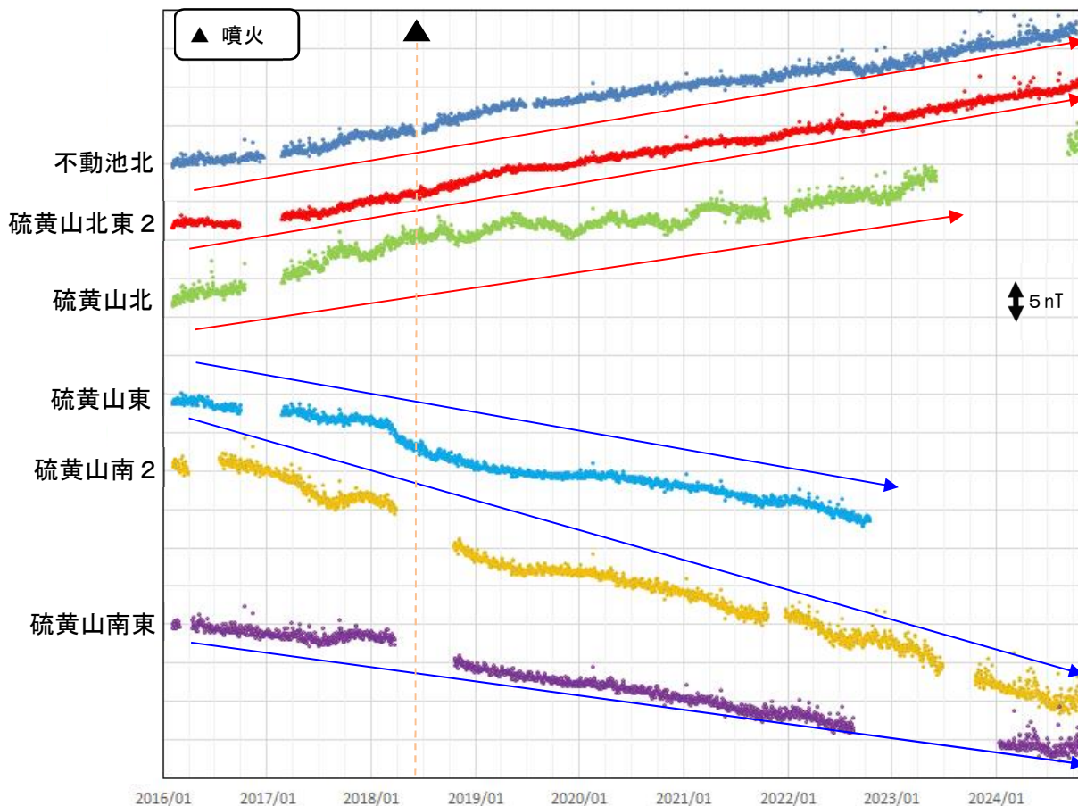
図 6-2 霧島山（えびの高原（硫黄山）周辺） 全磁力観測点で観測された全磁力変動 (2016 年 1 月～2024 年 10 月)
