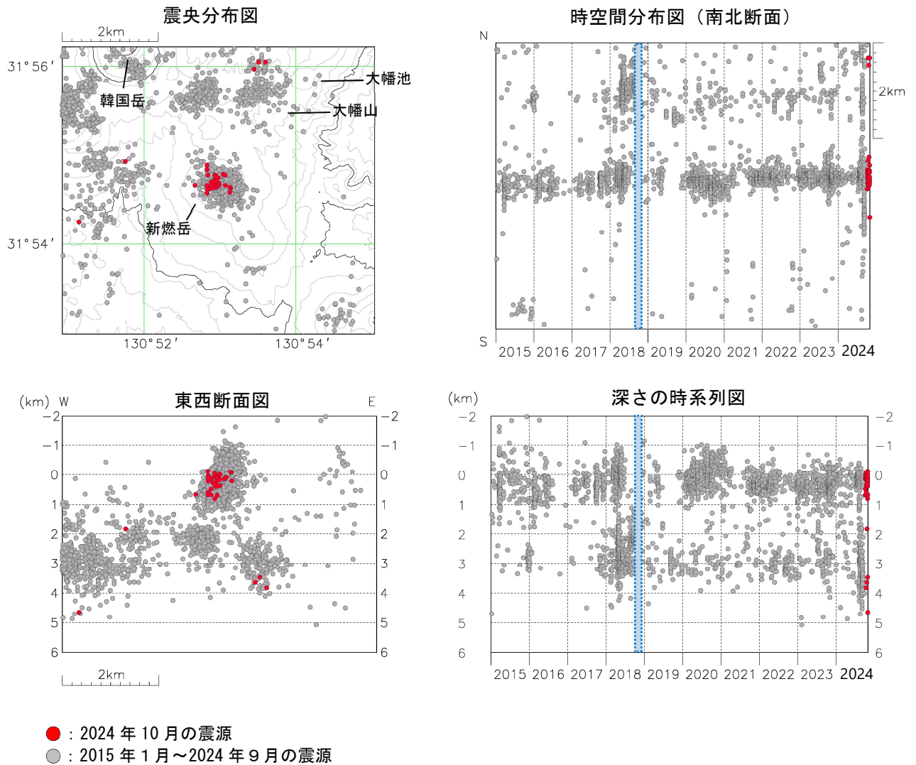
図3 霧島山（新燃岳） 震源分布図（2015 年 1 月～2024 年 10 月）
