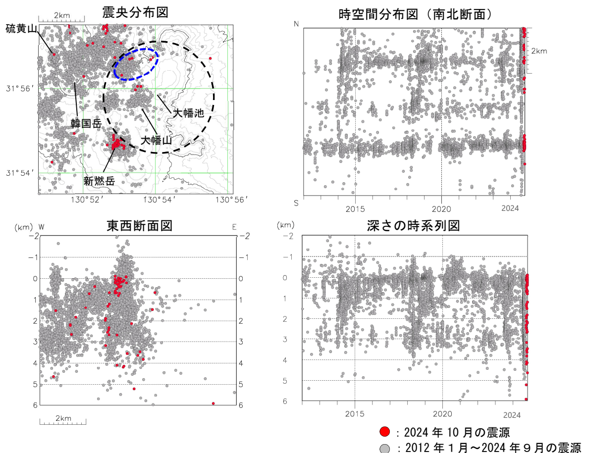
図3 霧島山（大幡池） 震源分布図（2012年1月～2024年10月）
