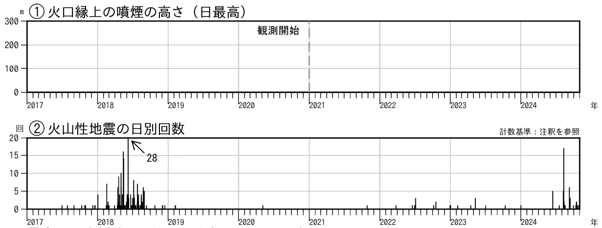
図2 霧島山（大幡池） 火山活動経過図（2017年1月～2024年10月）
