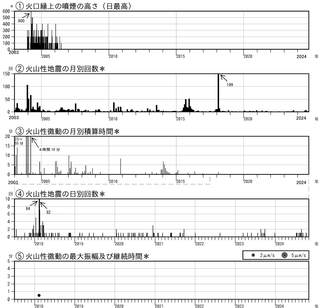
図3 霧島山（御鉢） 火山活動経過図（2003年1月～2024年10月）
