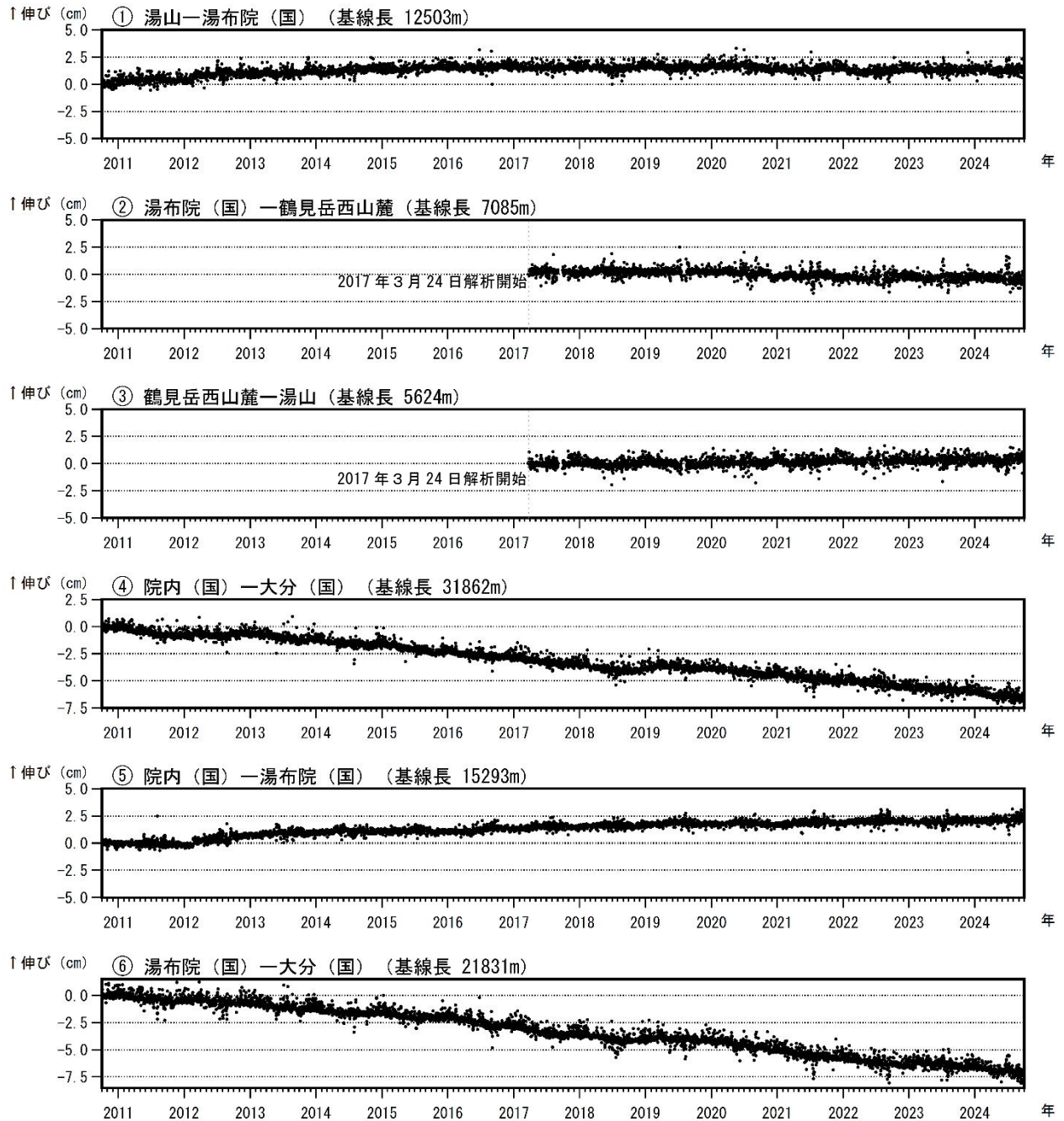
図4 鶴見岳・伽藍岳 GNSS連続観測による基線長変化（2010年10月～2024年9月）
