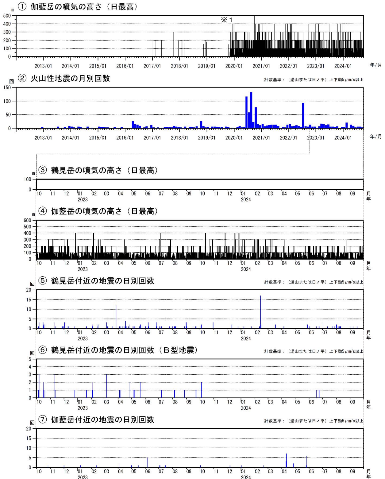
図2 鶴見岳・伽藍岳 火山活動経過図（2012年1月～2024年9月）
