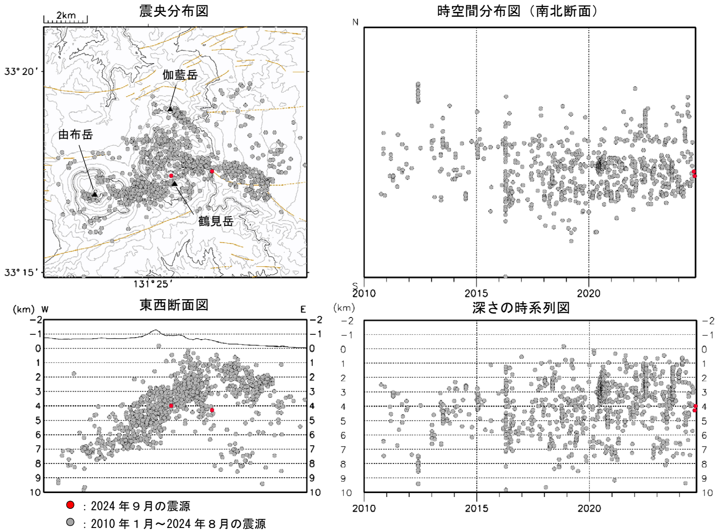
図3 鶴見岳・伽藍岳 震源分布図（2010年1月～2024年9月）
