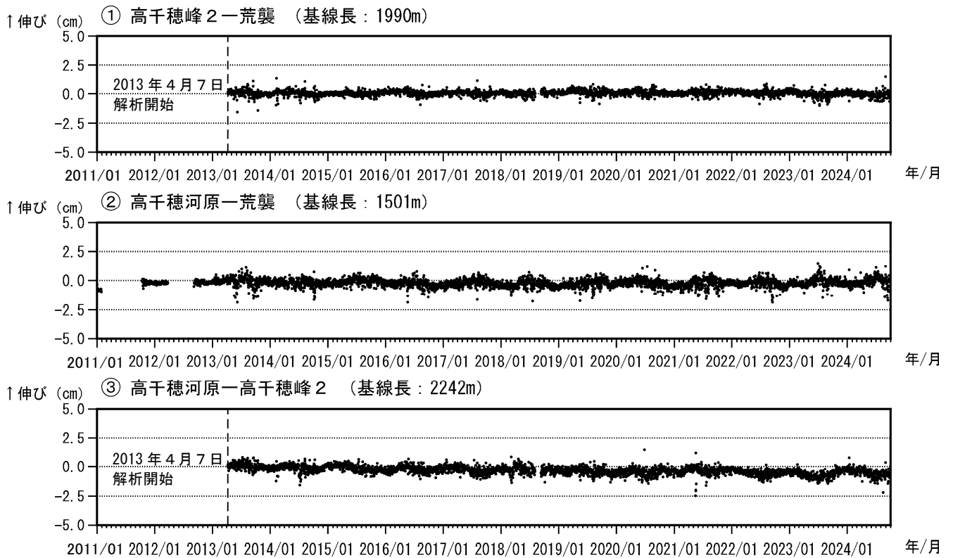
図4 霧島山（御鉢） GNSS 連続観測による基線長変化（2011年1月～2024年9月）
