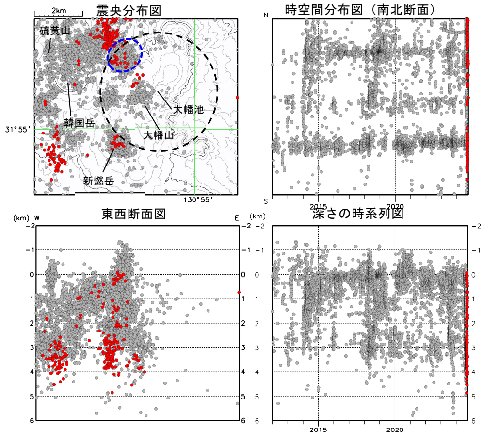
図3 霧島山（大幡池） 震源分布図（2012年1月～2024年9月）
