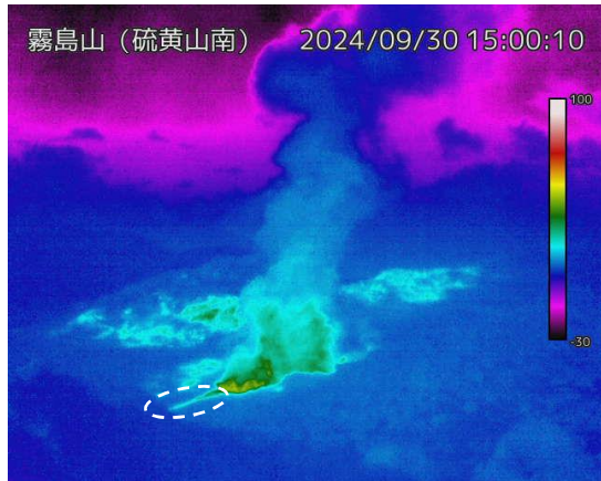
図 1-2 霧島山（えびの高原（硫黄山）周辺） 硫黄山南側の状況 （9月30日、硫黄山南監視カメラ）
