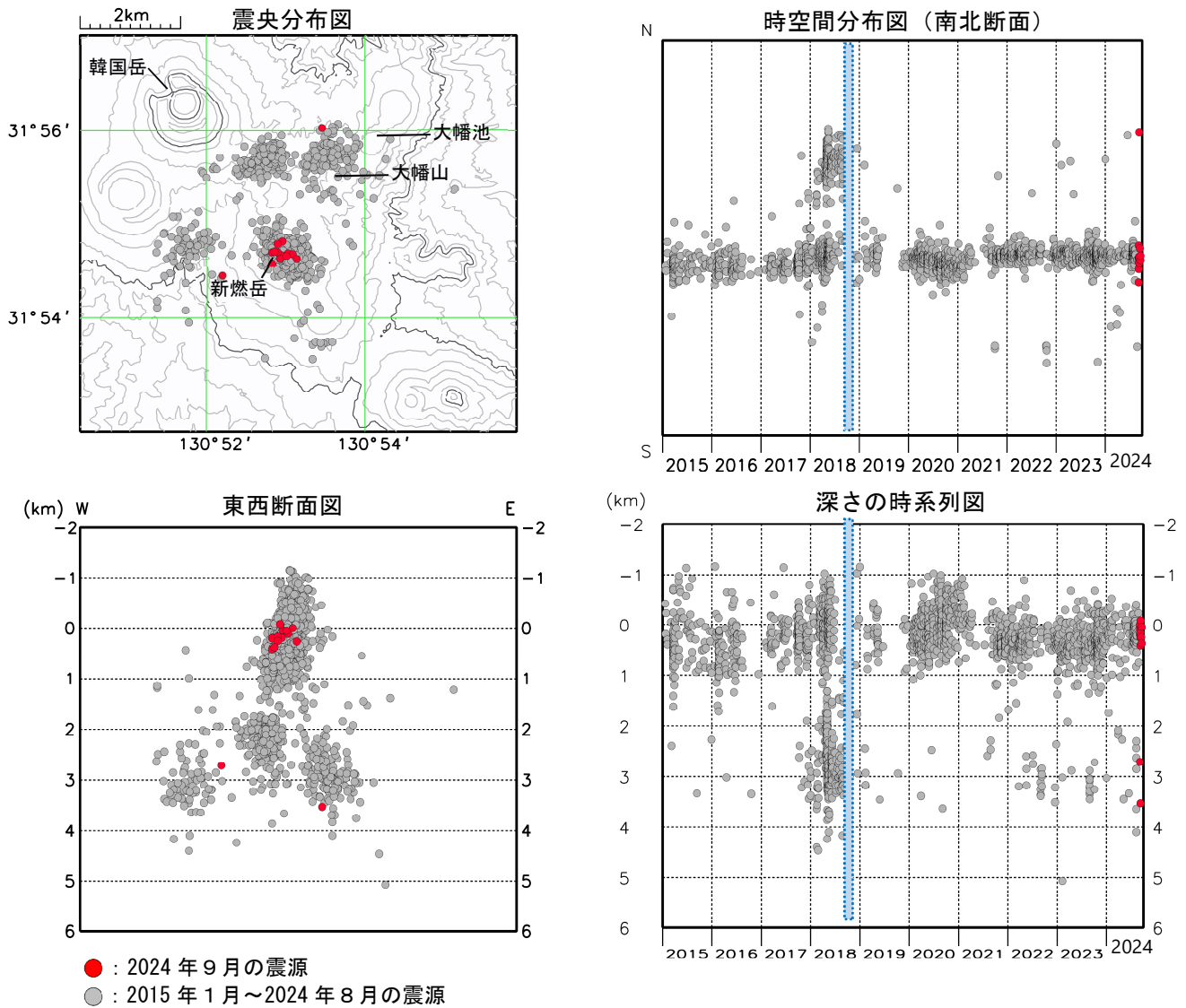
図3 霧島山（新燃岳） 震源分布図（2015 年 1 月～2024 年 9 月）
