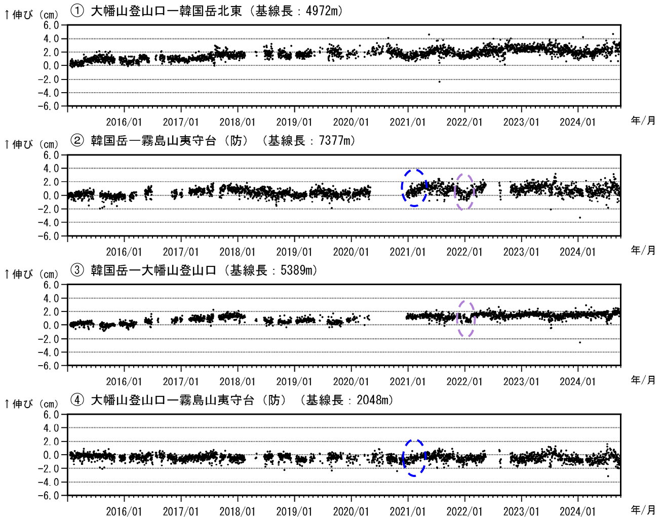
図4 霧島山（大幡池） GNSS 連続観測による基線長変化（2015年1月～2024年9月）
