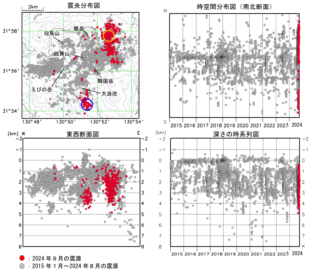
図6 霧島山（えびの高原（硫黄山）周辺） 震源分布図（2015 年 1 月～2024 年 9 月）
