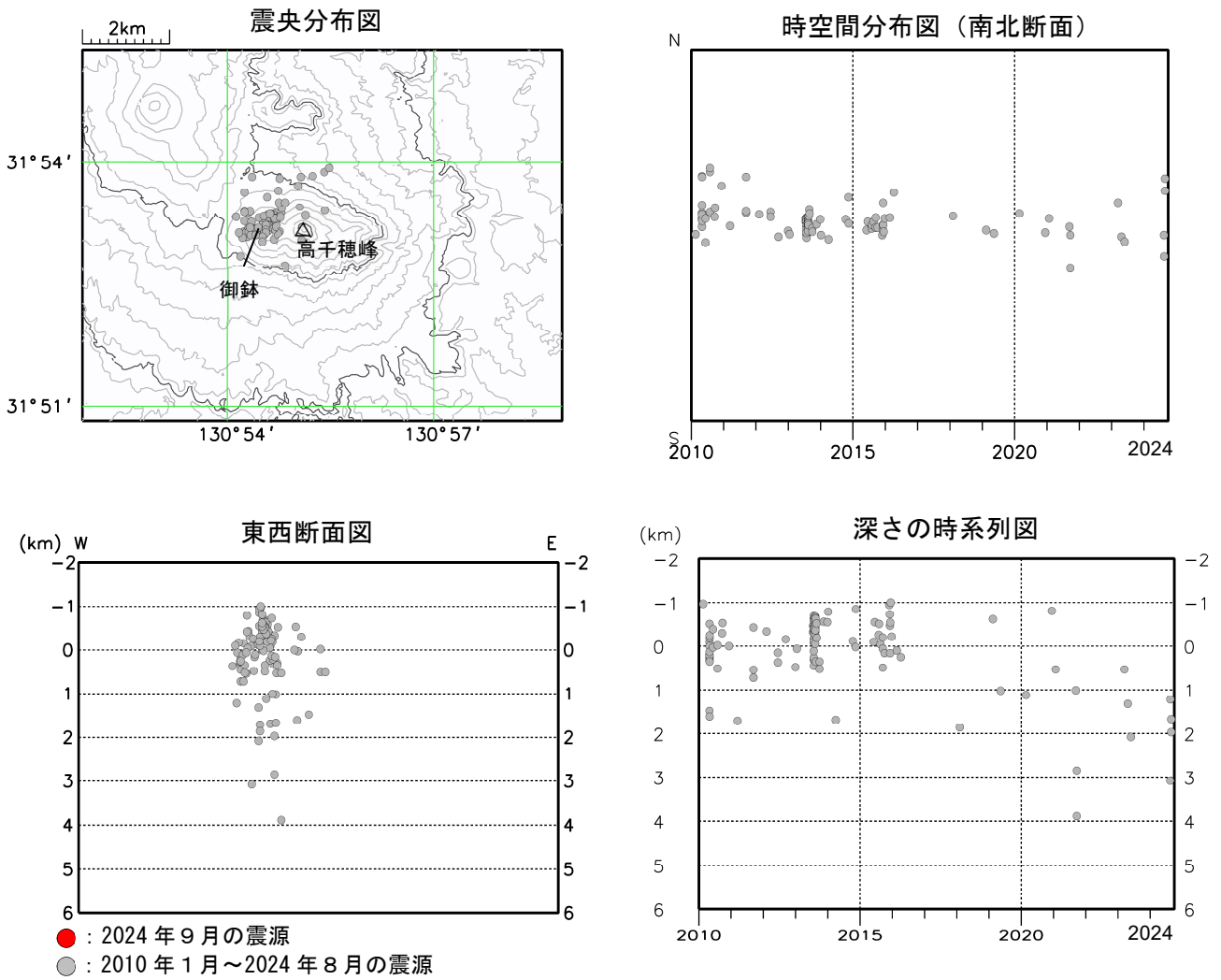
図2 霧島山（御鉢） 震源分布図（2010年1月～2024年9月）
