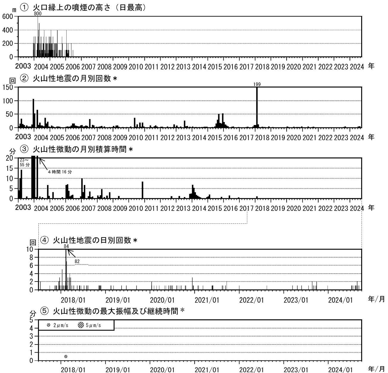
図3 霧島山（御鉢） 火山活動経過図（2003年1月～2024年9月）
