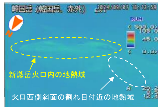
図 1 霧島山（新燃岳） 噴煙及び地熱域の状況（9 月 7 日、韓国岳監視カメラ）
