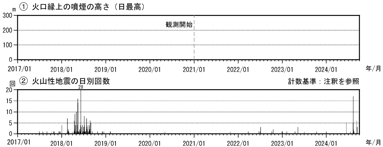
図2 霧島山（大幡池） 火山活動経過図（2017年1月～2024年9月）
