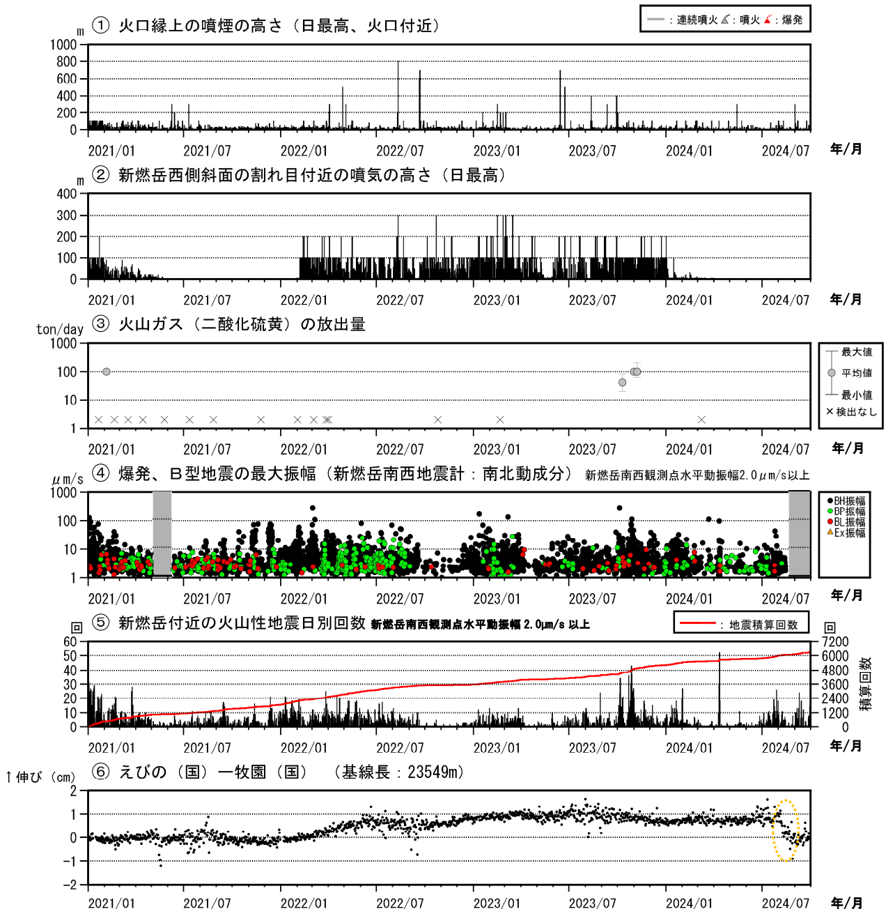
図2 霧島山（新燃岳） 火山活動経過図（2021年1月～2024年9月）
