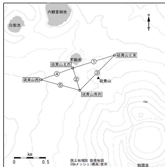
図5 霧島山（えびの高原（硫黄山）周辺） 図4及び図7のGNSS連続観測点と基線番号 白丸（○）は気象庁の観測点位置を示しています。
