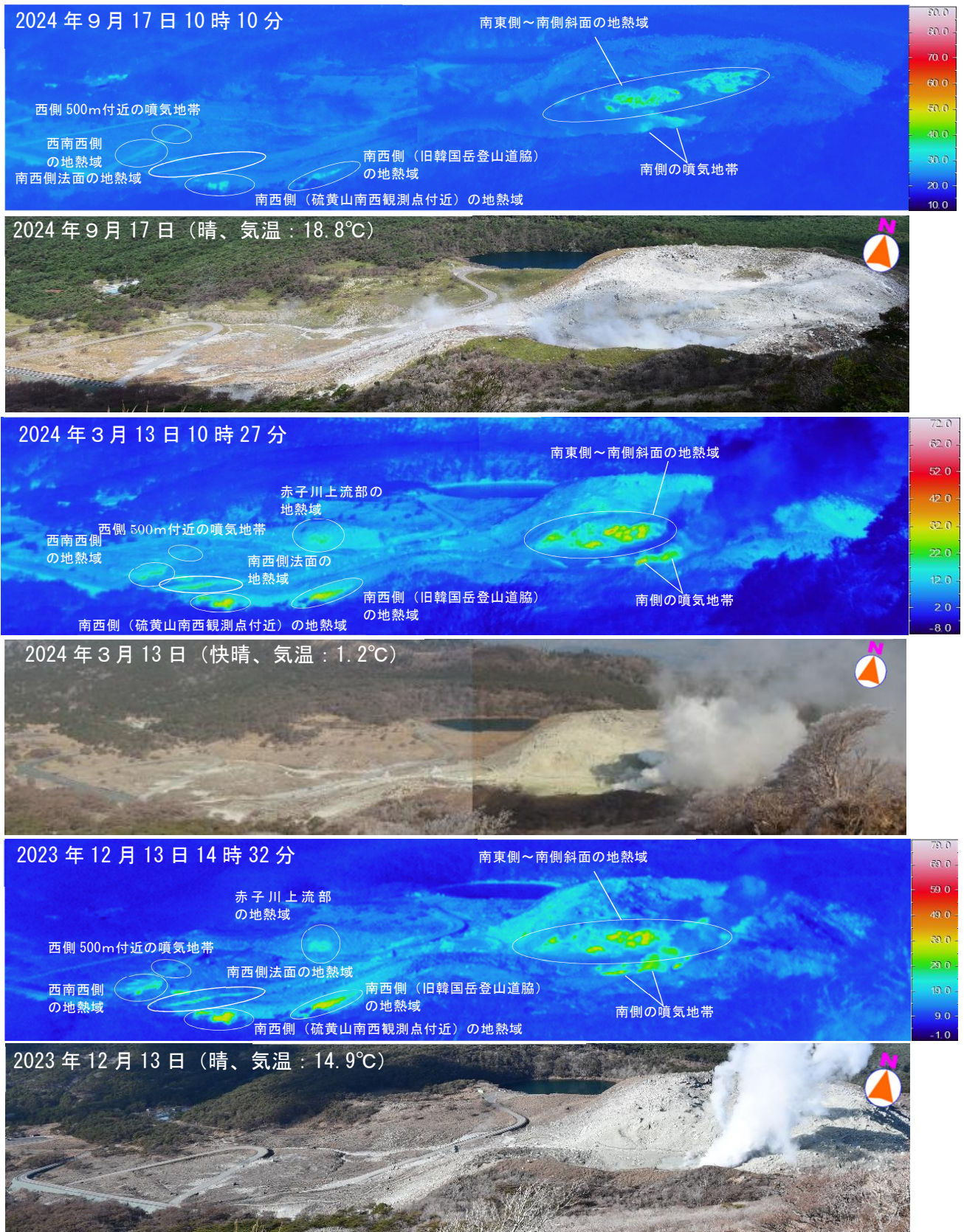
図3 霧島山（えびの高原（硫黄山）周辺 硫黄山の火口及びその周辺の状況
