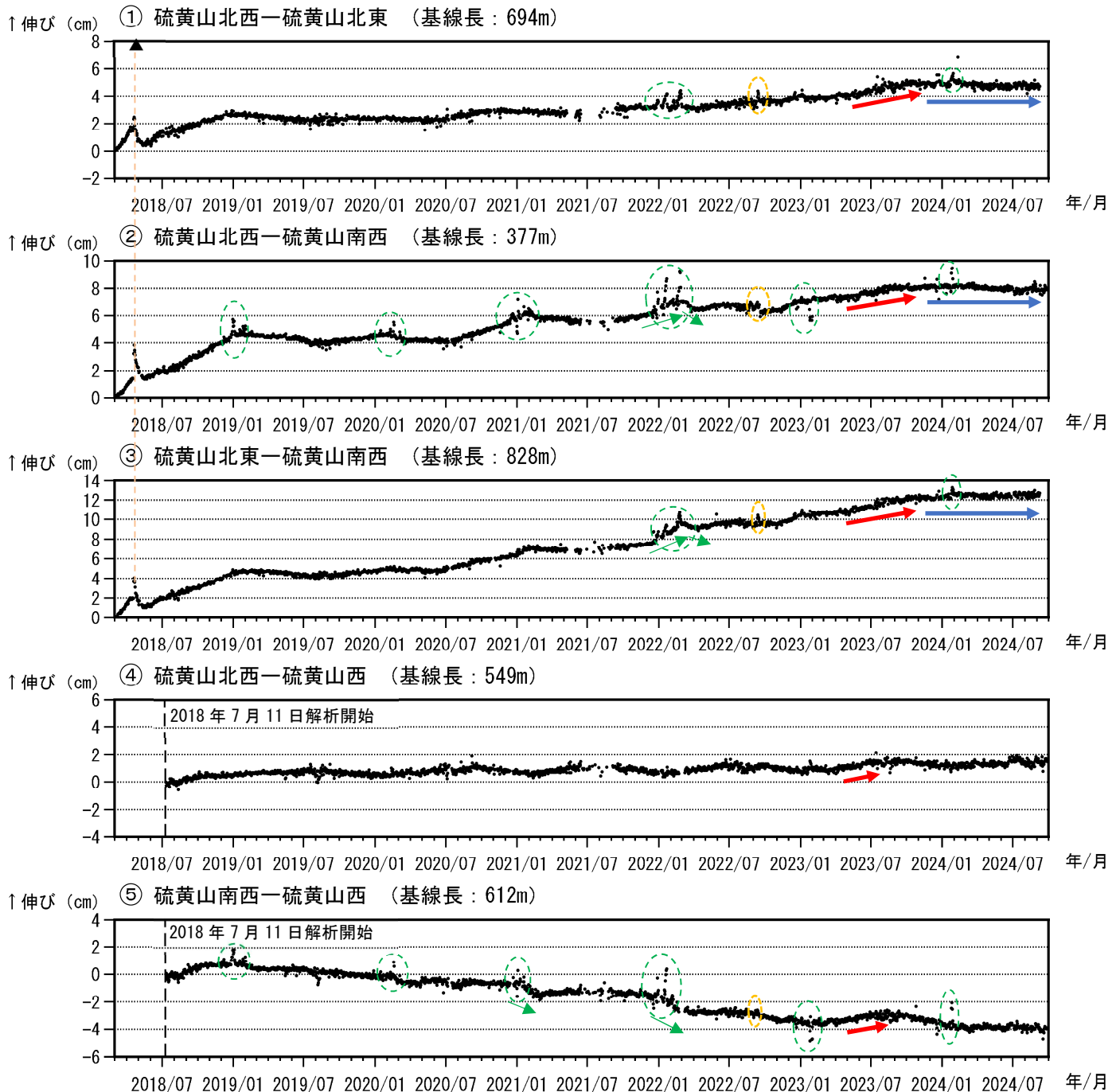
図7 霧島山（えびの高原（硫黄山）周辺） GNSS 連続観測による基線長変化 (2018年3月～2024年9月)
