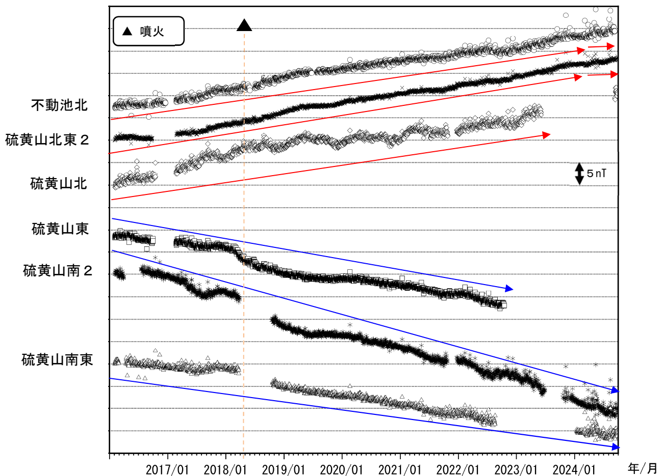
図 8-2 霧島山（えびの高原（硫黄山）周辺） 全磁力観測点で観測された全磁力変動 (2016 年 1 月～2024 年 9 月)
