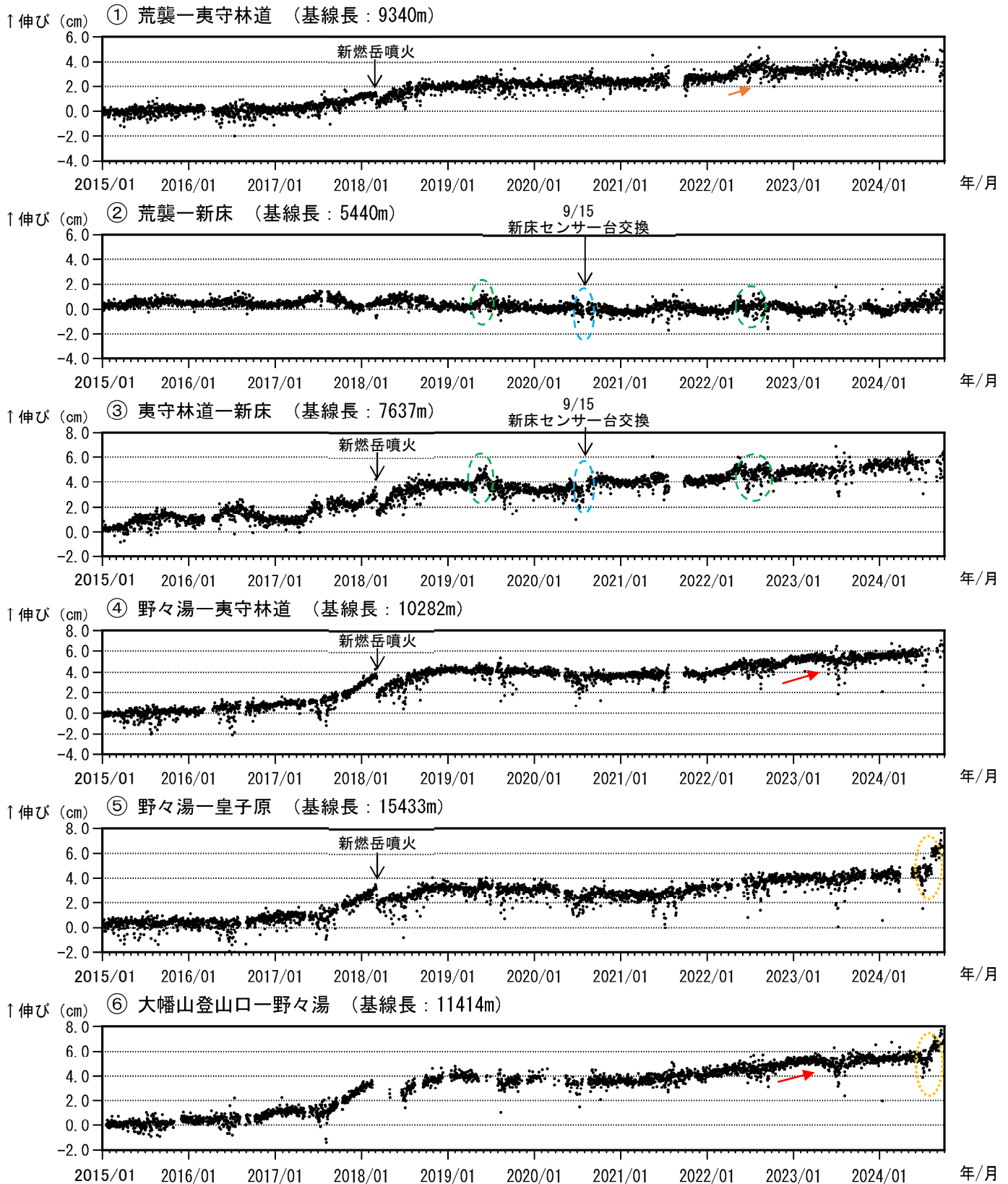
図4 霧島山（新燃岳） GNSS 連続観測による基線長変化（2015年1月～2024年9月）
