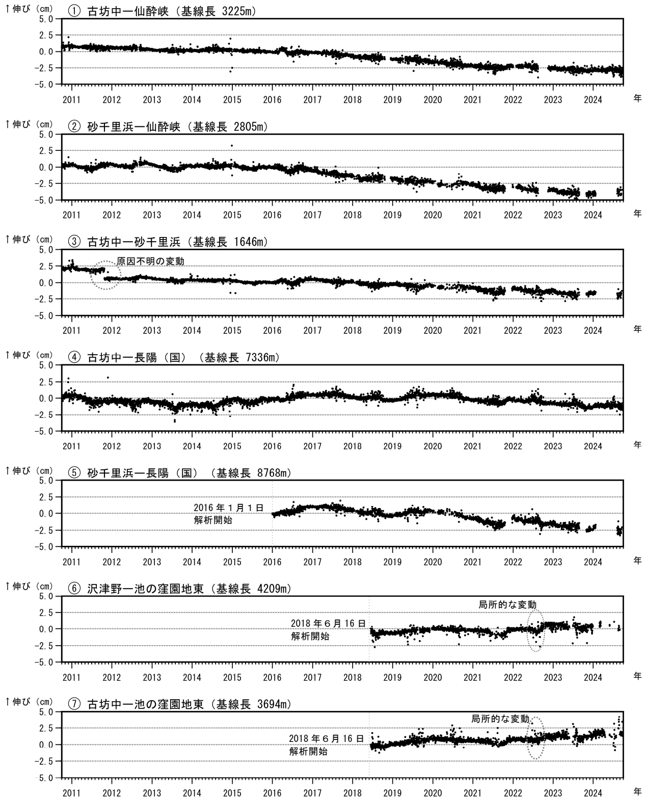
図5 阿蘇山 GNSS 連続観測による基線長変化（2010年10月～2024年9月）
