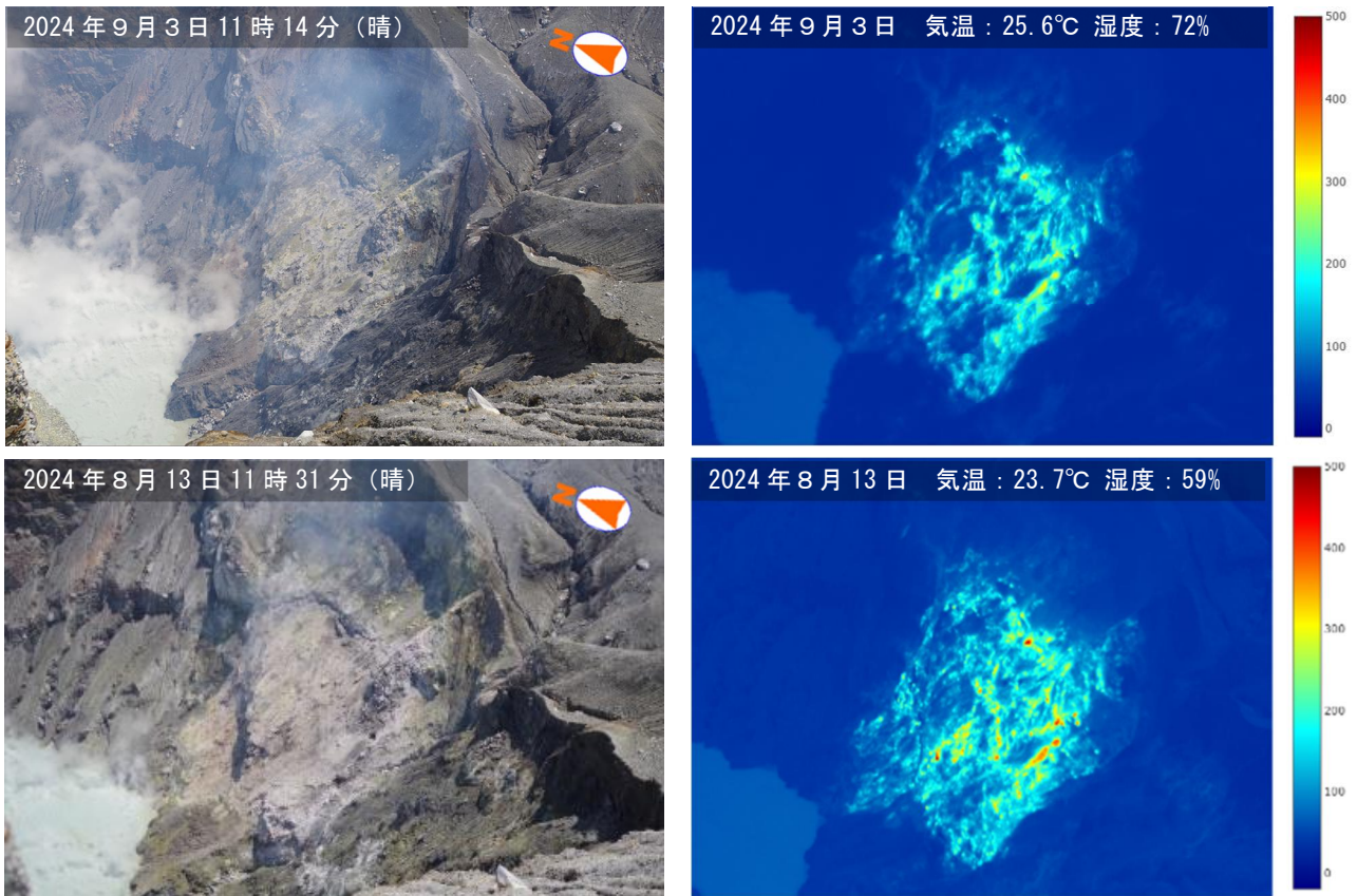
図 2-2 阿蘇山 中岳第一火口 南側火口壁の状況 （火口南西側観測定点から撮影 上図：9月3日、下図：8月13日）
