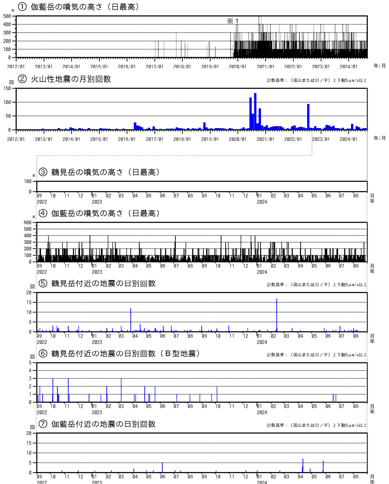
図2 鶴見岳・伽藍岳 火山活動経過図（2012年1月～2024年8月）
