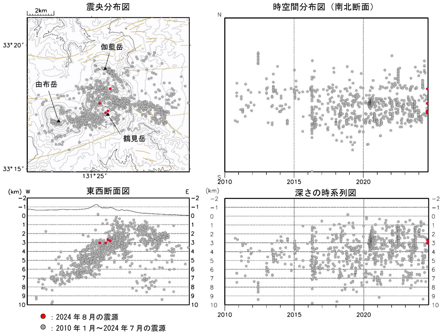
図3 鶴見岳・伽藍岳 震源分布図（2010年1月～2024年8月）
