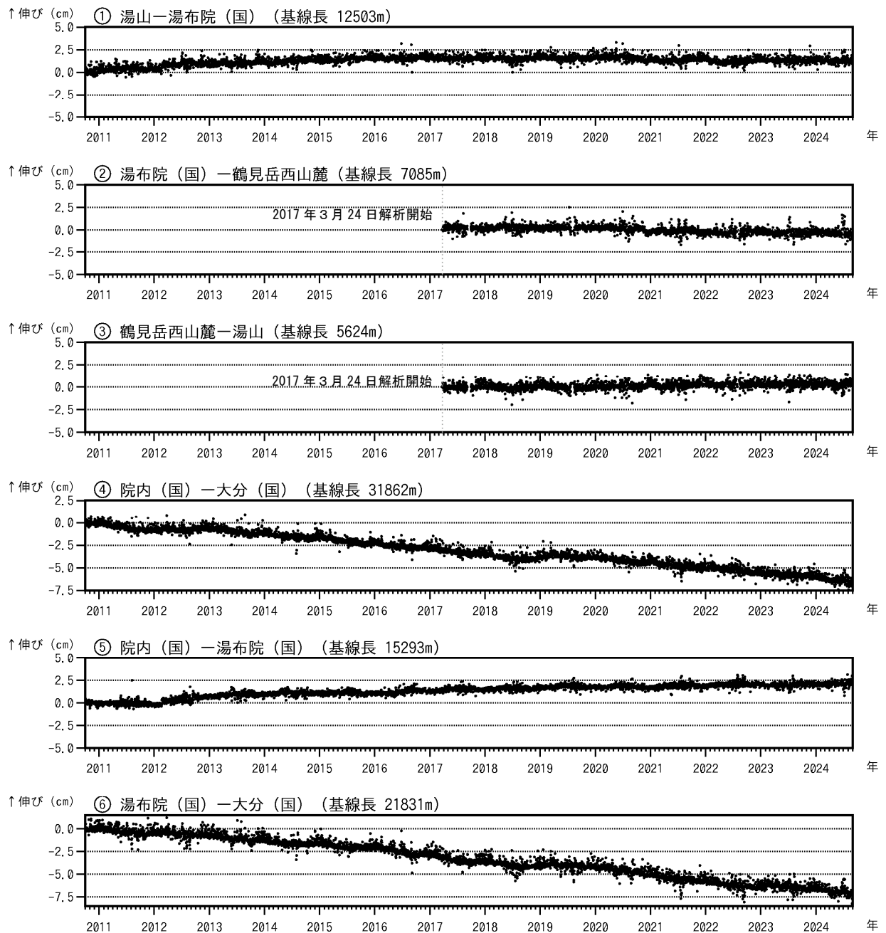
図4 鶴見岳・伽藍岳 GNSS連続観測による基線長変化（2010年10月～2024年8月）
