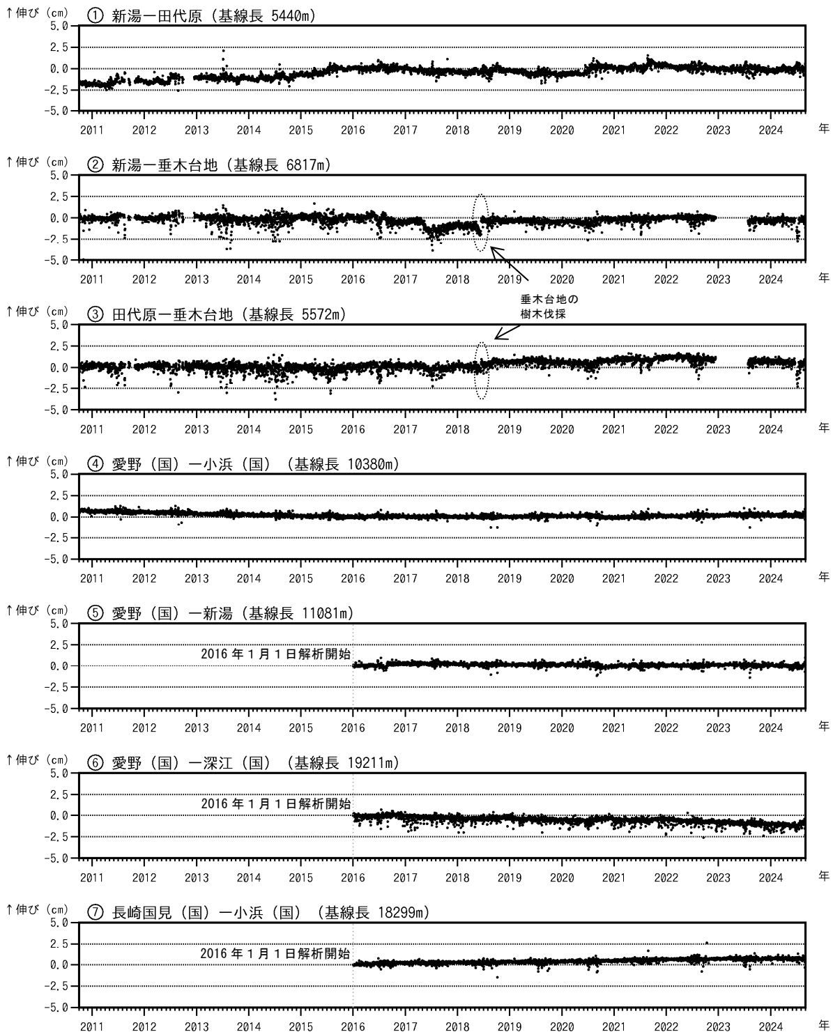
図4 雲仙岳 GNSS連続観測による基線長変化（2010年10月～2024年8月）
