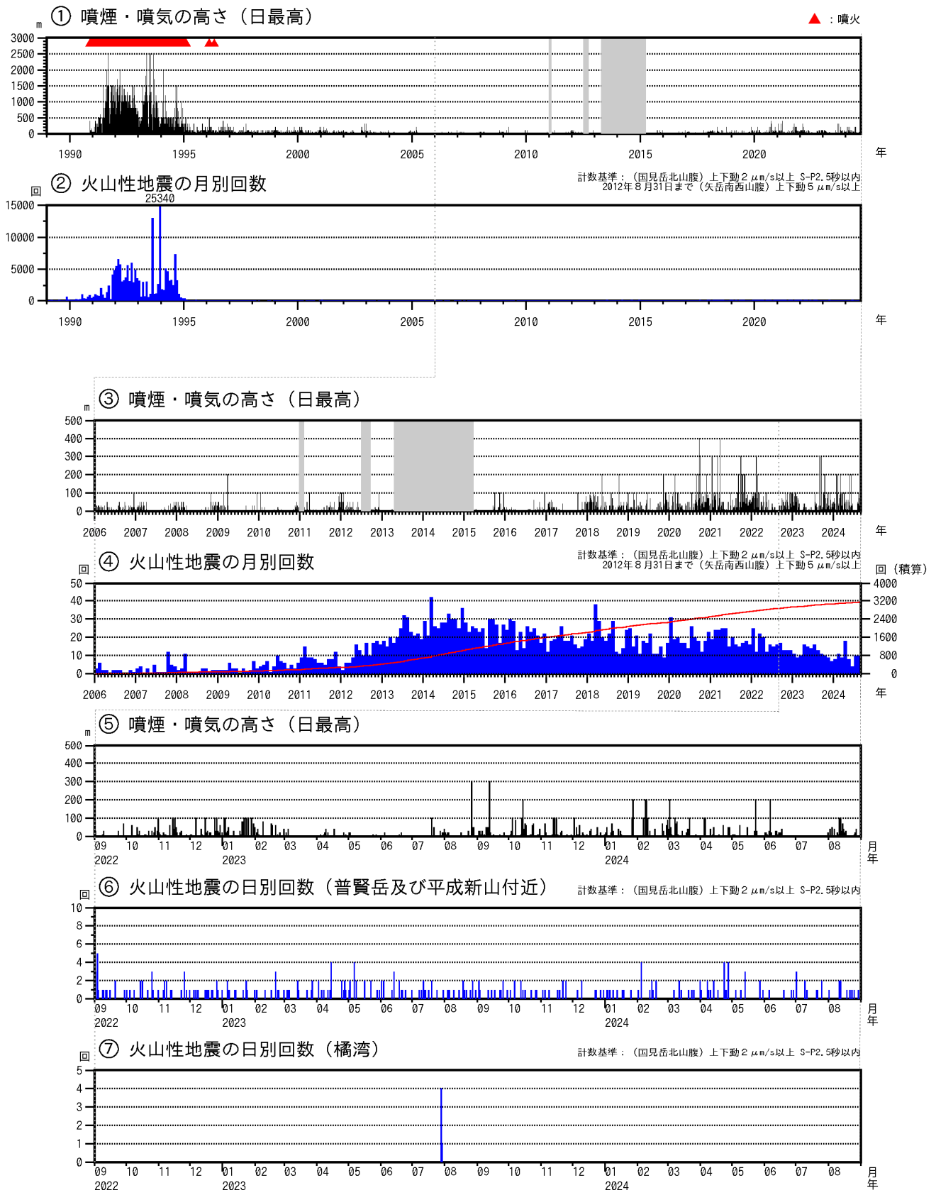
図2 雲仙岳 火山活動経過図（1989年1月～2024年8月）
