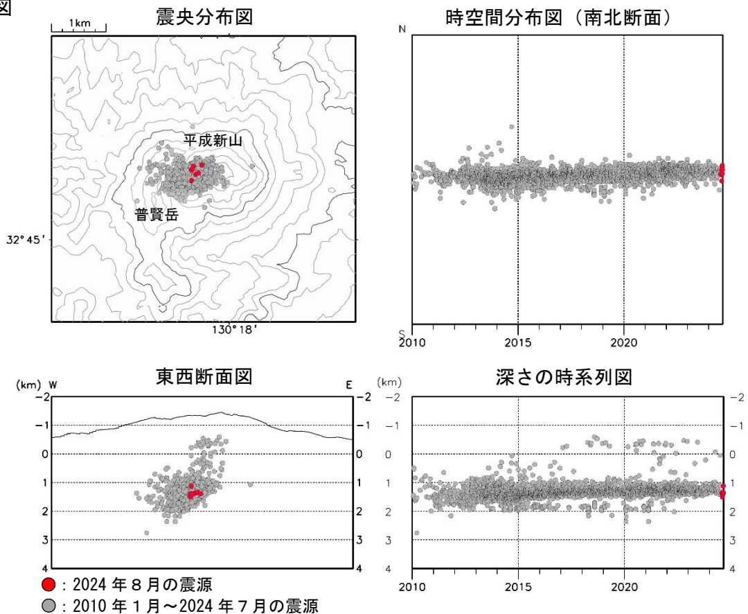
図3 雲仙岳 震源分布図 ①広域図 ②狭域図（2010年1月～2024年8月）
