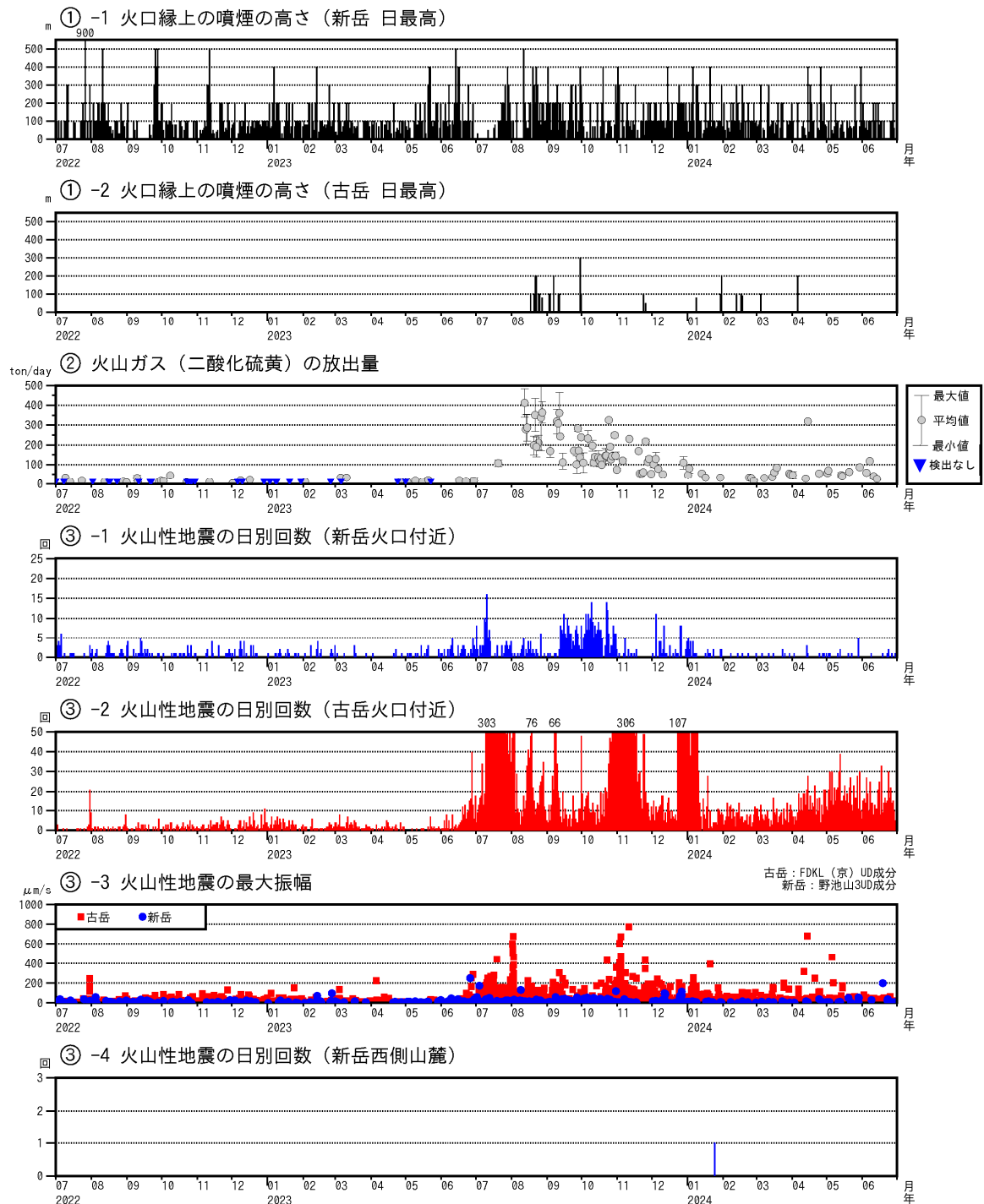
図5 口永良部島 最近の火山活動経過図（2022年7月～2024年6月）
