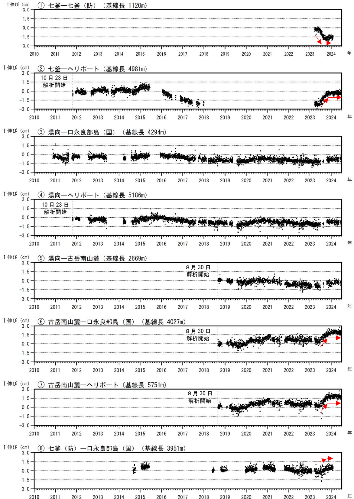
図 7-2 口永良部島 GNSS 連続観測による基線長変化 (2010 年 10 月～2024 年 6 月)
