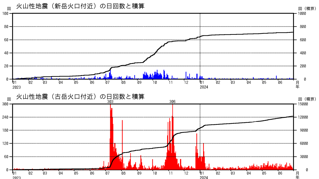
図1 口永良部島 新岳及び古岳火口付近の火山性地震の日別回数及び積算回数
