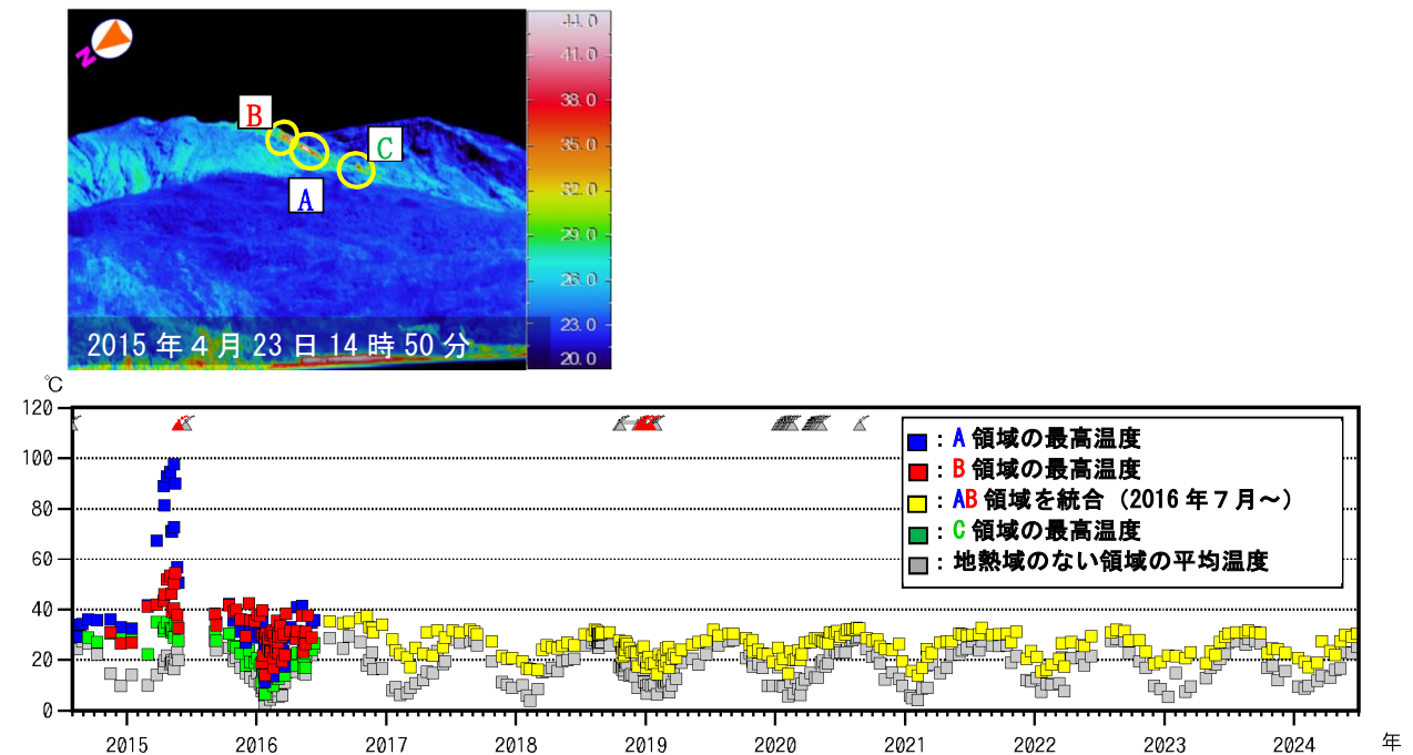
図 3-5 口永良部島 新岳火口西側割れ目付近及び新岳南西側斜面の地熱域の温度時系列
