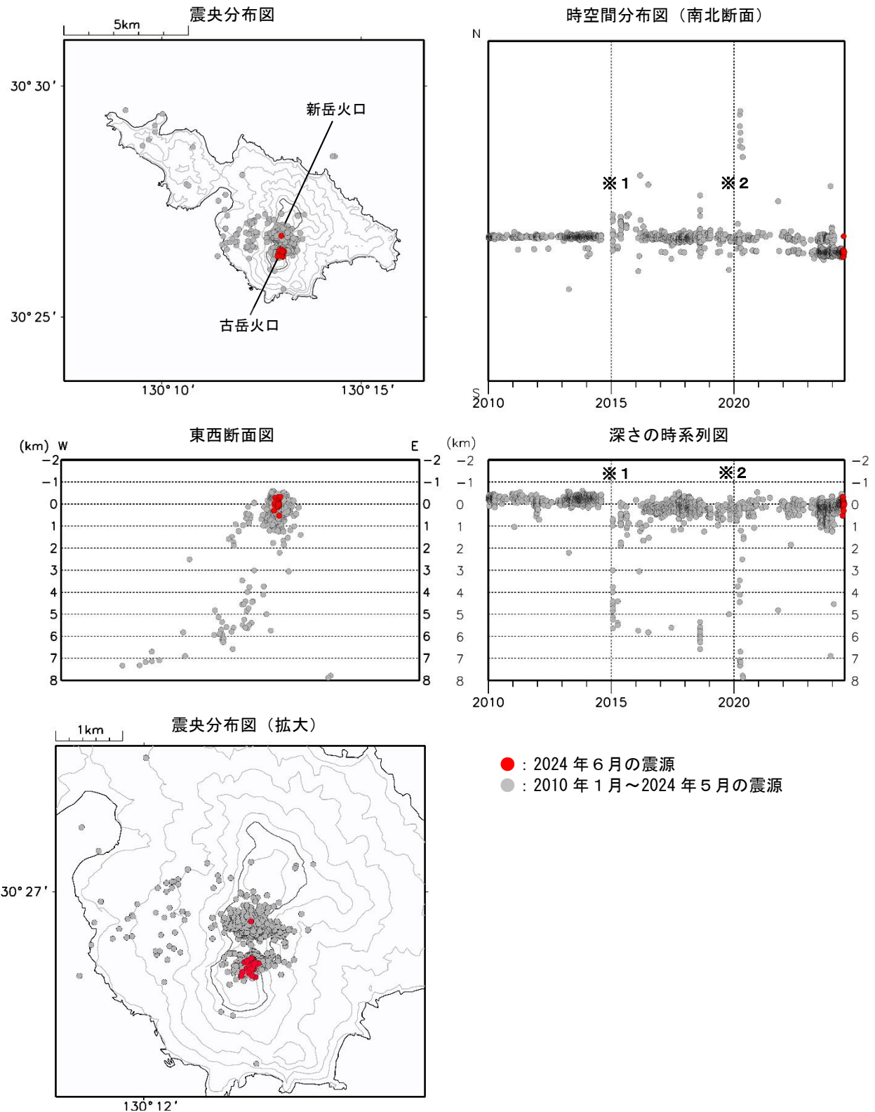
図6 口永良部島 震源分布図（2010年1月～2024年6月）
