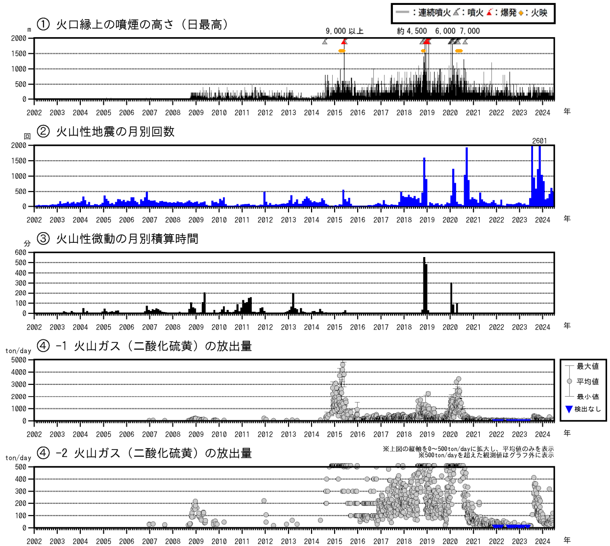
図4 口永良部島 火山活動経過図（2002年1月～2024年6月）
