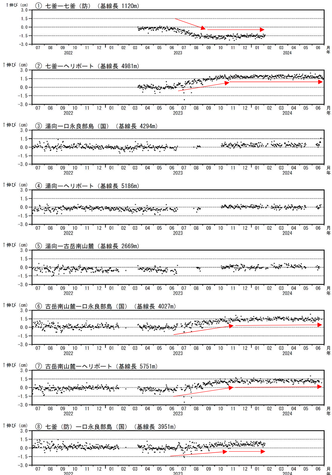
図 7-1 口永良部島 GNSS 連続観測による基線長変化（2022 年 7 月～2024 年 6 月）
