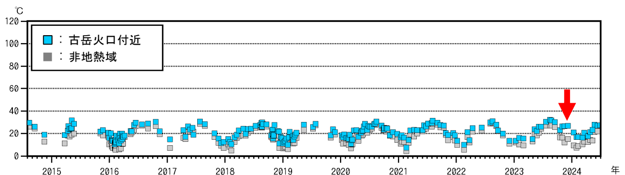
図 3-3 古岳火口付近の地熱域の温度時系列（2014年8月～2024年6月、湯向から観測）
