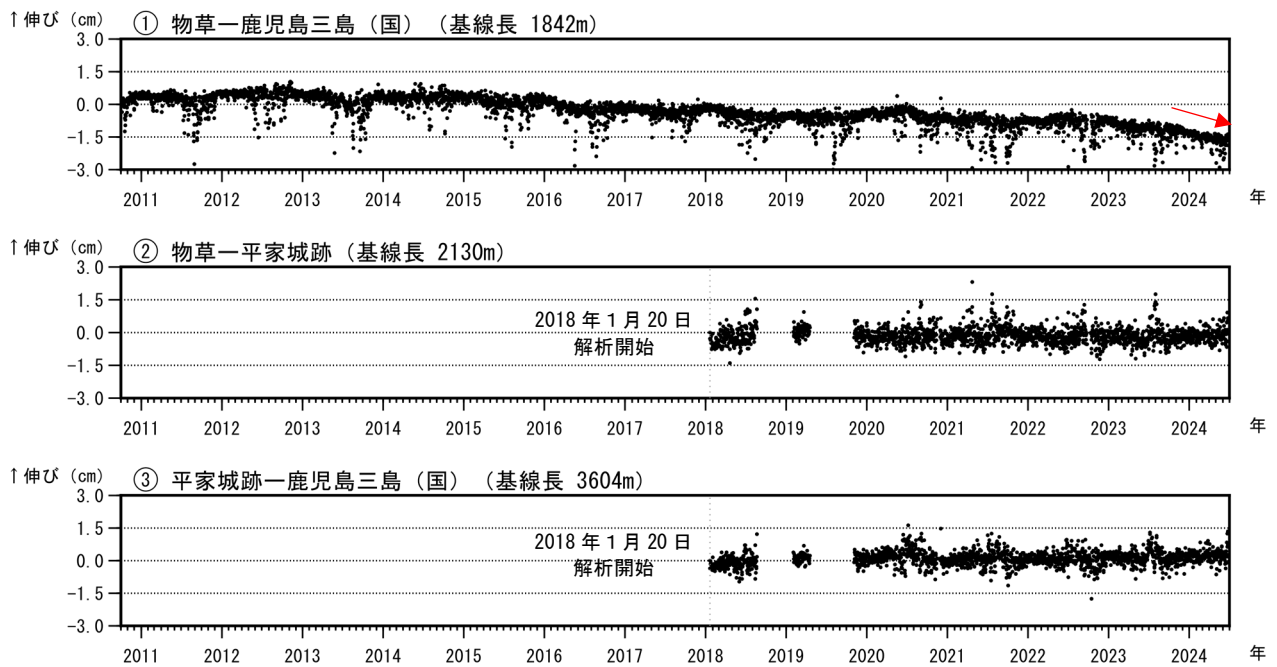
図5 薩摩硫黄島 GNSS連続観測による基線長変化（2010年10月～2024年6月）
