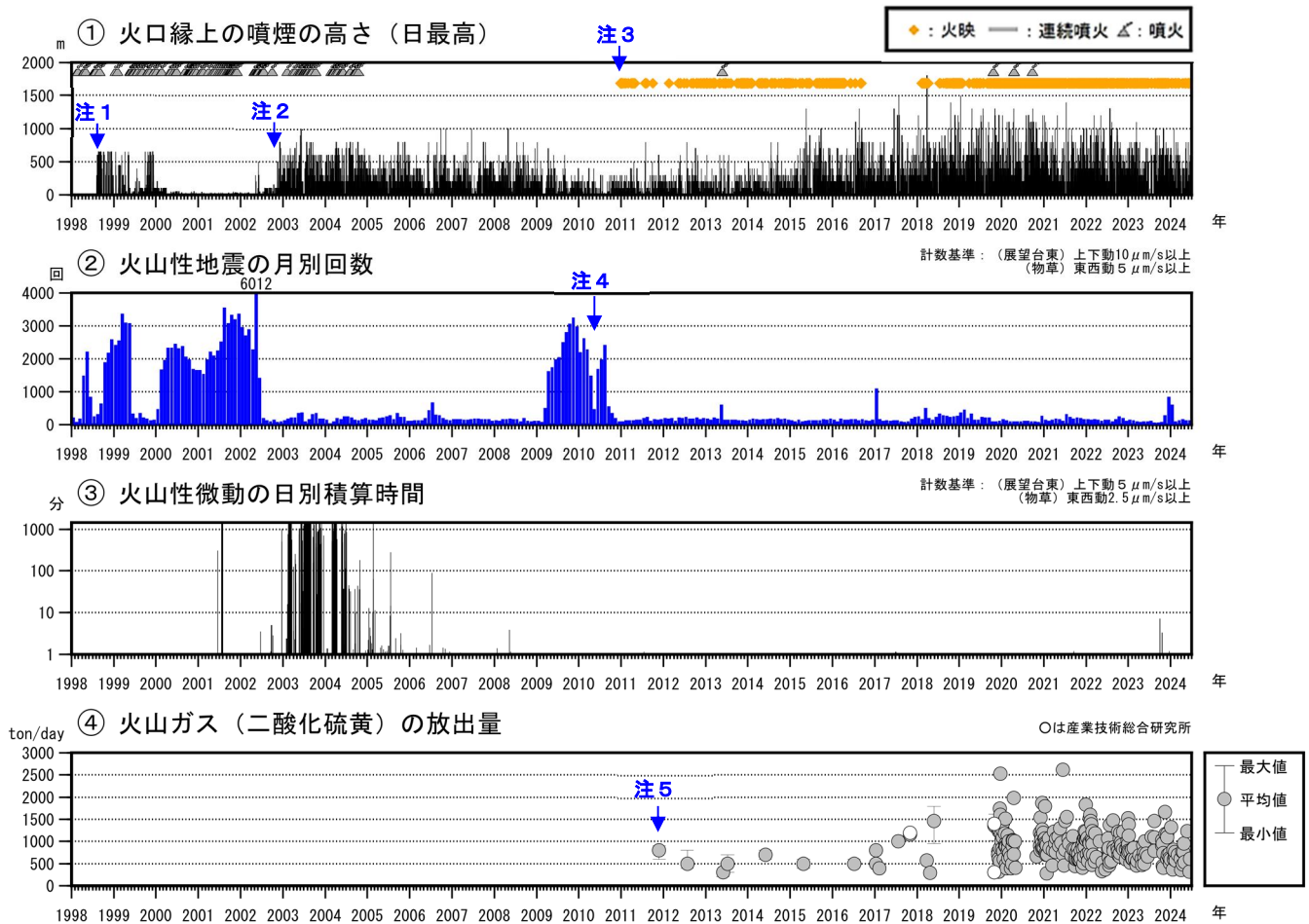
図3 薩摩硫黄島 火山活動経過図（1998年1月～2024年6月）
