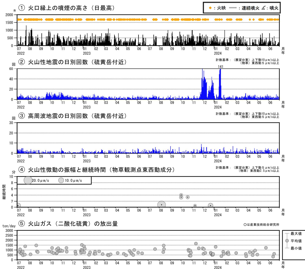
図4 薩摩硫黄島 火山活動経過図（2022年7月～2024年6月）
