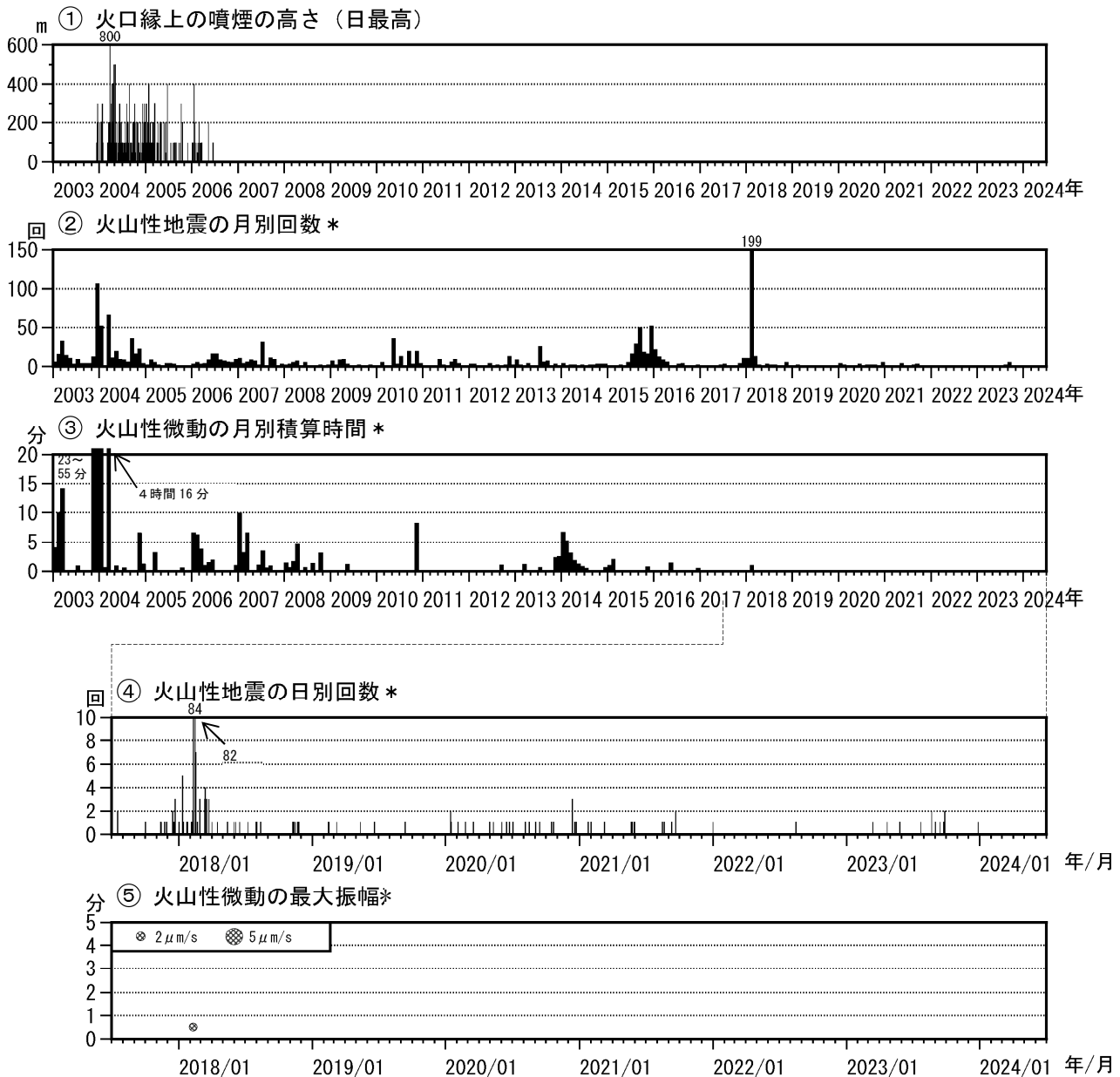
図3 霧島山（御鉢） 火山活動経過図（2003年1月～2024年6月）
