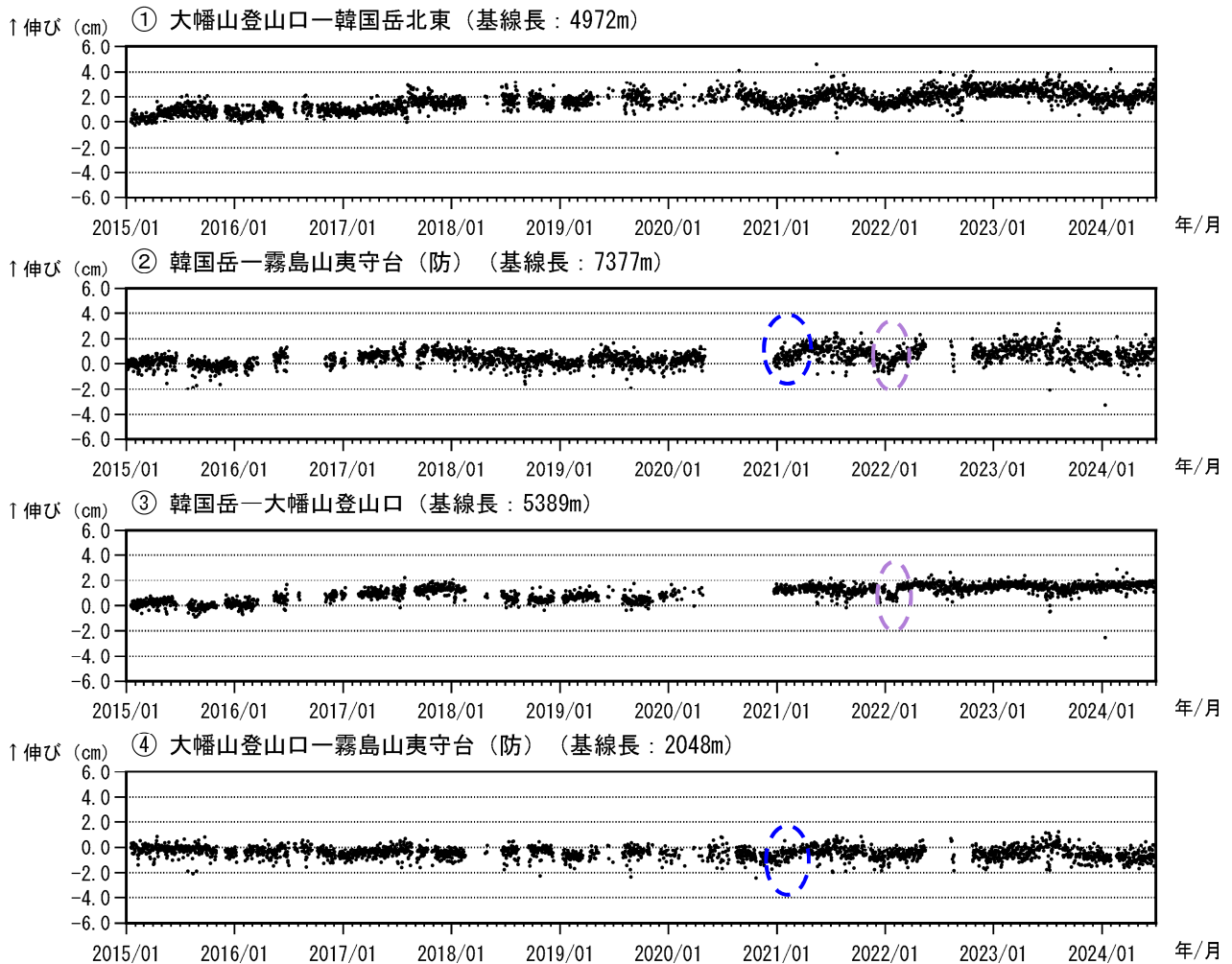
図4 霧島山（大幡池） GNSS 連続観測による基線長変化（2015年1月～2024年6月）
