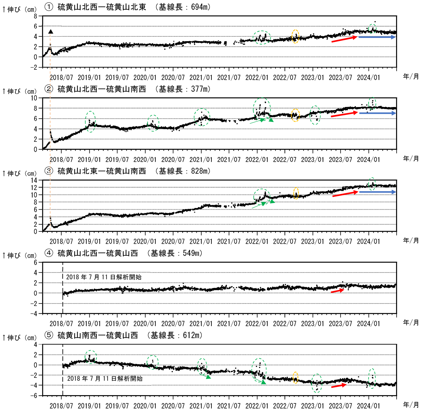
図5 霧島山（えびの高原（硫黄山）周辺） GNSS 連続観測による基線長変化 （2018年3月～2024年6月）
