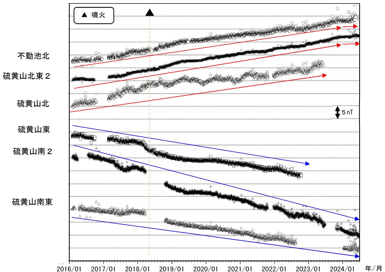
図 6-2 霧島山（えびの高原（硫黄山）周辺） 全磁力観測点で観測された全磁力変動
