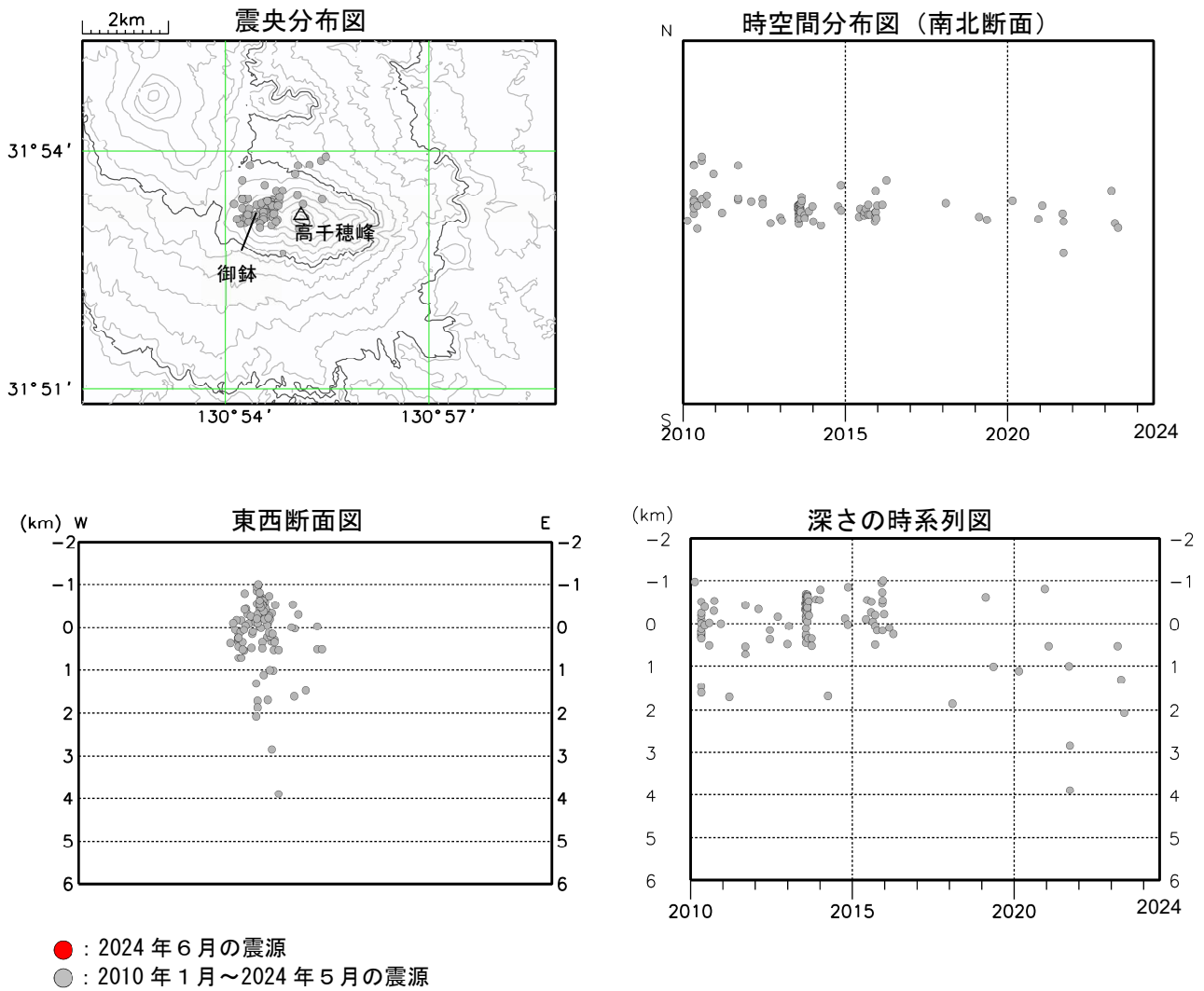
図2 霧島山（御鉢） 震源分布図（2010 年 1 月～2024 年 6 月）
