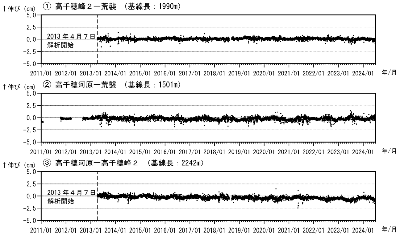
図4 霧島山（御鉢） GNSS 連続観測による基線長変化（2011年1月～2024年6月）
