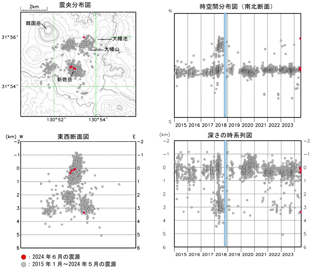
図3 霧島山（新燃岳） 震源分布図（2015 年 1 月～2024 年 6 月）
