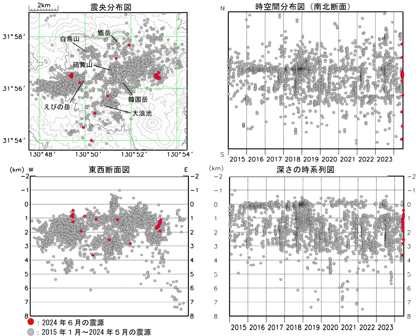
図3 霧島山（えびの高原（硫黄山）周辺） 震源分布図（2015 年 1 月～2024 年 6 月）
