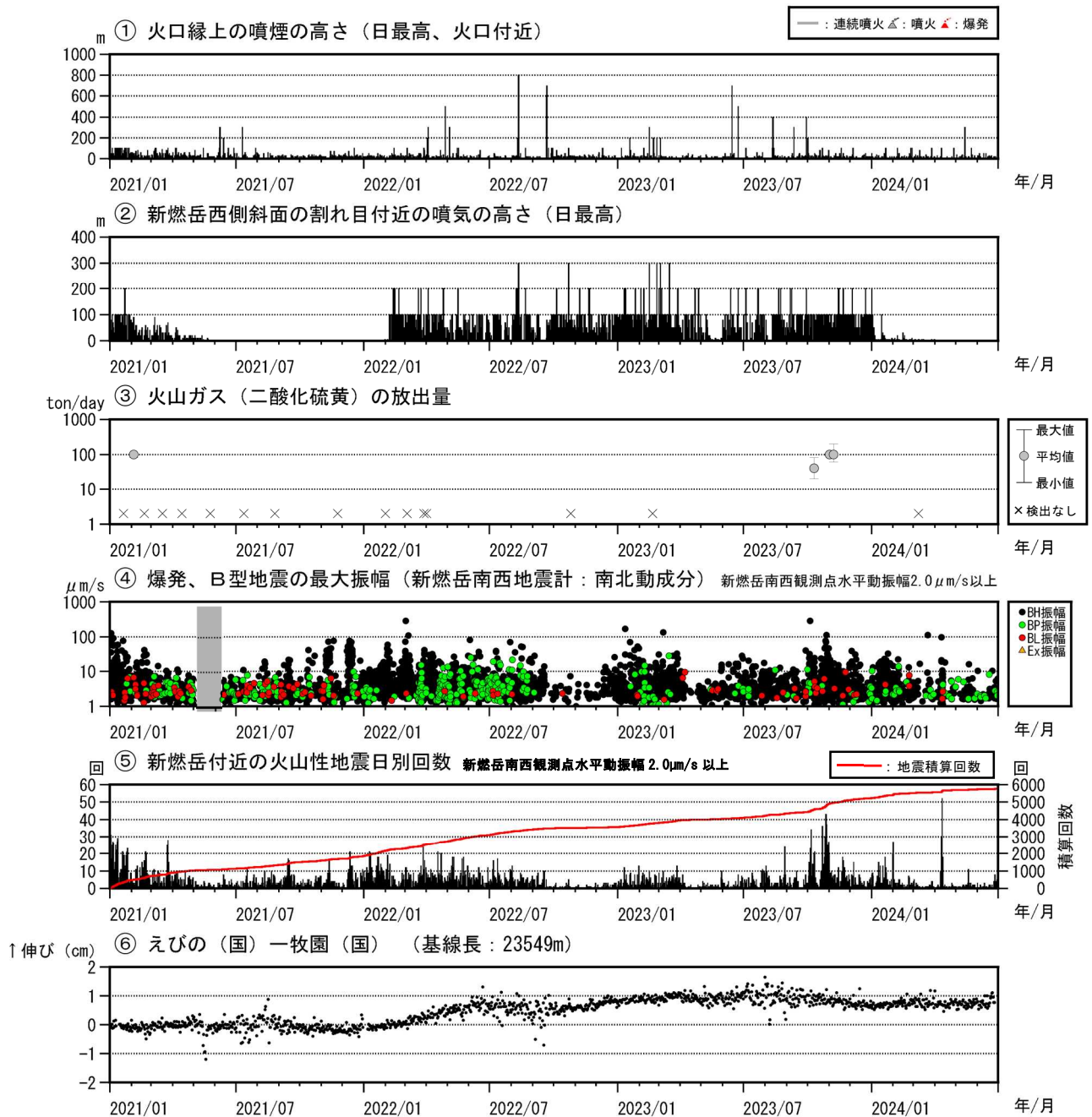
図2 霧島山（新燃岳） 火山活動経過図（2021年1月～2024年6月）
