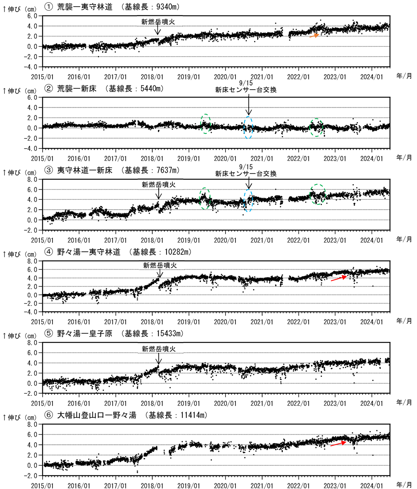
図4 霧島山（新燃岳） GNSS 連続観測による基線長変化（2015年1月～2024年6月）
