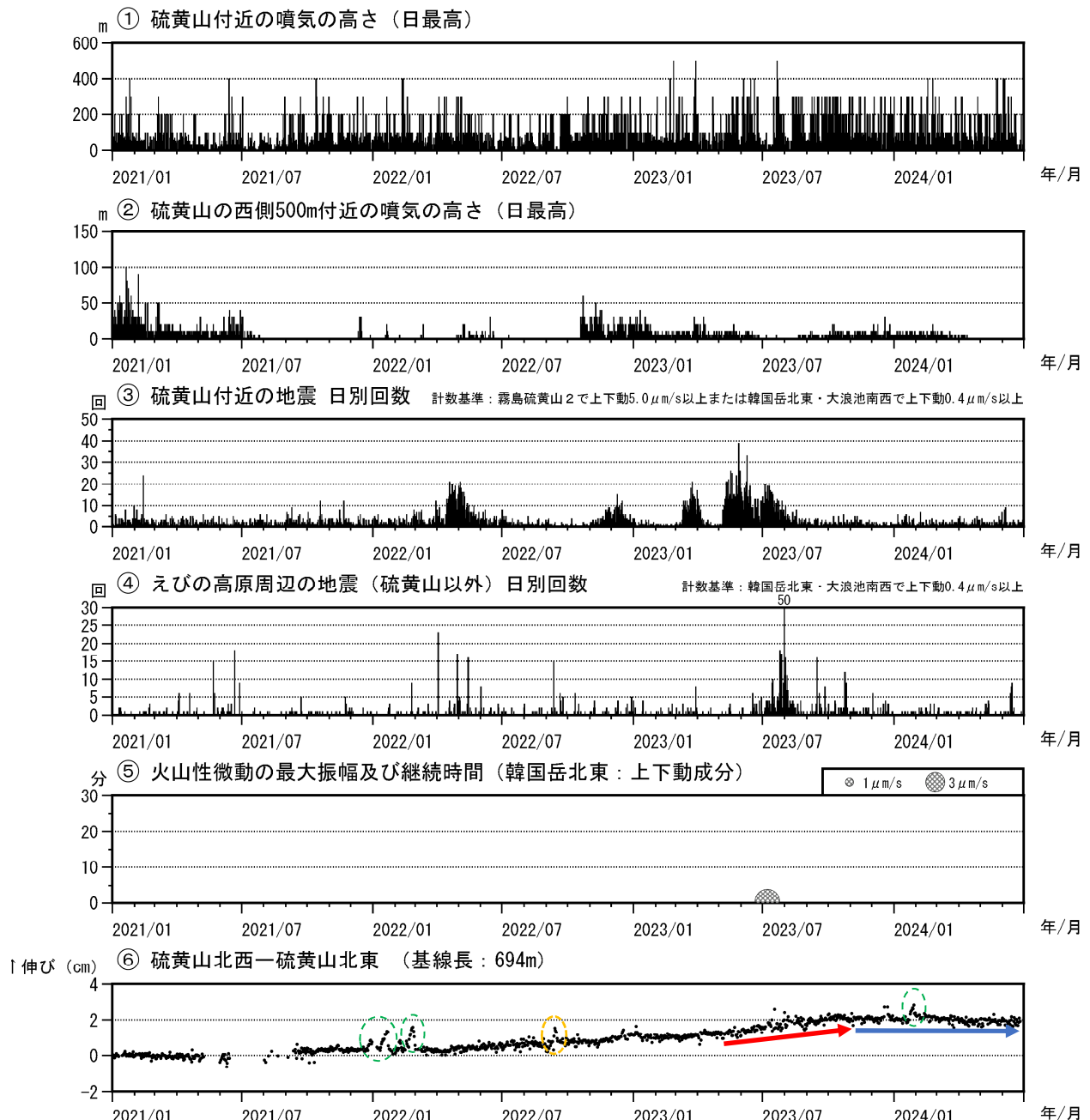
図2 霧島山（えびの高原（硫黄山）周辺） 火山活動経過図（2021年1月～2024年6月）
