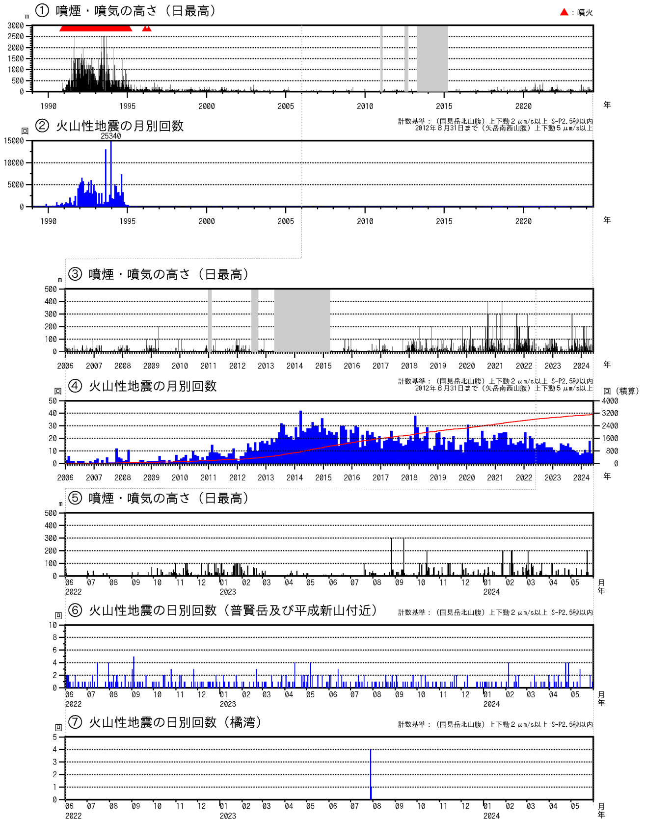
図4 雲仙岳 火山活動経過図（1989年1月～2024年5月）
