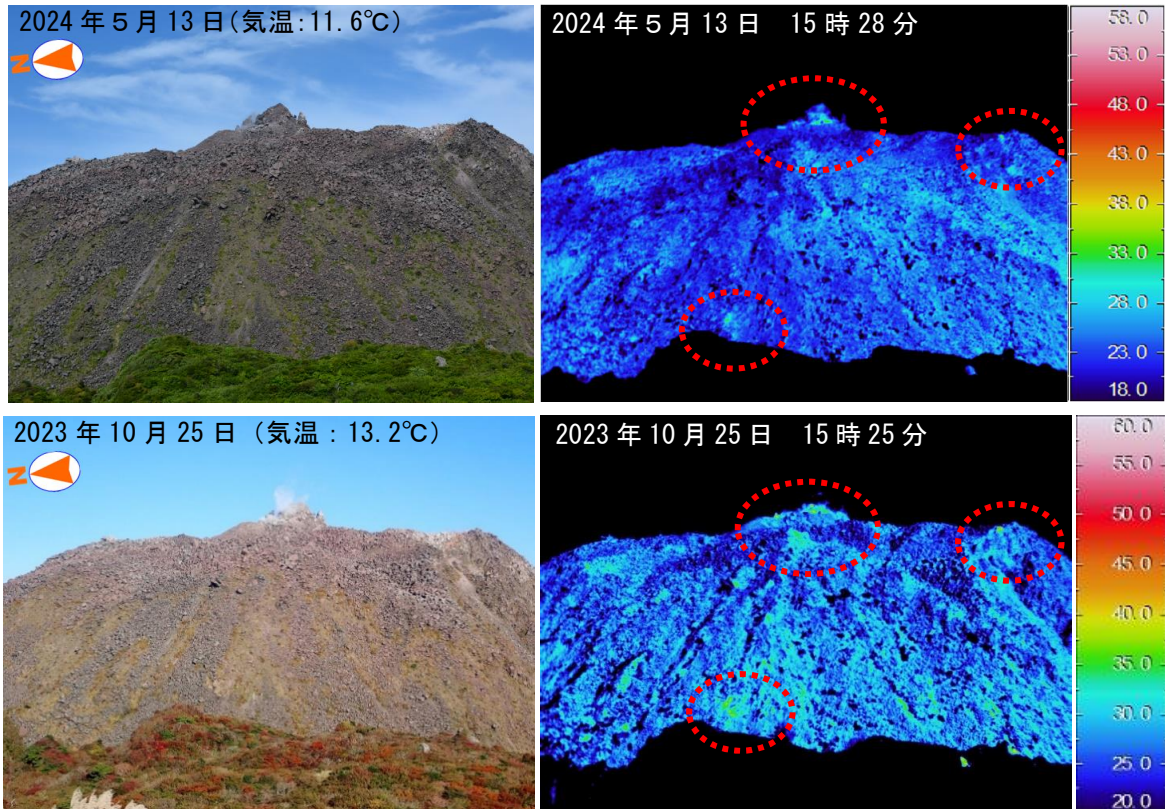
図 3-2 赤外熱映像装置による平成新山の地表面温度分布および可視画像（普賢岳山頂から観測）
