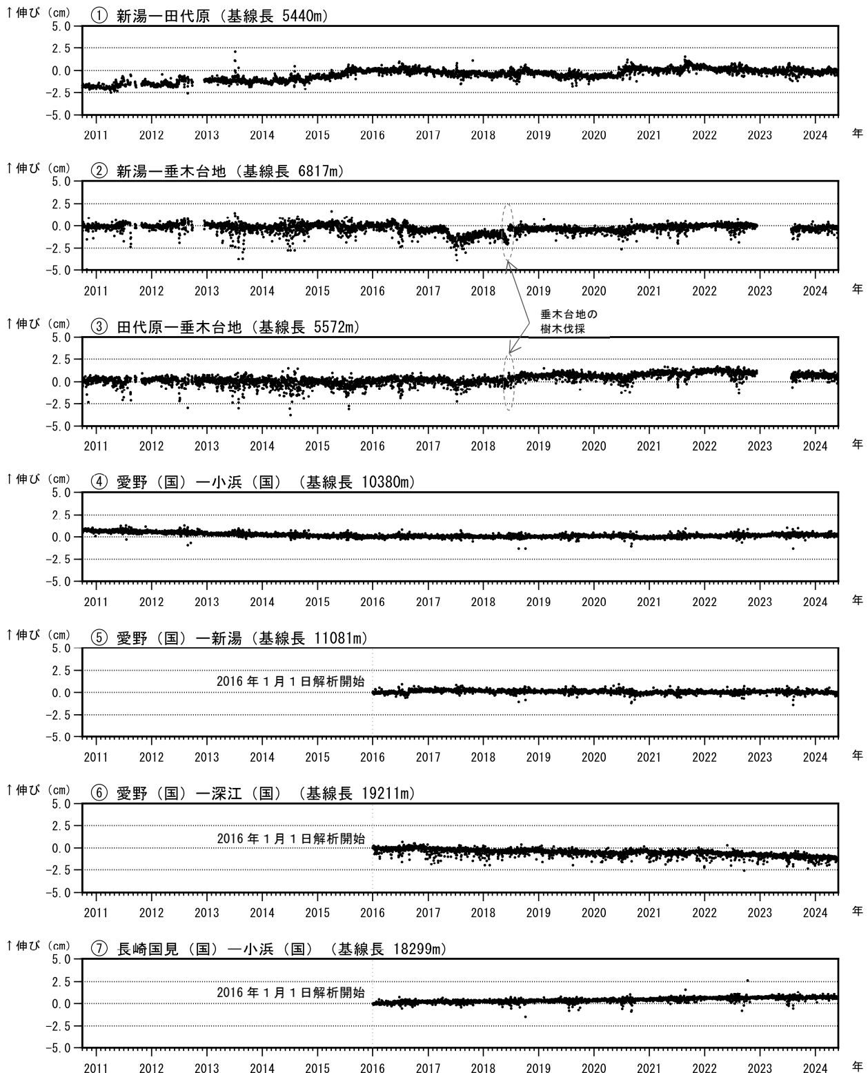
図6 雲仙岳 GNSS連続観測による基線長変化（2010年10月～2024年5月）
