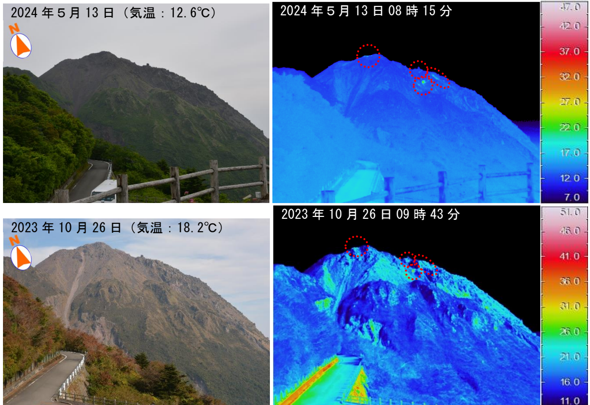
図 3-3 赤外熱映像装置による平成新山の地表面温度分布および可視画像（仁田峠第2展望台から観測）
