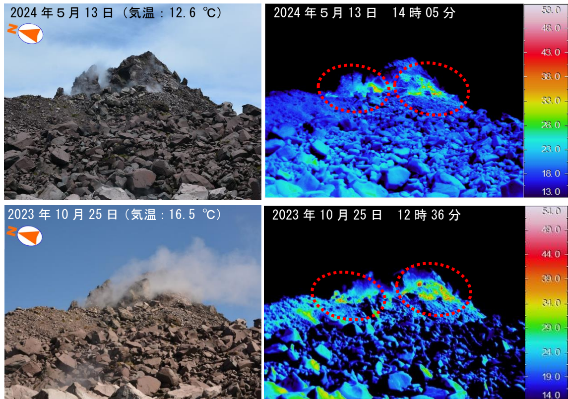
図 3-1 赤外熱映像装置による平成新山の地表面温度分布および可視画像（平成新山山腹から観測）
