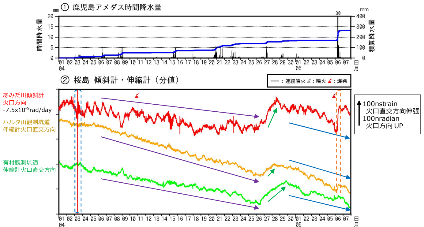
図6 桜島 傾斜計及び伸縮計による地殻変動の状況（2024年4月～5月7日（期間外））
