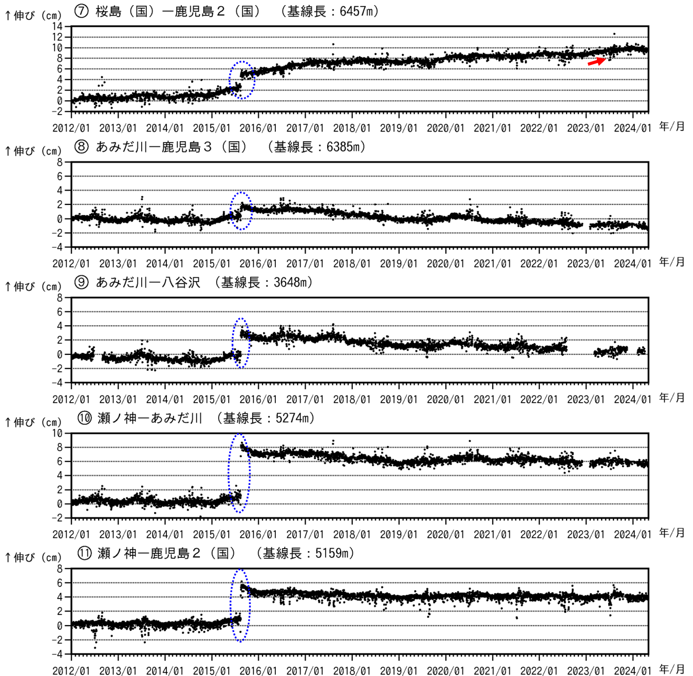
図 7-2 桜島 GNSS 連続観測による基線長変化（2012 年 1 月～2024 年 4 月）
