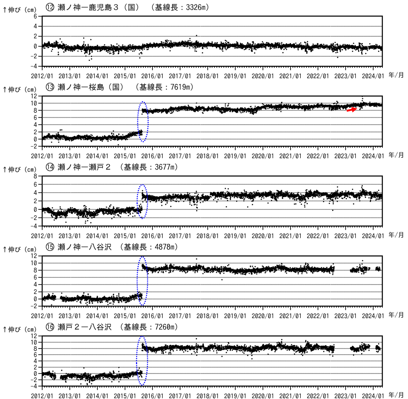
図 7-3 桜島 GNSS 連続観測による基線長変化 (2012 年 1 月～2024 年 4 月)
