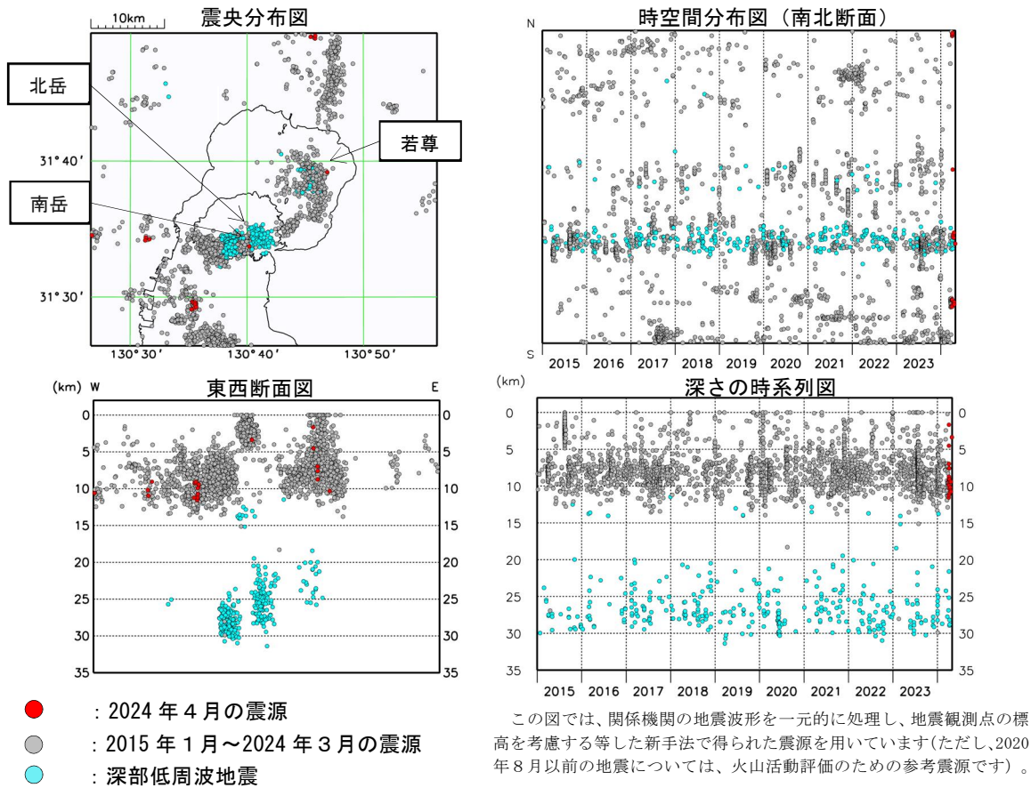
図 2-1 桜島 始良カルデラ周辺の震源分布図（2015 年 1 月～2024 年 4 月）
