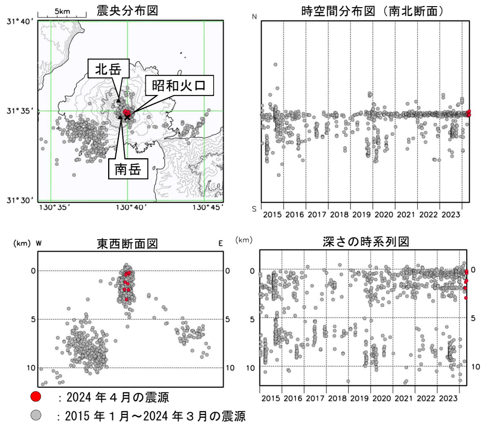
図 2-2 桜島 桜島付近の震源分布図（2015 年 1 月～2024 年 4 月）
