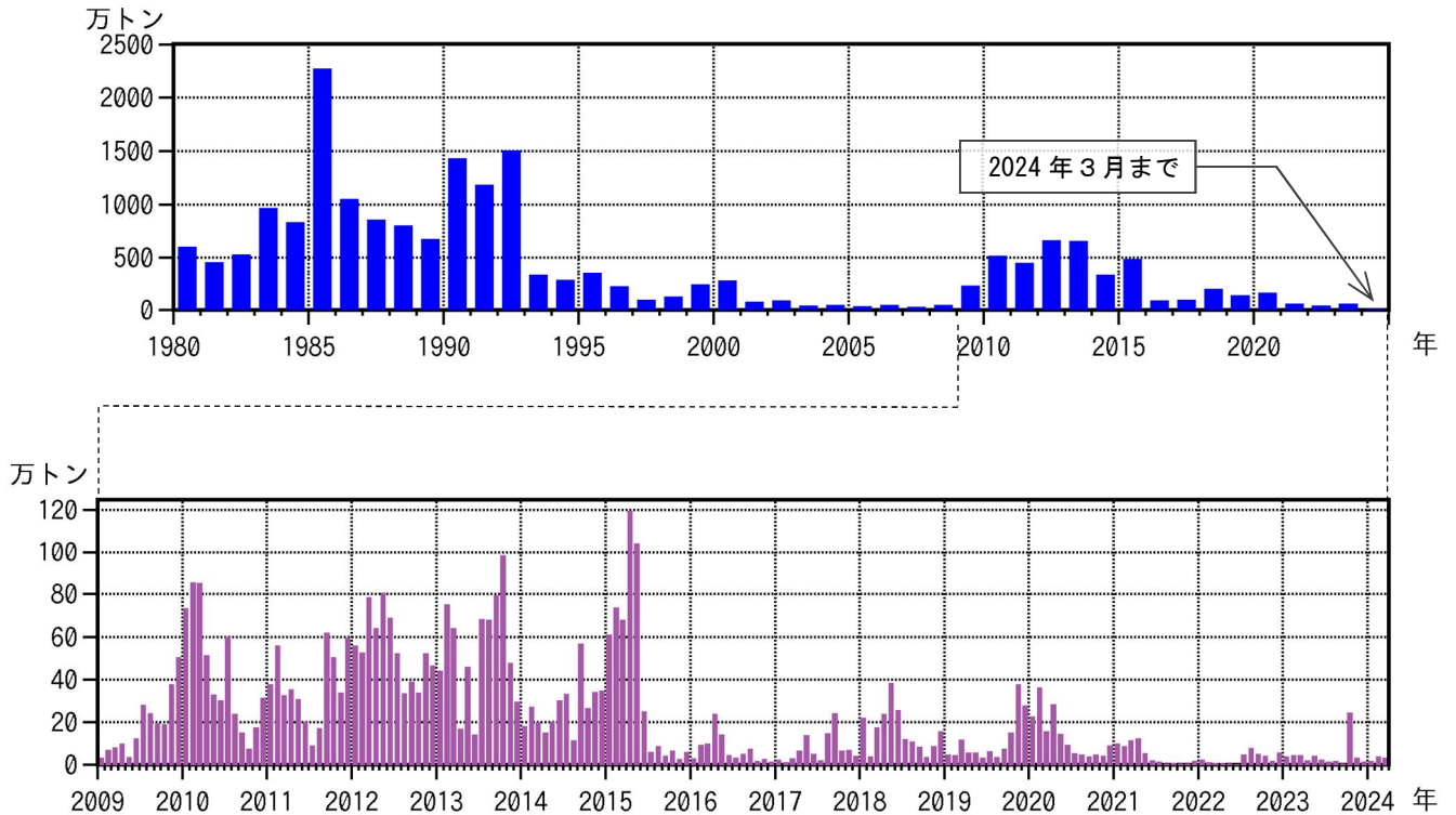
図4 桜島 鹿児島県が実施している降灰の観測データから推定した火山灰の総噴出量 （上段：1980年1月～2024年3月の年別値、下段：2009年1月～2024年3月の月別値）
