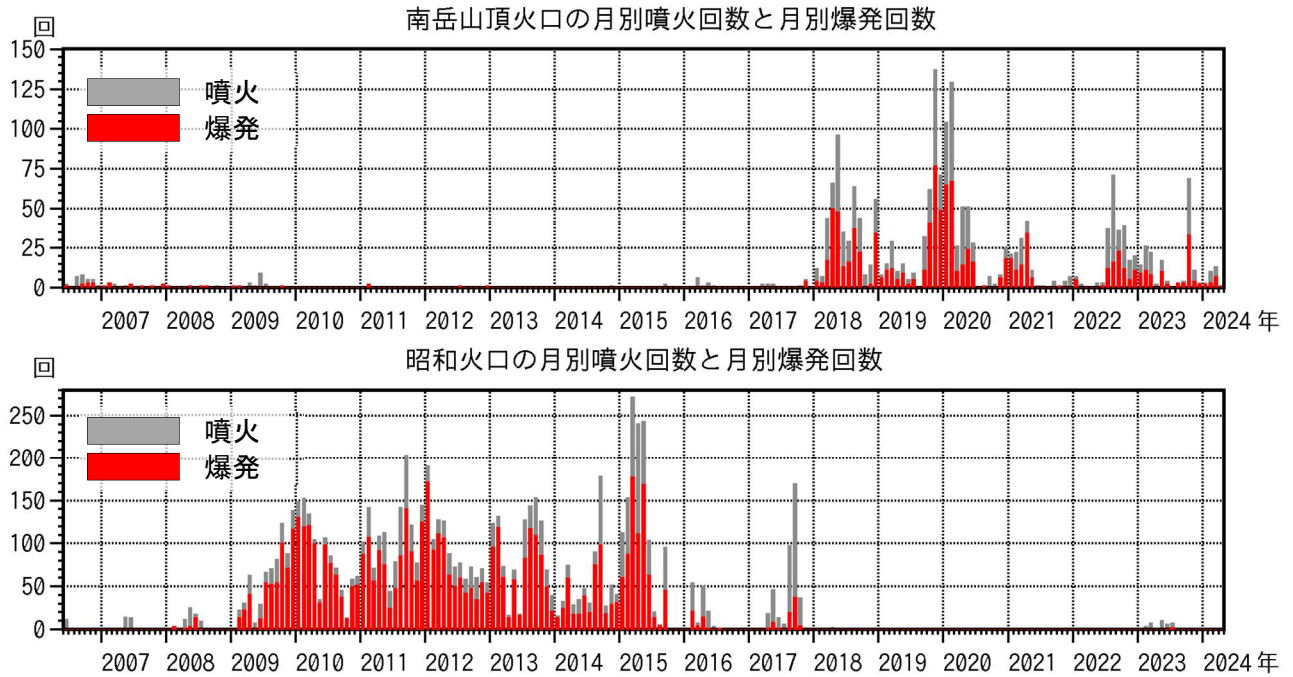
図3 桜島 南岳山頂火口（上図）と昭和火口（下図）の月別噴火回数と月別爆発回数 （2006年6月～2024年4月）
