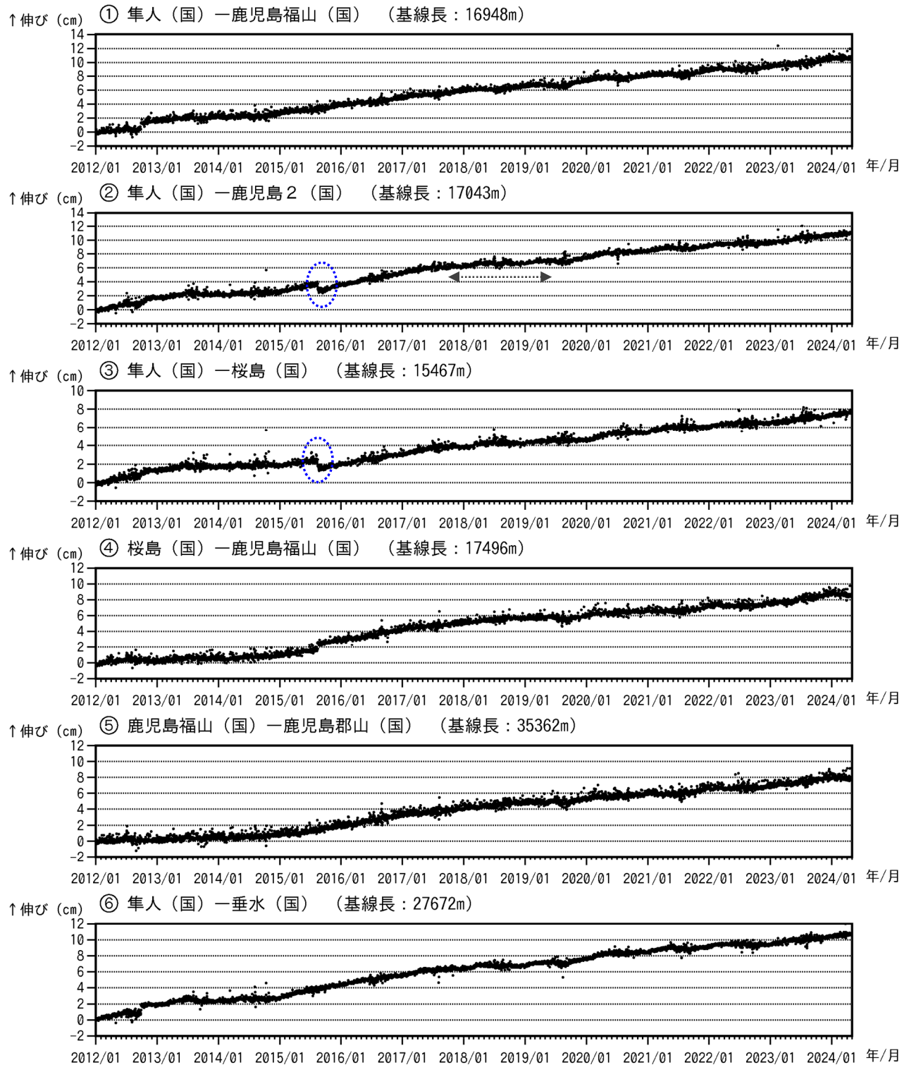
図 7-1 桜島 GNSS 連続観測による基線長変化 (2012 年 1 月～2024 年 4 月)
