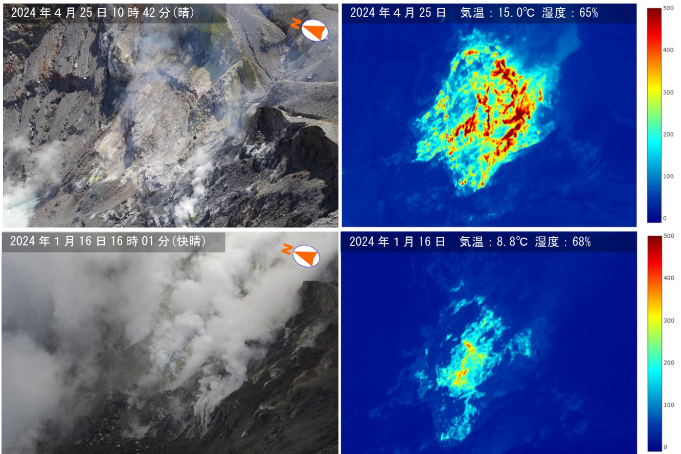
図 2-2 阿蘇山 中岳第一火口 南側火口壁の状況 (火口南西側観測定点から撮影 上図：4月25日、下図：1月16日)
