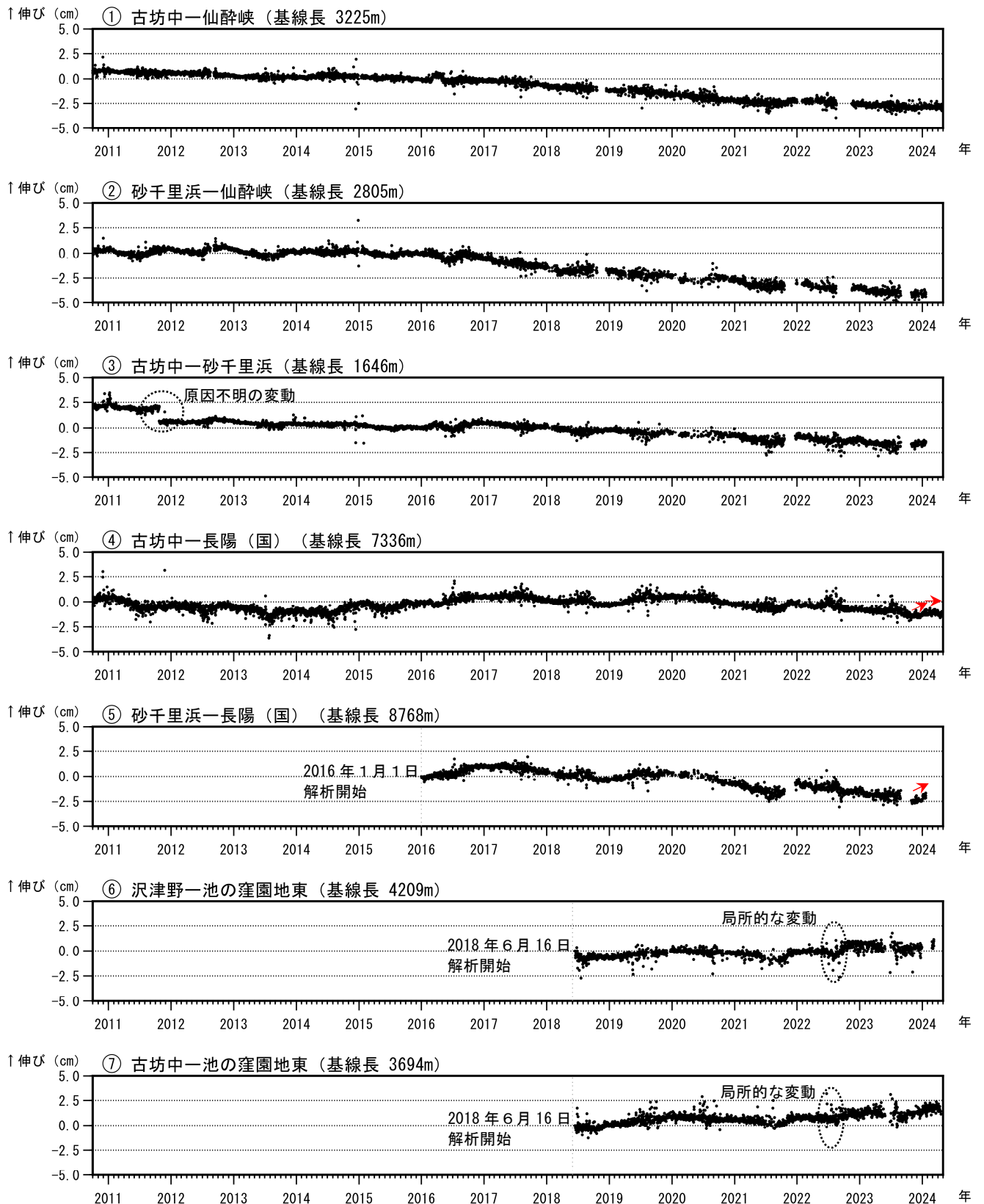
図5 阿蘇山 GNSS 連続観測による基線長変化（2010年10月～2024年4月）
