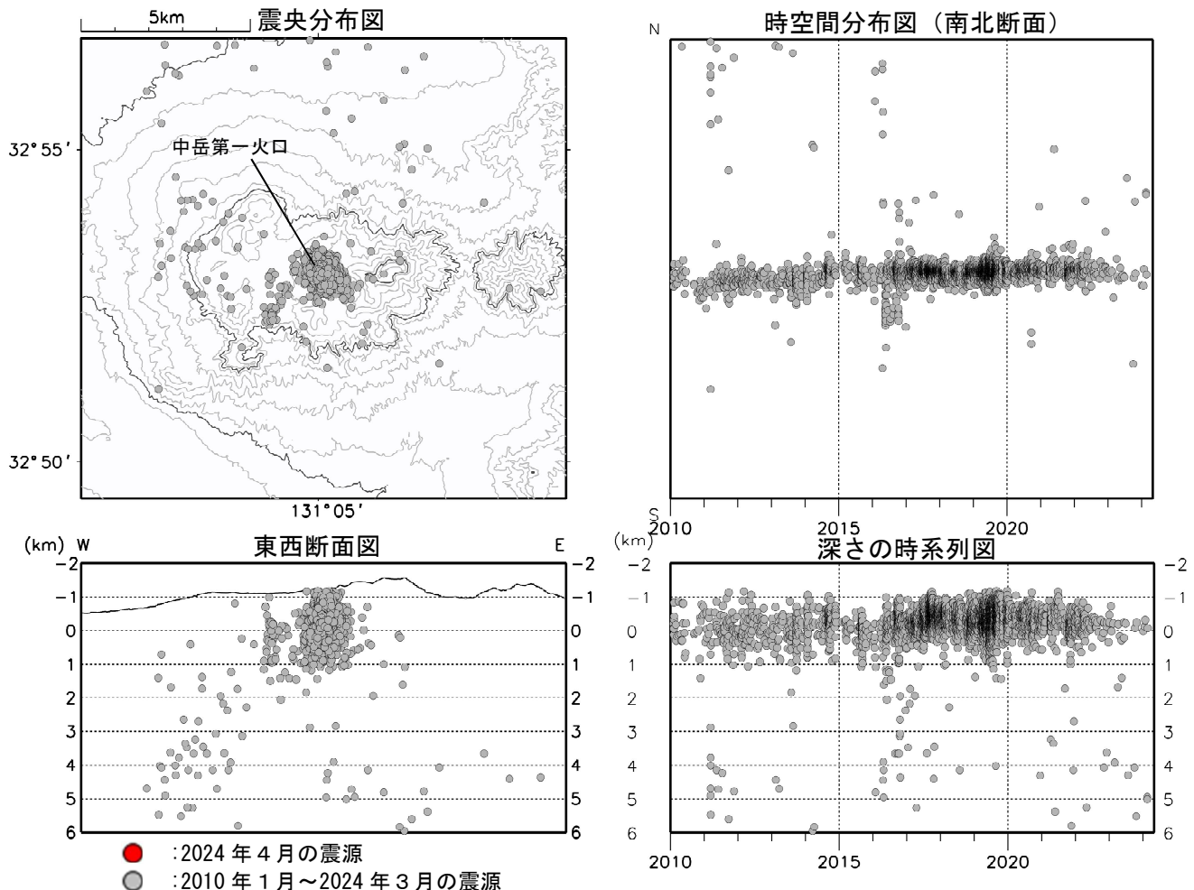
図4 阿蘇山 火山性地震の震源分布
