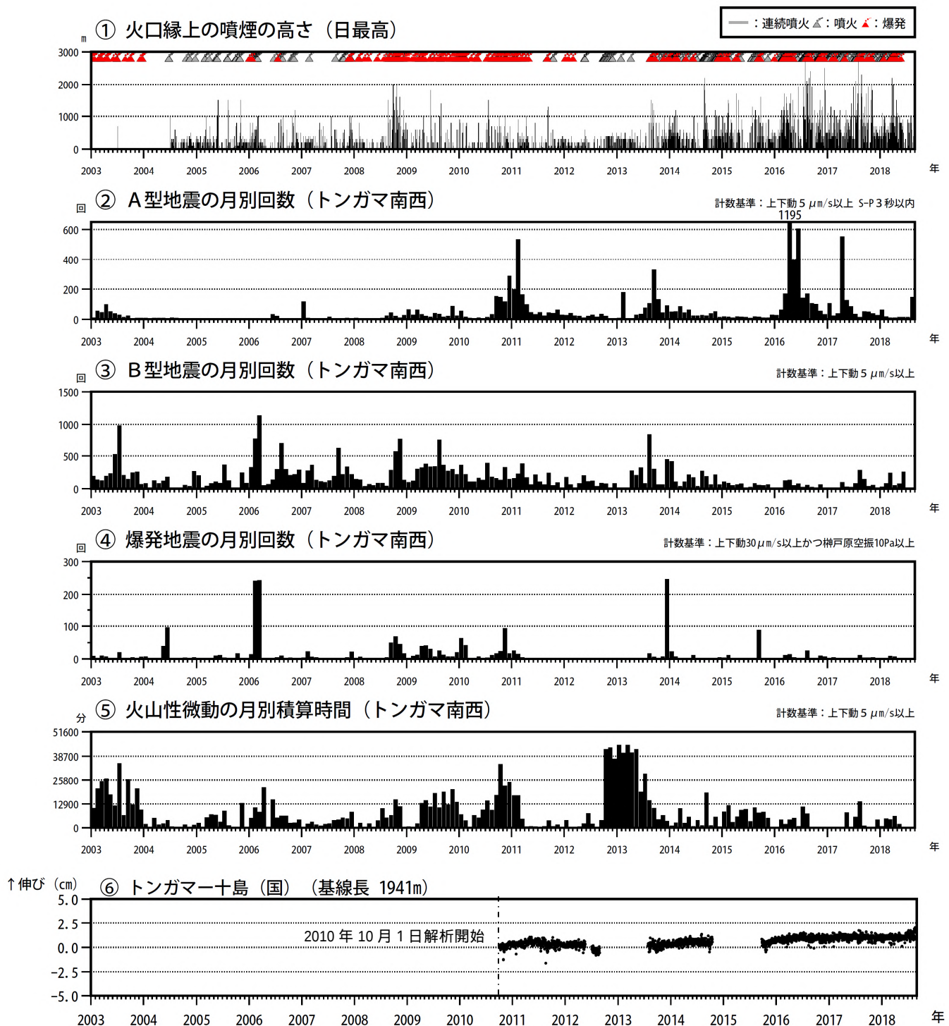
図 2 諏訪之瀬島 長期の火山活動経過図（2003 年 1 月～2018 年 8 月）
