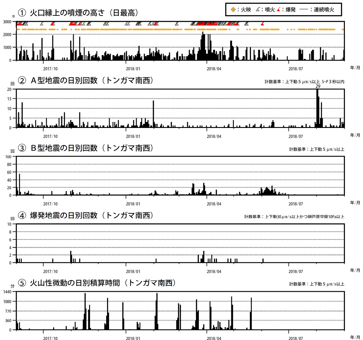
図3 諏訪之瀬島 最近の火山活動経過図（2017年8月～2018年8月）
