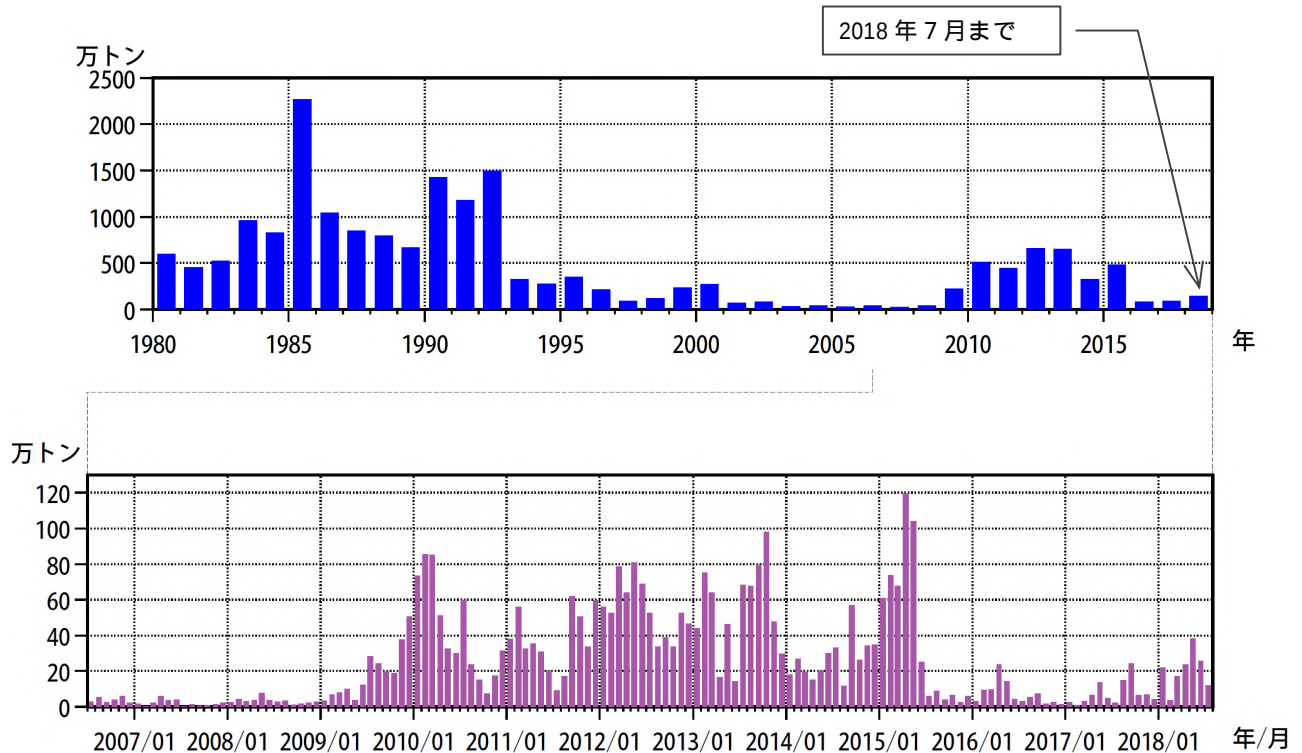
図 9 桜島 鹿児島県が実施している降灰の観測データから推定した火山灰の総噴出量 （上段：1980 年 1 月～2018 年 7 月の年別値、下段：2006 年 8 月～2018 年 7 月の月別値）
