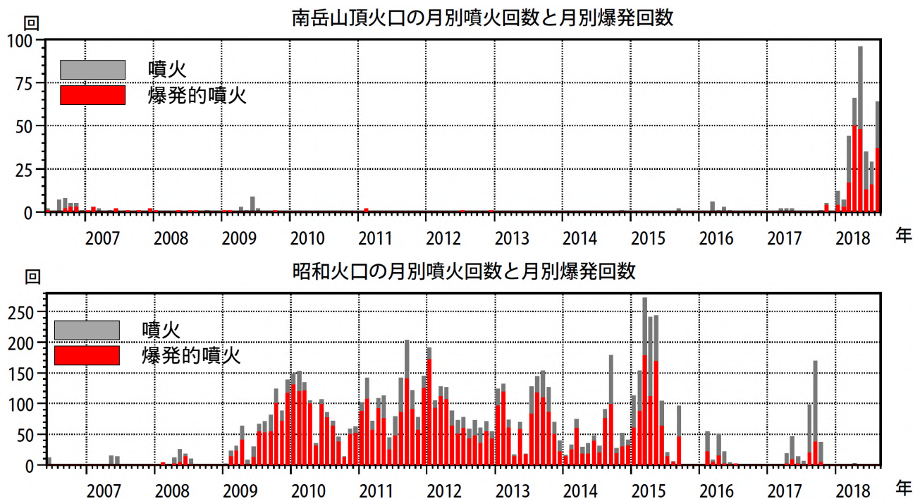
図 4 桜島 南岳山頂火口（上図）と昭和火口（下図）の月別噴火回数と月別爆発回数 （2006 年 6 月～2018 年 8 月）
