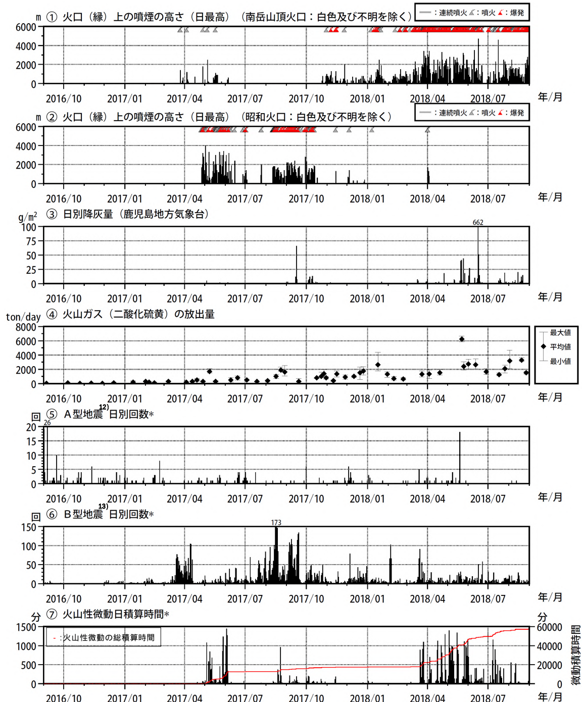
図5 桜島 最近2年間の活動経過図（2016年9月～2018年8月）
