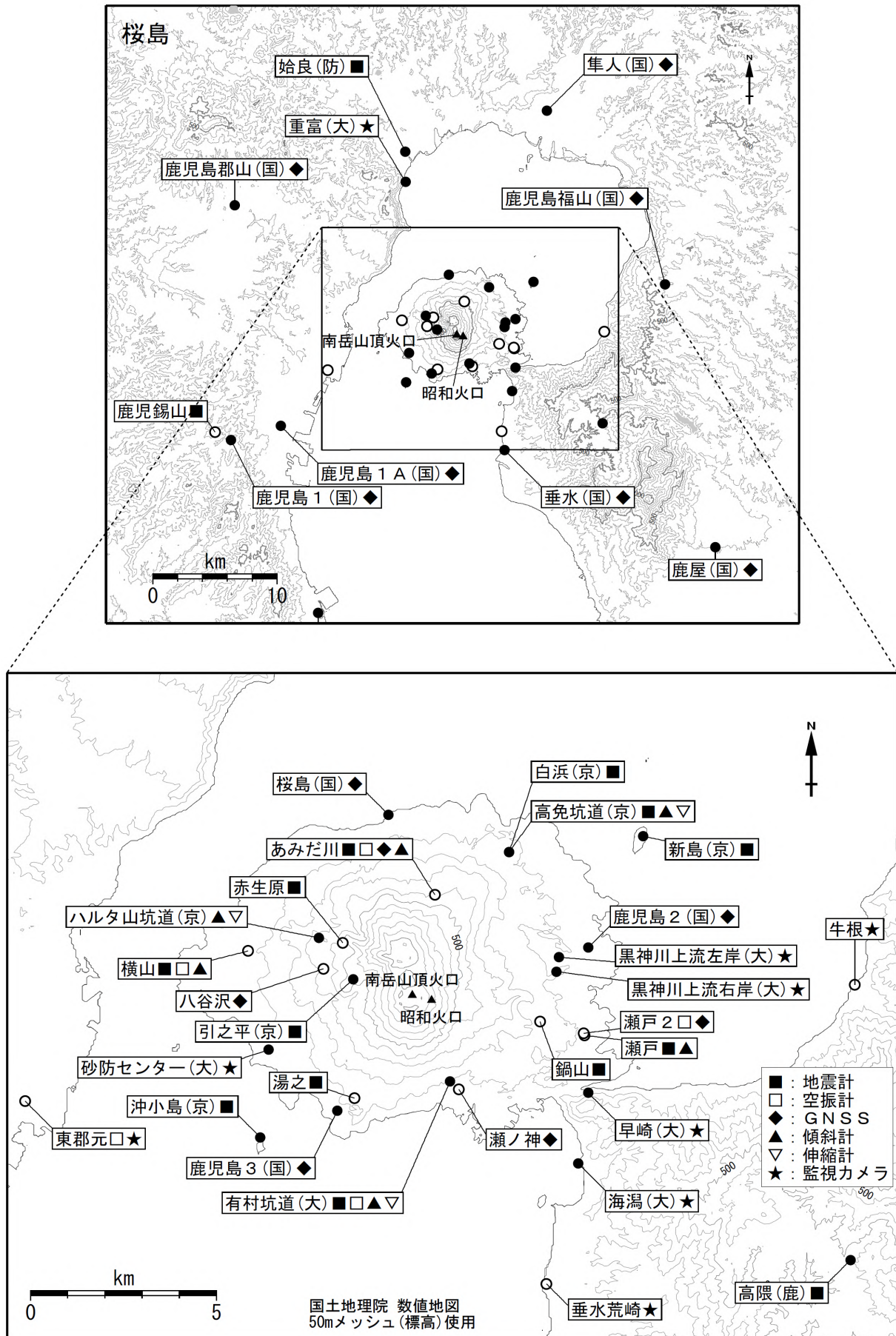
図 10 桜島 観測点配置図
