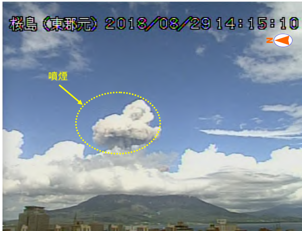
図1 桜島 29日14時09分の南岳山頂火口の噴火の状況（東郡元監視カメラ） 噴煙が火口縁上2,800mまで上がりました。
