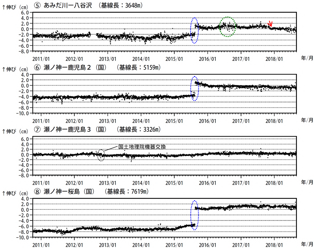
図 7-2 桜島 GNSS 連続観測による基線長変化 (2010 年 10 月 ~ 2018 年 8 月)
