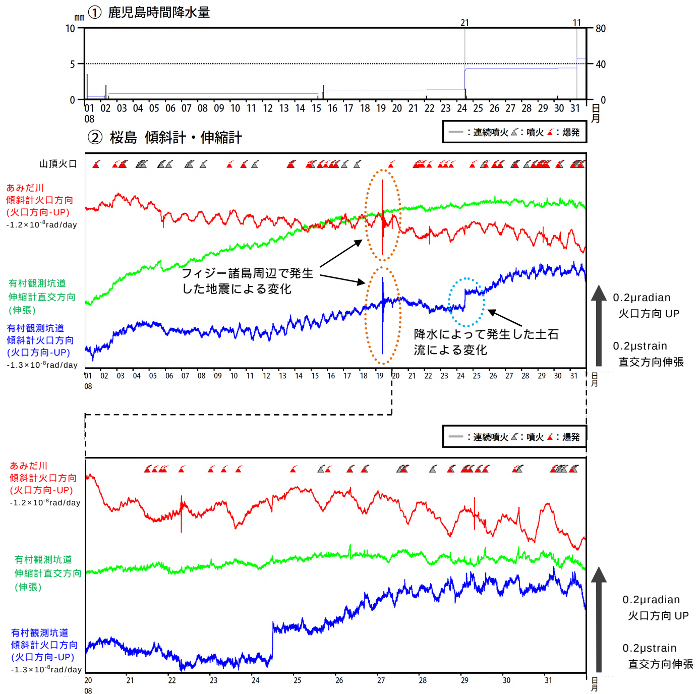
図 6 桜島 傾斜計及び伸縮計による地殻変動の状況（2018 年 8 月 1 日～8 月 31 日）
