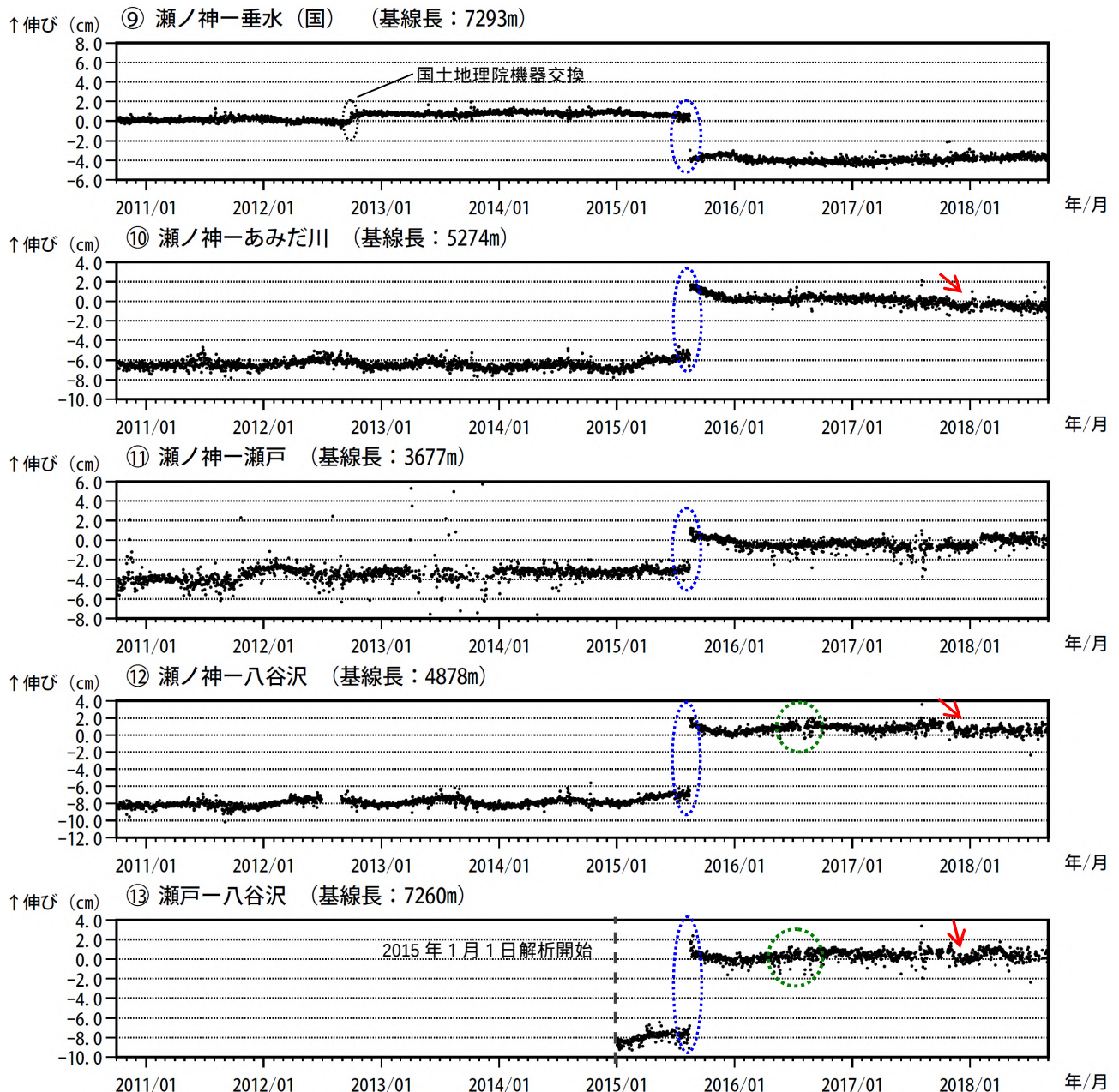
図 7-3 桜島 GNSS 連続観測による基線長変化 (2010 年 10 月 ~ 2018 年 8 月)
