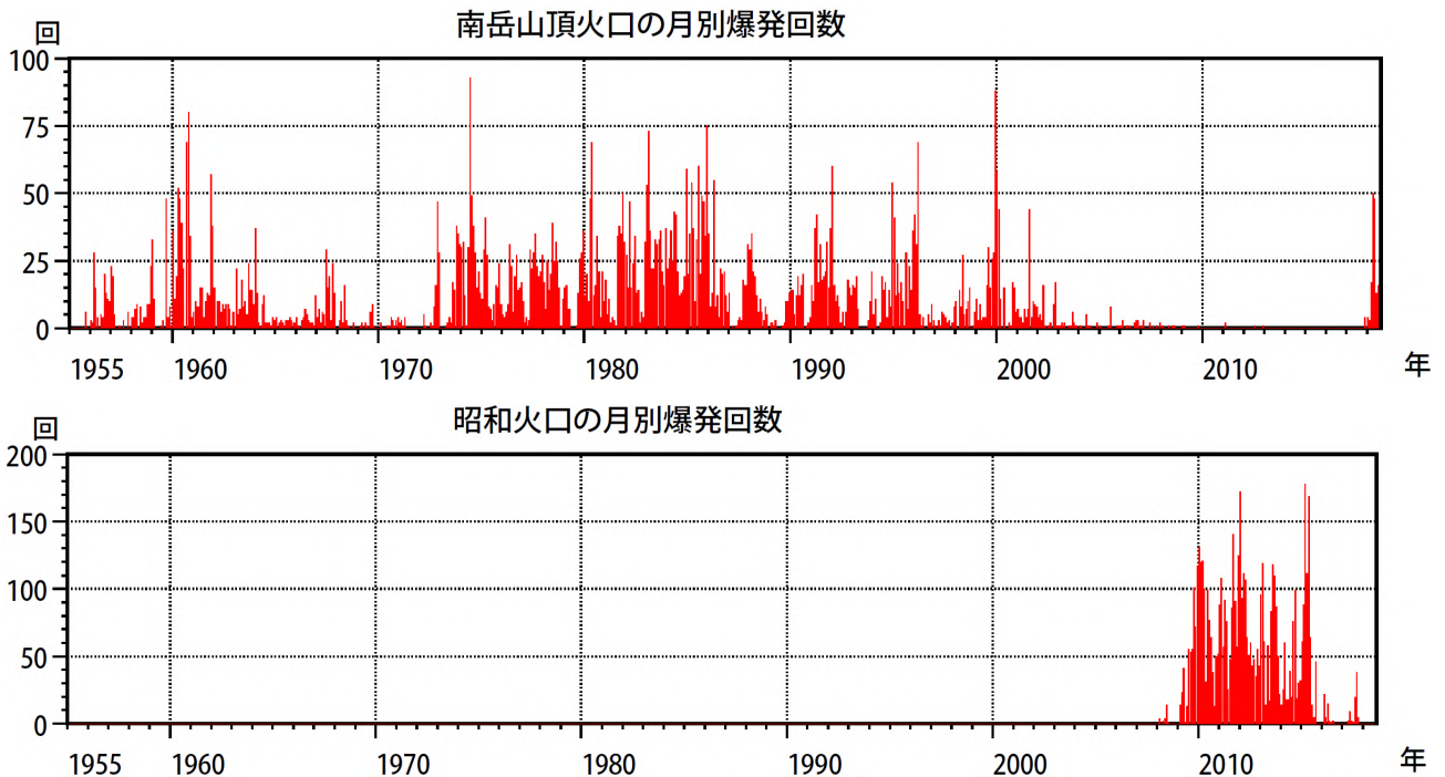
図 3 桜島 南岳山頂火口（上図）と昭和火口（下図）の月別爆発回数 （1955 年 1 月～2018 年 8 月）
