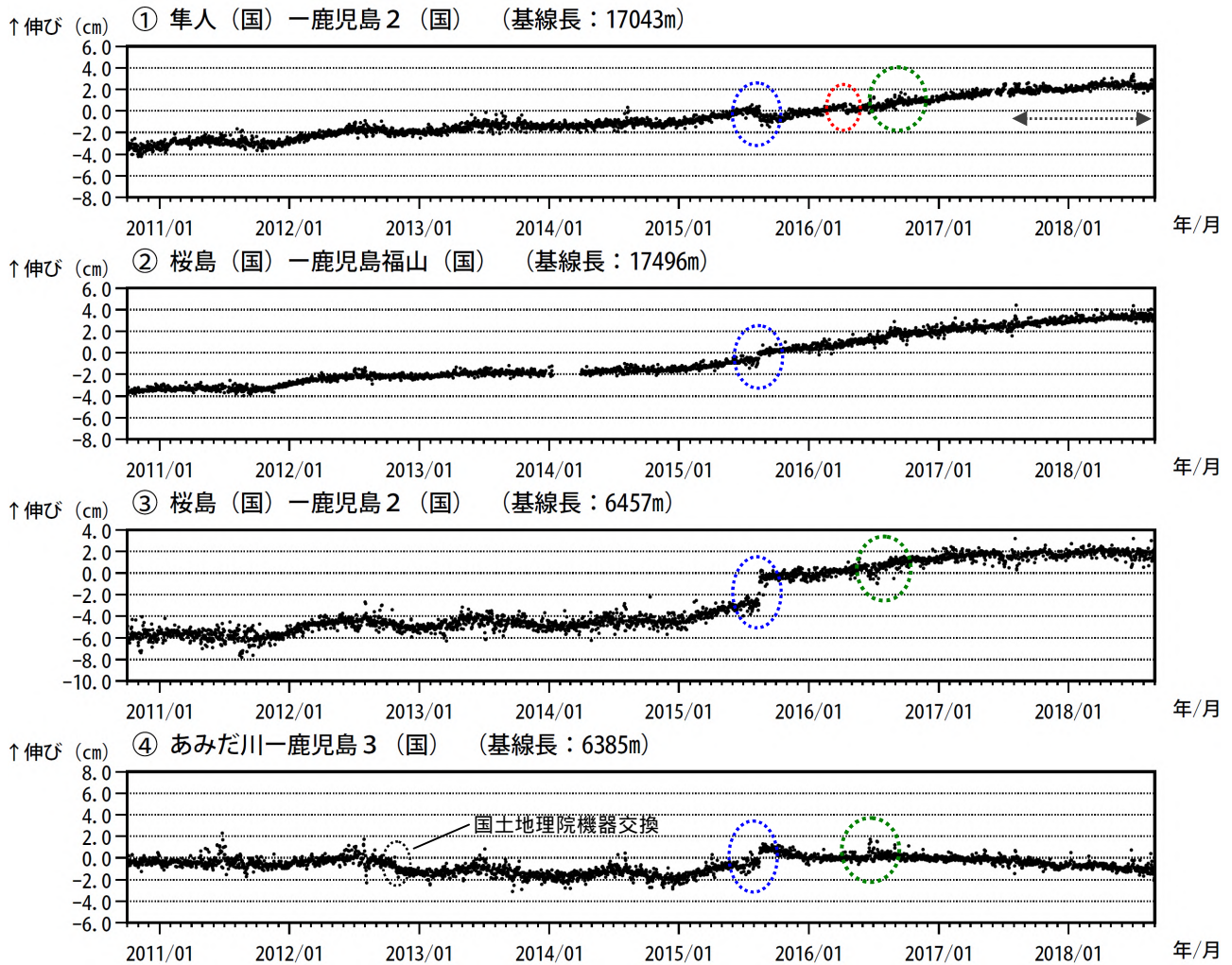
図 7-1 桜島 GNSS 連続観測による基線長変化（2010 年 10 月～2018 年 8 月）
