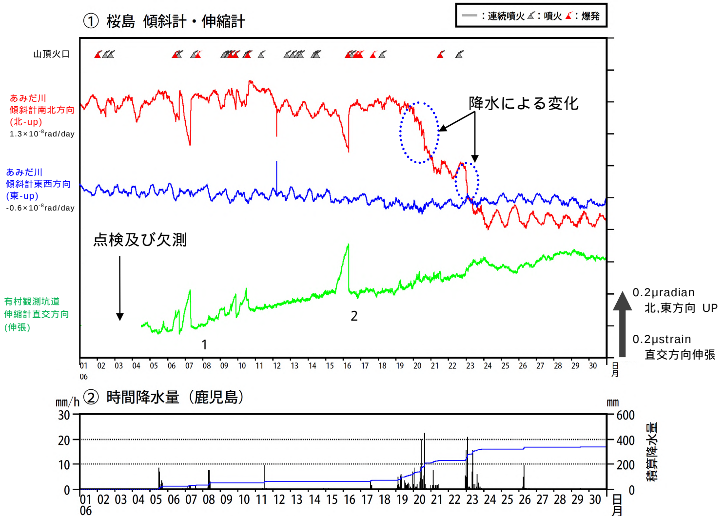
図 9 桜島 傾斜計及び伸縮計による地殻変動の状況（2018 年 6 月 1 日～6 月 30 日）
