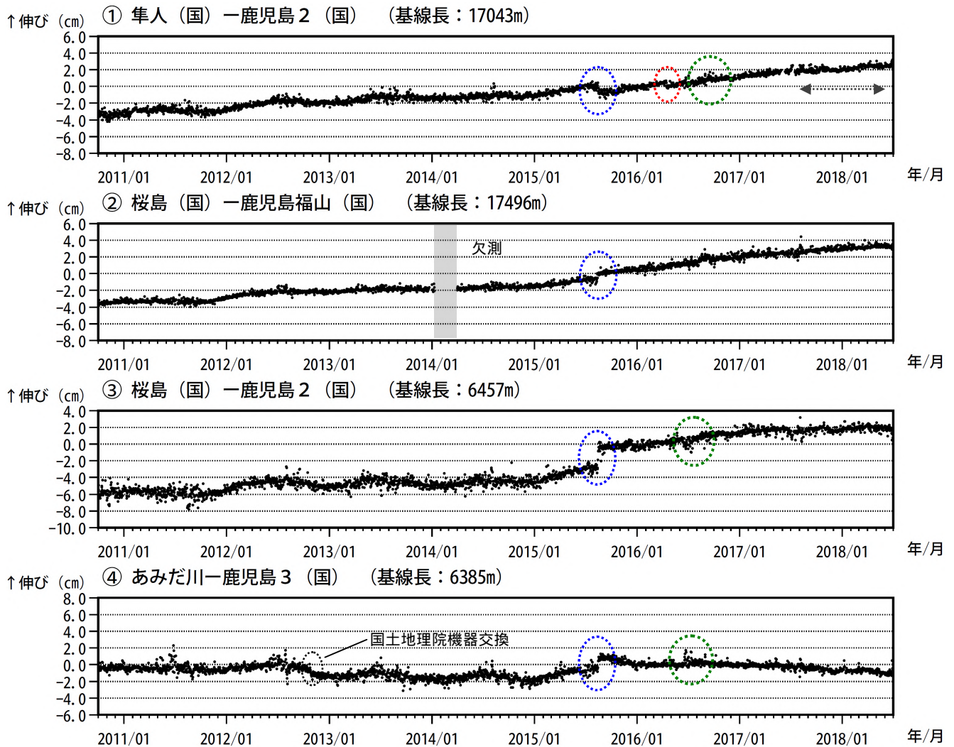
図 10-1 桜島 GNSS 連続観測による基線長変化 (2010 年 10 月 ~ 2018 年 6 月)
