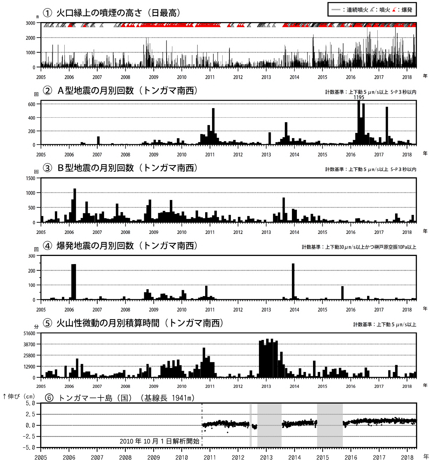
図 3 諏訪之瀬島 長期の火山活動経過図（2005 年 1 月～2018 年 4 月）
