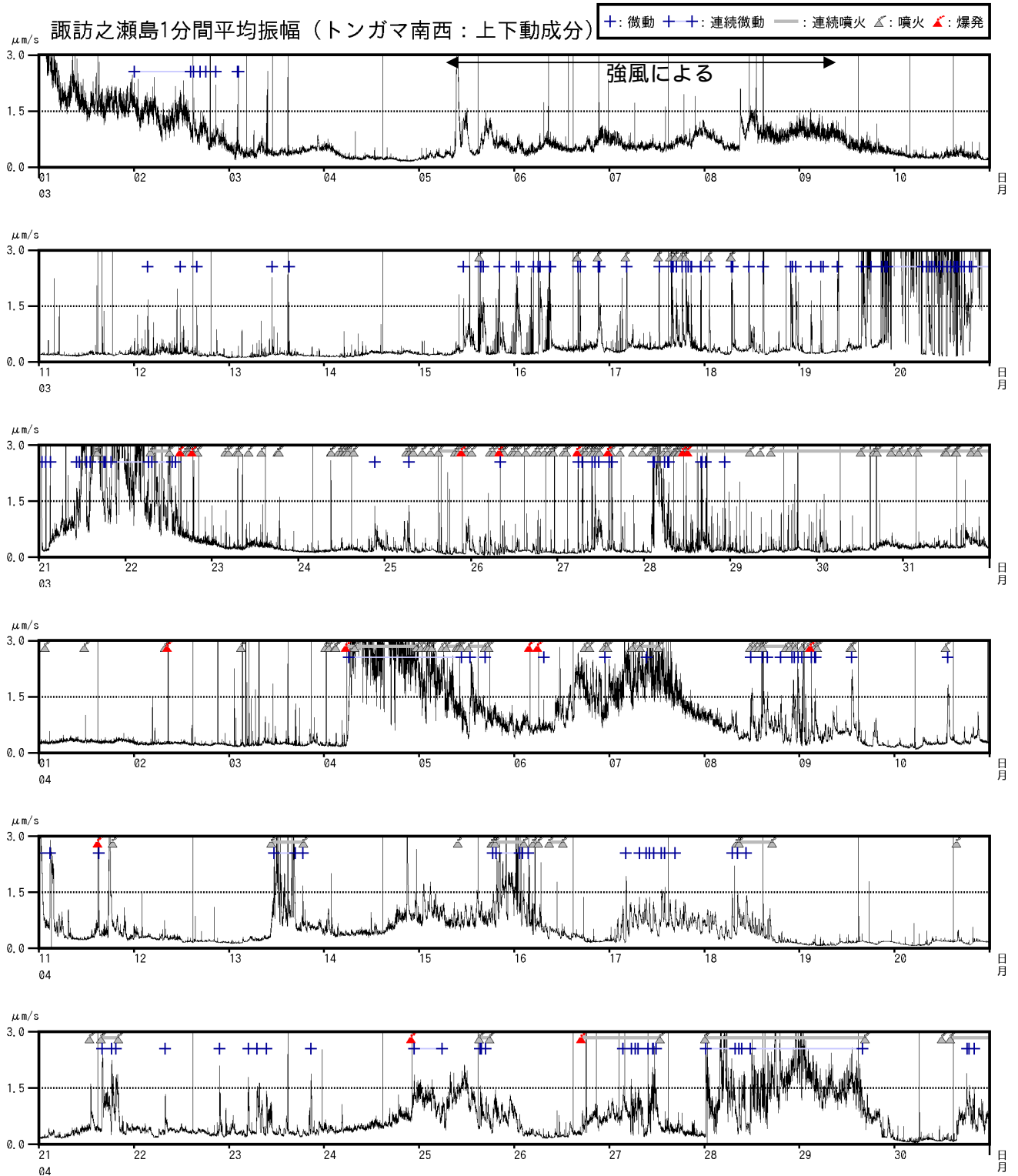
図 5 諏訪之瀬島 1 分間平均振幅の時間変化（トンガマ南西観測点上下動成分、2018 年 3 月～ 4 月）
