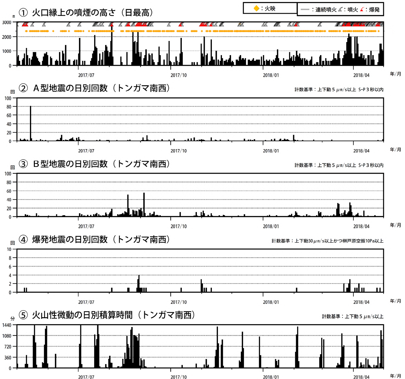
図4 諏訪之瀬島 最近の火山活動経過図（2017年5月～2018年4月）
