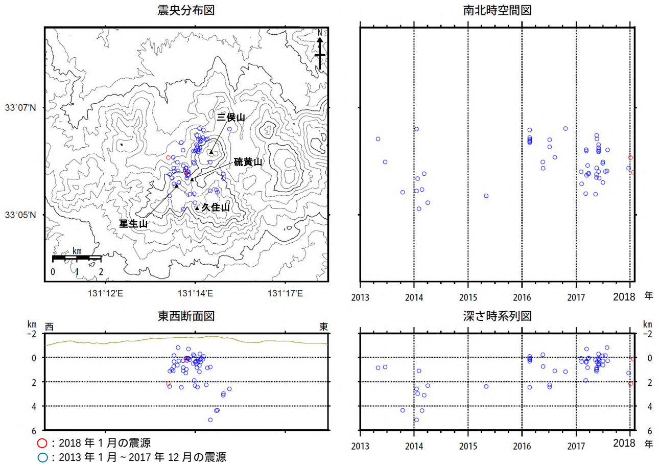
図 4 九重山 震源分布図（2013 年 1 月 ~ 2018 年 1 月）
