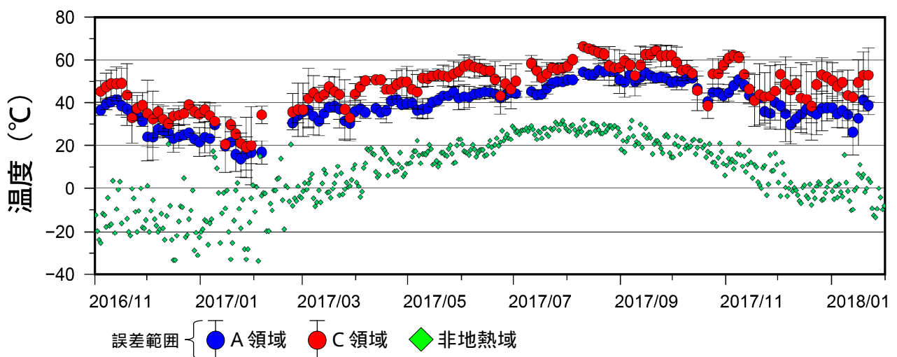
図 2-2 九重山 星生山北尾根赤外熱映像装置による日別最高温度の 7 日間移動平均値（2016 年 11 月～2018 年 1 月）
