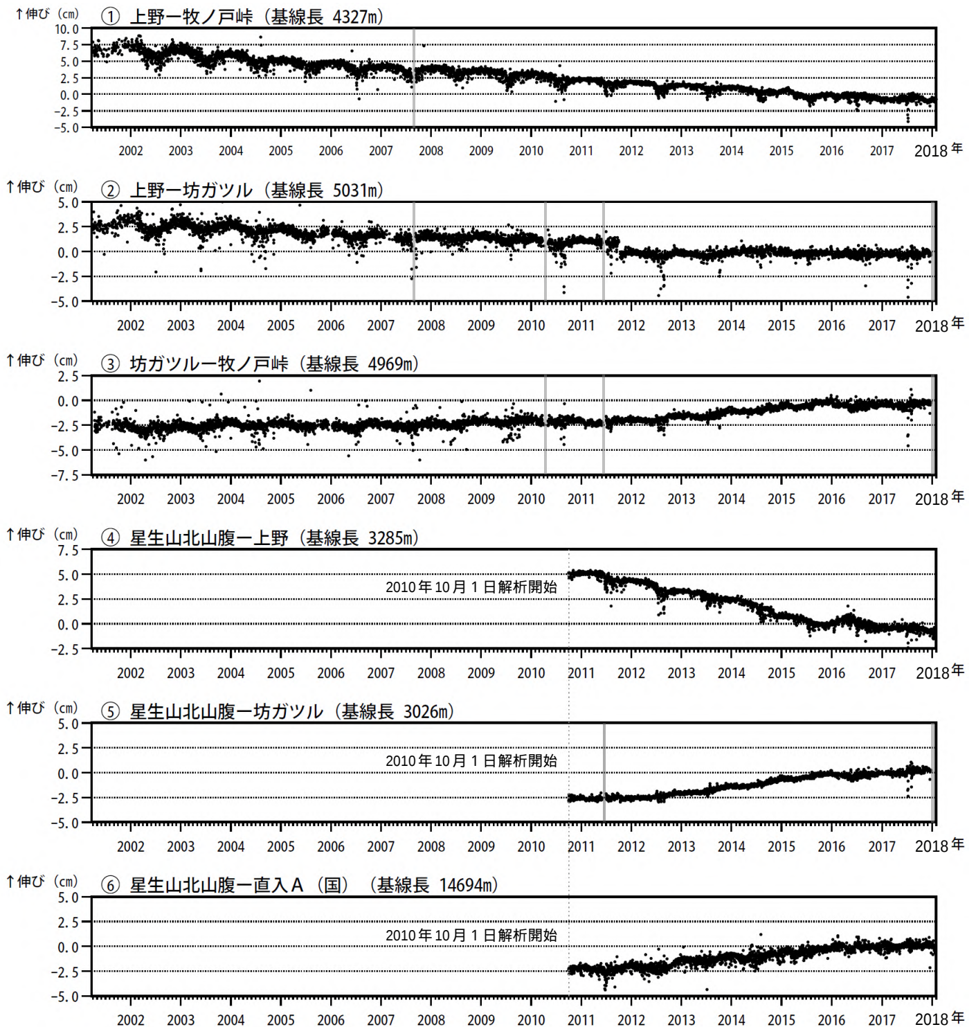
図 5 九重山 GNSS 連続観測による基線長変化 (2001 年 3 月 ~ 2018 年 1 月)
