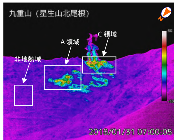
図 2-1 九重山 地熱域の状況（1 月 31 日、星生山北尾根赤外熱映像装置による）
