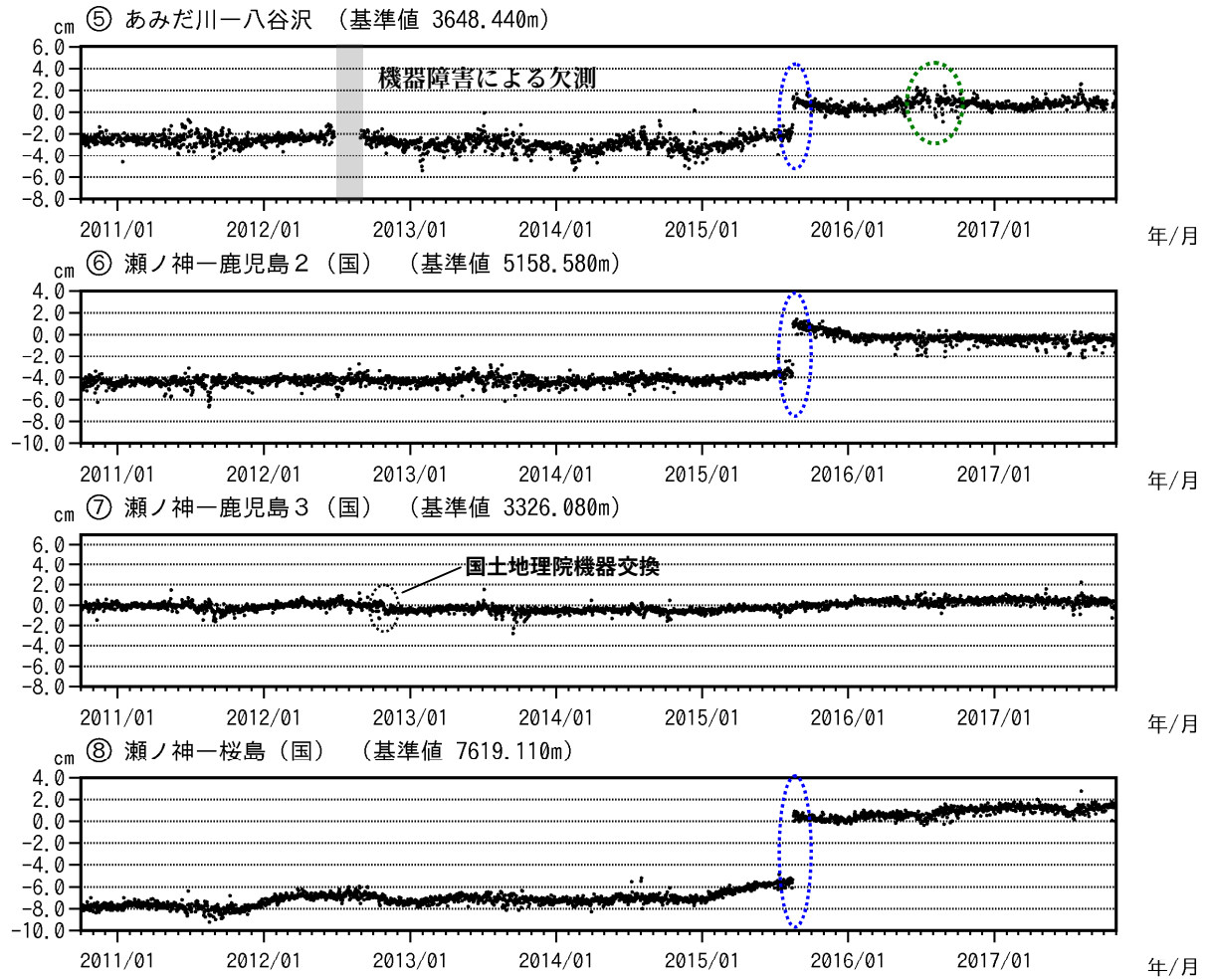
図 11-2 桜島 GNSS 連続観測による基線長変化（2010 年 10 月～2017 年 10 月）
