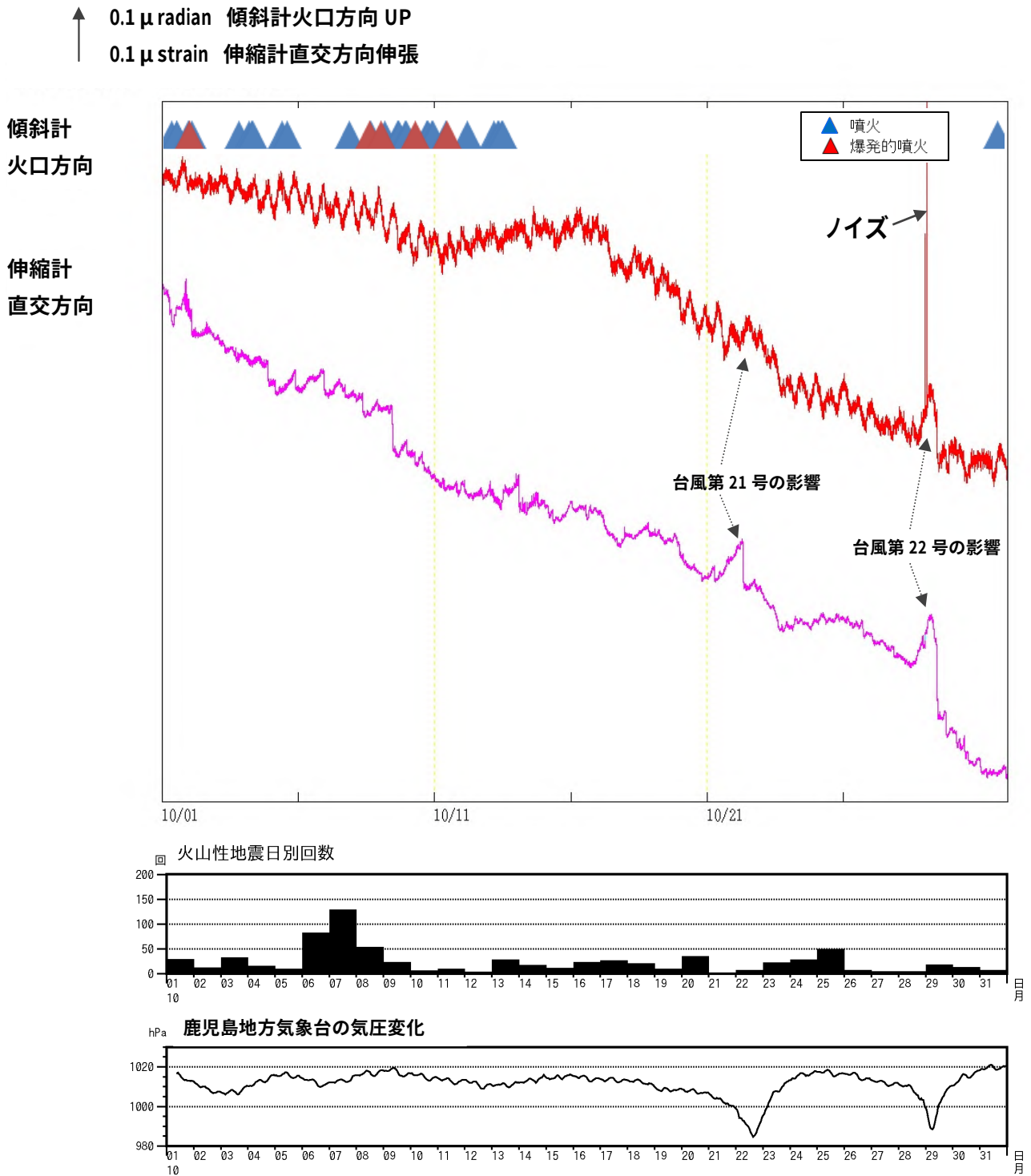
図 10 桜島 有村観測坑道の地殻変動と火山性地震の回数、気圧の状況（2017 年 10 月）
