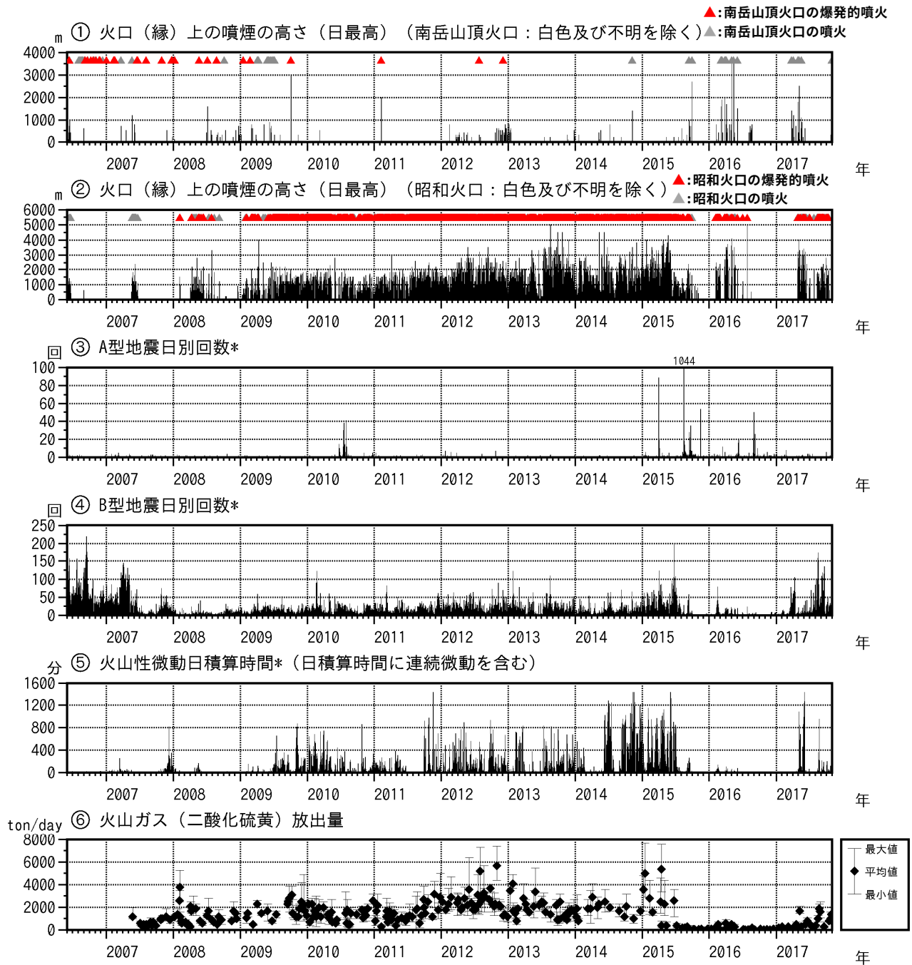
図 8 桜島 昭和火口噴火活動再開（2006 年 6 月）以降の活動経過図
