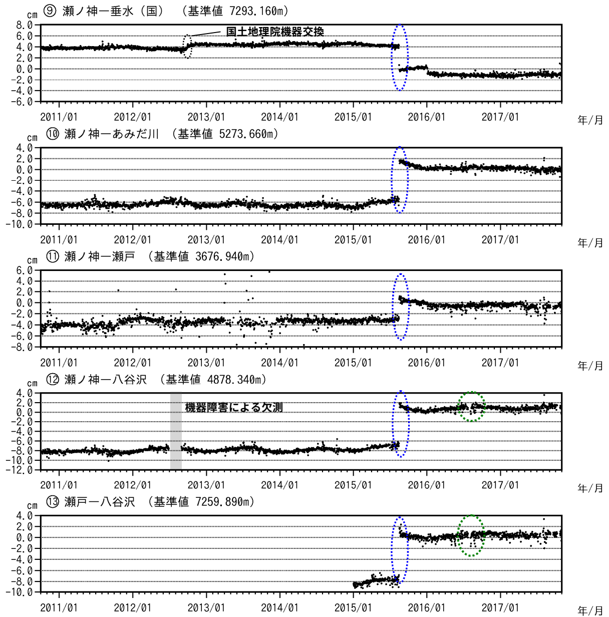
図 11-3 桜島 GNSS 連続観測による基線長変化（2010 年 10 月～2017 年 10 月）
