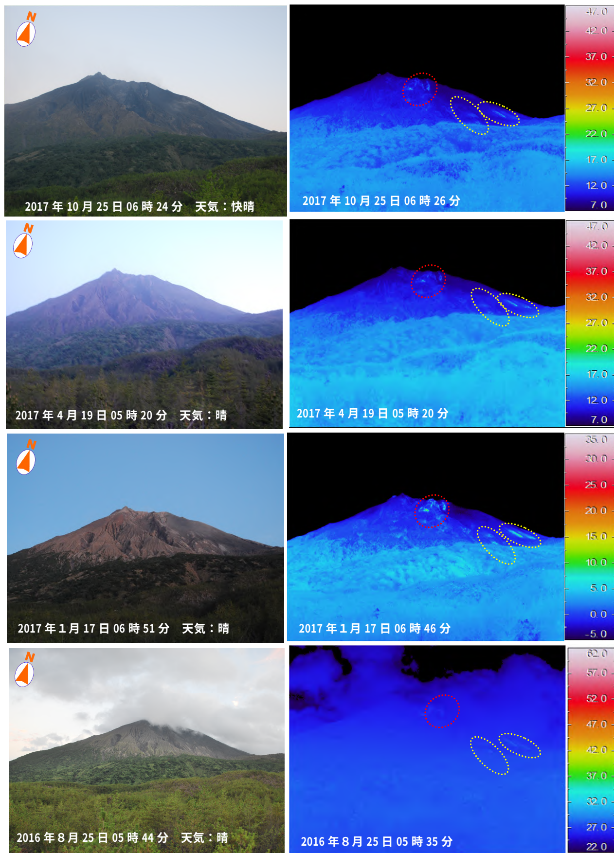
図5 桜島 可視画像及び地表面温度分布（有村町から観測）
