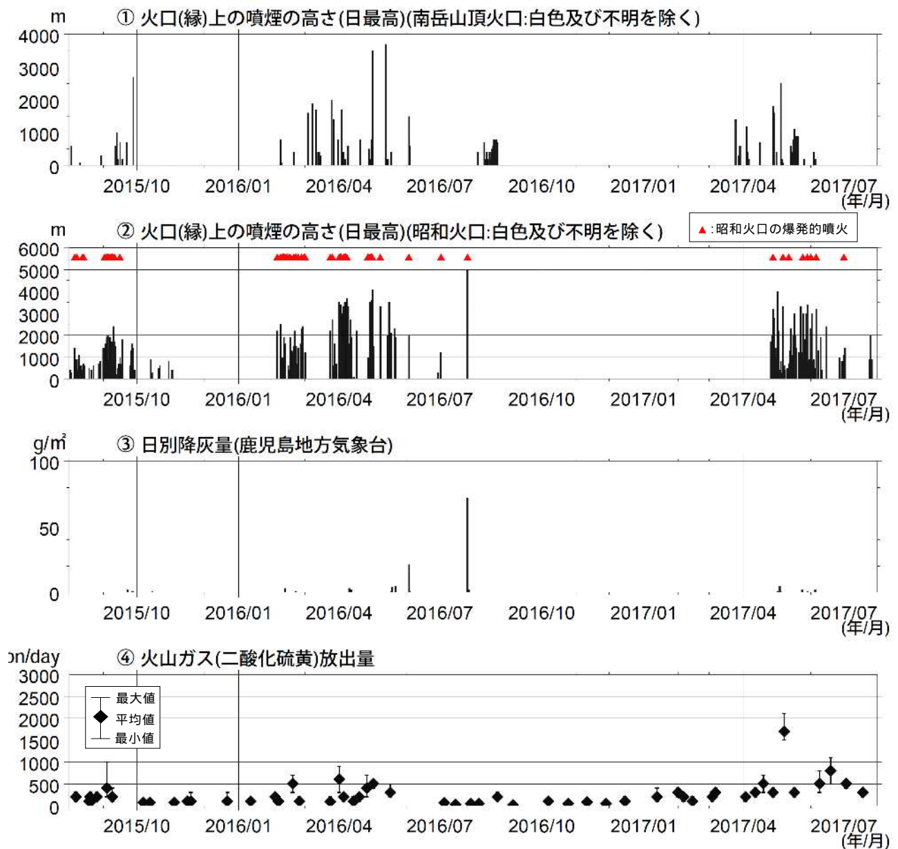
図 4 桜島 最近 2 年間の活動経過図（2015 年 8 月～2017 年 7 月）
