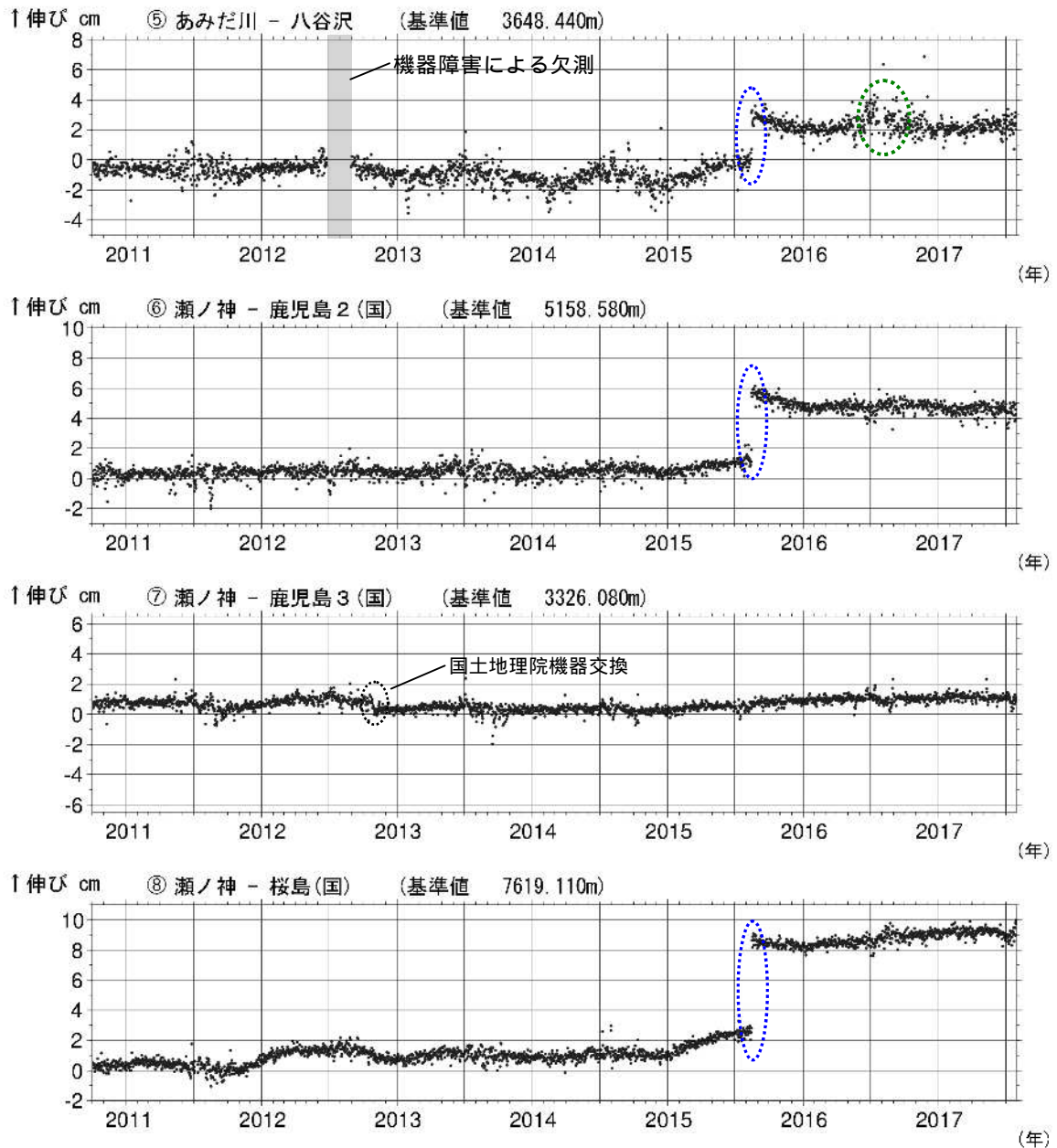
図 8-2 桜島 GNSS 連続観測による基線長変化（2010 年 10 月～2017 年 7 月）
