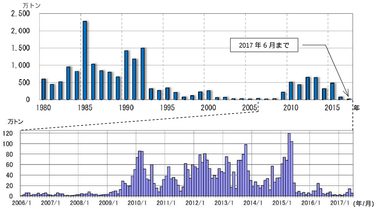
図 10 桜島 鹿児島県が実施している降灰の観測データから推定した火山灰の総噴出量 （1980 年 1 月～2017 年 6 月、上段：年別値 下段：月別値）
