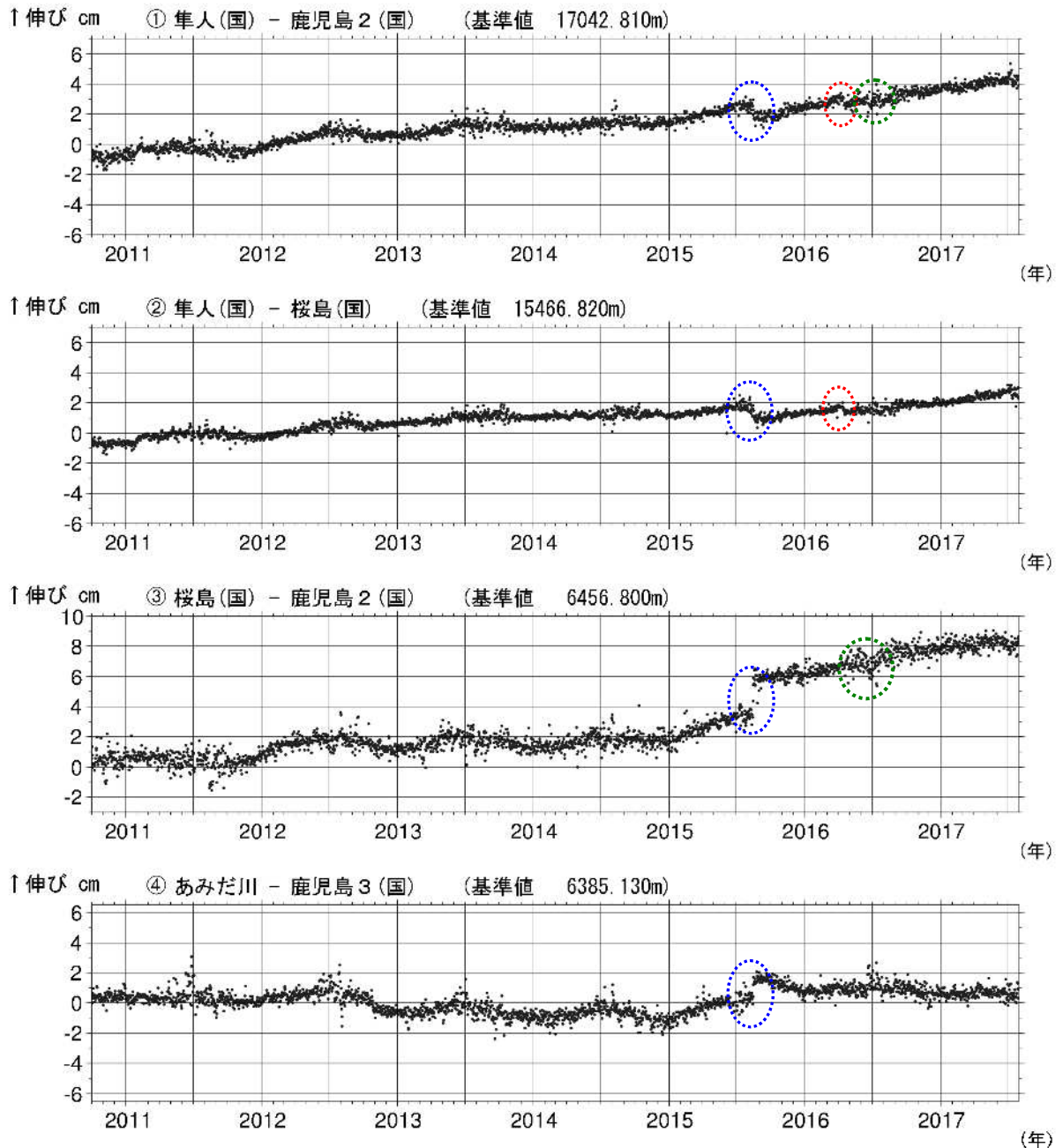
図 8-1 桜島 GNSS 連続観測による基線長変化（2010 年 10 月～2017 年 7 月）
