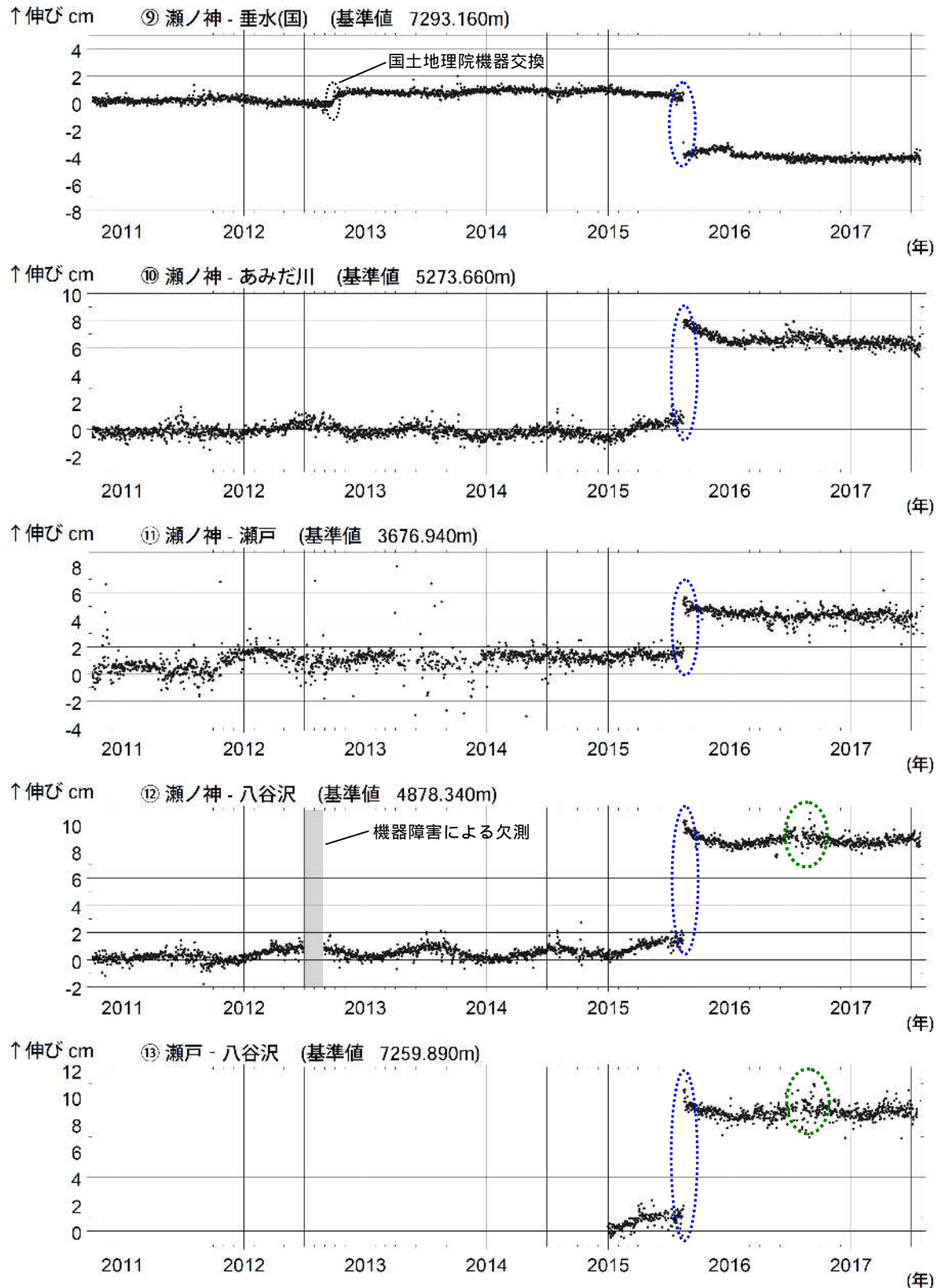
図 8-3 桜島 GNSS 連続観測による基線長変化（2010 年 10 月～2017 年 7 月）
