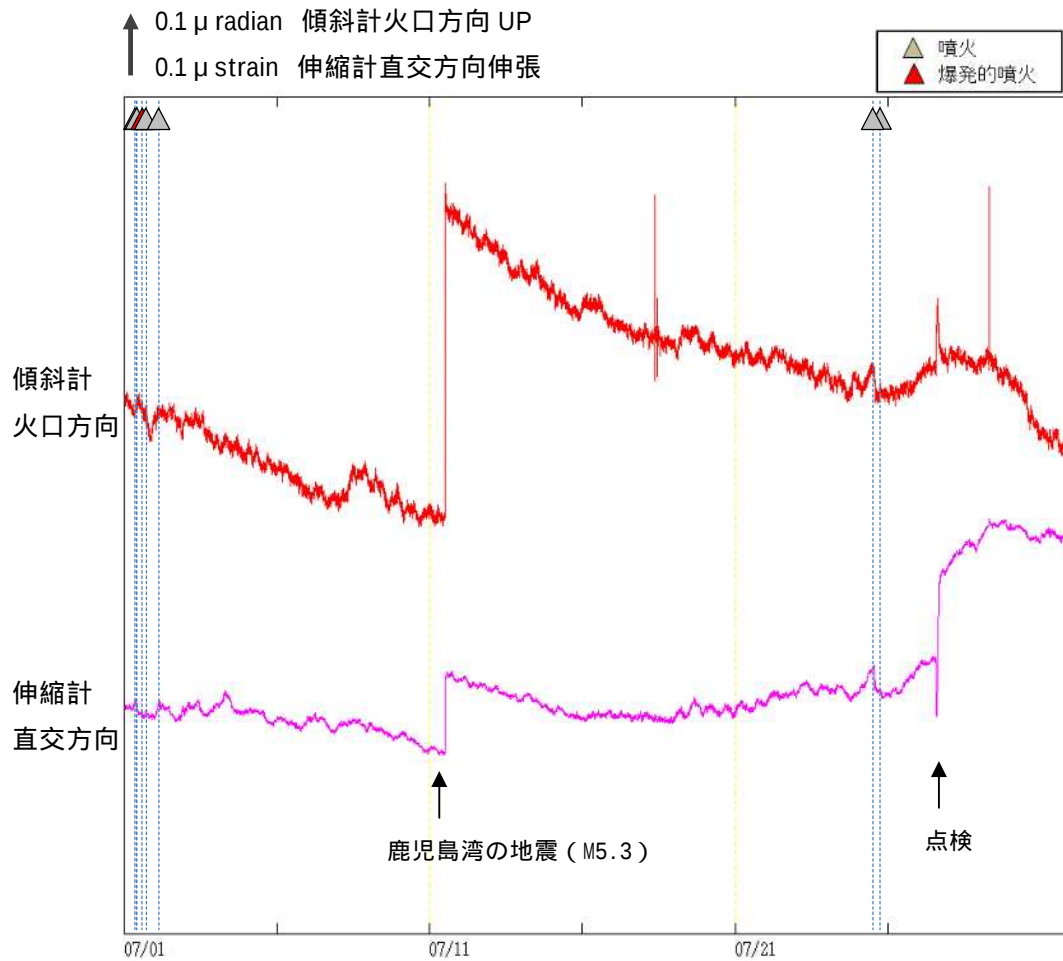
図7 桜島 有村観測坑道の傾斜計及び伸縮計の状況（2017年7月1日～7月31日）
