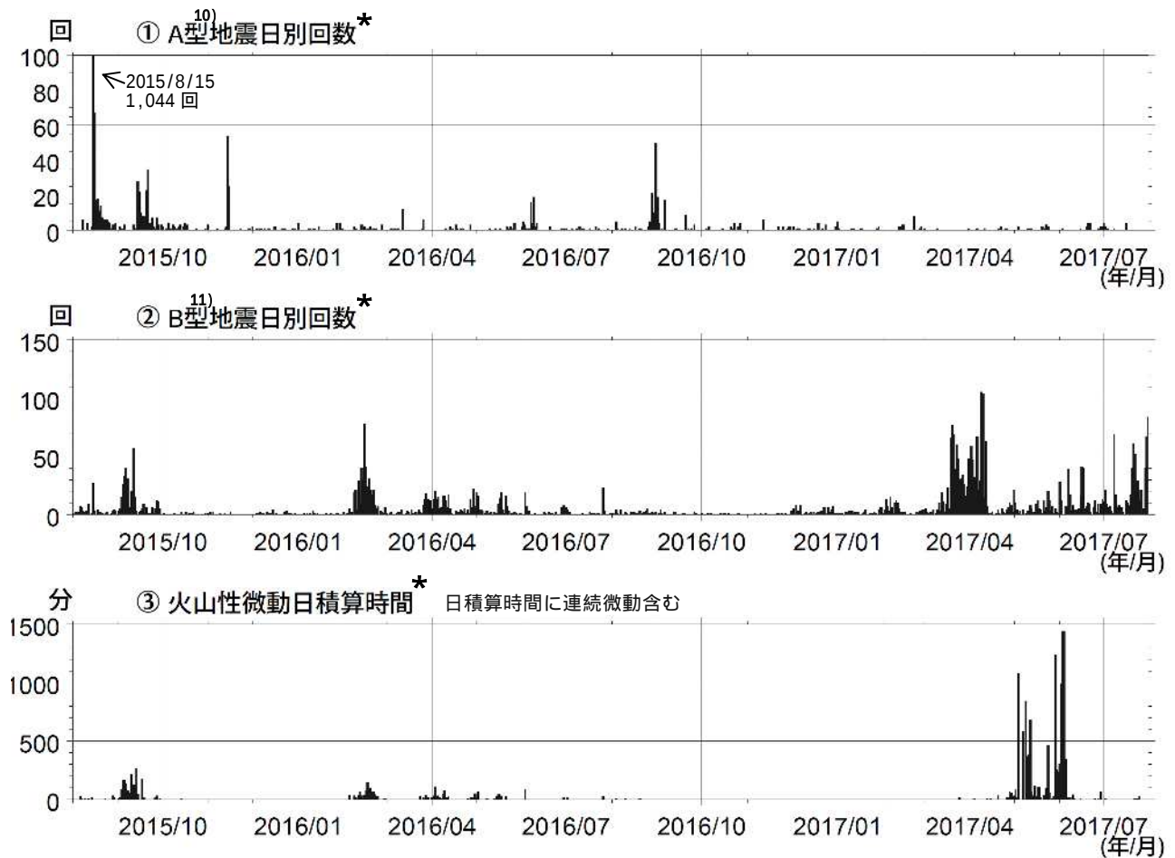
図3 桜島 最近2年間の活動経過図（2015年8月～2017年7月）
