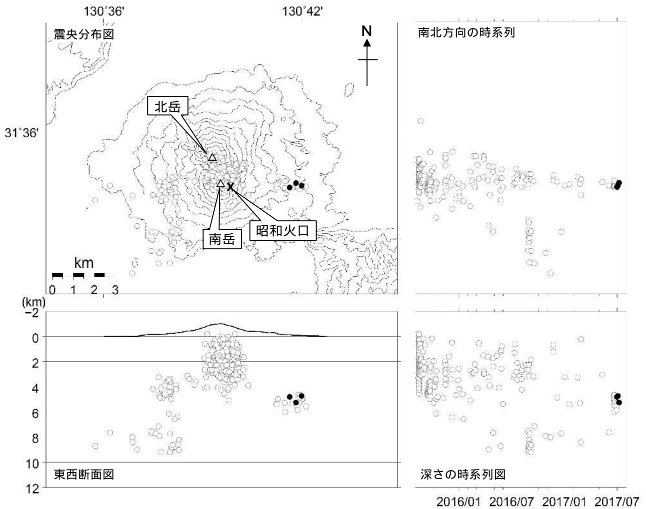
図 6 桜島 火山性地震の震源分布図（2015 年 8 月～2017 年 7 月）
