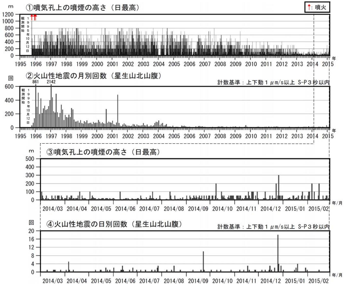
図 3 九重山 火山活動経過図（1995 年 11 月～2015 年 2 月）
