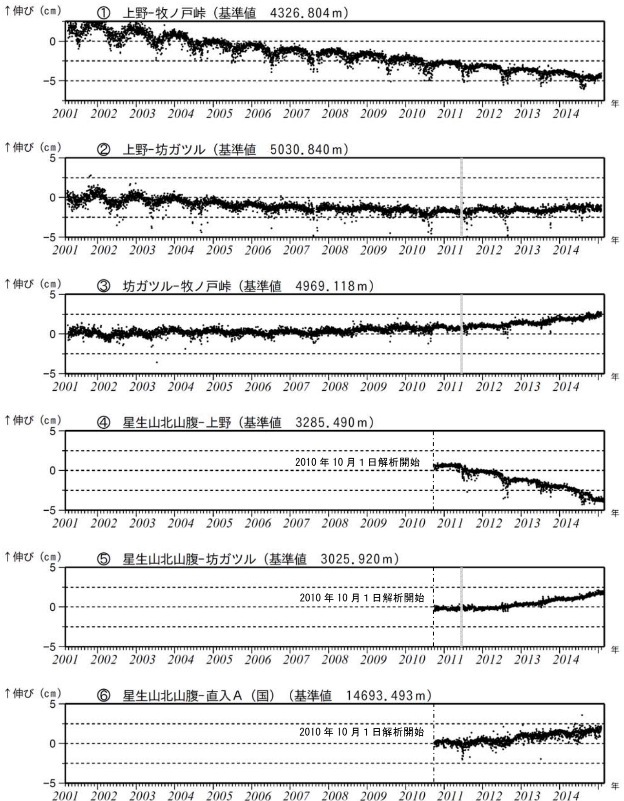
図5 九重山 GNSS 連続観測による基線長変化 (2001年3月～2015年2月)
